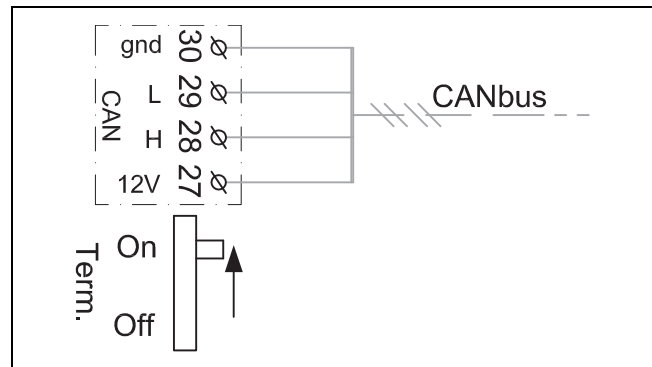
Bild 32 CAN-BUS-Terminierung
