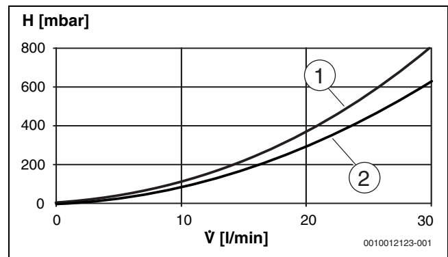
Bild 7 Druckverlust Sekundärseite
