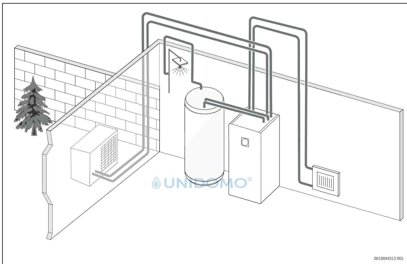
Bild 7 Außeneinheit WLW MB/MBE+ AR, Inneneinheit Logatherm WLW176i.2 /WLW186i.2 TP70 mit integriertem Pufferspeicher
