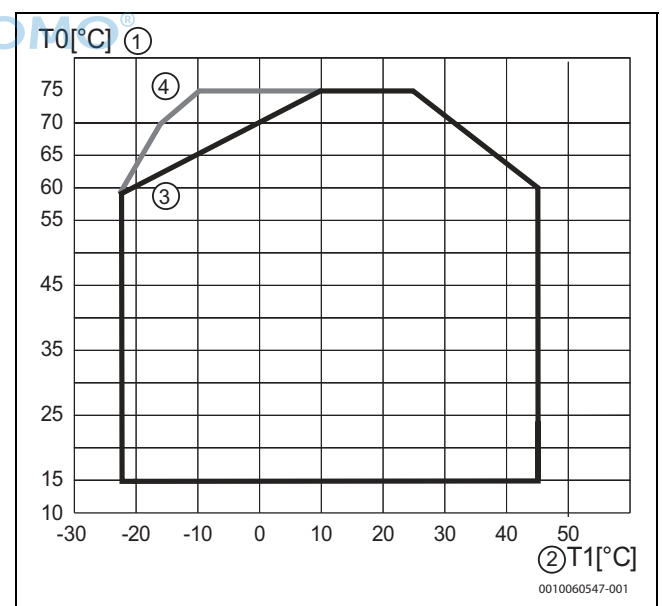
Bild 4 Wärmepumpe im Heizbetrieb ohne elektrischen Zuheizter
