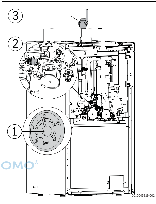
Bild 14 Position der Komponenten für Inspektion und Wartung
