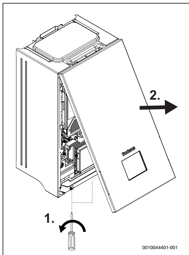
Bild 15 Frontplatten abnehmen
