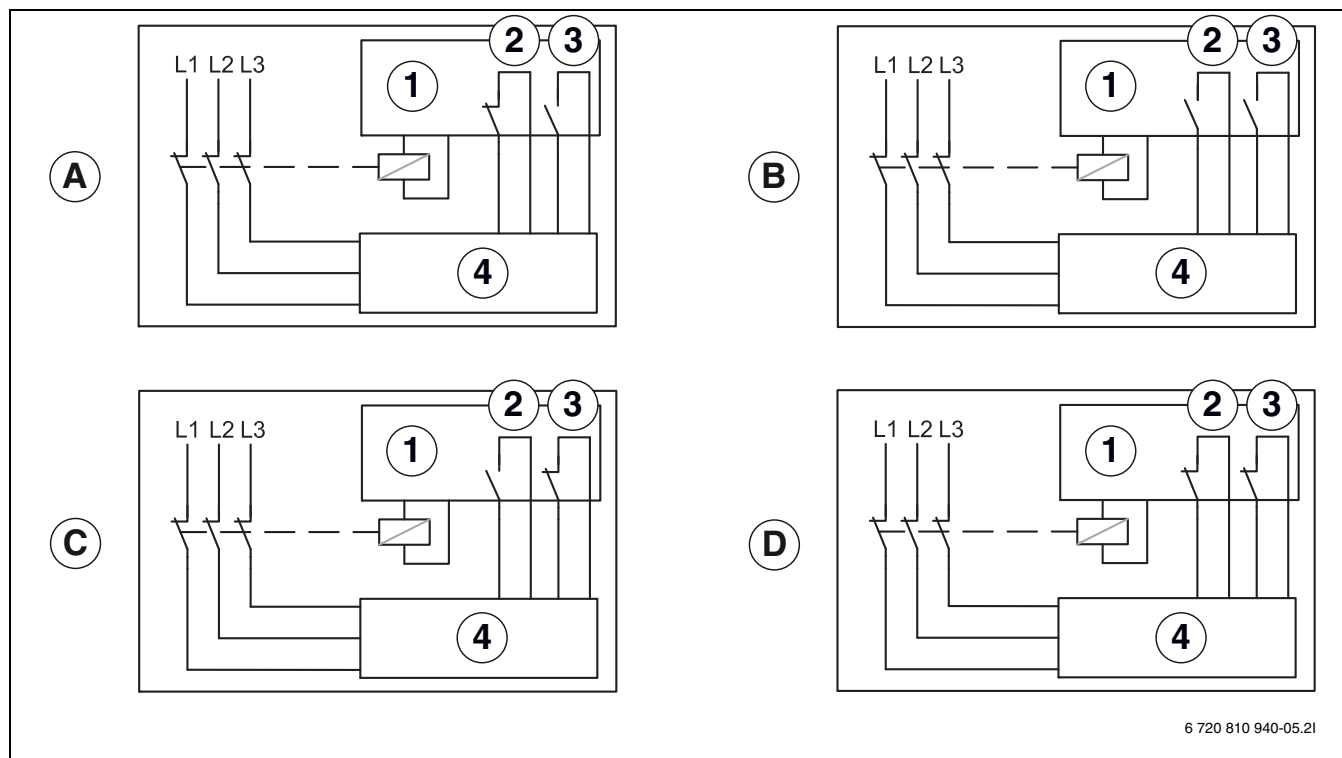
Bild 42 Anschlussplan für EVU-Sperre/SG
