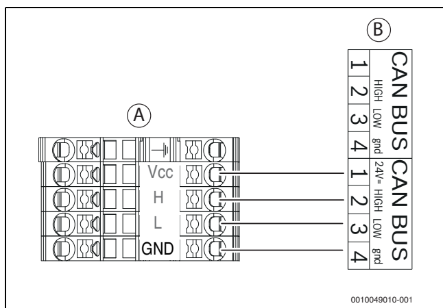
Bild 26 CAN-BUS Wärmepumpe - Inneneinheit
