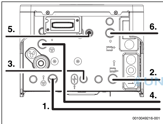
Bild 19 Rohranschlüsse
