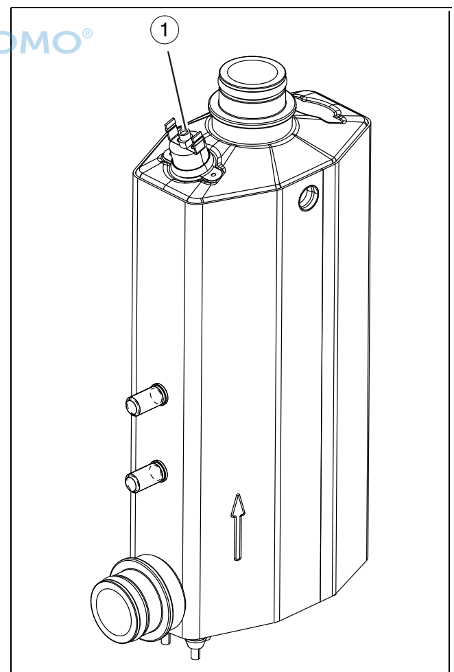
Bild 45 Elektrischer Zuheizer
