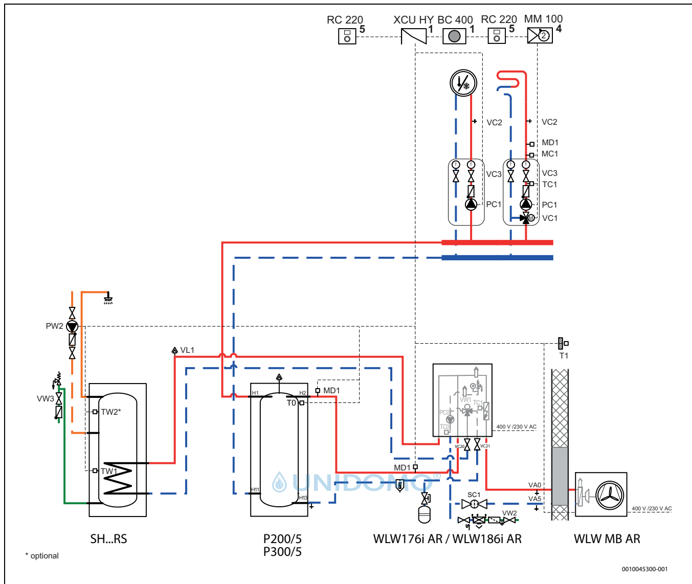
Bild 48 Wärmepumpe, zwei Heizkreise, Inneneinheit, Pufferspeicher und Warmwasserspeicher
