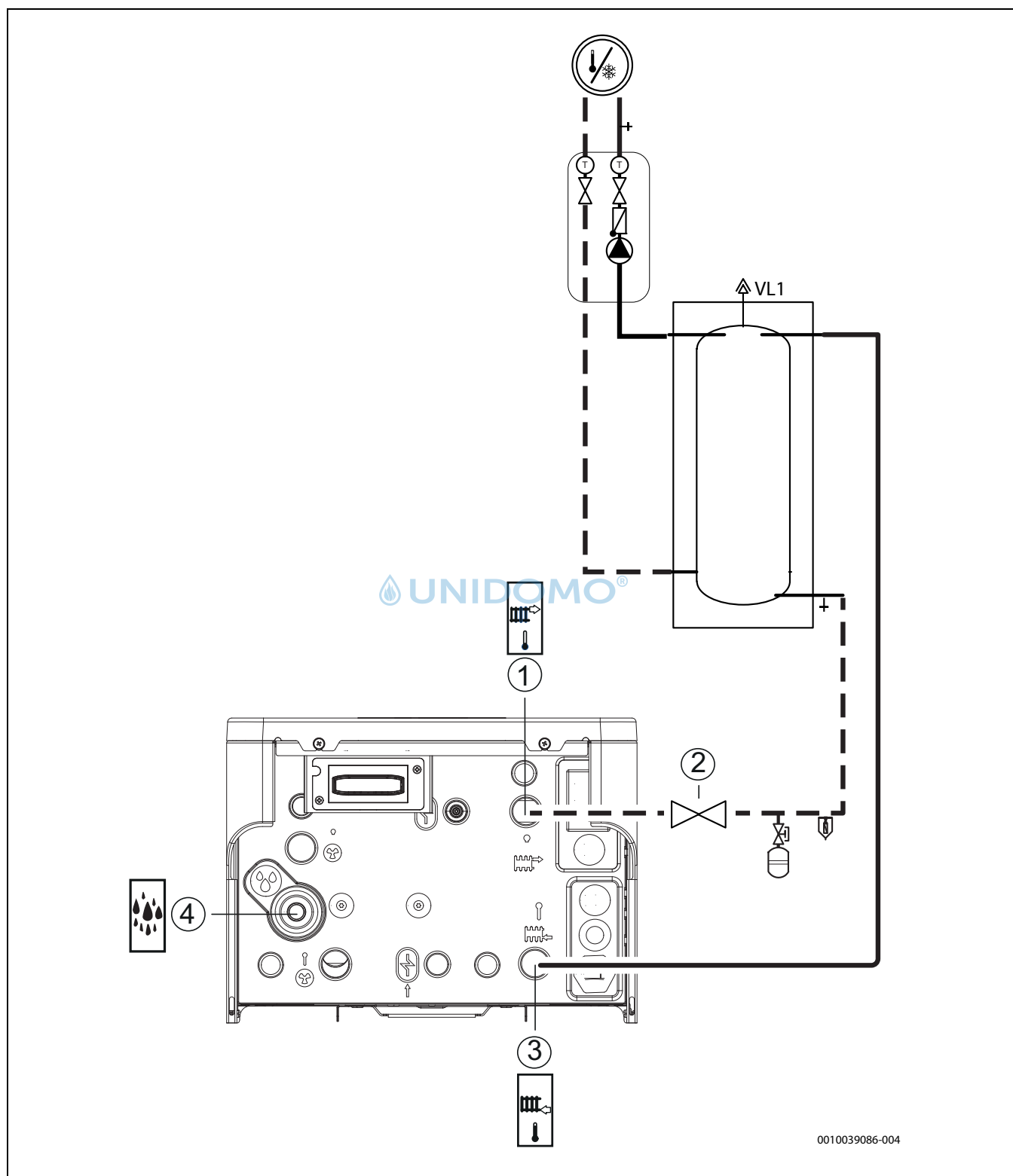
Bild 22 Anschluss der Inneneinheit an die Heizungsanlage
