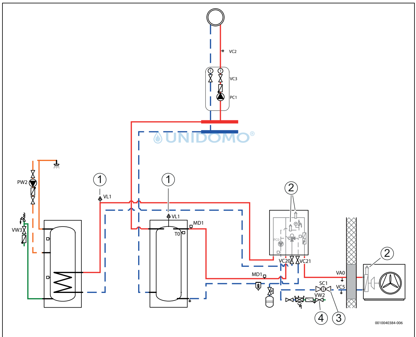
Bild 24 Inneneinheit, Wärmepumpe, Warmwasserspeicher und Heizungsanlage mit Puffer
