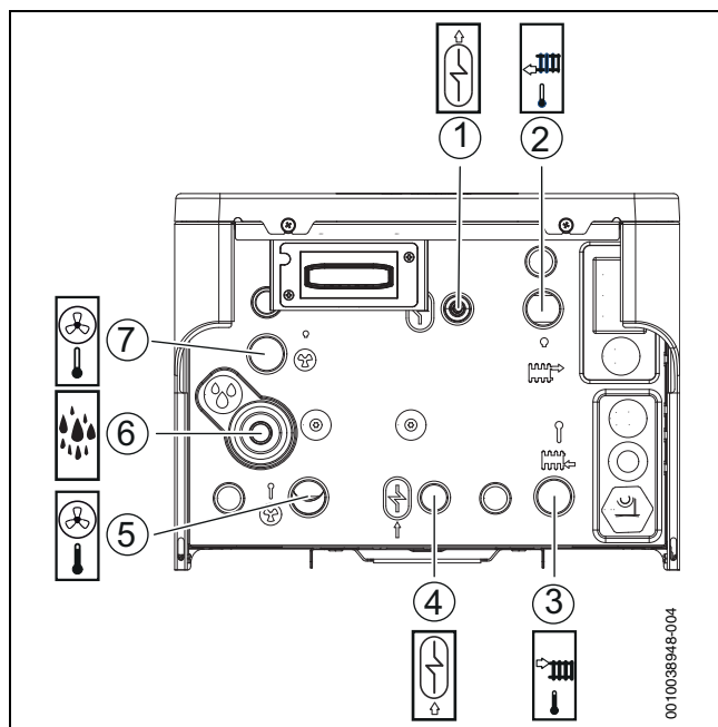
Bild 6 Rohranschlüsse
