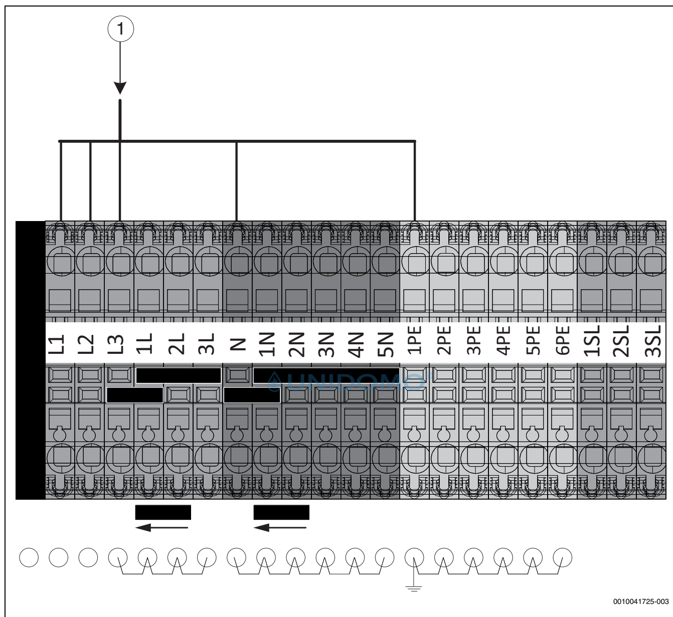
Bild 36 Elektrische Anschlüsse ohne EVU-Sperre
