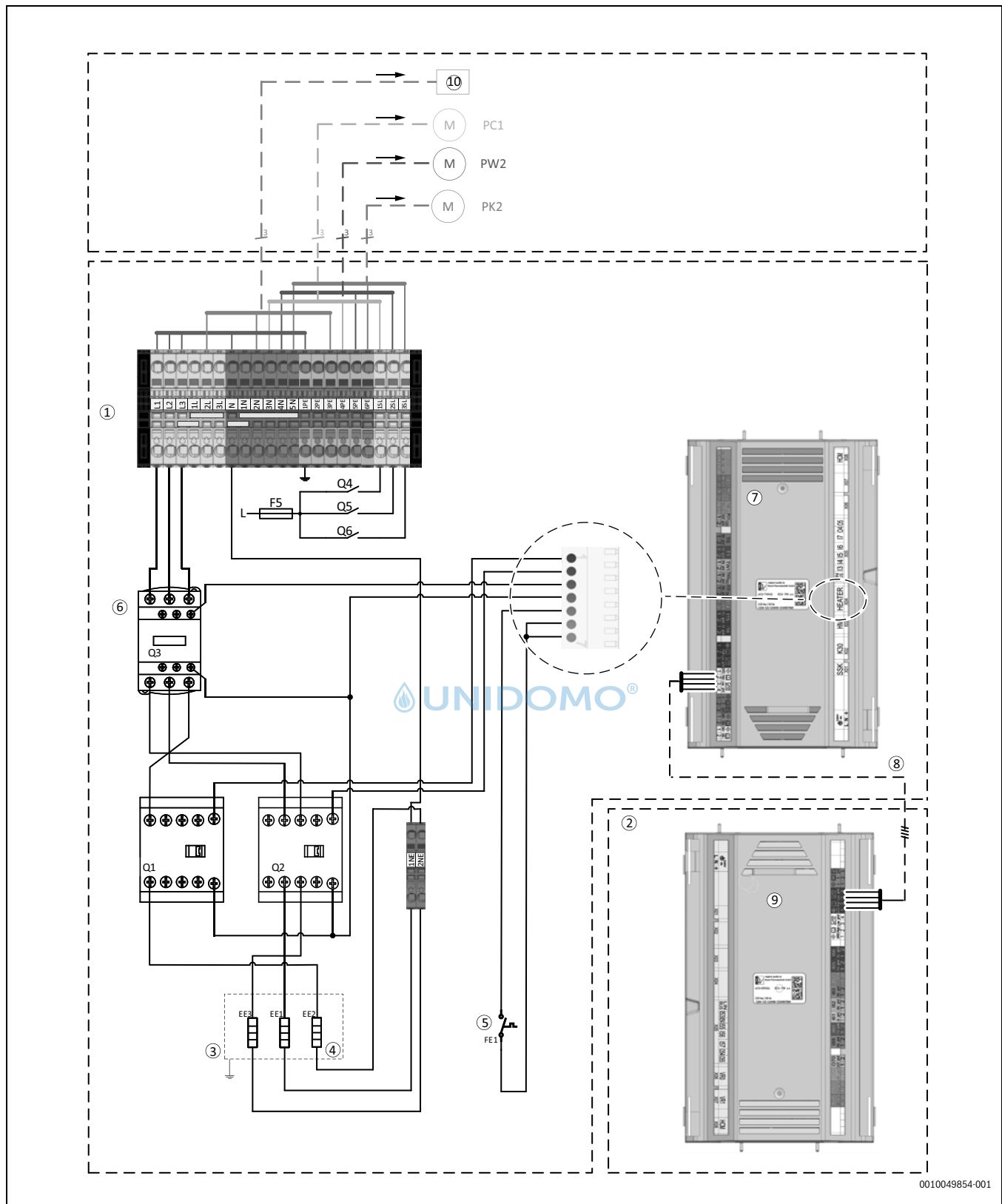
Bild 51 Spannungsversorgung Inneneinheit, Standard
