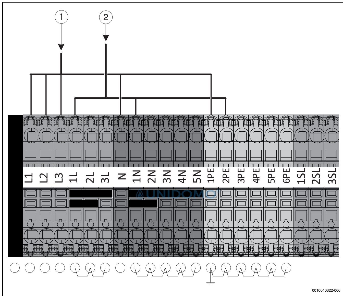
Bild 38 Elektrische Anschlüsse mit EVU-Sperre
