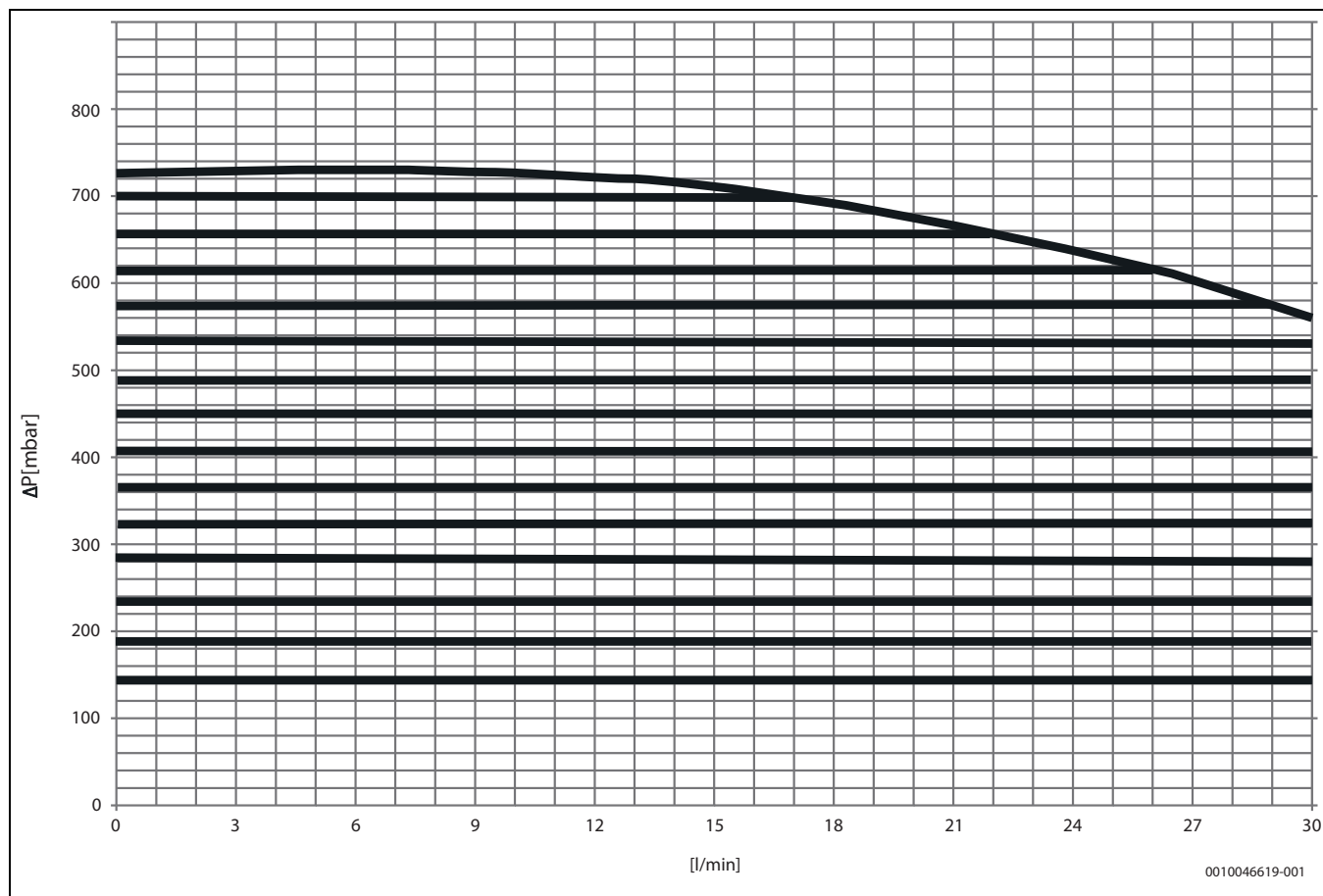
Bild 49 Leistungsdiagramm für PCO
