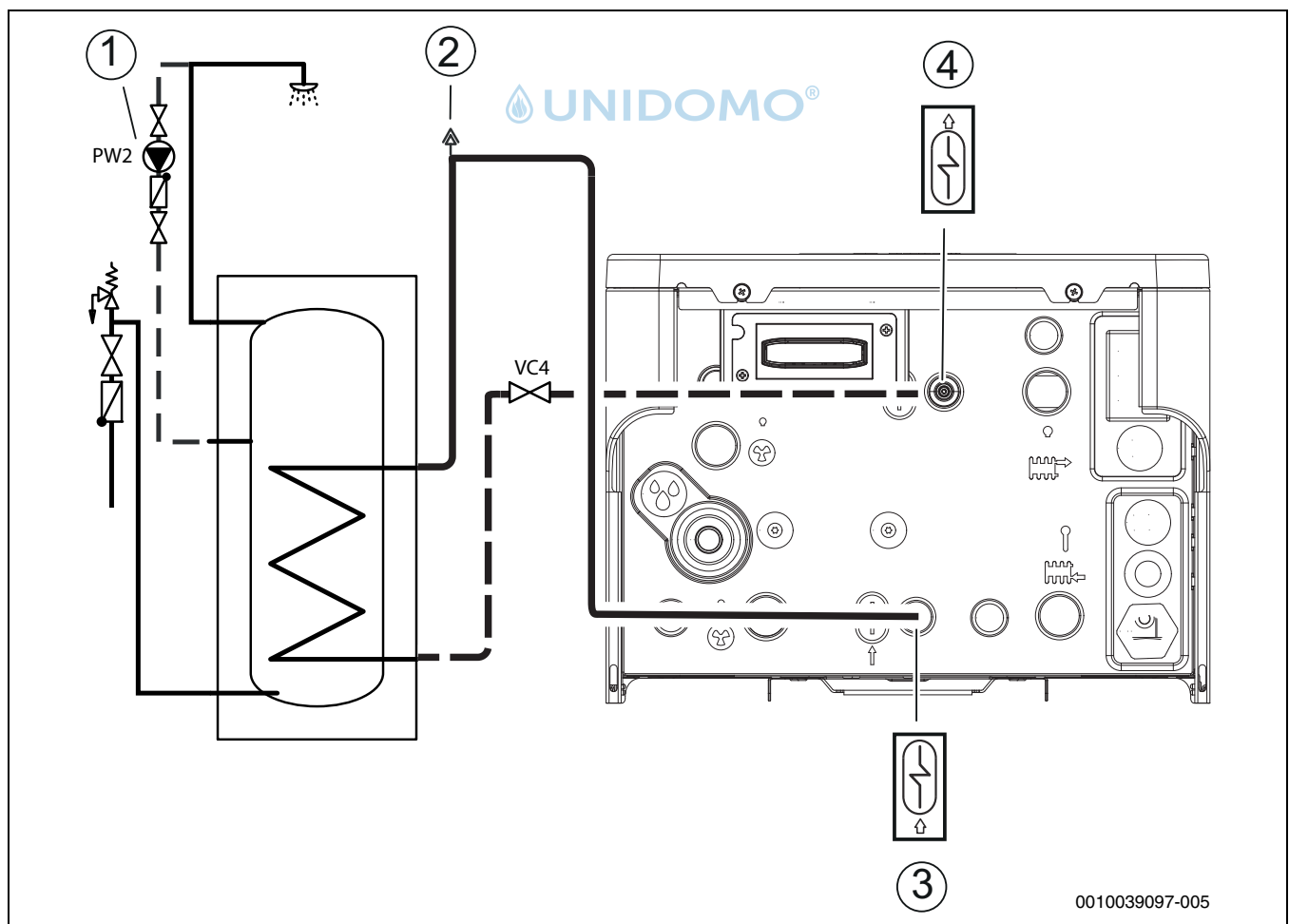
Bild 23 Trinkwasseranschlüsse Inneneinheit
