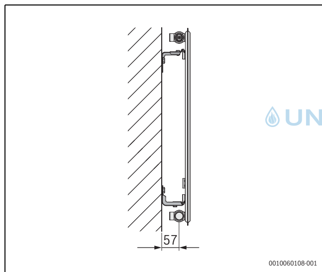
Sl.219 Držač za radijatore vrste 10 za VC-, VCM-, C-Plan/Profil.2
