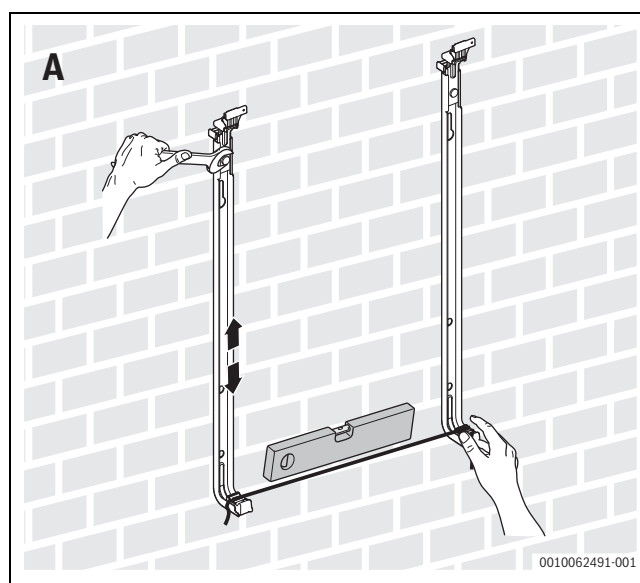
Fig. 300 Fissaggio dei supporti alla parete (cont.)
