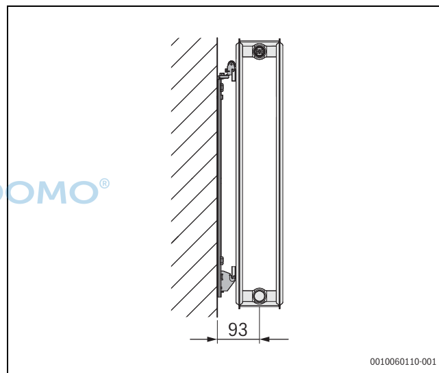
Fig. 167 Type de console de radiateur 20 pour VC-, VCM-, C-Plan/Profil.2
