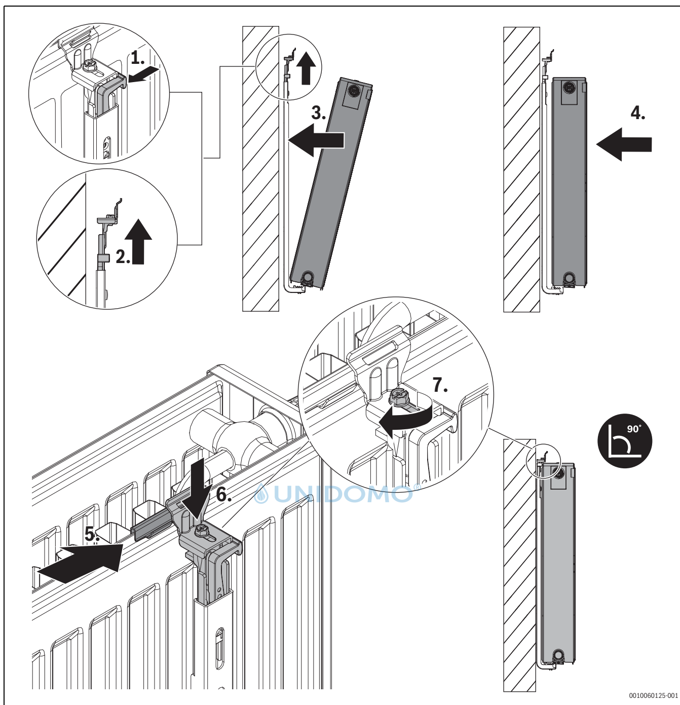
Σχ. 139 Τοποθέτηση του θερμαντικού σώματος στον βραχίονα (συνέχ.)
