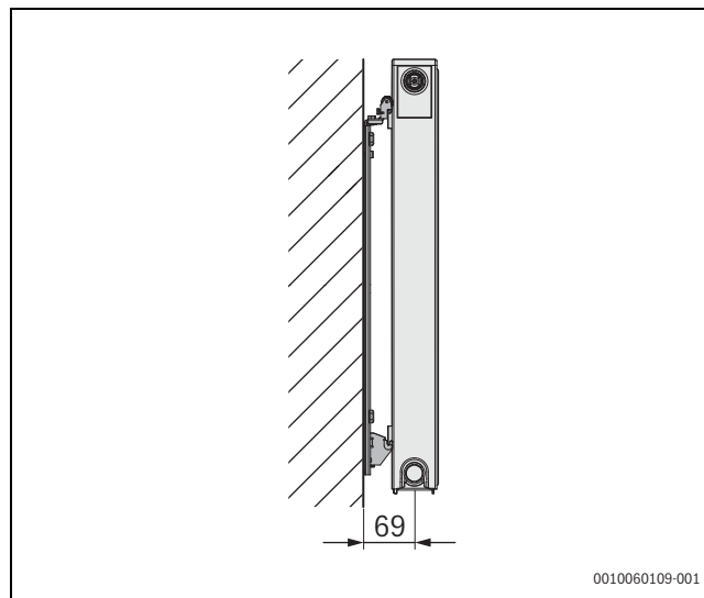
Σχ. 112 Βραχίονας θερμαντικού σώματος τύπου 11 για VC-, VCM-, C-Plan/Profil.2
