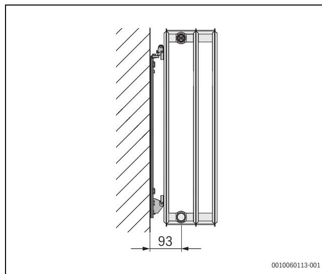
Σχ. 116 Βραχίονας θερμαντικού σώματος τύπου 30 για VC-, VCM-, C-Plan/Profil.2
