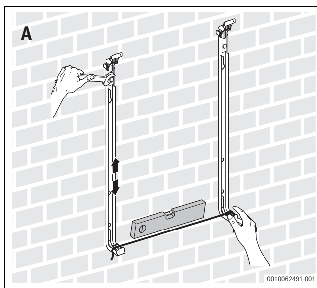
Fig. 192 Fixation des supports au mur (suite)
