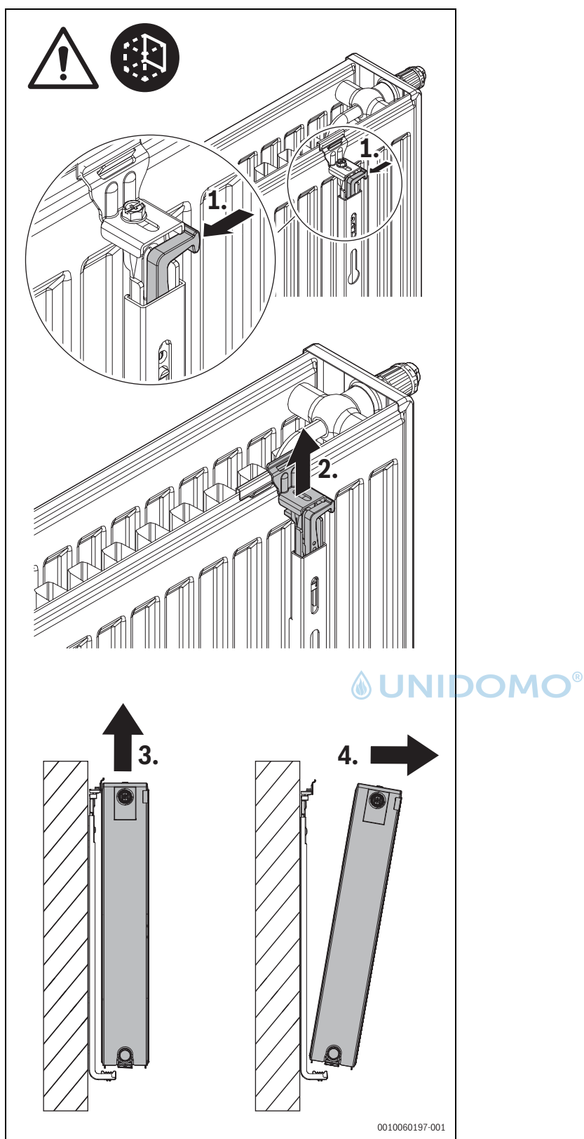
Fig. 285 Smontaggio a parete
