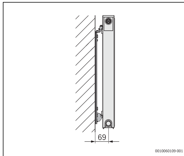
Fig. 166 Type de console de radiateur 11 pour VC-, VCM-, C-Plan/Profil.2
