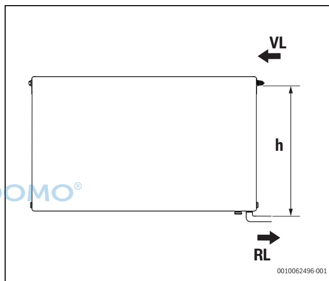
Σχ. 157 Ισοσκελής σύνδεση
