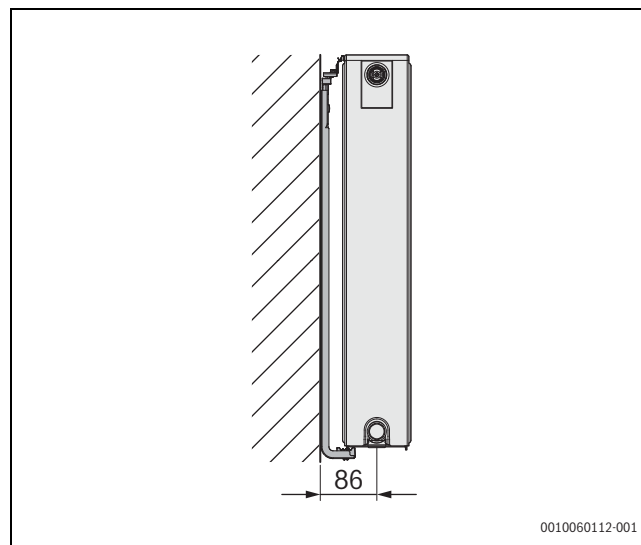
Sl.223 Držač za radijatore vrste 22 za VC-, VCM-, C-, A-Plan/Profil.2
