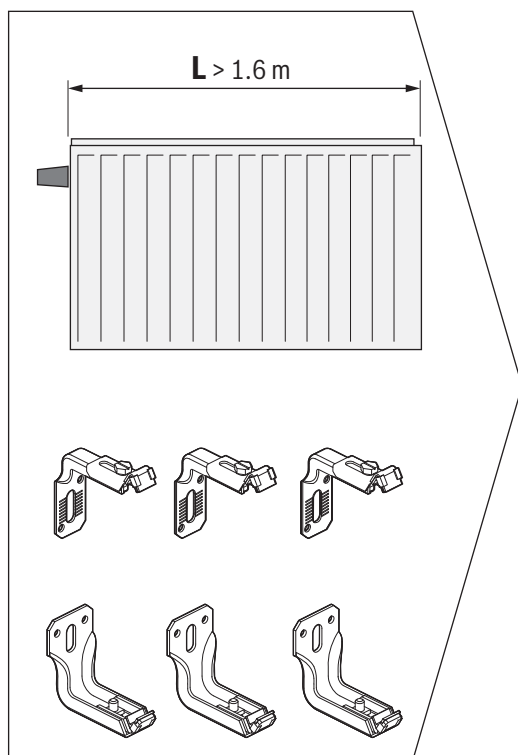
Sl.232 Držać za radijatore vrste 10 za VC-, VCM-, C-Plan/Profil.2
