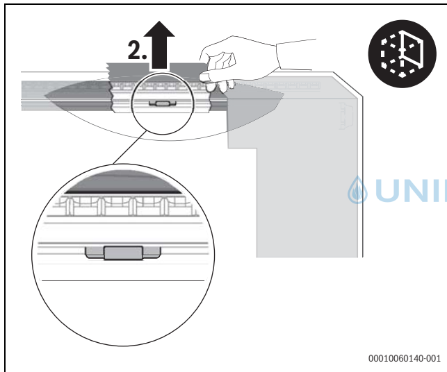
Σχ. 160 Άνοιγμα του επάνω μέρους του κουτιού
