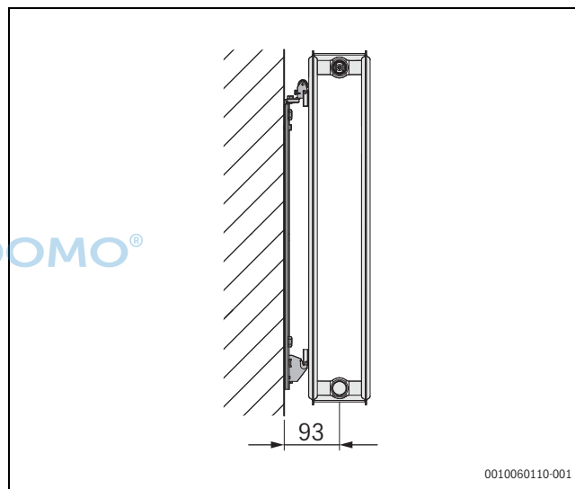
Σχ. 113 Βραχίονας θερμαντικού σώματος τύπου 20 για VC-, VCM-, C-Plan/Profil.2
