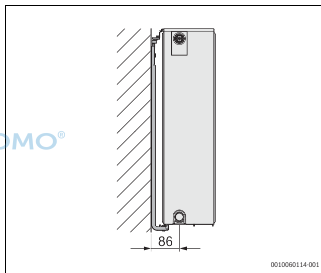
Σχ. 117 Βραχίονας θερμαντικού σώματος τύπου 33 για VC-, VCM-, C-, A-Plan/Profil.2
