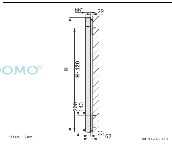
Bild 10 Heizkörperinstallation Typ 20 für VC-, VCM-, C-Profil/Plan.2
