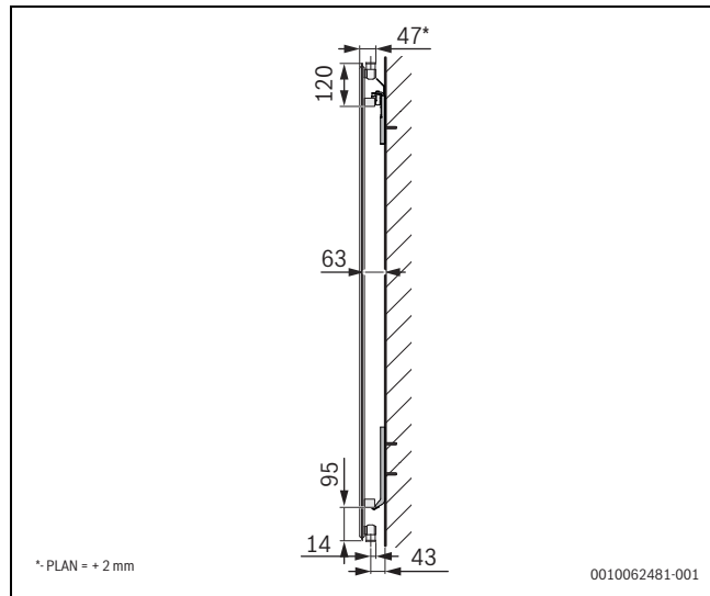
Fig. 172 Installation des radiateurs de type 10 pour CV Profil/ Plan.2
