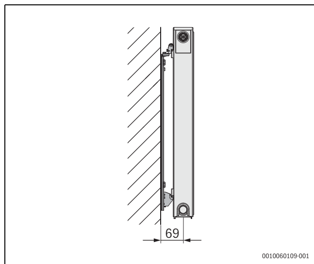
Sl.220 Držač za radijatore vrste 11 za VC-, VCM-, C-Plan/Profil.2
