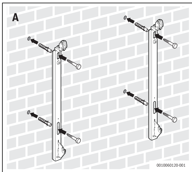
Sl.239 Pričvrščivanje držača na zid
