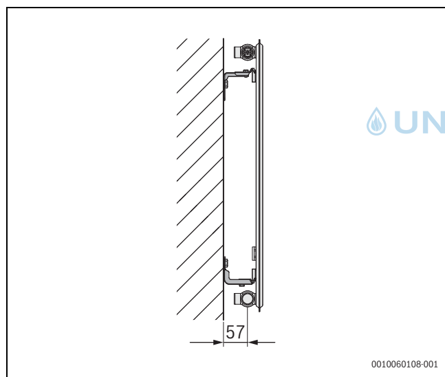
Fig. 273 Supporto per radiatore tipo 10 per VC-, VCM-, C-Plan/Profil.2
