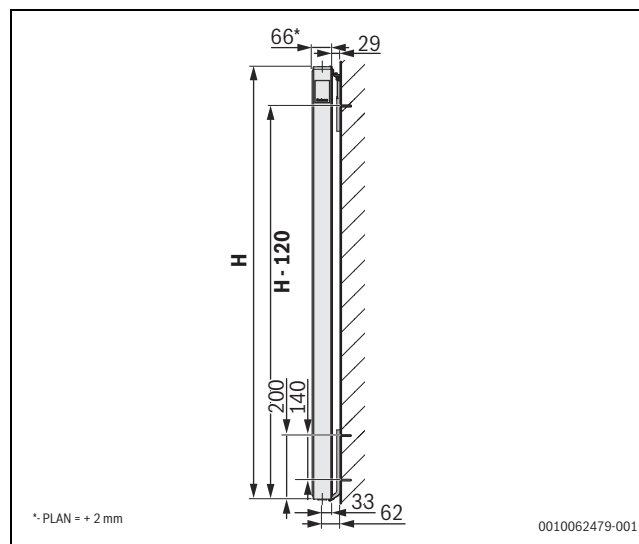
Σχ. 120 Εγκατάσταση θερμαντικών σωμάτων τύπου 21 για CV Profil/Plan.2
