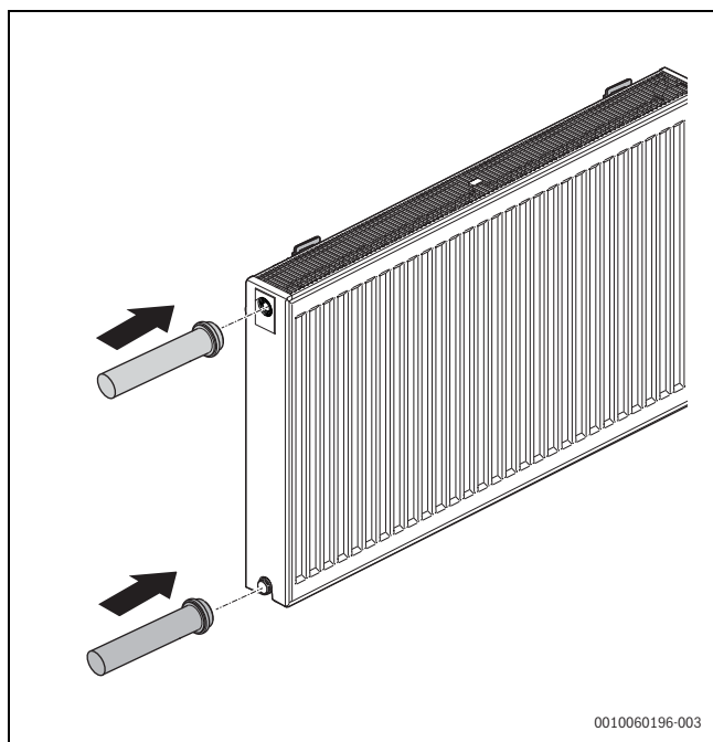
Sl.252 Pričvršćivanje cijevi na radijator
