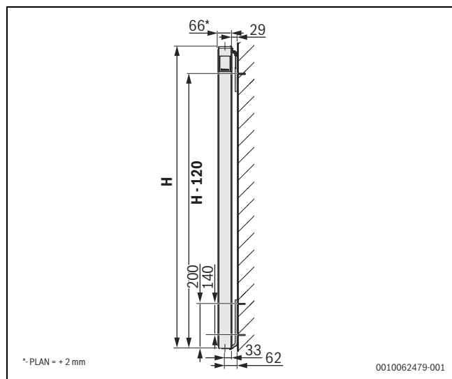
Fig. 174 Installation des radiateurs de type 21 pour CV Profil/ Plan.2
