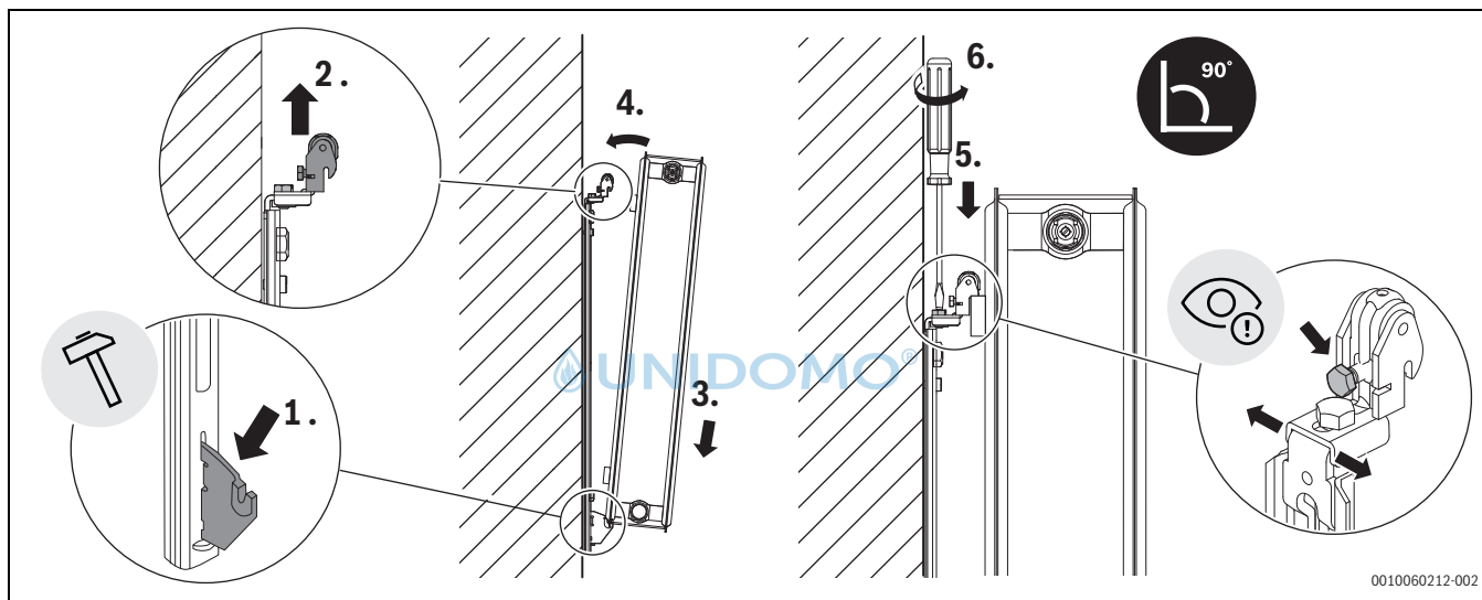
Sl.241 Montaža radijatora na držač
