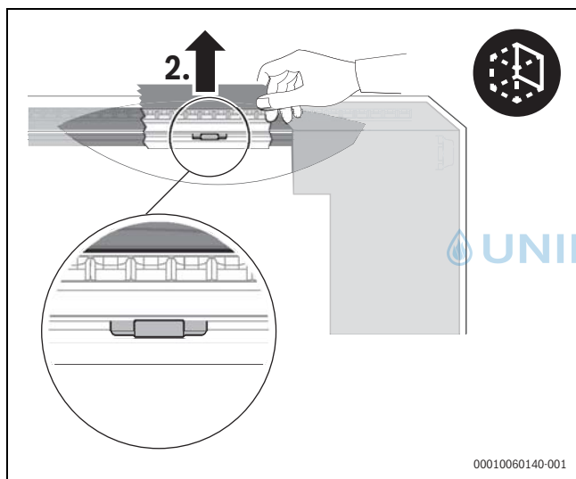
Sl.268 Otvaranje gornje strane kutije
