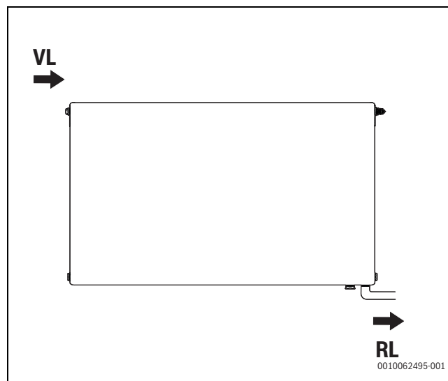
Bild 47 Wechelseitiger Anschluss
