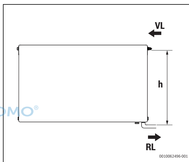
Bild 48 Gleichseitiger Anschluss
