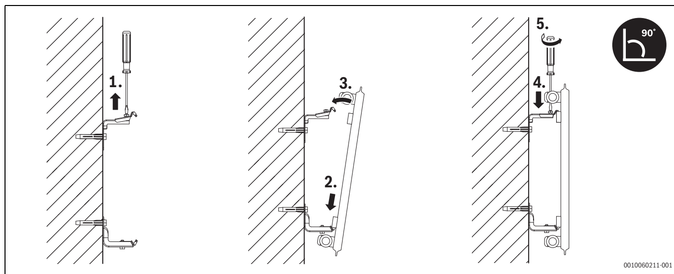
Σχ. 127 Τοποθέτηση του θερμαντικού σώματος στον βραχίονα
