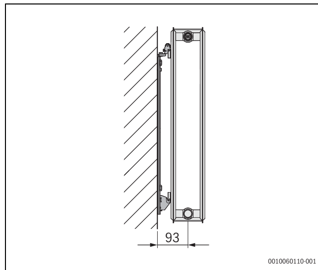
Sl.221 Držač za radijatore vrste 20 za VC-, VCM-, C-Plan/Profil.2
