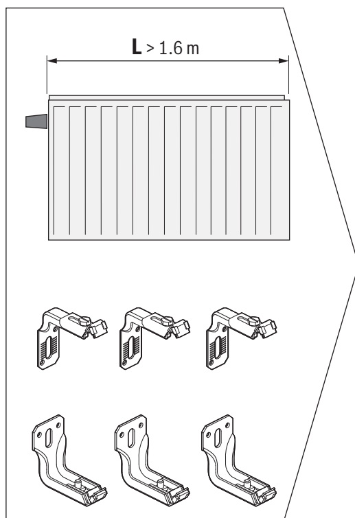
Σχ. 124 Βραχίονας θερμαντικού σώματος τύπου 10 για VC-, VCM-, C- Plan/Profil.2
