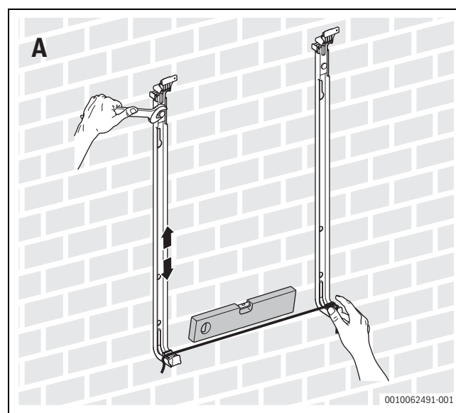
Bild 29 Anbringen der Konsolen an der Wand (Forts.)
