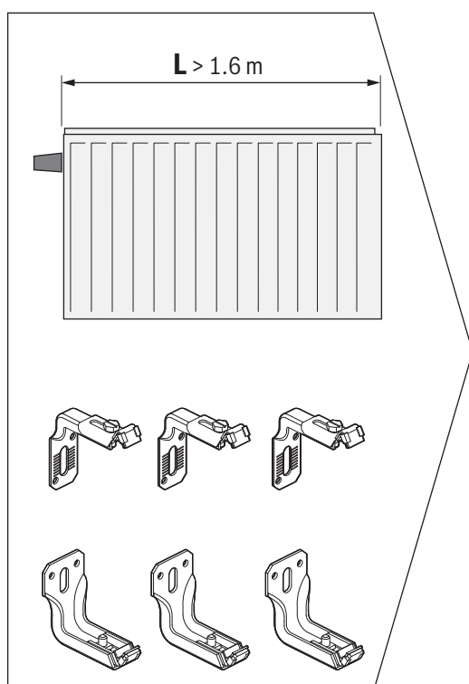
Fig. 178 Type de console de radiateur 10 pour VC-, VCM-, C-Plan/Profil.2
