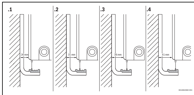
Sl.230 Mogućnosti pričvršćivanja zidnih držača za radijatore vrste 21, 22, 33 VC-, VCM-, A- i C-Profil/Plan
