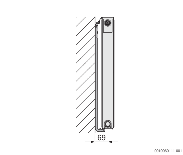
Fig. 59 Radiator bracket Type 21 for VC-, VCM-, C-, A-Plan/Profil.2
