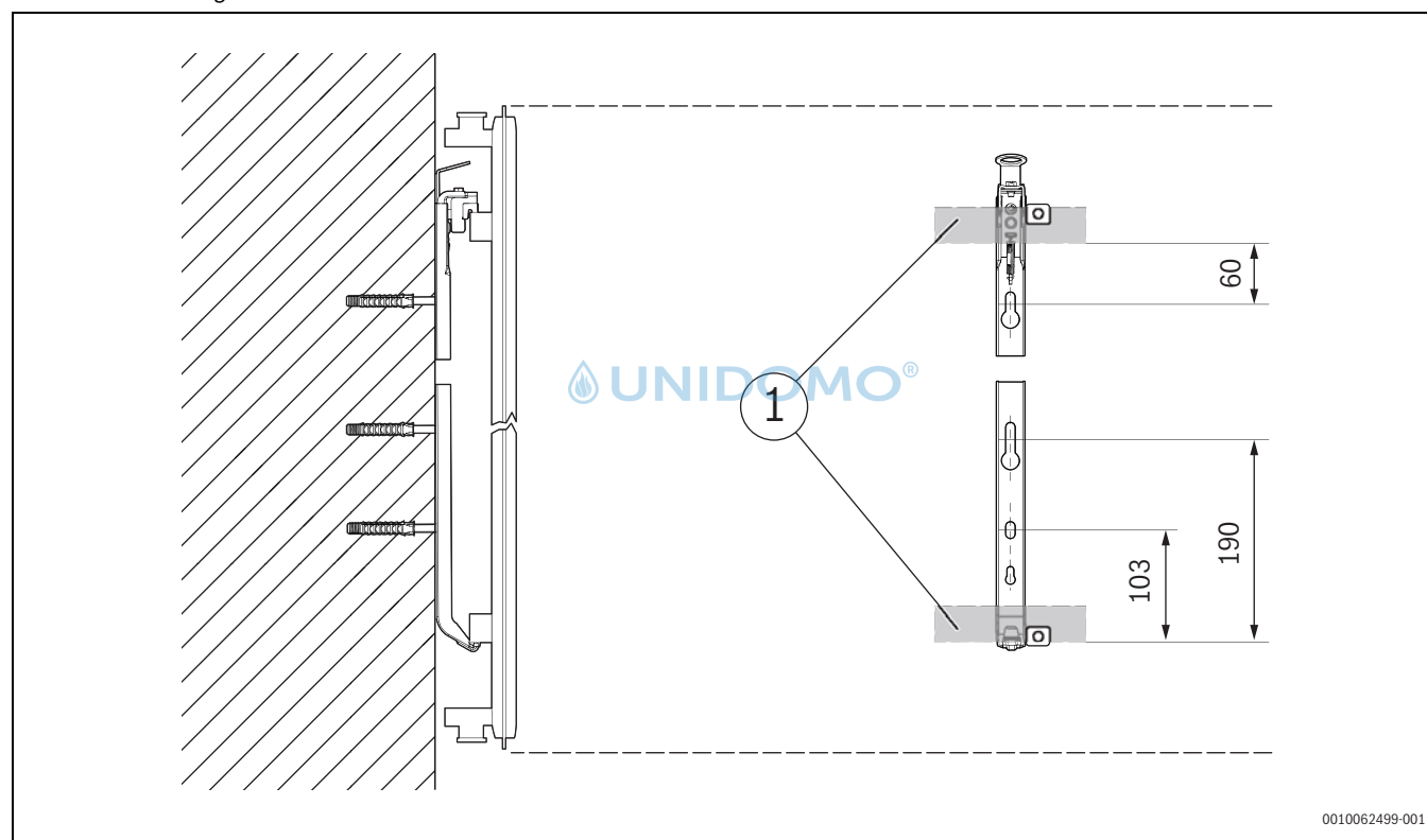
Bild 38 Bohrungsmaße für Heizkörperkonsolen F8 Typ 10 für CV
