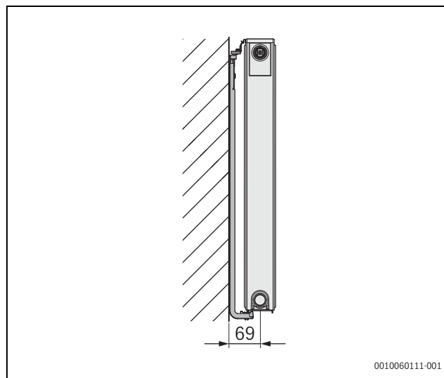
Fig. 276 Supporto per radiatore tipo 21 per VC-, VCM-, A-Plan/Profil.2
