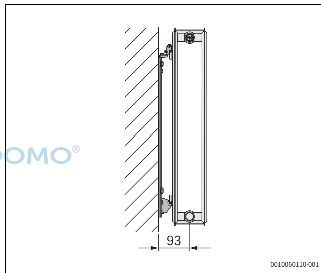
Fig. 275 Supporto per radiatore tipo 20 per VC-, VCM-, C-Plan/Profil.2
