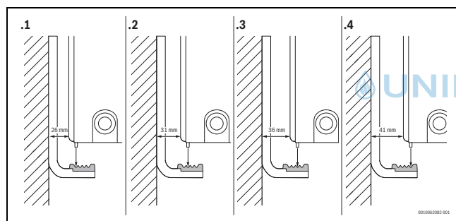
Fig. 176 Options de fixation du support mural pour les types 21, 22, 33 de radiateurs VC-, VCM-, A- et C-Profil/Plan
