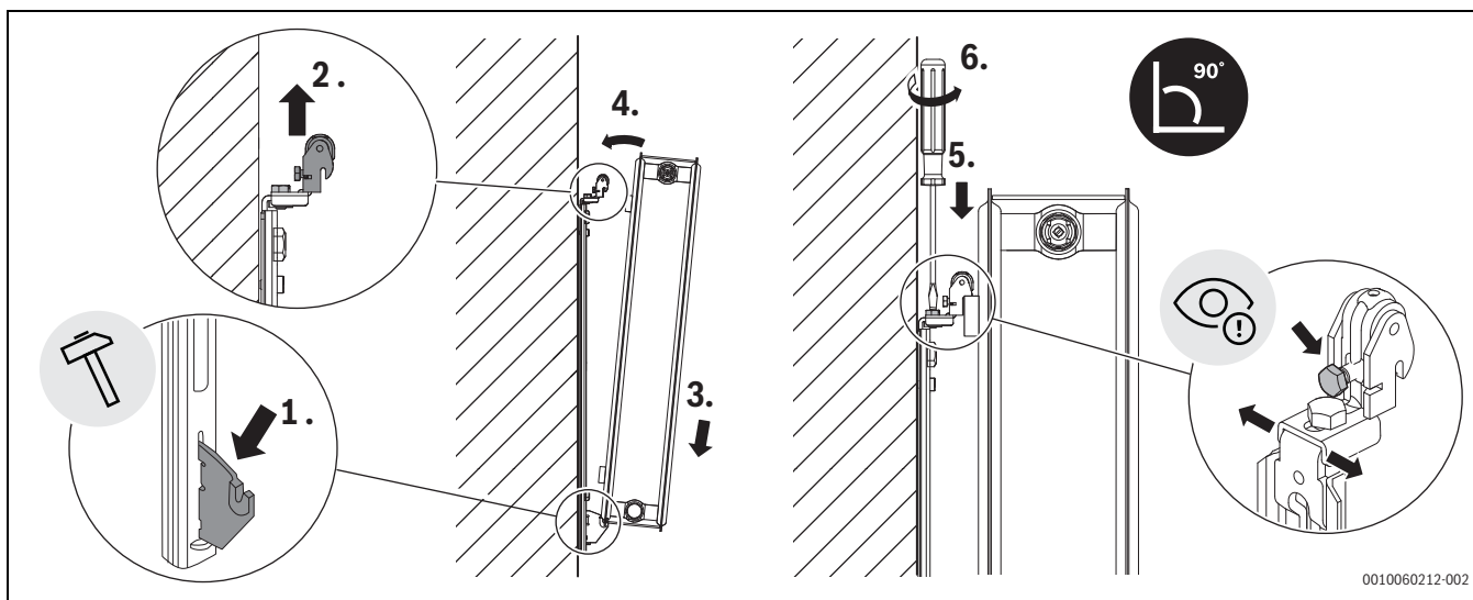
Σχ. 133 Τοποθέτηση του θερμαντικού σώματος στον βραχίονα
