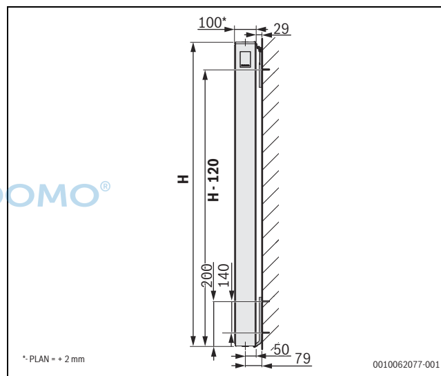
Σχ. 121 Εγκατάσταση θερμαντικών σωμάτων τύπου 22 για CV Profil/Plan.2
