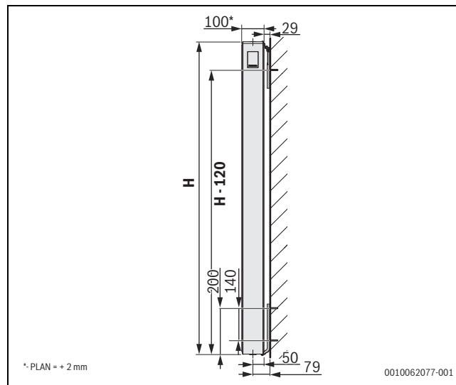
Fig. 175 Installation des radiateurs de type 22 pour CV Profil/ Plan.2
