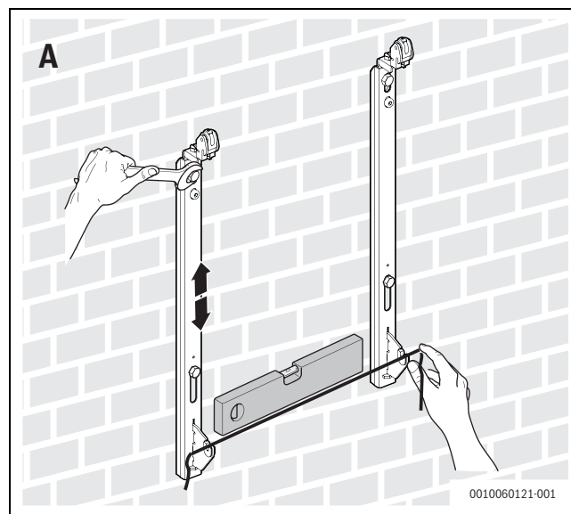
Sl.240 Pričvrščivanje držača na zid (nastavak)
