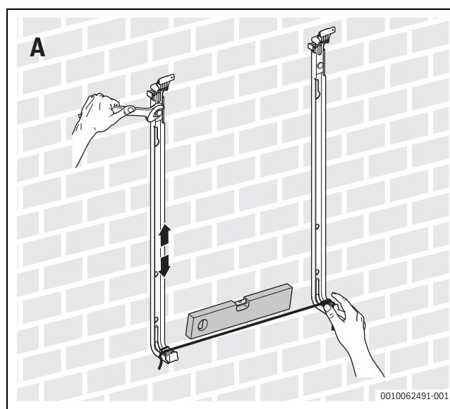
Sl.246 Pričvršćivanje držača na zid (nastavak)
