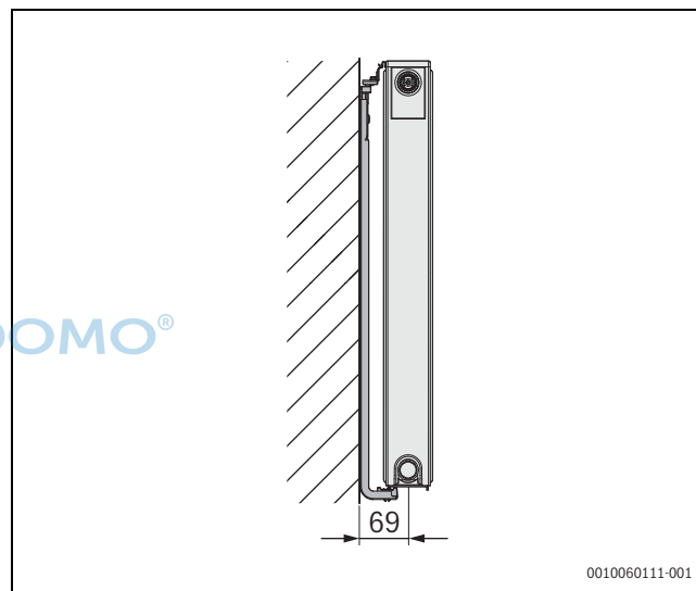
Sl.222 Držač za radijatore vrste 21 za VC-, VCM-, C-, A-Plan/Profil.2
