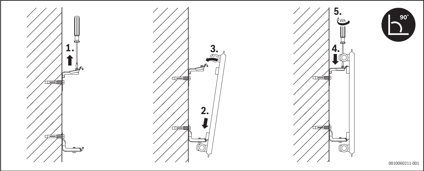
Fig. 289 Installazione del radiatore al supporto
