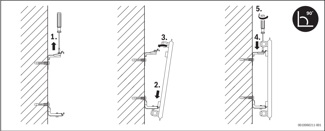
Fig. 181 Montage du radiateur sur le support
