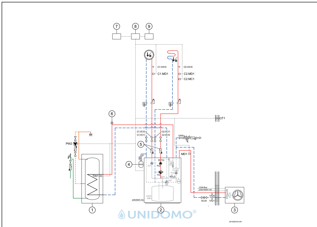
Bild 48 Anlage mit Zubehör Erweiterungs-Set intern - 2. Heizkreis
