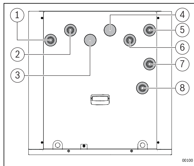
Bild 15 Hydraulische Anschlüsse
