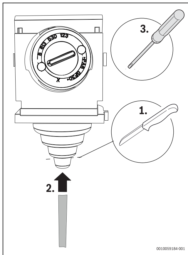
Bild 29 Kabel in die Zugentlastung einführen
