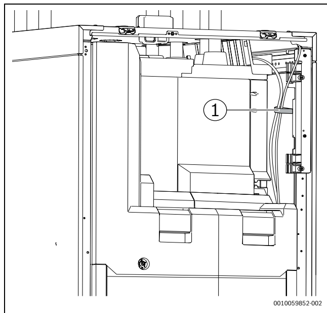
Bild 27 Netzkabel-Klettband sichern
