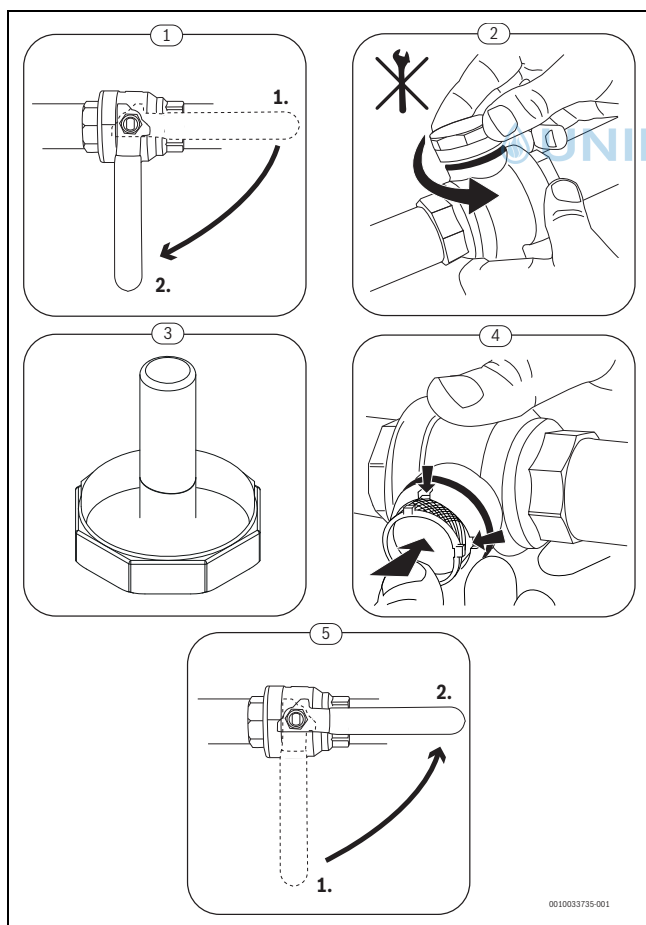
Bild 45 Filterreinigung
