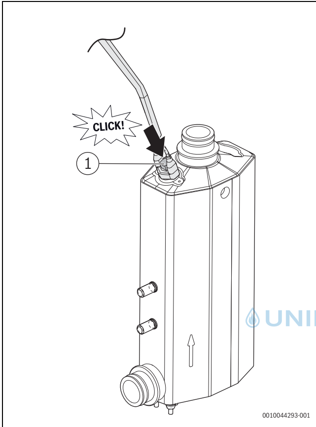
Bild 43 Elektrischer Zuheizer
