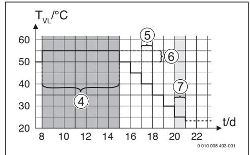
Bild 17 Ablauf der Estrichrocknung mit den Grundeinstellungen in der Abkühlphase
