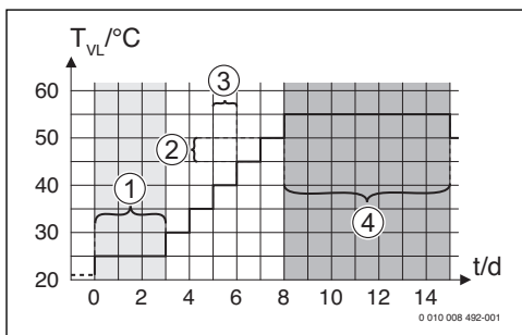
Bild 16 Ablauf der Estrichrocknung mit den Grundeinstellungen in der Aufheizphase
