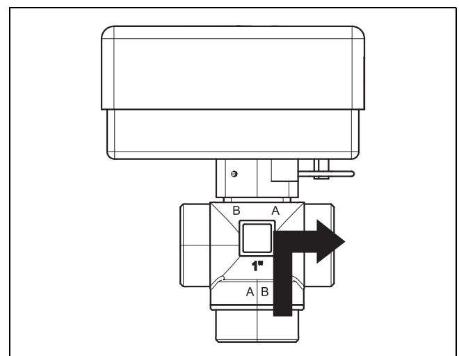
Bild 24 Kontakt geschlossen, Anschluss A offen
