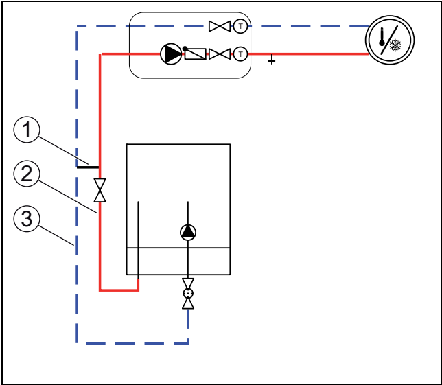
Bild 28 Inneneinheit mit Heizkreis und Bypass
