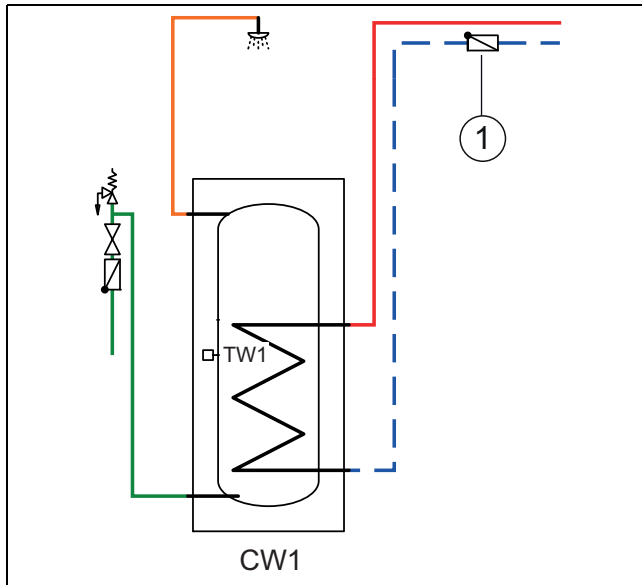
Bild 21 Warmwasserspeicher
