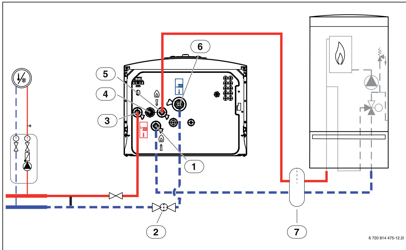
Bild 8 Anschluss der Inneneinheit mit Mischer für externen Zuheizter an die Heizungsanlage und den Zuheizter
