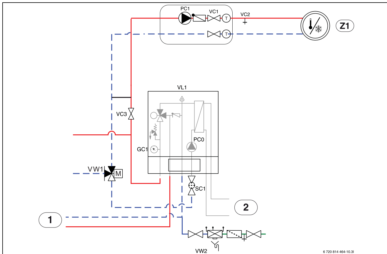
Bild 18 Inneneinheit mit externem Zuheizer und Heizsystem
