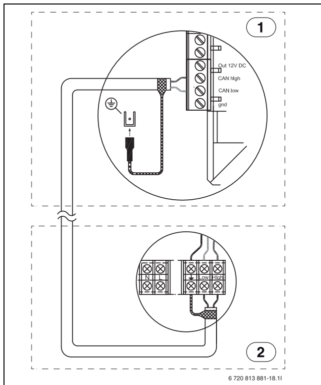
Bild 10 CAN-BUS-Verbindung
