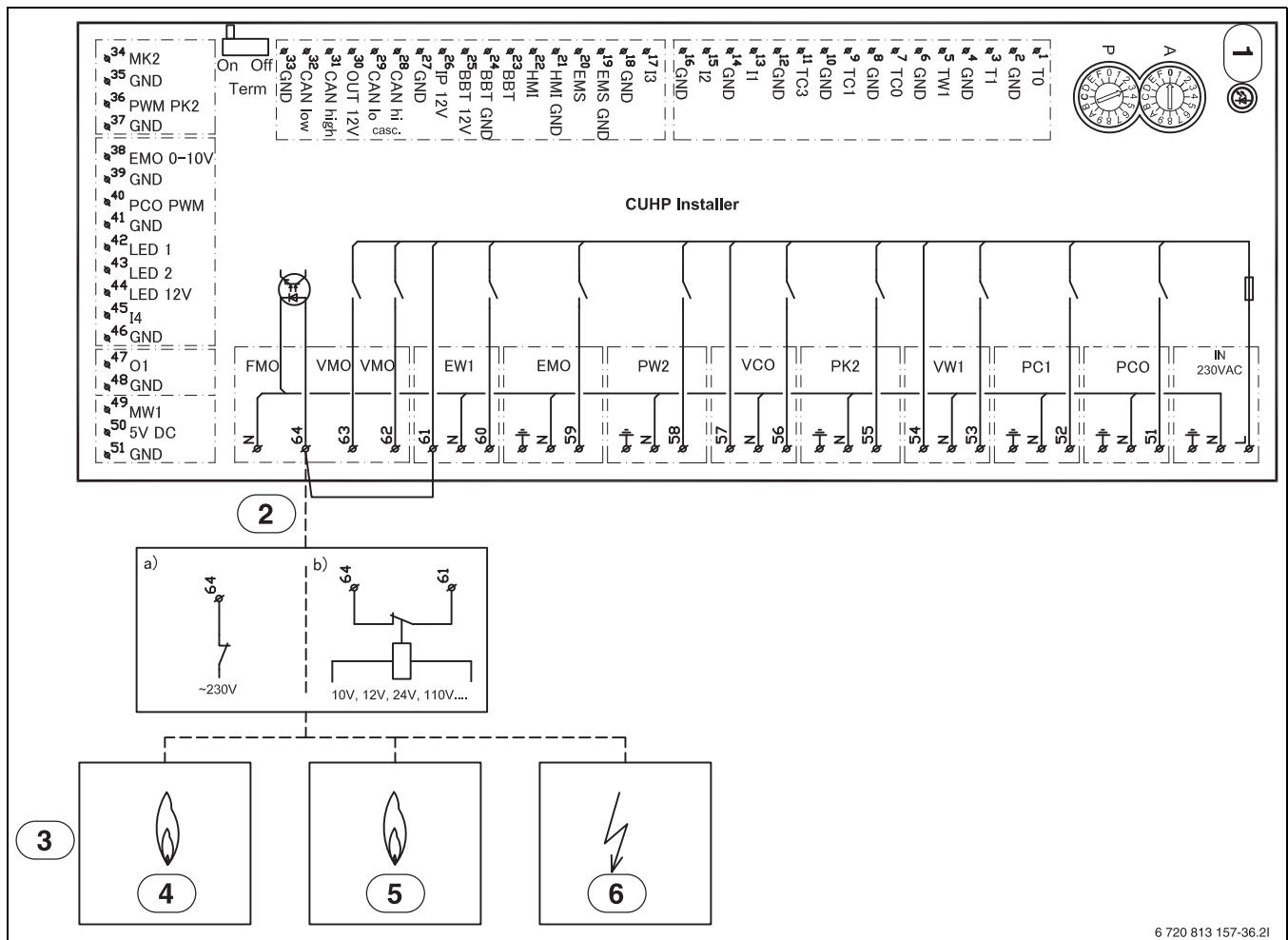
Bild 15 Schaltschema des Installationsmoduls, Alarm für externen Zuheizter
