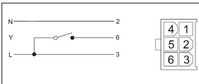
Bild 26 Molex-Stecker
