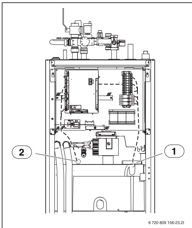
Bild 14 Kabeldurchführungen
