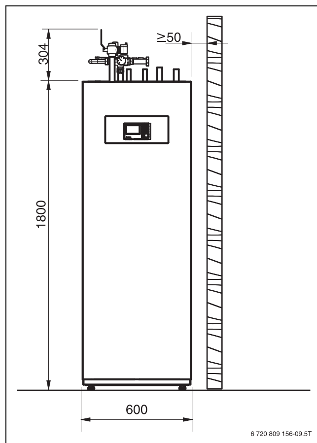
Bild 4 Abmessungen (mm)
