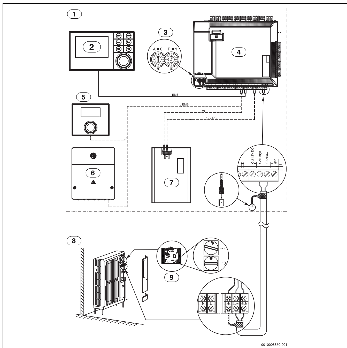
Bild 31 EMS/CAN-BUS-Schaltplan
