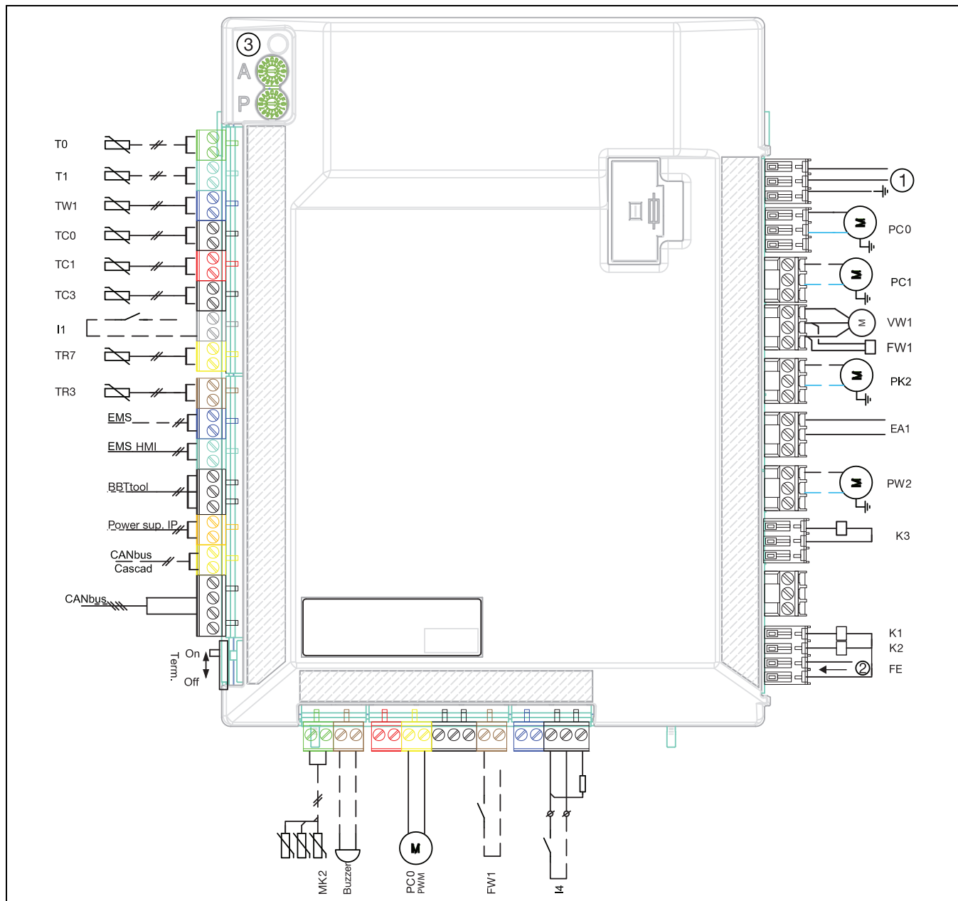
Bild 15 Schaltplan Installationsmodul
