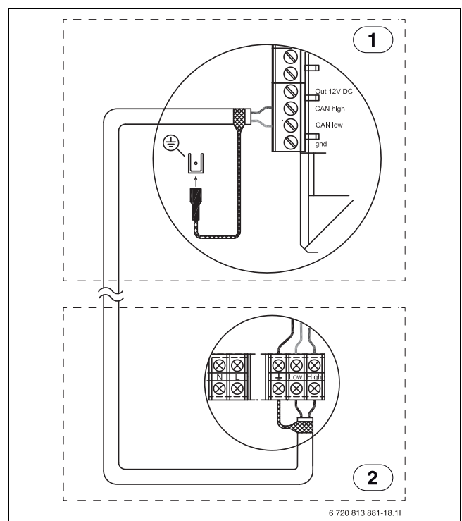
Bild 11 CAN-BUS-Verbindung
