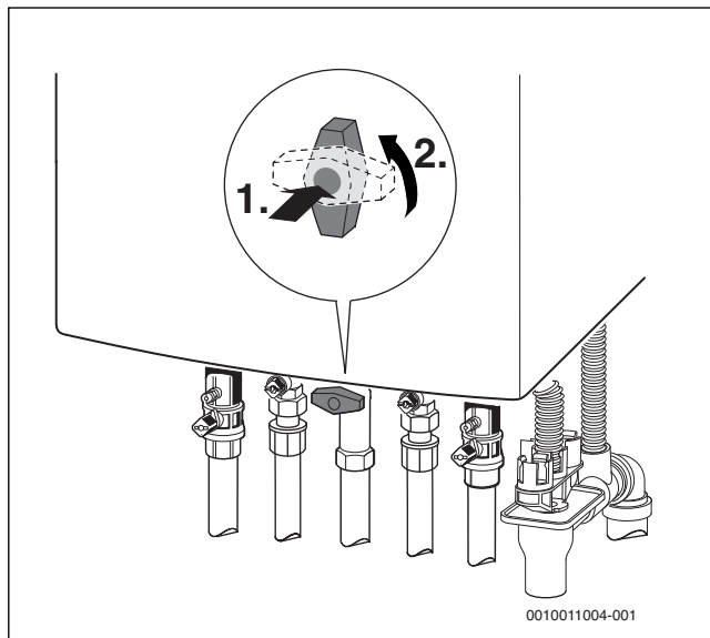
Bild 2 Gashahn öffnen
