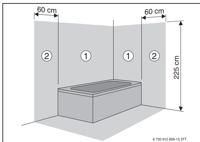
Bild 37 Schutzbereiche
