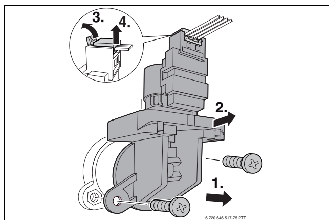
Bild 76 3-Wege-Ventil ausbauen
