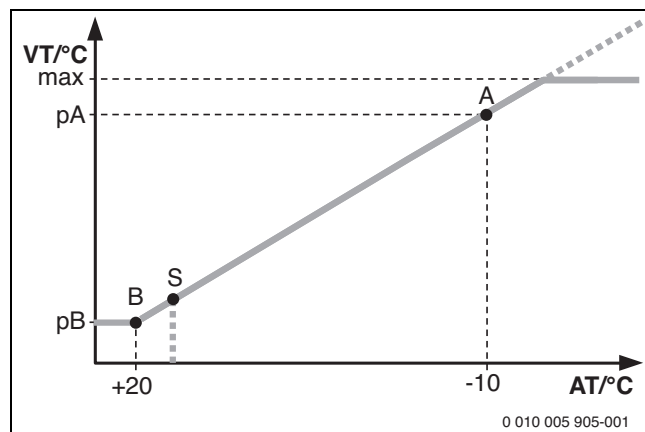
Bild 90 Heizkurve
