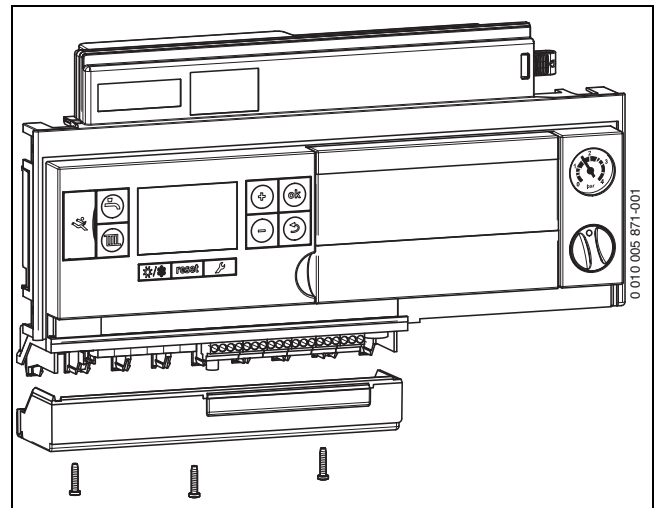
Bild 80 Abdeckung entfernen
