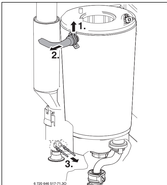
Bild 84 Vorlaufrohr lösen und Kabel abziehen
