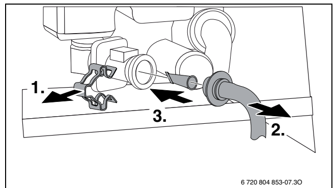
Bild 72 Sieb aus Kaltwasserrohr ausbauen
