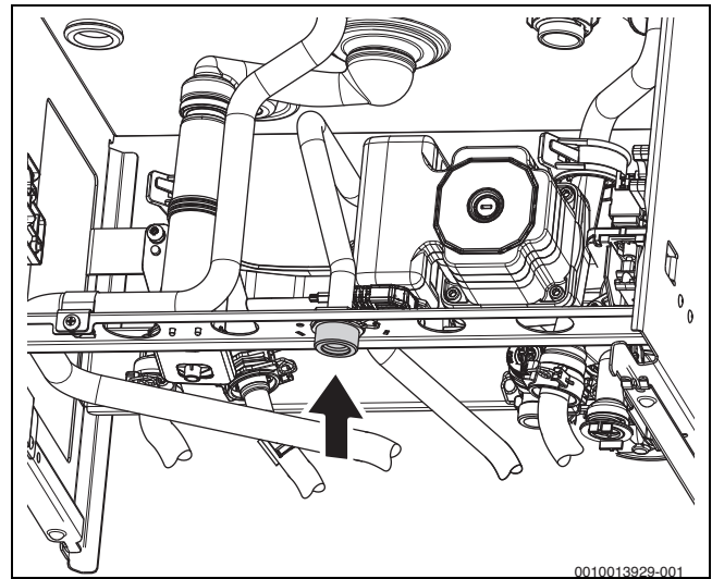
Bild 30 Anschluss externes Ausdehnungsgefäß
