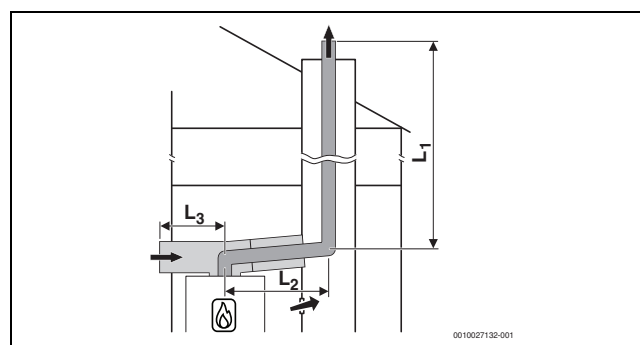
Bild 13 Starre Abgasführung nach C 53x im Schacht und Luft-Abgas-Führung mit separater Luftzufuhr und konzentrischer Abgasableitung im Aufstellraum
