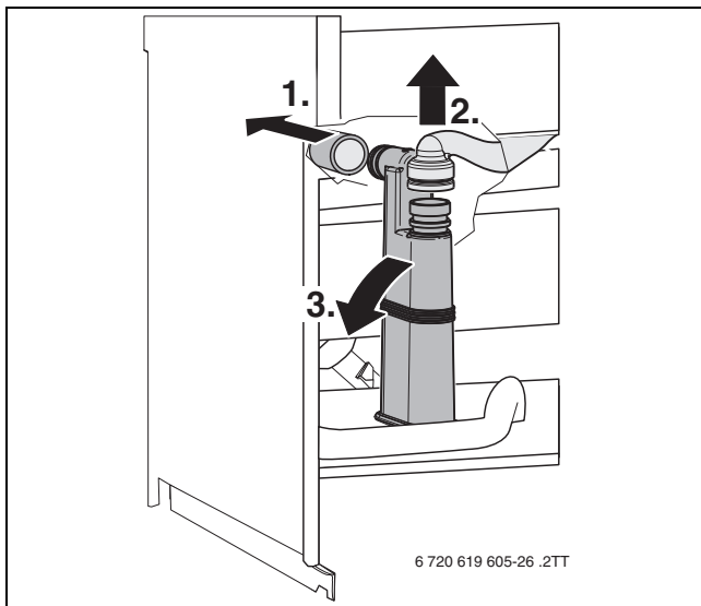
Bild 69 Kondensatsiphon ausbauen
