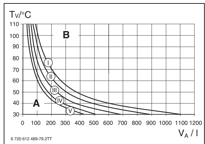
Bild 31 Kennlinien des Ausdehnungsgefäßes
