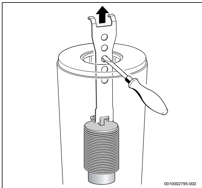
Bild 65 Unteren Verdrängungskörper herausnehmen
