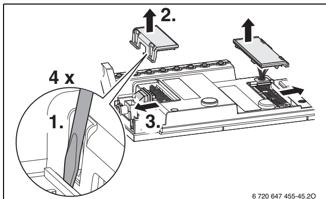
Bild 82 Abdeckung entfernen
