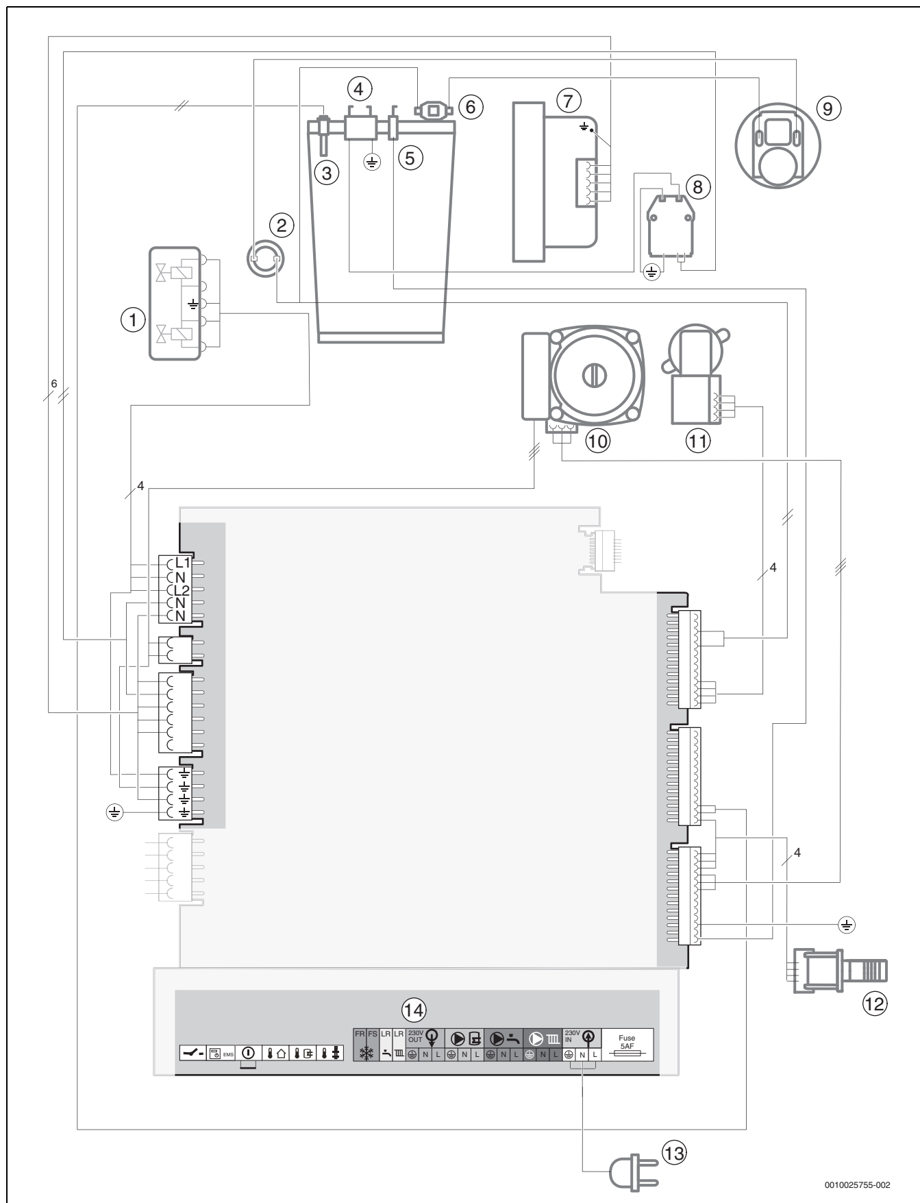
Bild 89 Elektrische Verdrahtung
