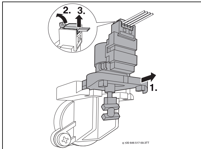
Bild 75 Motor des 3-Wege-Ventils ausbauen
