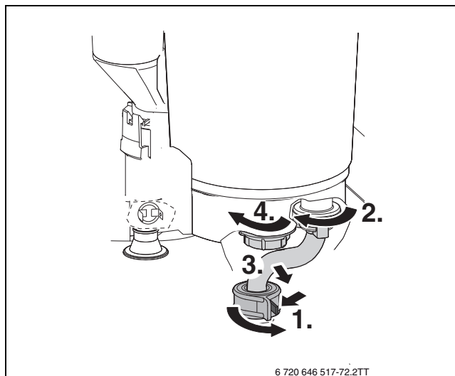
Bild 85 Mutter entfernen und Rücklaufrohr lösen
