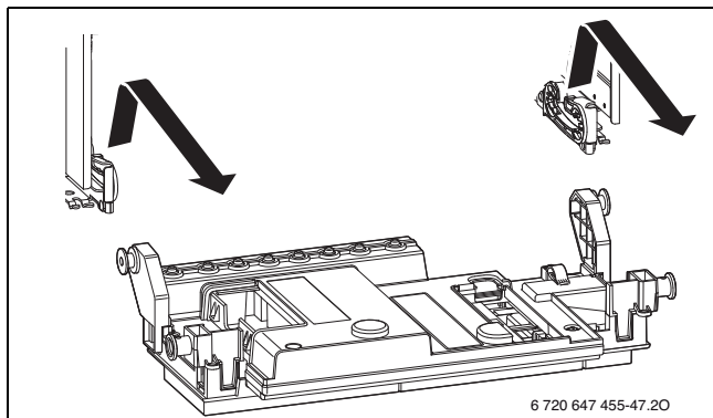
Bild 83 Steuergerät aushängen
