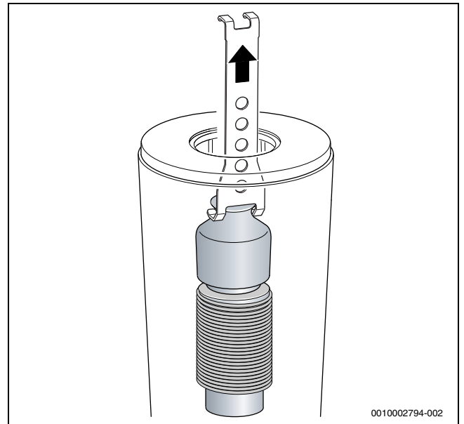
Bild 64 Oberen Verdrängungskörper herausnehmen
