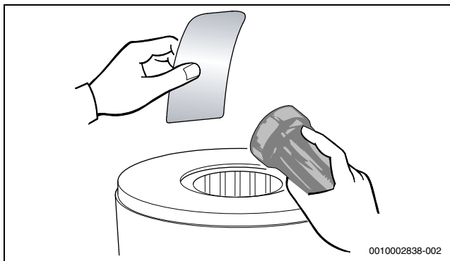
Bild 67 Wärmeblock auf Rückstände prüfen
