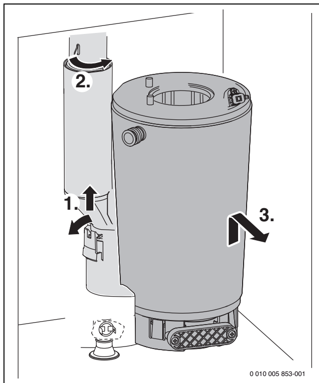
Bild 86 Wärmeblock ausbauen
