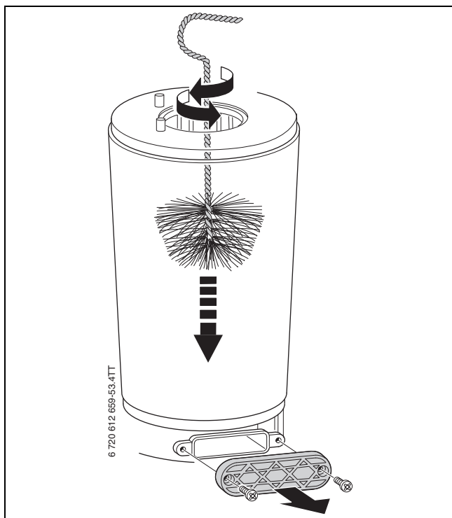
Bild 66 Wärmeblock reinigen
