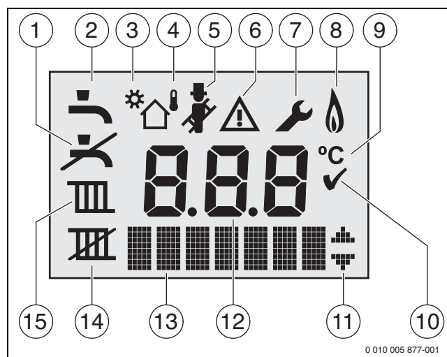
Bild 42 Displayanzeigen
