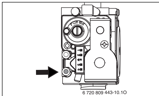
Bild 57 Messstutzen für Gas-Anschlussdruck
