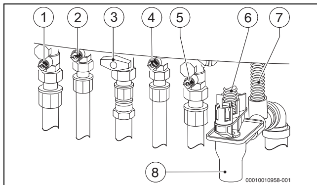
Bild 36 Gas- und wasserseitige Anschlüsse (Zubehör)
