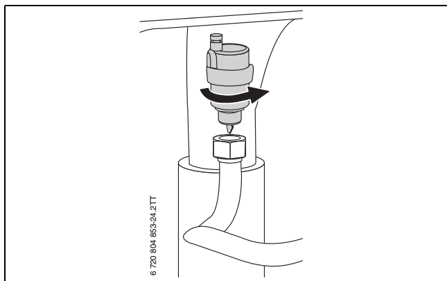
Bild 74 Automatischen Entlüfter ausbauen
