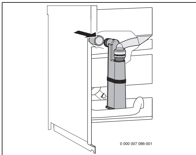
Bild 34 Schlauch am Kondensatsiphon montieren
