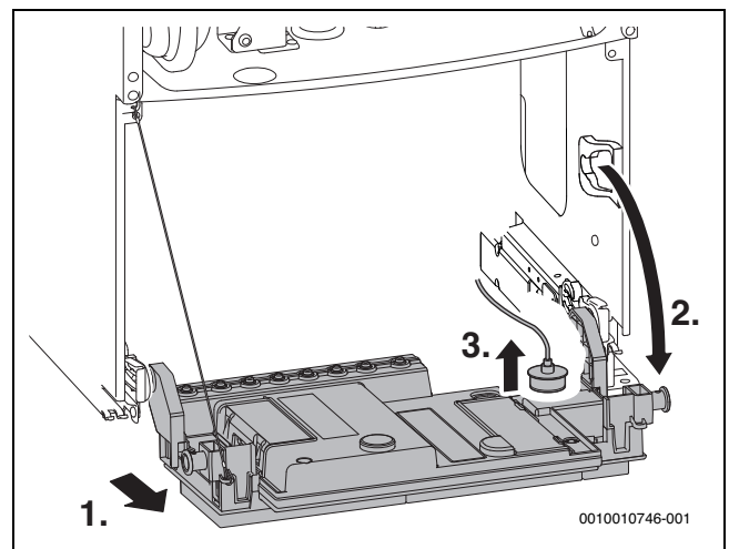
Bild 81 Steuergerät nach unten klappen
