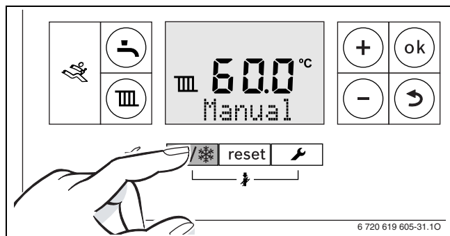
Bild 53 Manuellen Betrieb einstellen
