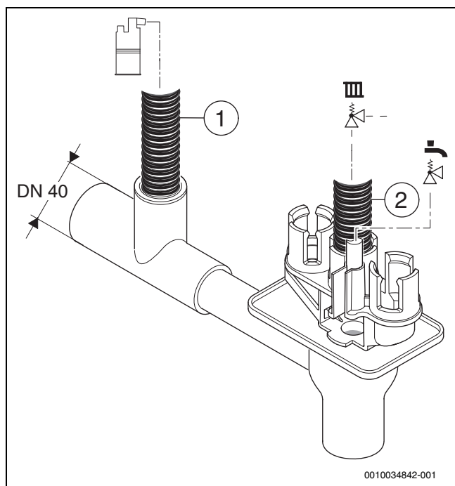
Bild 35 Kondensatschlauch und Schlauch vom Sicherheitsventil am Siphon montieren
