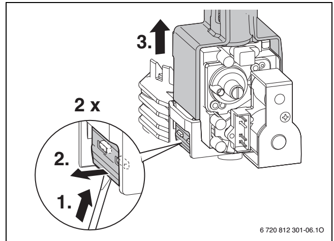
Bild 79 Gasarmatur ausbauen
