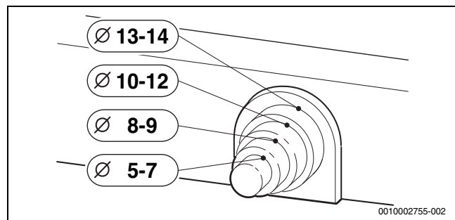
Bild 40 Zugentlastung an Kabeldurchmesser anpassen
