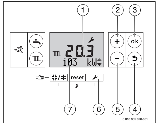
Bild 54 Übersicht der Bedienelemente
