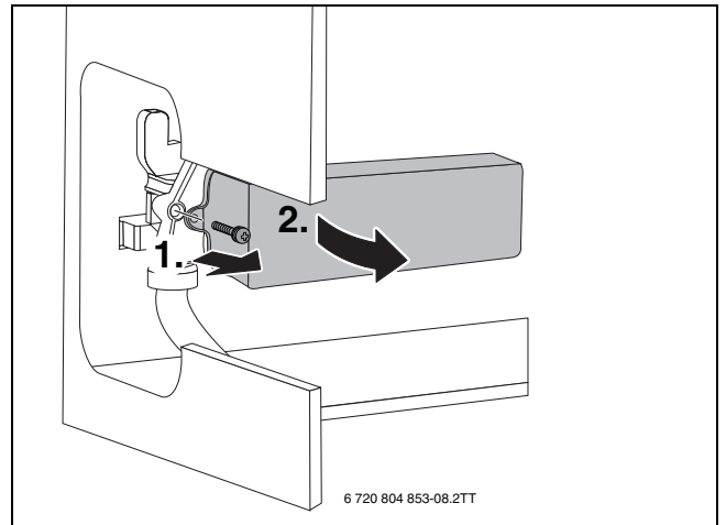
Bild 71 Plattenwärmetauscher ausbauen
