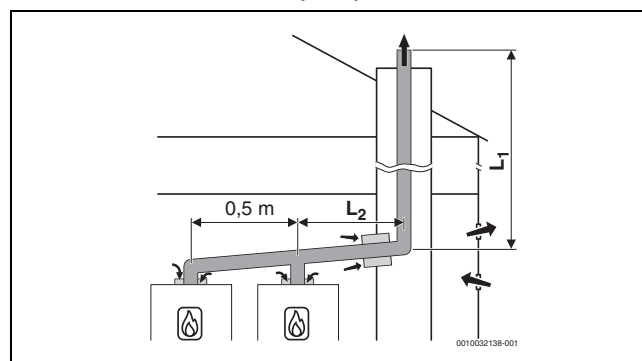
Bild 27 Kaskade mit 2 Geräten:
