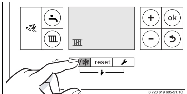
Bild 51 Manuellen Sommerbetrieb einschalten
