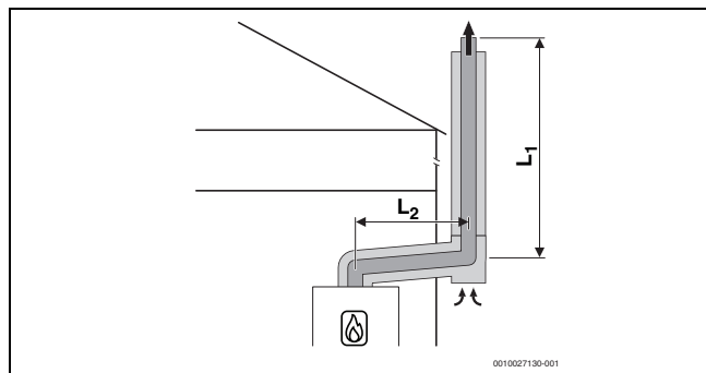
Bild 15 Konzentrische Luft-Abgas-Führung nach C_{53(x)} an der Außenwand
