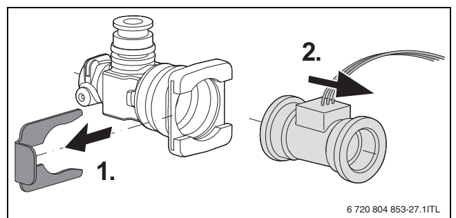
Bild 73 Turbine am Kaltwasserrohr ausbauen
