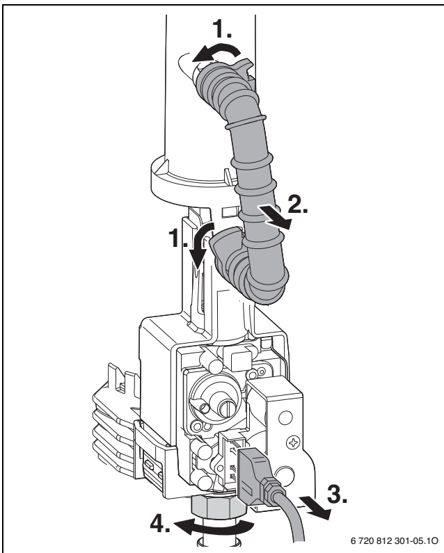
Bild 78 Gasarmatur ausbauen
