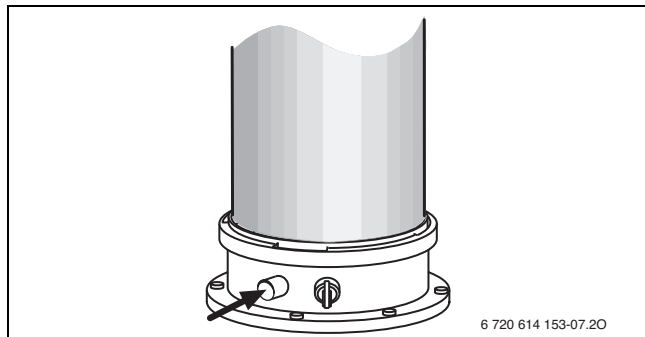
Bild 55 Abgasmessstutzen
