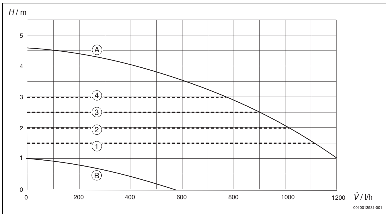
Bild 91 Pumpenkennfelder und Pumpenkennlinien
