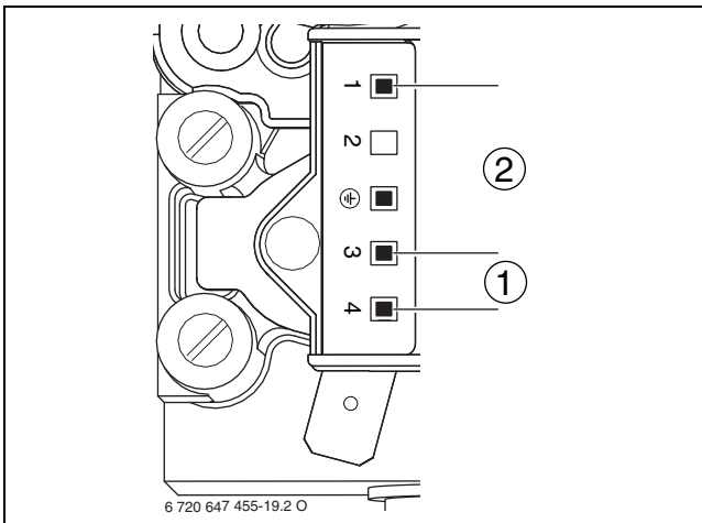
Bild 77 Messstellen an der Gasarmatur
