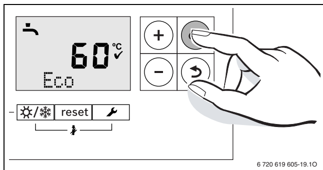
Bild 48 Anzeig eco-Betrieb bestätigen
