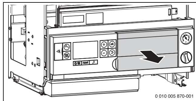
Bild 38 Abdeckung entfernen und Bedieneinheit montieren
