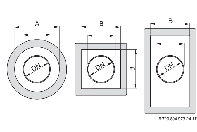
Bild 5 Schachtquerschnitte
