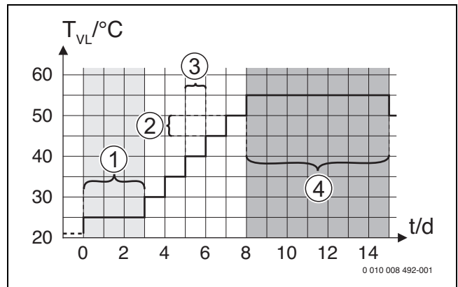
Bild 72 Ablauf der Estrich Trocknung mit den Grundeinstellungen in der Aufheizphase
