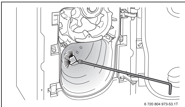
Bild 76 Feuerraum durchbürsten
