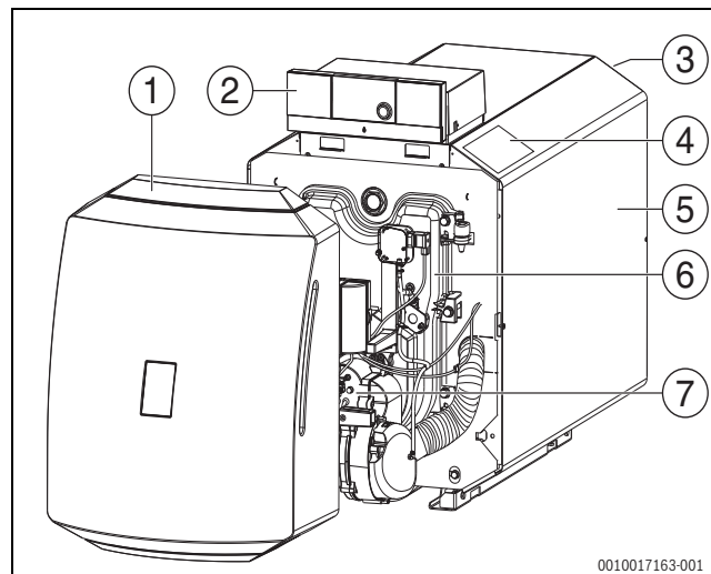
Bild 1 Vorderansicht
