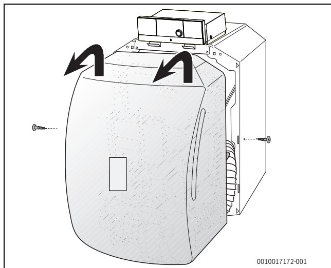
Bild 9 Brennerhaube abnehmen
