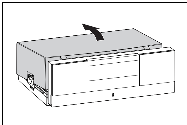
Bild 38 Abdeckhaube demontieren
