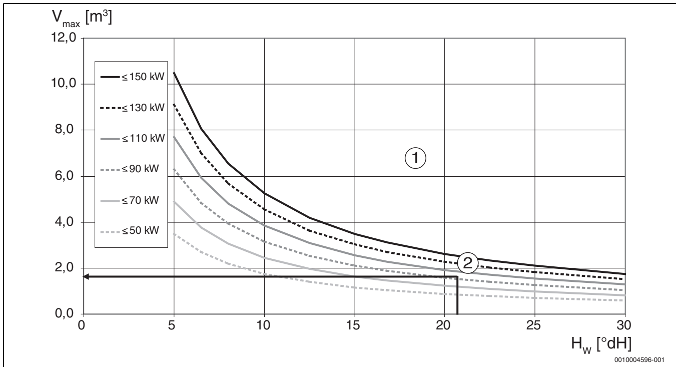
Bild 91 Anforderungen an die Füll- und Ergänzungwassermenge für Wärmeerzeuger aus Eisenwerkstoffen (Grauguss und unlegierte Stähle) bis 150 kW
