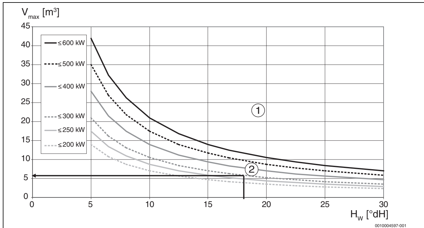
Bild 92 Anforderungen an die Füll- und Ergänzungwassermenge für Wärmeerzeuger aus Eisenwerkstoffen (Grauguss und unlegierte Stähle) von 200 kW bis 600 kW
