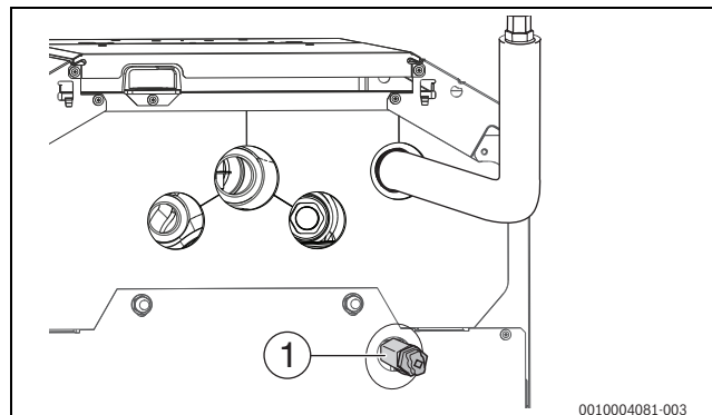
Bild 36 Wärmetauscher entlüften
