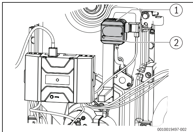
Bild 90 Störung am Druckwächter zurücksetzen
