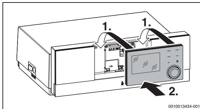
Bild 53 Bedieneinheit einhängen
