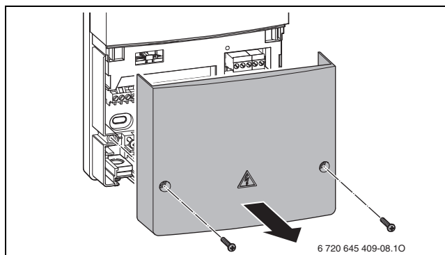
Bild 42 Gehäuse öffnen
