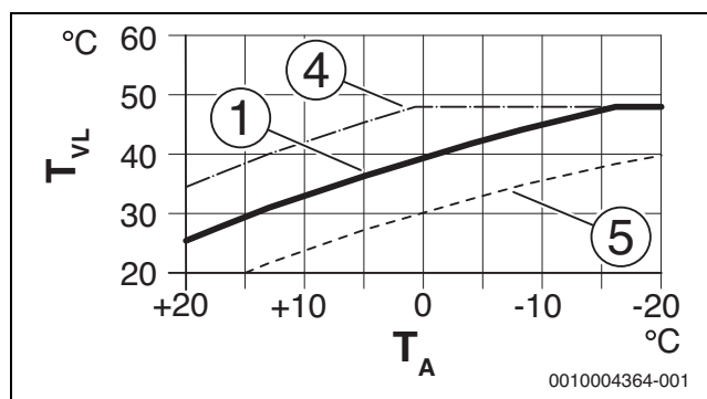
Bild 69 Einstellung der Heizkurve für Fußbodenheizung Parallelverschiebung über Raumtemperatur-Offset oder gewünschte Raumtemperatur
