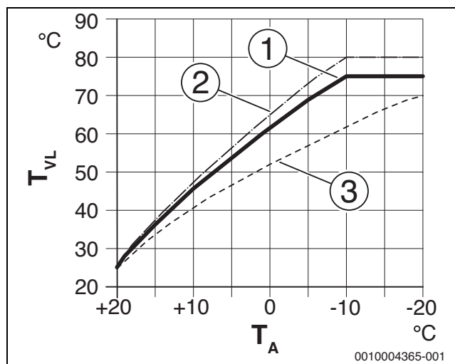
Bild 70 Einstellung der Heizkurve für Heizkörper Steigung über Auslegungstemperatur T_{AL} und minimale Außentemperatur T_{A,min}
