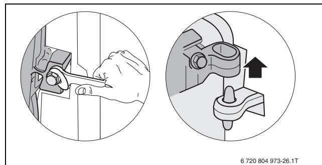
Bild 10 Feuerraumtür demontieren
