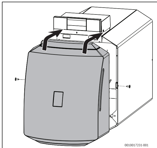
Bild 65 Brennerhaube montieren
