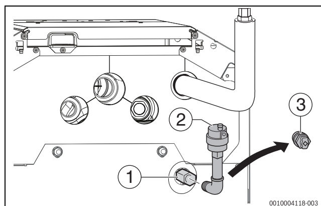
Bild 32 Entlüftungs-Set anschließen
