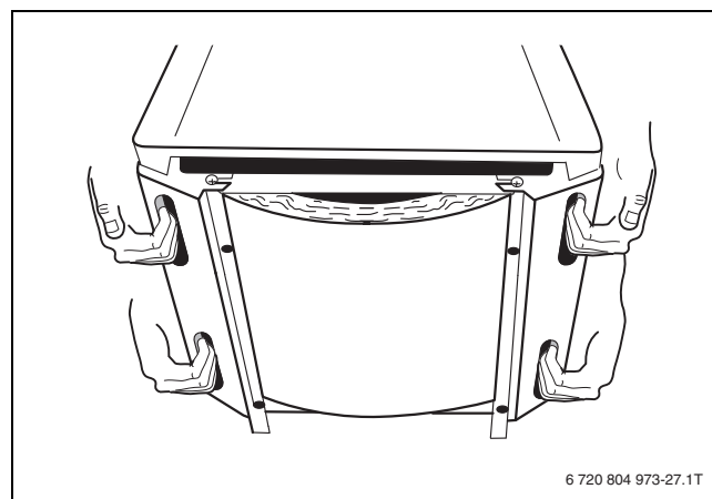
Bild 11 Kessel heben und tragen (18-49 kW)
