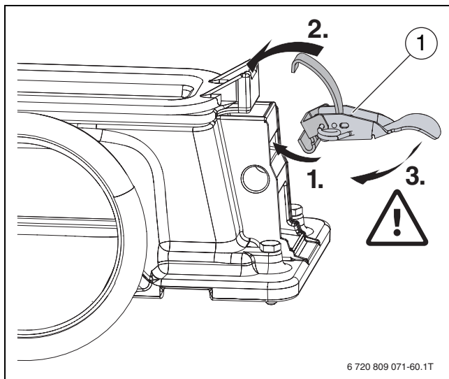
Bild 81 Schnellverschlüsse montieren
