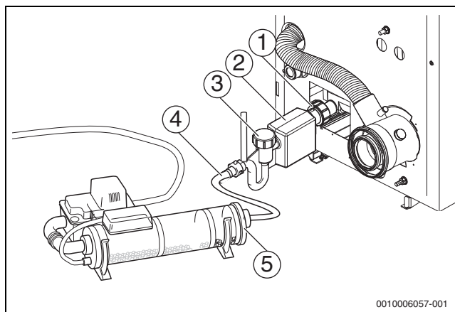
Bild 25 Kondensatablauf mit Neutralisation; dargestellt mit Siphon Version 1
