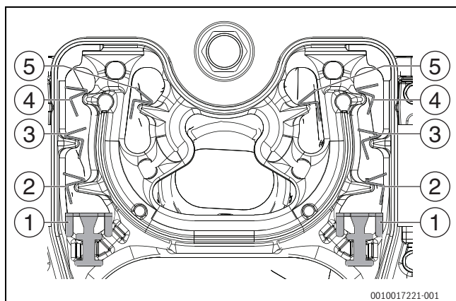
Bild 51 Heizgaslenkplatten 60 kW
