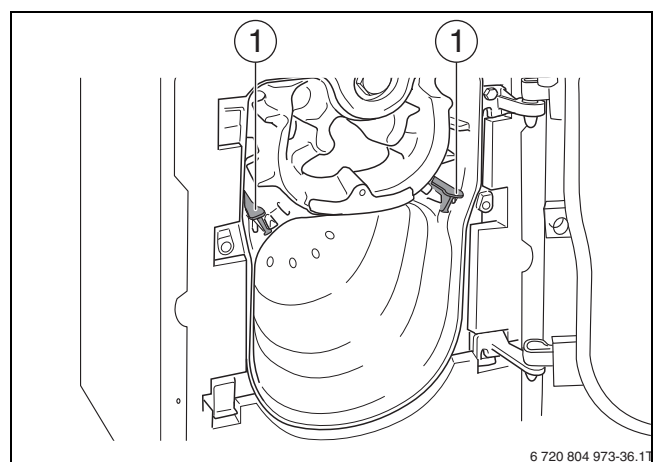
Bild 50 Heizgaslenkplatten 35 kW
