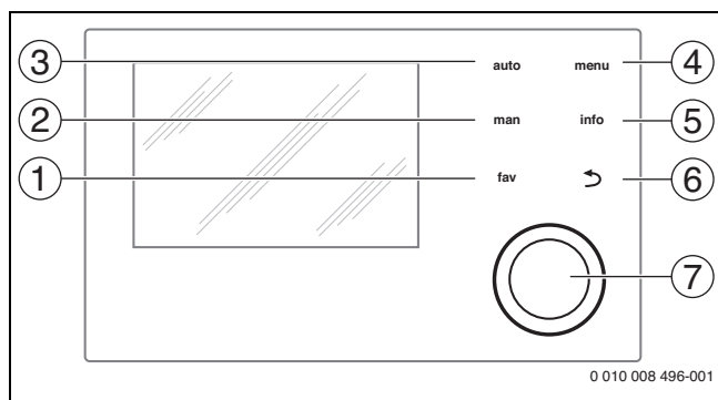
Bild 55 Bedienelemente
