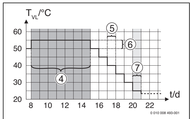
Bild 73 Ablauf der Estrich Trocknung mit den Grundeinstellungen in der Abkühlphase
