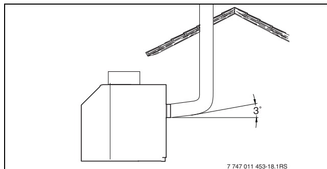
Bild 23 Abgasleitung
