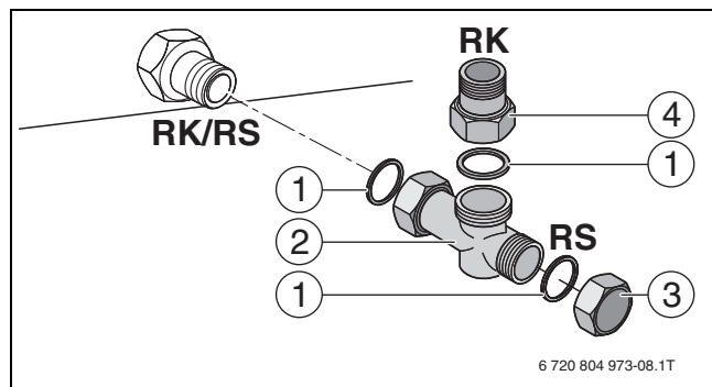
Bild 29 Rücklaufanschlussstück montieren
