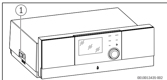
Bild 54 Ein-/Ausschalten
