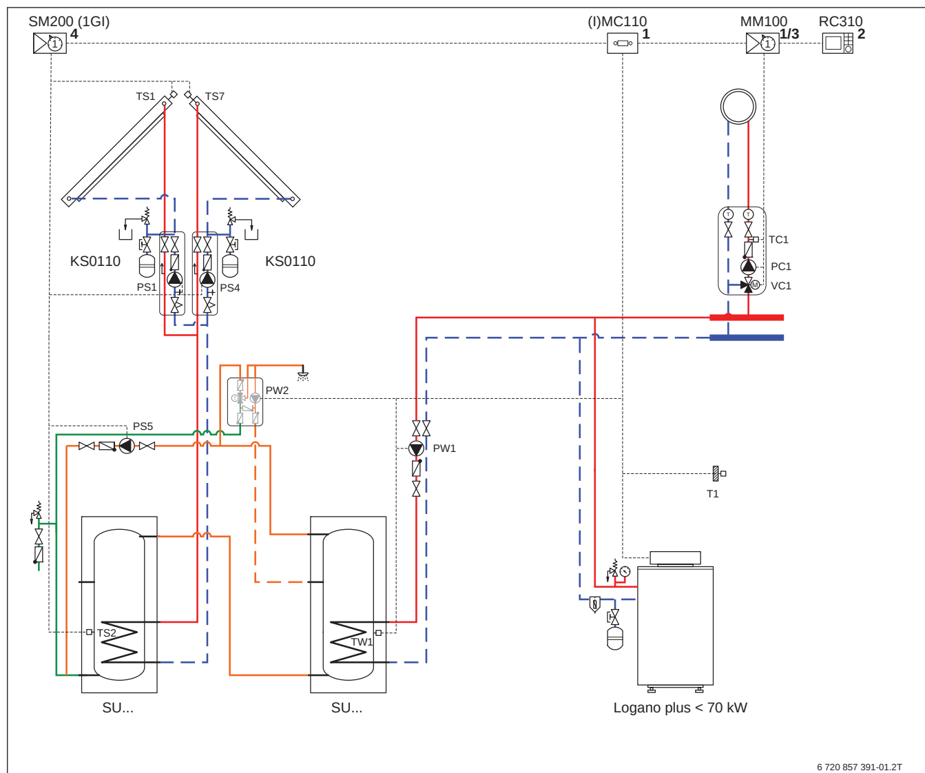
Bild 95 Anlagenbeispiel einer 2-Speicher-Anlage als Großanlage mit Vorwärm Speicher und Bereitschaftsspeicher; Steuerung der Speicherumladung und thermische Desinfektion gemäß DVGW-Arbeitsblatt W551 durch SM100
