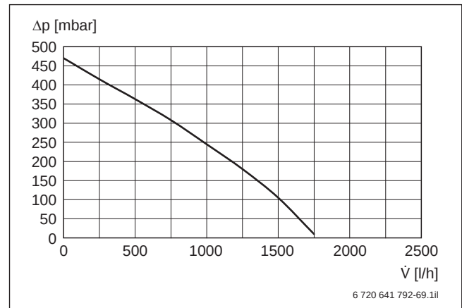
Bild 24 Restförderhöhe SBL
