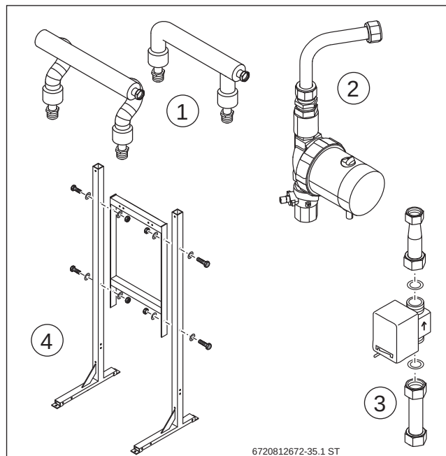
Bild 56 Zubehör für die Frischwasserstationen
