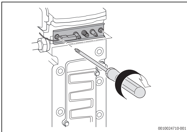
Bild 66 Elektroden-Set montieren
