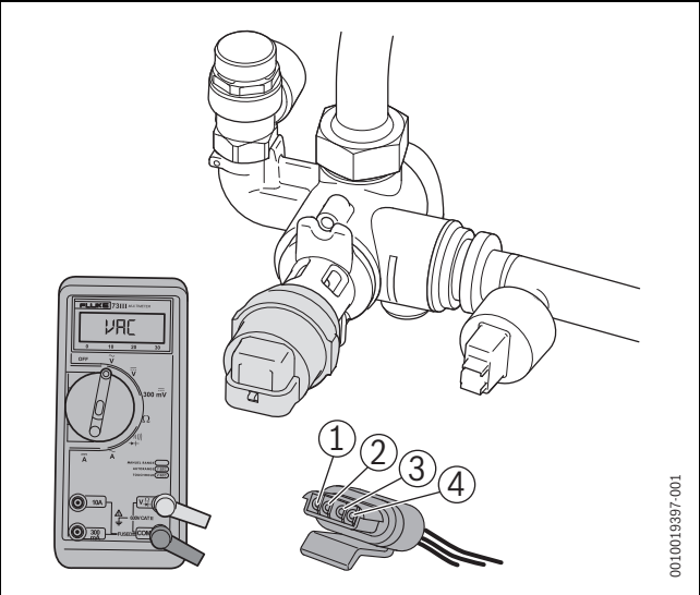
Bild 77 3-Wege-Ventil
