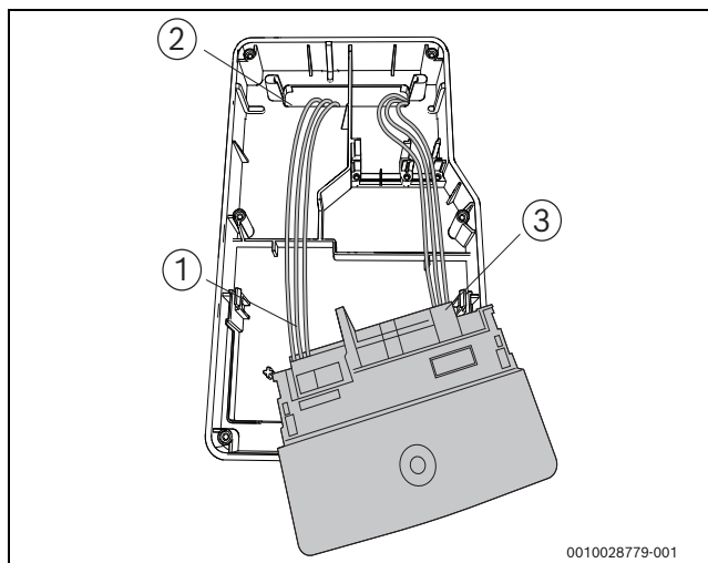
Bild 51 Funktionsmodul anschließen
