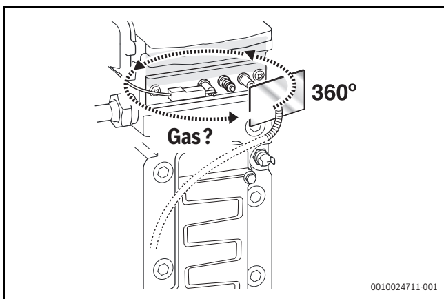
Bild 67 Dichtheitsprüfung
