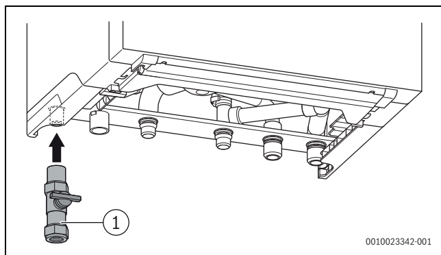
Bild 13 Gasanschluss herstellen
