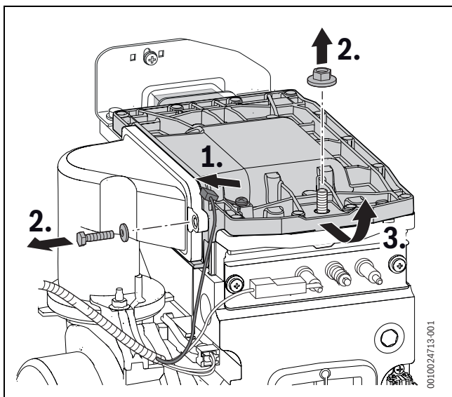
Bild 68 Brennerdeckel ausbauen
