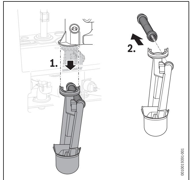
Bild 72 Kondensatsiphon
