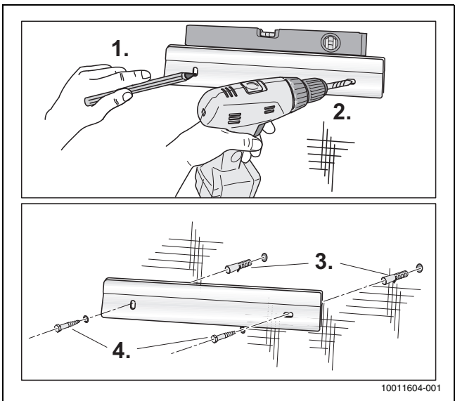
Bild 11 Aufhängeschiene montieren
