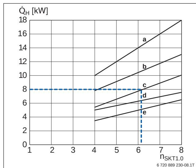
Bild 130 Diagramm zur überschlägigen Bestimmung der Kollektoranzahl Logasol SKT1.0 für Warmwasserbereitung und Heizungsunterstützung (Beispiel hervorgehoben)
