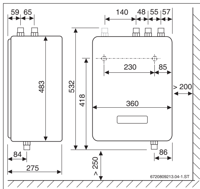
Bild 54 Abmessungen (Maße in mm)
