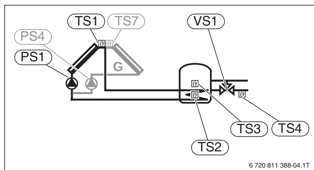
Bild 108 Hydraulikschema 1AG mit Solar-Funktionsmodul SM200 für 2 Kollektorfelder (Ost-/West-Schaltung)
