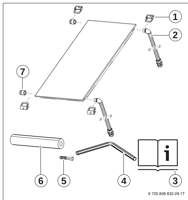
Bild 220 Anschluss-Set Logasol SKT1.0 Indach
