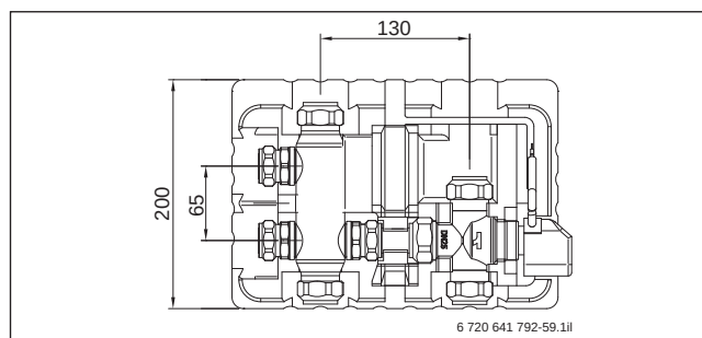
Bild 89 Abmessungen SBU (Maße in mm)
