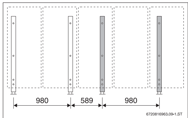
Bild 235 Grundaufstellung für 2 Kollektoren und Erweiterung für 3 Kollektoren, Maße in mm
