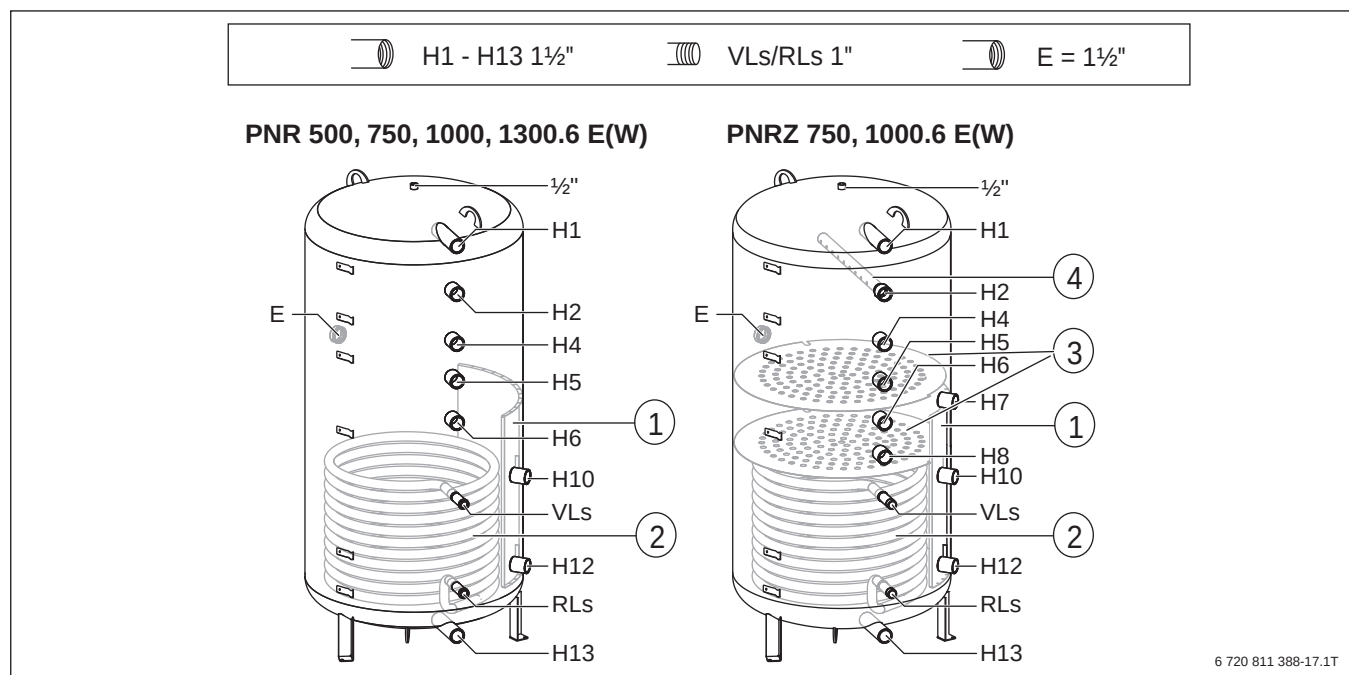
Bild 33 Aufbau und Anschlüsse PNR(Z)....6 E
