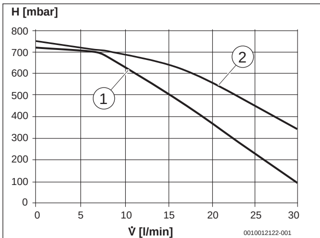
Bild 55 Restförderhöhe Primärkreispumpe
