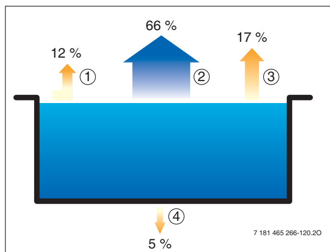
Bild 136 Wärmeverluste Schwimmbecken
