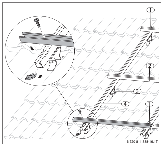
Bild 176 Aufdachmontage-Set für senkrechte Kollektoren mit Schneelastprofil und Zusatzschiene
