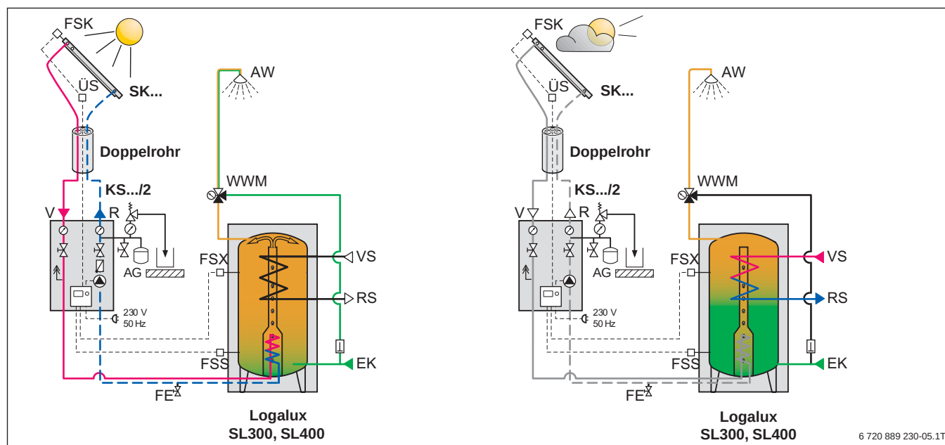
Bild 76 Funktionsschema der solaren Warmwasserbereitung mit der Temperaturdifferenzregelung SC20/2 und Flachkollektoren bei eingeschalteter Solaranlage (links) und konventioneller Nachheizung bei unzureichender Sonnenstrahlung (rechts)
