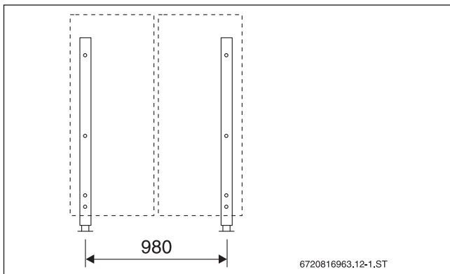
Bild 232 Grundaufstellung für 2 Kollektoren, Maße in mm
