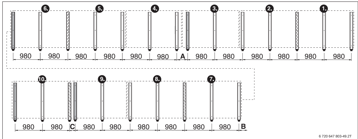
Bild 197 Grundaufführung: Abstände Kollektorstützen bei Verwendung von Beschwerungswannen für 10 waagerechte Kollektoren SKN4.0-w (Angaben in mm), Zusatzstützen in grau
