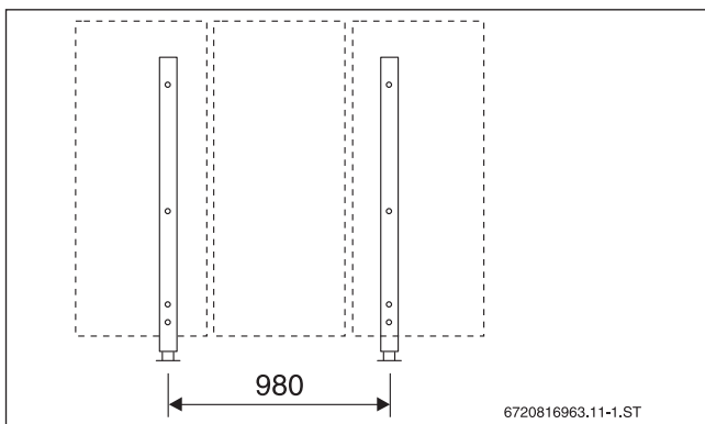
Bild 233 Grundaufstellung für 3 Kollektoren, Maße in mm
