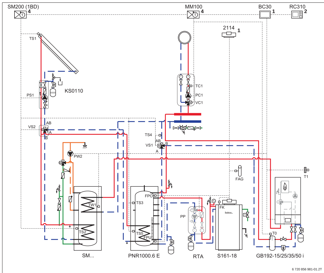
Bild 124 Schaltbild mit Kurzbeschreibung (Allgemeine Hinweise und Abkürzungsverzeichnis → Tabelle 46, Seite 84)
