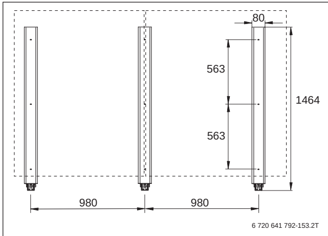
Bild 200 Abstände der Kollektorstützen bei Grundausführung für 2 senkrechte Kollektoren Logasol SKN4.0-s oder SKT1.0-s, Maße in mm
