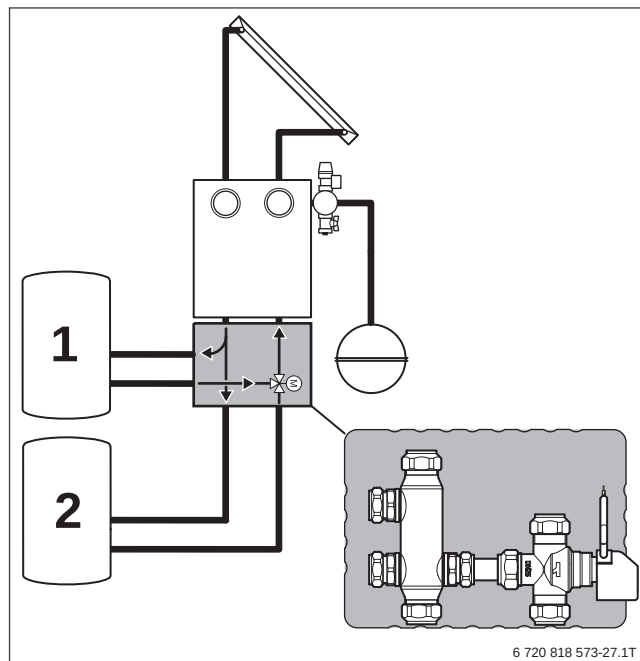
Bild 88 Anlagenschema mit Umschaltmodul SBU
