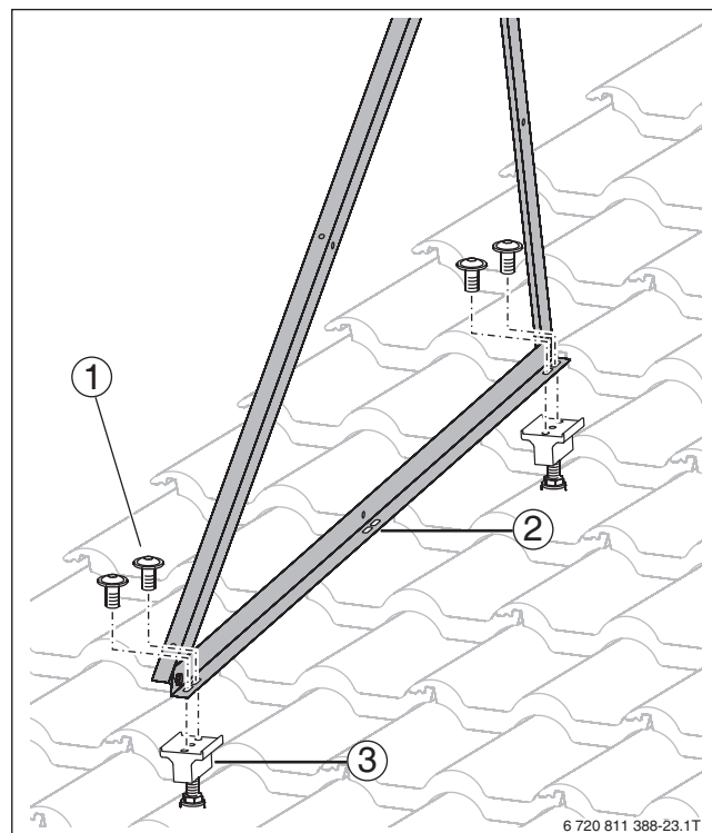
Bild 187 Aufständerung für Flachkollektoren in Verbindung mit Stockschrauben
