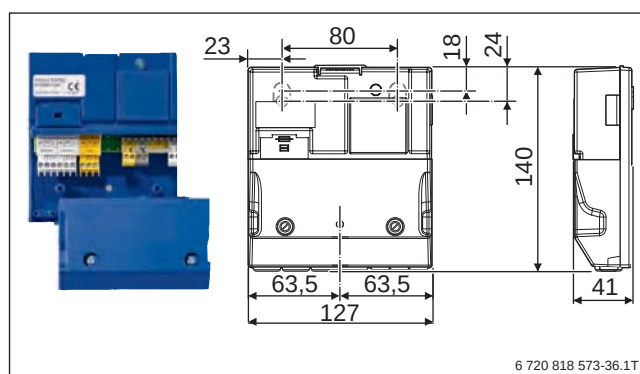
Bild 81 Solar-Funktionsmodul SM50 mit Abmessungen (Maße in mm)
