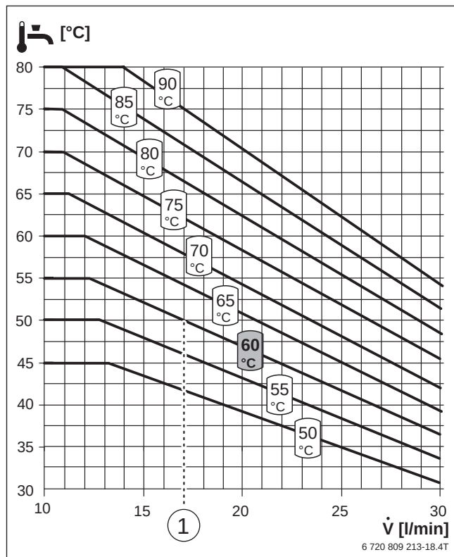
Bild 133 Temperaturverhalten Frischwasserstation
