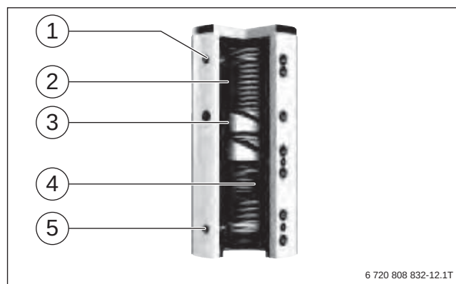
Bild 30 Aufbau Kombispeicher HS; Abmessungen, Anschlüsse und technische Daten → Seite 29
