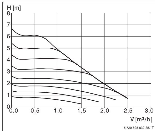
Bild 50 Kennlinie der integrierten Solarpumpe
