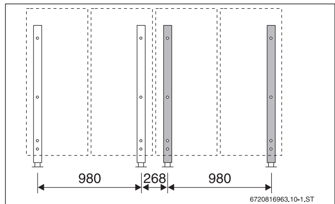
Bild 234 Grundaufstellung für 2 Kollektoren und Erweiterung für 2 Kollektoren, Maße in mm
