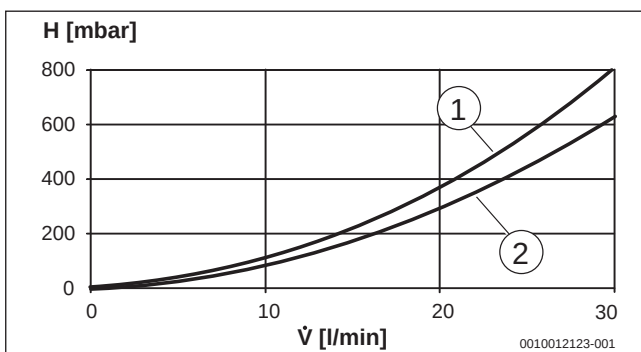
Bild 56 Druckverlust Sekundärseite
