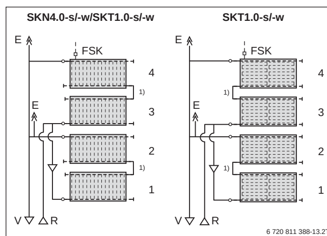
Bild 143 Verschaltung von 4 waagerechten Kollektoren übereinander
