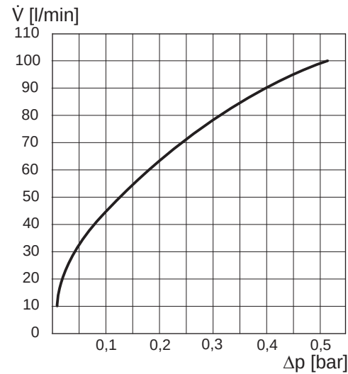
Bild 92 Druckverlust VS-SU und HZG-Set
