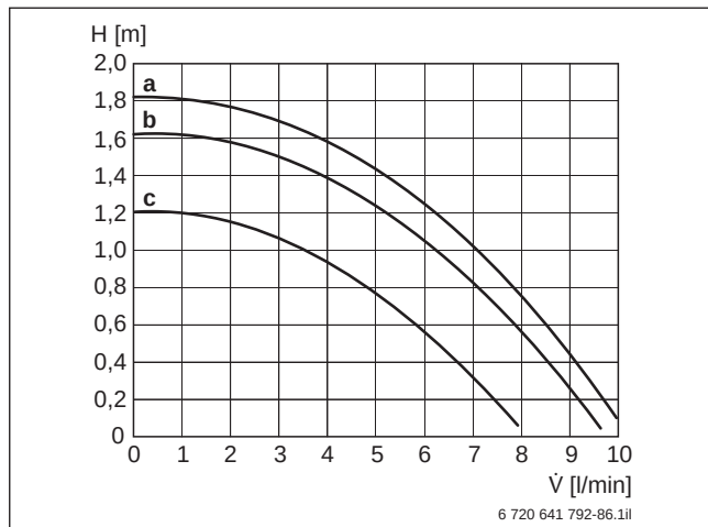
Bild 75 Restförderhöhe Zirkulationspumpe
