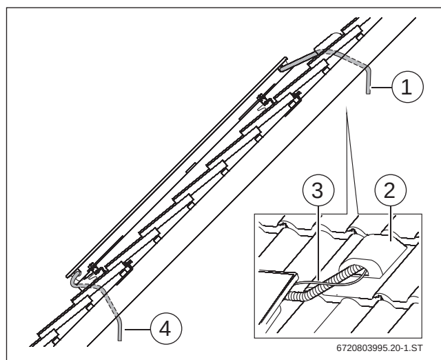
Bild 181 Anschlussrohr durch das Dach führen
