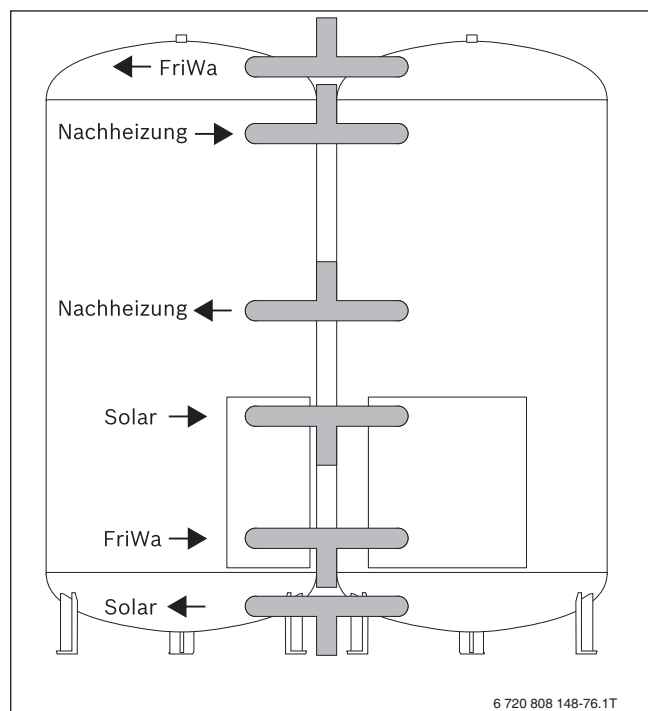
Bild 44 2 Logalux PR....6 mit Kaskadierungssets mit R\ 1\frac{1}{2} T-Stück
