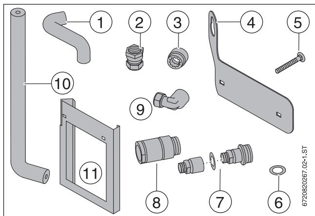
Bild 61 Lieferumfang Speichermontage-Set
