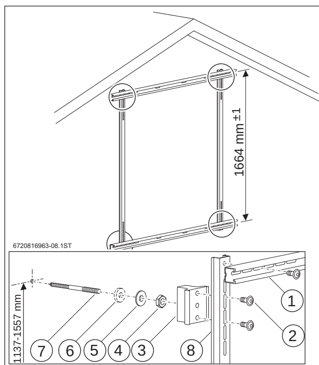
Bild 246 Aufdach-Schienen-Set mit dem Stockschauben-Set an der Fassade montieren
