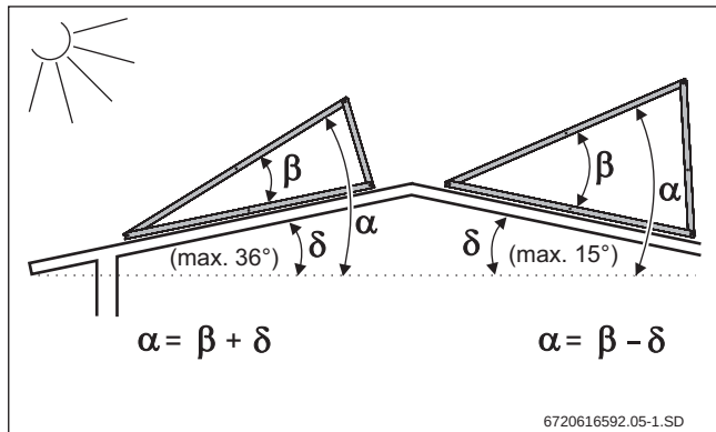
Bild 186 Anstellwinkel bei geneigten Dächern
