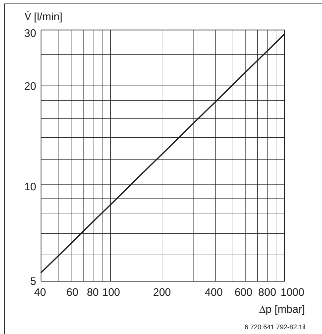
Bild 70 Druckverlust thermostatischer Warmwassermischer R \frac{3}{4} bei 80 °C Warmwassertemperatur, 60 °C Mischwassertemperatur und 10 °C Kaltwassertemperatur
