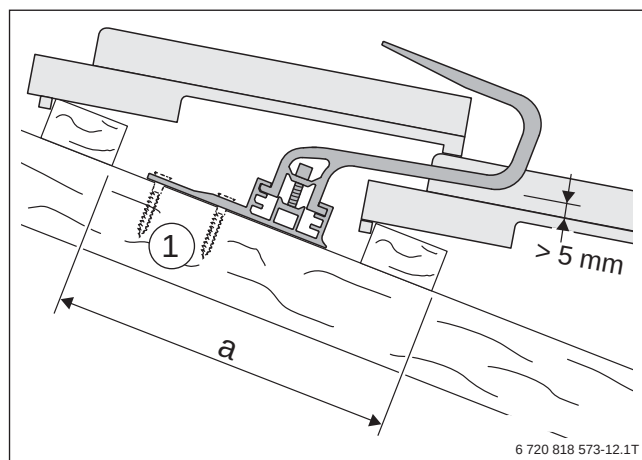
Bild 172 Dachanbindung mit Sparrenanker
