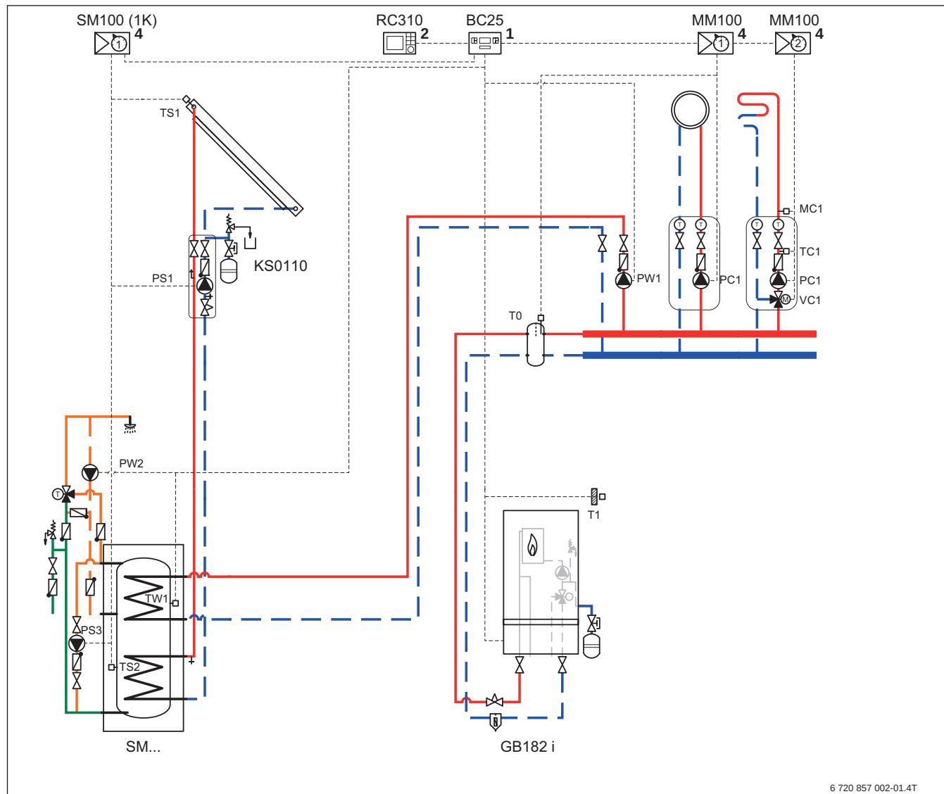
Bild 114 Schaltbild mit Kurzbeschreibung (Allgemeine Hinweise und Abkürzungsverzeichnis → Tabelle 46, Seite 84)
