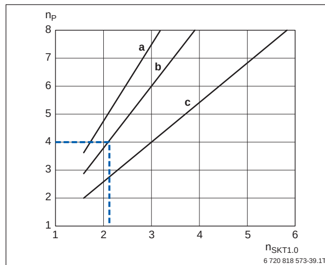
Bild 126 Diagramm zur überschlägigen Bestimmung der Kollektoranzahl Logasol SKT1.0 zur Warmwasserbereitung (Beispiel hervorgehoben)
