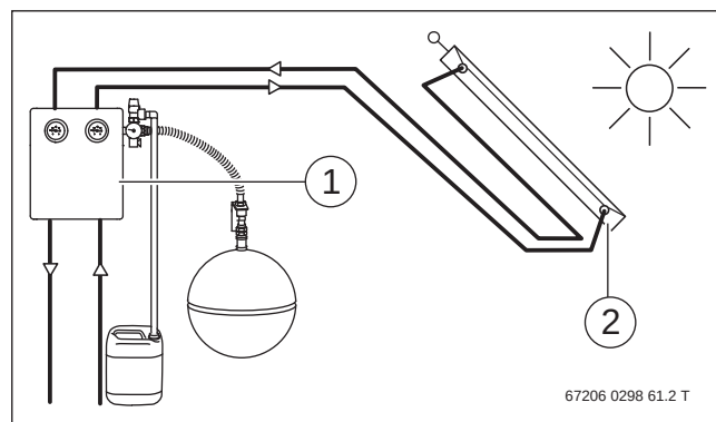
Bild 64 Beispiel: Dachheizzentrale
