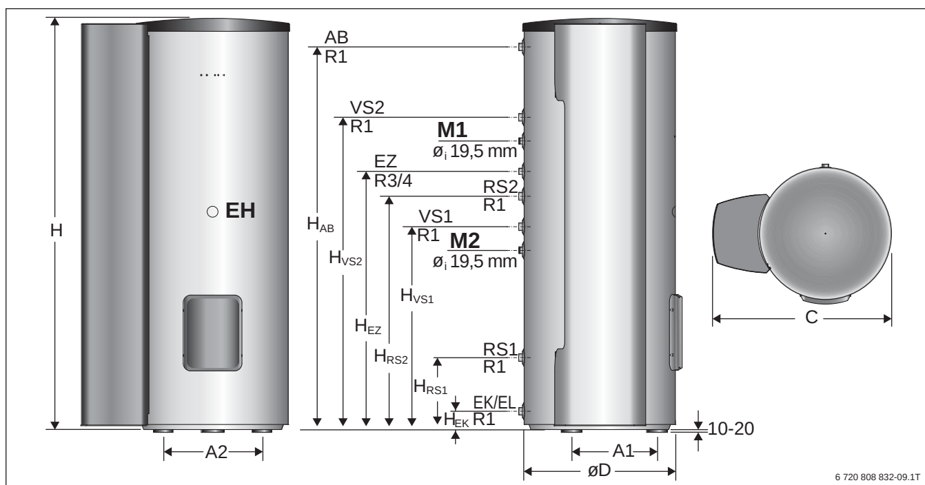
Bild 19 Abmessungen und Anschlüsse Logalux ESM300 E, SMS290/5 E und SMS400/5 E
