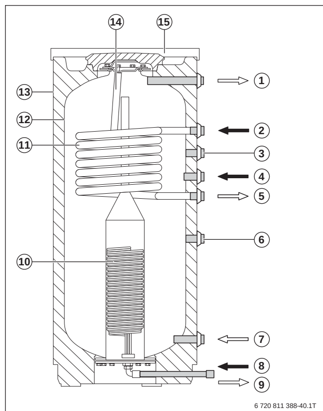
Bild 22 Aufbau Logalux SL300; Abmessungen, Anschlüsse und technische Daten → Seite 21
