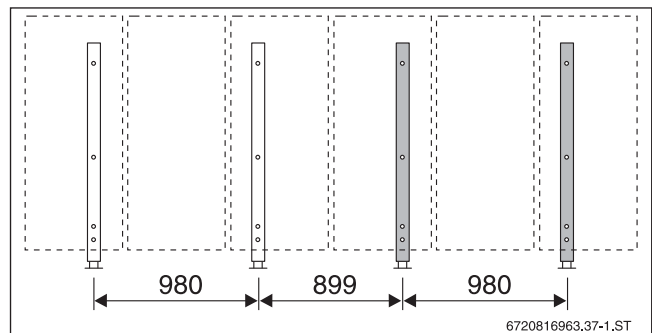
Bild 236 Grundaufstellung für 3 Kollektoren und Erweiterung für 3 Kollektoren, Maße in mm
