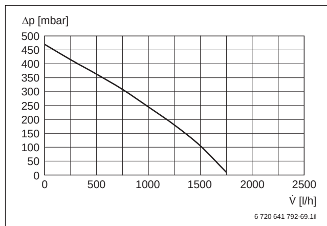
Bild 102 Restförderhöhe SBL
