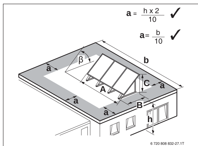
Bild 188 Einzuhaltende Abstandsmaße
