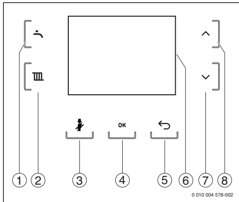
Bild 3 Bedienfeld
