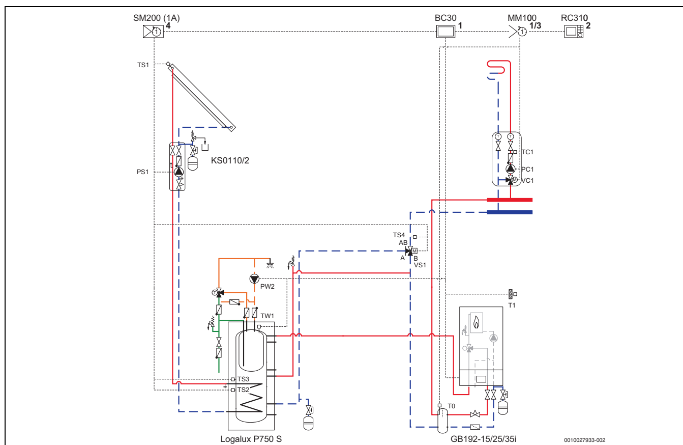
Σχ. 8 Παράδειγμα διαγράμματος υδραυλικής σύνδεσης με θερμαντήρα νερού Kombi P750 S σε συνδυασμό με ηλιακό σύστημα και συμβατικό επίτοχο λέβητα αερίου
