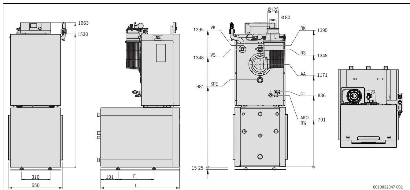
Bild 7 Abmessungen und Anschlüsse Logano plus KB195i BZ mit Logamatic und Logalux L135-200.3 RS (Maße in mm)
