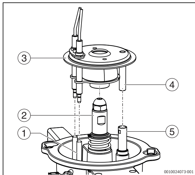
Bild 70 Mischsystem montieren
