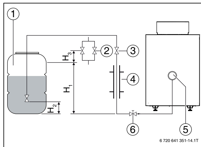
Bild 29 Installationsbeispiel
