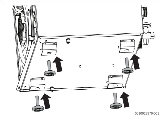
Bild 13 Stellfüße montieren
