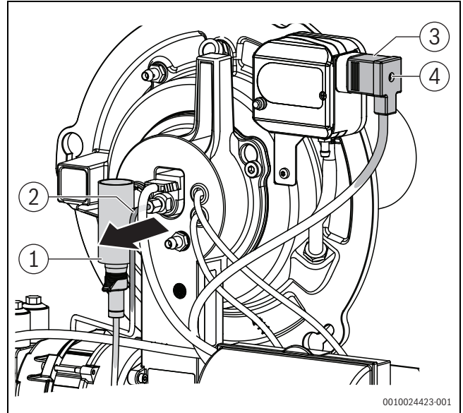
Bild 72 Ölleitung herausziehen
