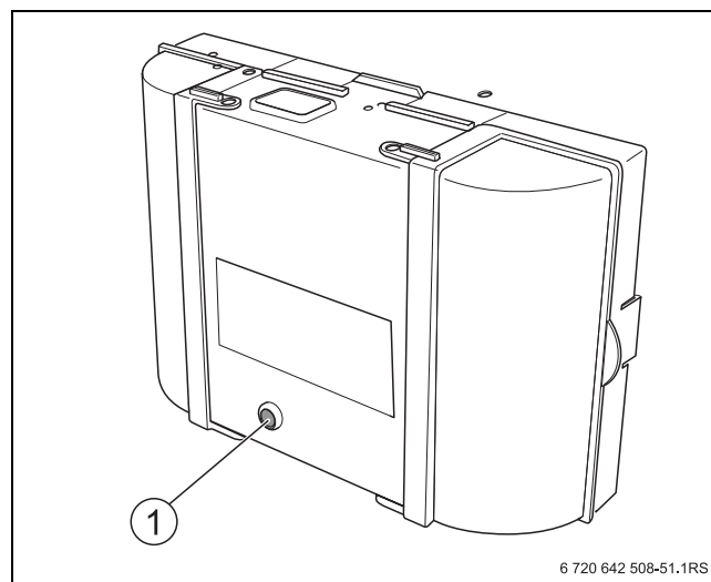
Bild 51 Entstörtaste am Feuerungsautomaten
