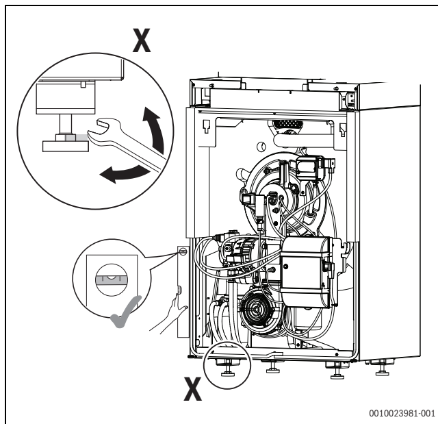
Bild 14 Heizkessel ausrichten
