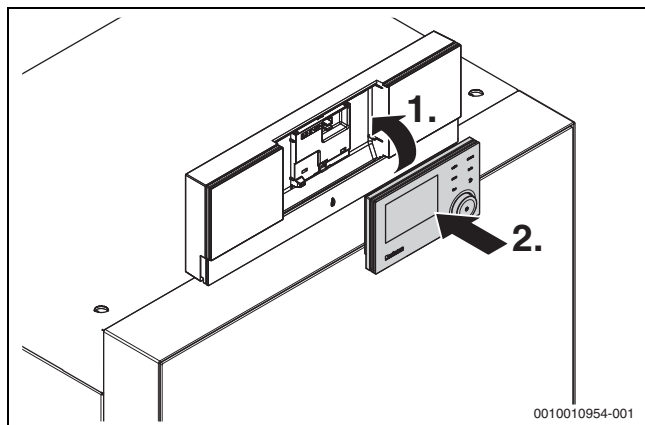
Bild 48 Bedieneinheit montieren
