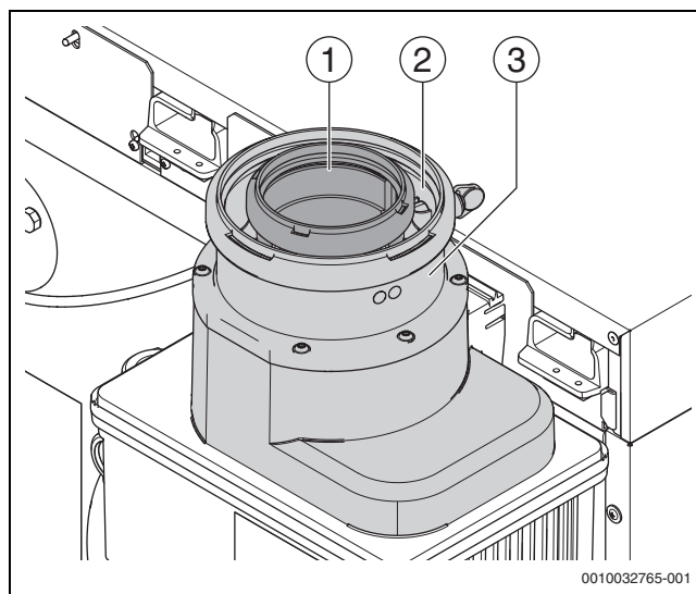
Bild 16 Abgasanschluss montieren
