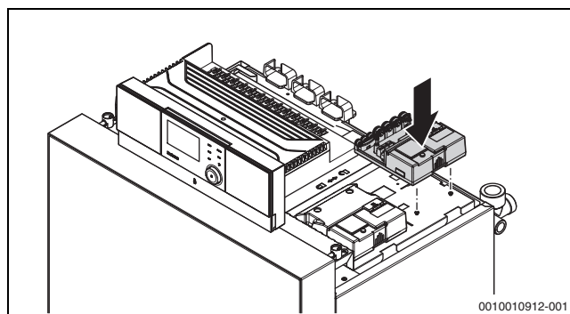
Bild 45 Funktionsmodul aufsetzen
