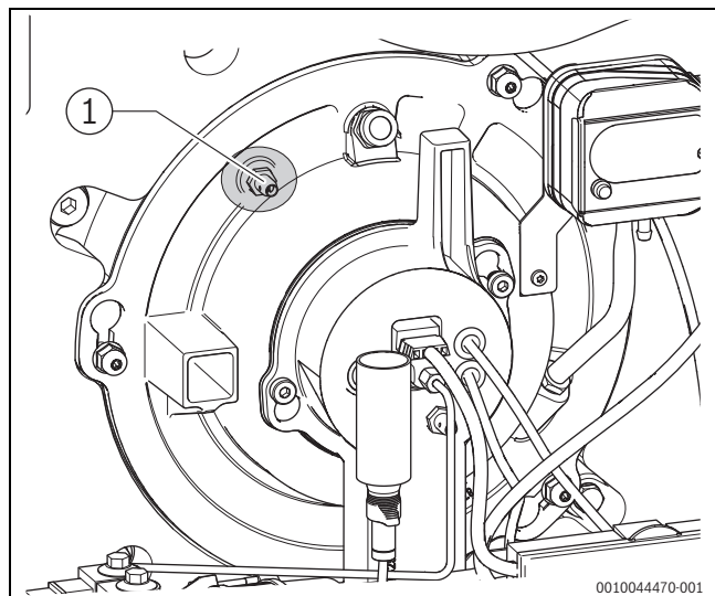
Bild 79 Druckmessstelle am Brenner
