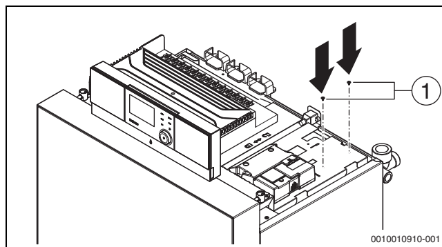
Bild 44 Schrauben eindrehen
