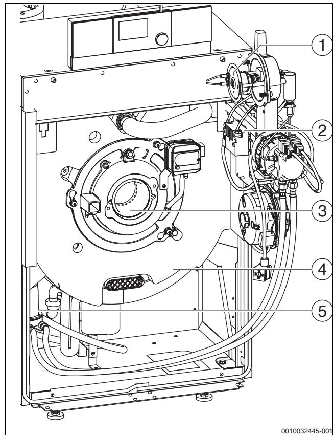
Bild 3 Ölbrenner in Serviceposition 1
