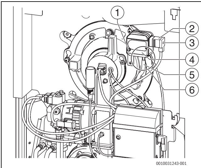
Bild 90 Störung am Druckwächter zurücksetzen
