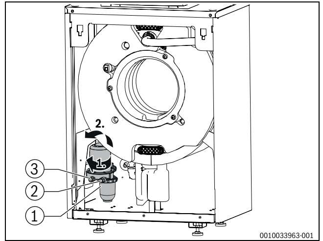
Bild 77 Ölfilter demontieren
