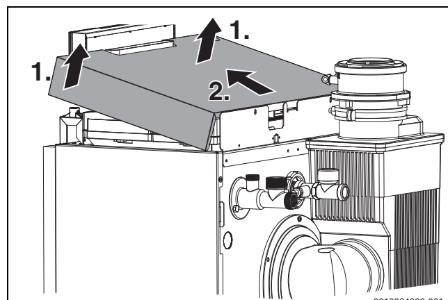
Bild 34 Kesselhaube abnehmen
