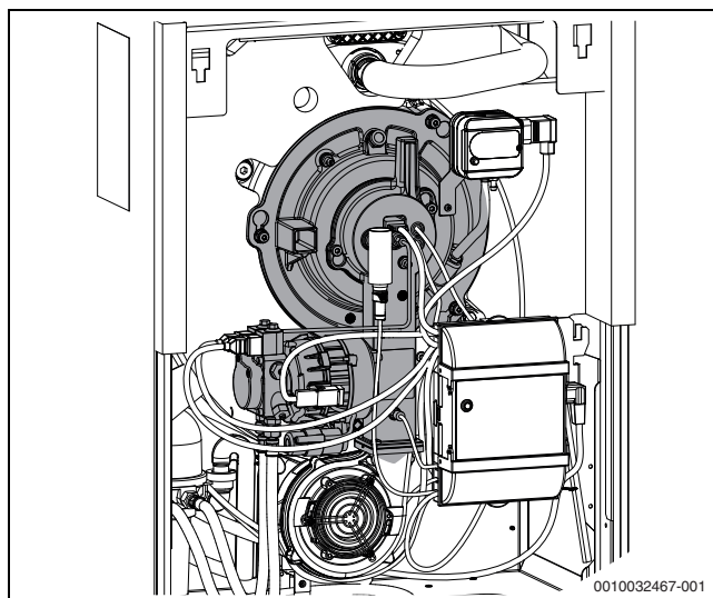
Bild 62 Heiße Bauteile am Brenner/Wärmetauscher
