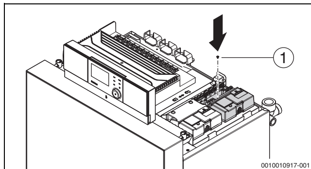
Bild 46 Funktionsmodul verschrauben
