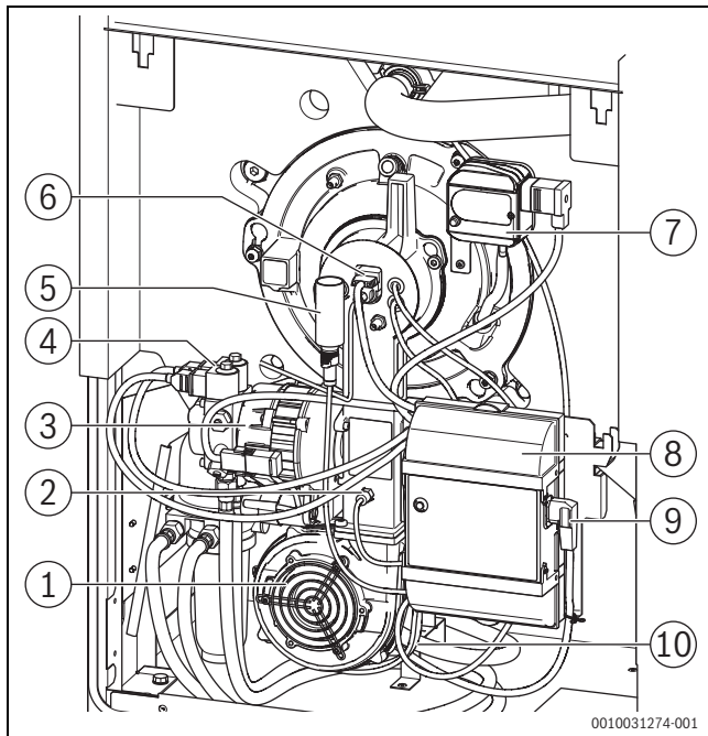
Bild 2 Ölbrenner
