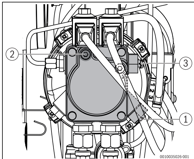
Bild 58 Druck einstellen
