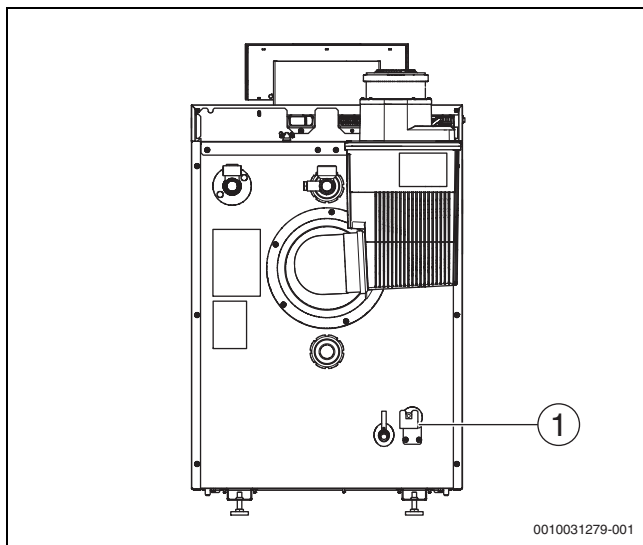
Bild 31 Haltewinkel montieren
