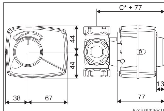
Bild 200 Abmessungen Mischermotor
