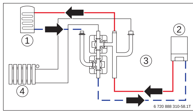
Bild 196 Hydraulik Warmwasserkreis
