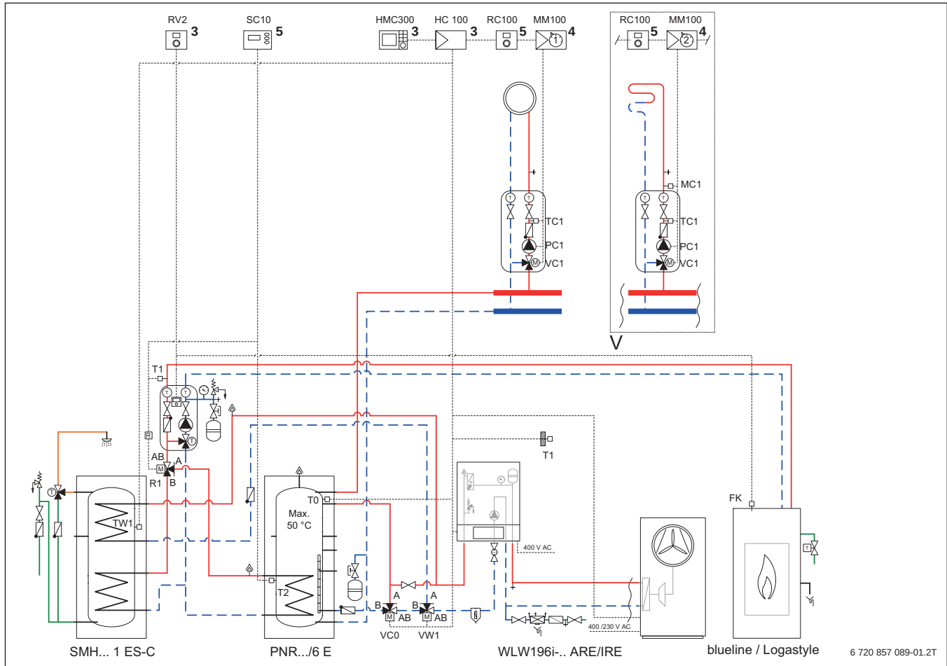
Bild 244 Anlagenschema mit Regelung (unverbindliche Prinzipskizze)
