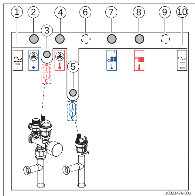
Bild 83 Anschlüsse der Inneneinheit mit ungemischtem Heizkreis
