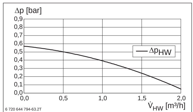
Bild 114 Restförderdruck Logatherm WLW196i-8 IR/AR
