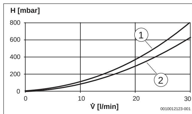
Bild 181 Druckverlust Sekundärseite
