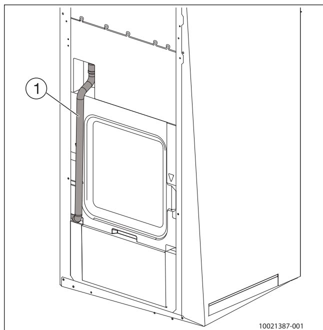
Bild 91 Rückansicht Ablaufschlauch
