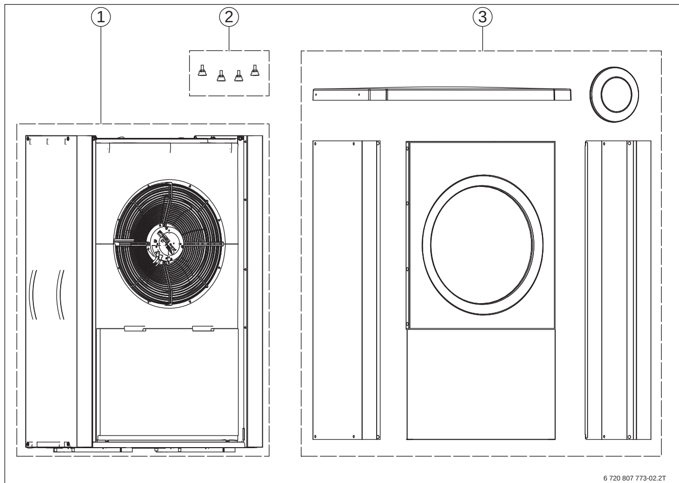
Bild 59 Lieferumfang Außeneinheit ODU4.2i ... ODU14i
