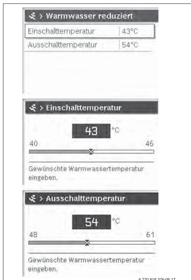
Bild 161 Einstellen der Ein- und Ausschalttemperatur
