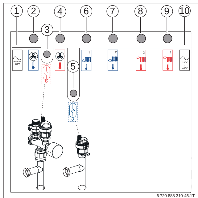
Bild 84 Anschlüsse der Inneneinheit mit 2 Heizkreisen (1 gemischter, 1 ungemischter)
