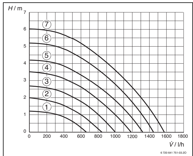
Bild 31 Pumpenkennlinien
