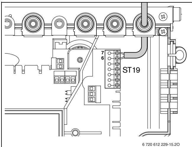
Bild 17 Anschluss Module
