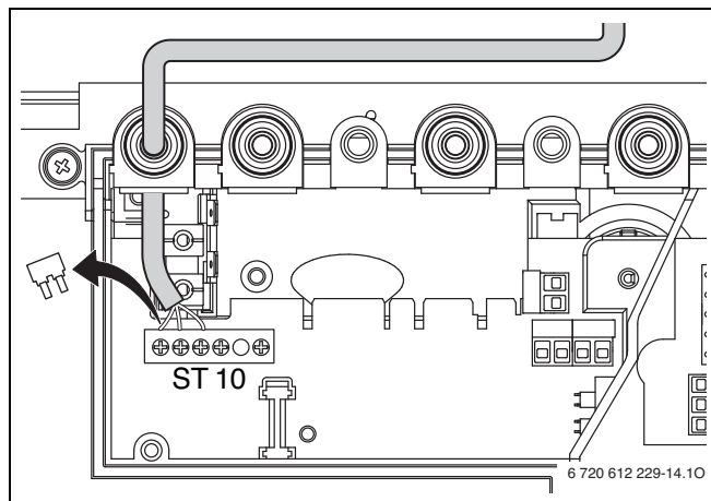
Bild 14 Anschluss Easyswitch
