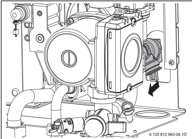
Bild 52 Sicherheitsventil (Heizung)
