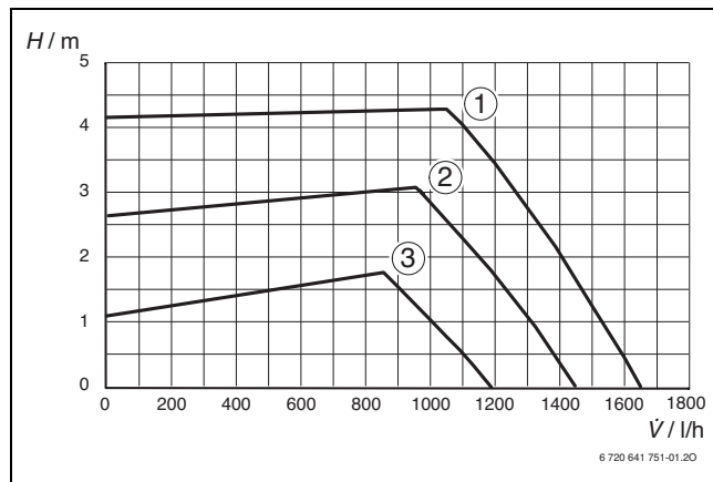
Bild 29 Konstantdruck
