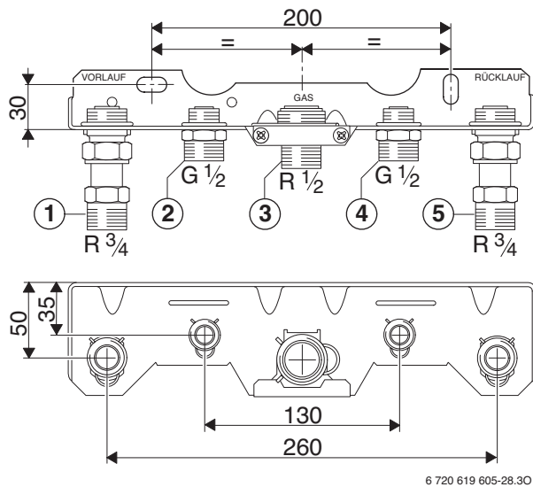
Bild 8 Beispiel: Montageanschlussplatte U-MA
