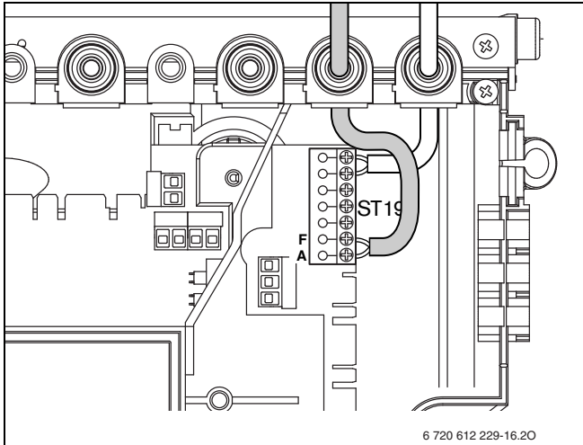
Bild 16 Anschluss Außentemperaturfühler
