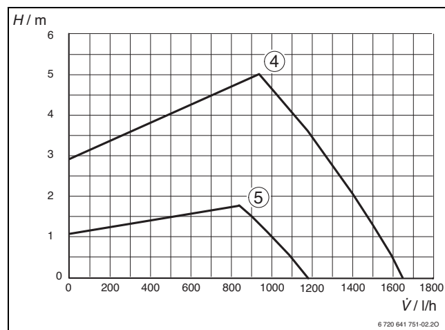
Bild 30 Proportionaldruck
