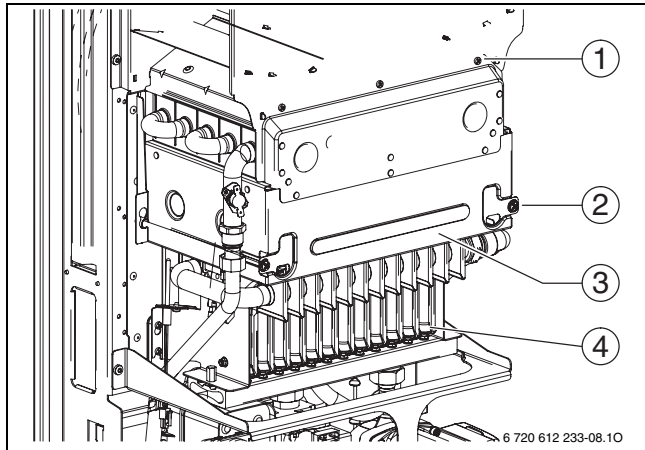
Bild 42 Brenner öffnen
