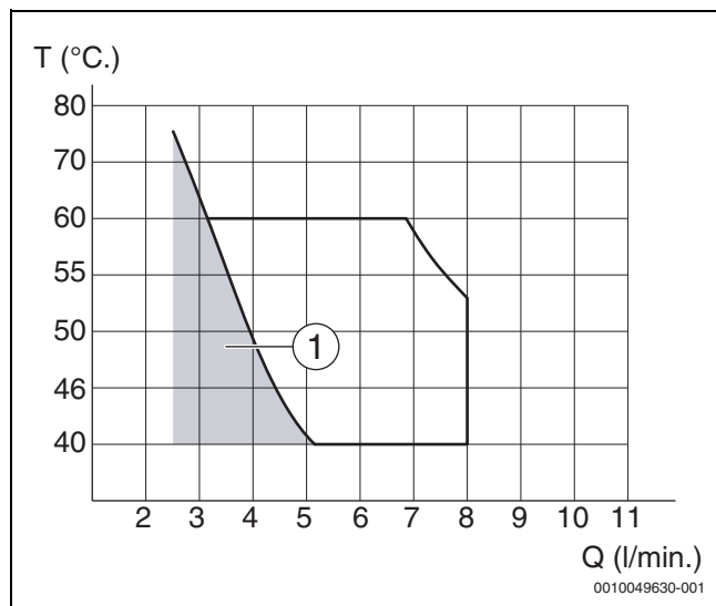
Bild 25 Diagramm für eine Kaltwassereinlauftemperatur von +10°C (U154-24K V2)
