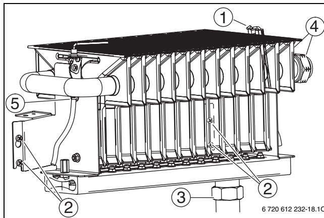
Bild 43 Baugruppe Brenner
