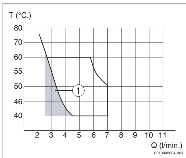
Bild 26 Diagramm für eine Kaltwassereinlauftemperatur von +10°C (U154-20K V2)
