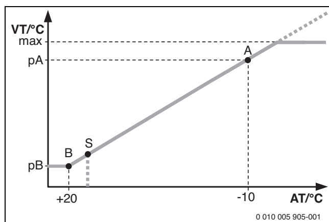
Bild 96 Heizkurve
