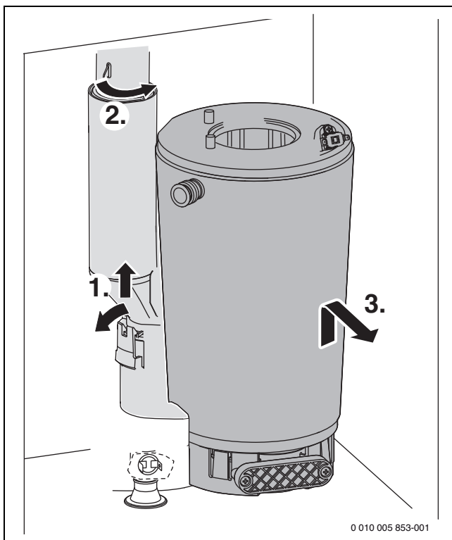
Bild 92 Wärmeblock ausbauen
