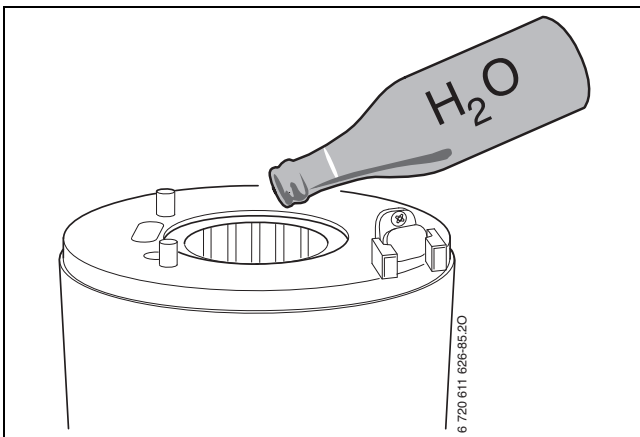
Bild 74 Wärmeblock mit Wasser spülen
