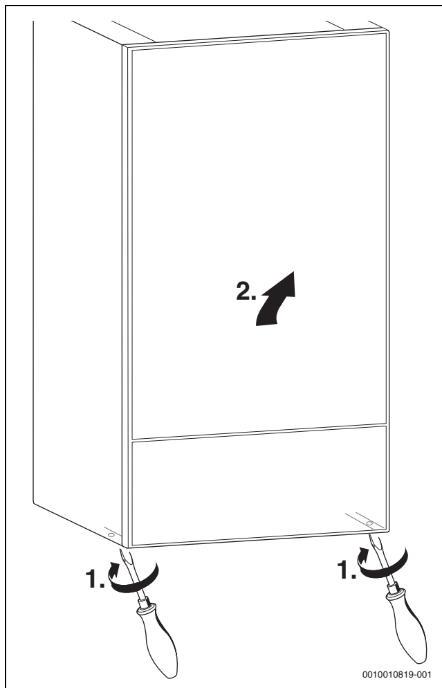
Bild 35 Verkleidung abnehmen
