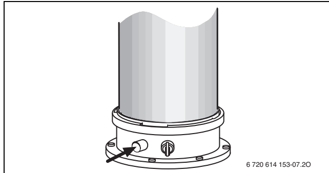
Bild 58 Abgasmessstutzen
