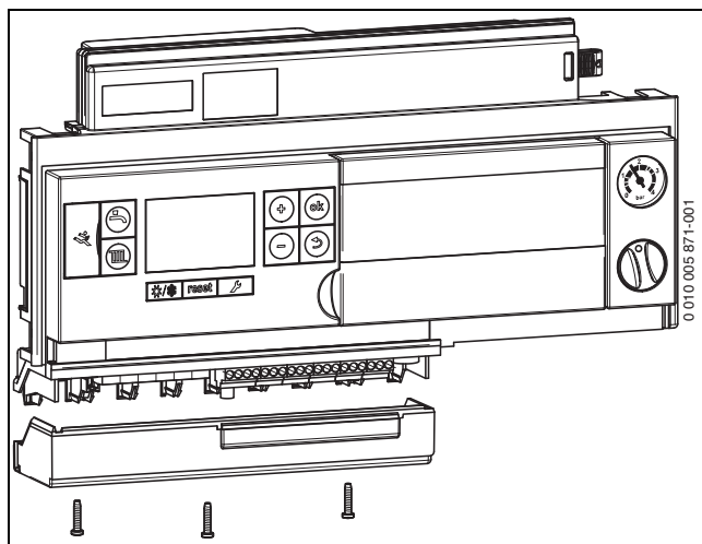
Bild 42 Abdeckung entfernen
