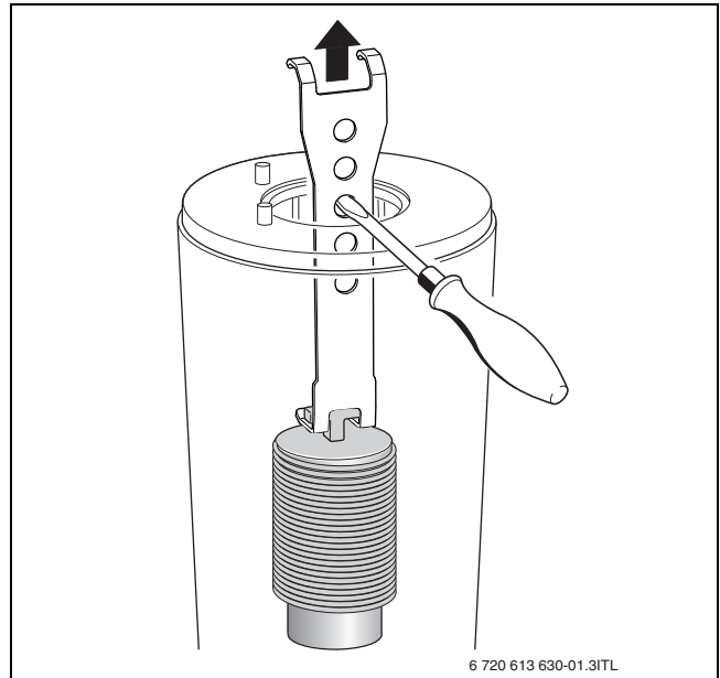
Bild 71 Unteren Verdrängungskörper herausnehmen
