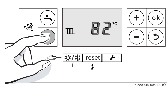
Bild 48 Anzeige Vorlauftemperatur
