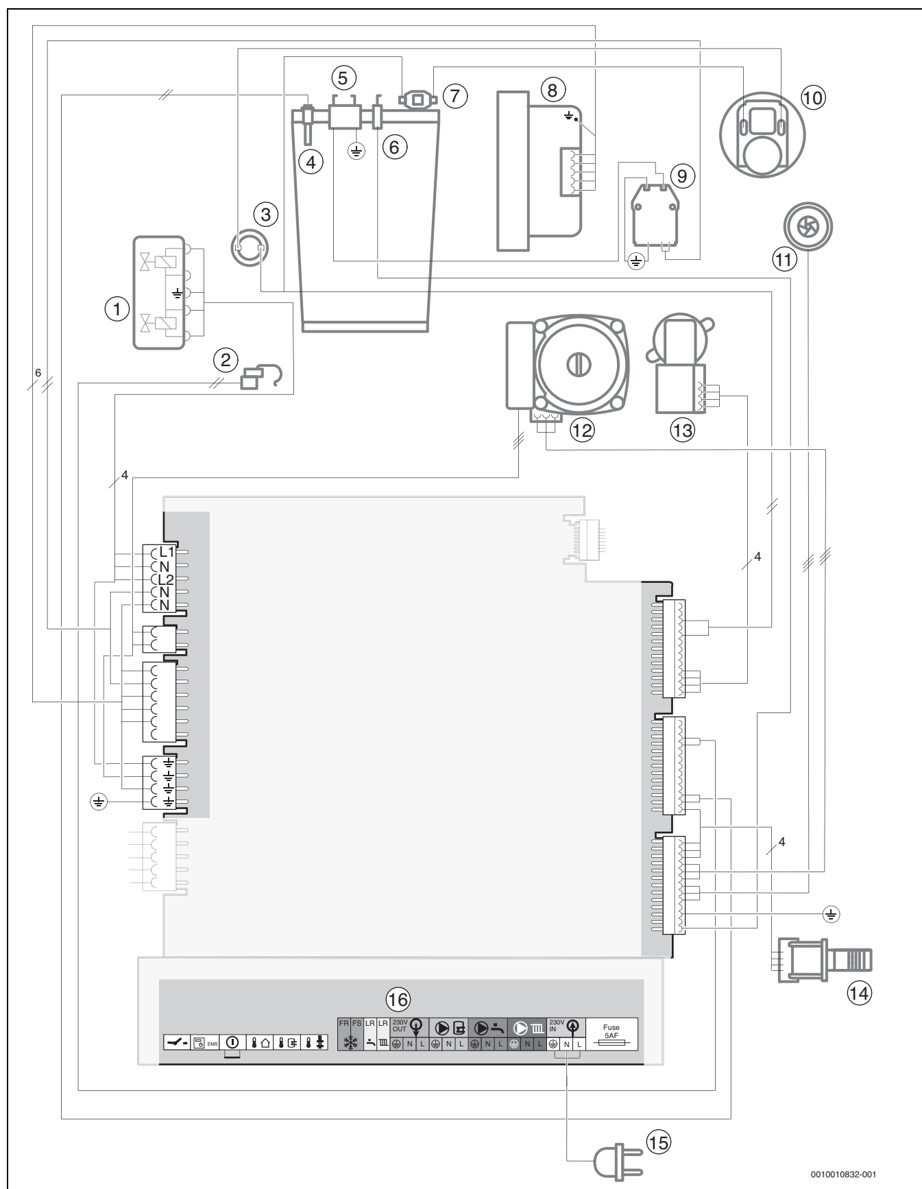
Bild 95 Elektrische Verdrahtung
