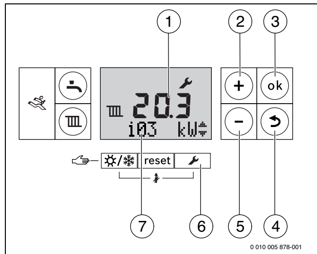
Bild 57 Übersicht der Bedienelemente
