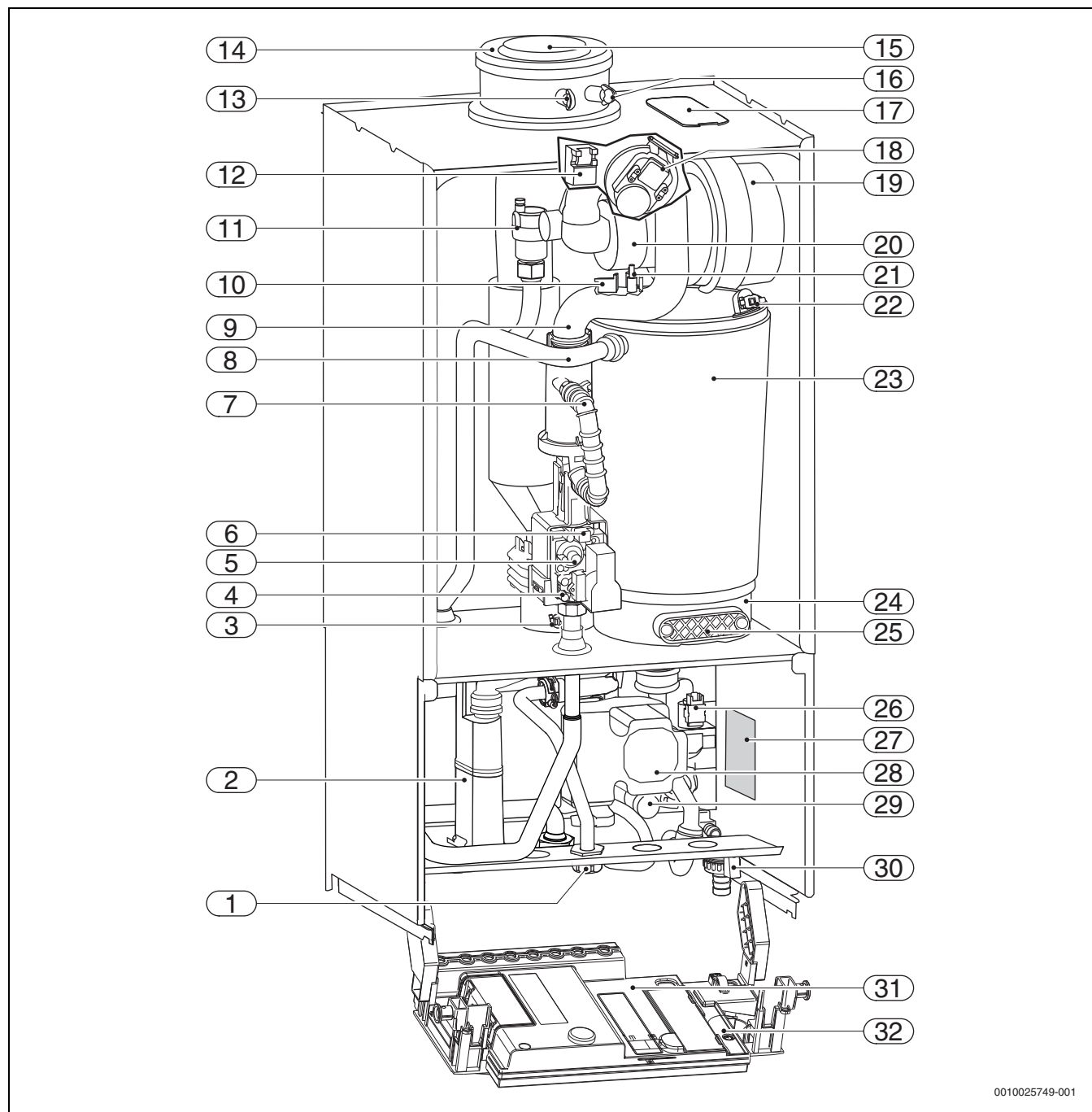
Bild 3 Produktübersicht GB182i..
