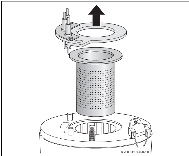
Bild 69 Brenner herausnehmen
