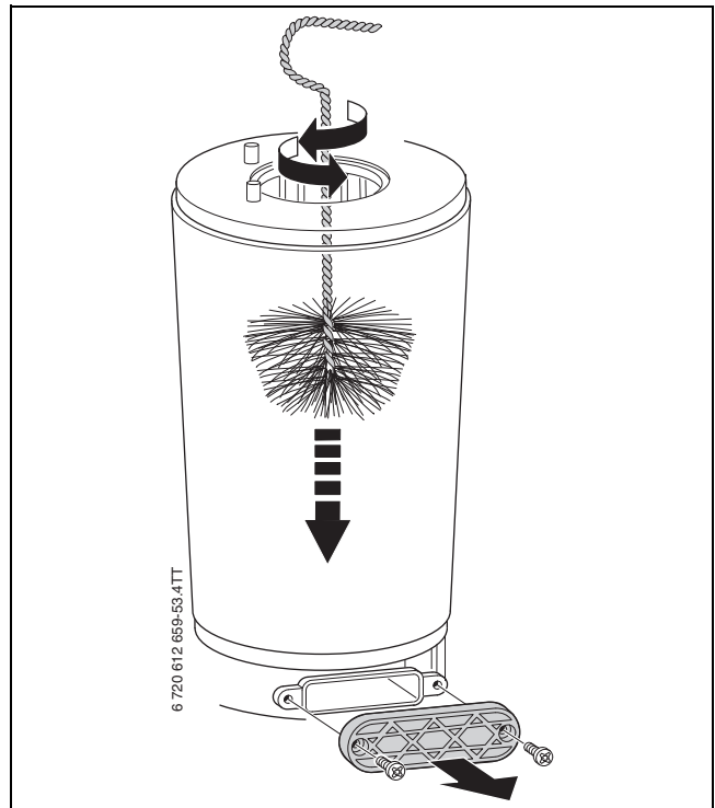
Bild 72 Wärmeblock reinigen
