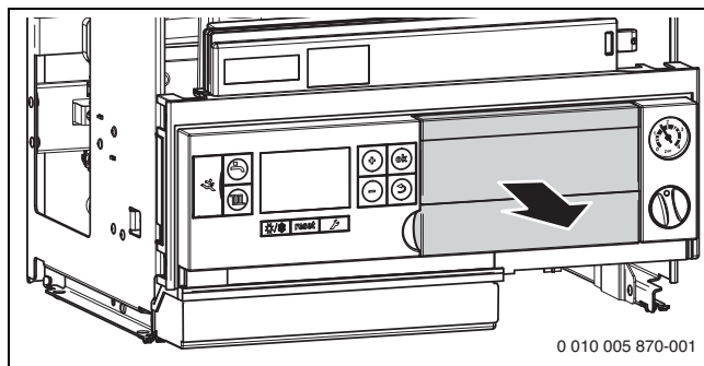
Bild 41 Abdeckung entfernen und Bedieneinheit montieren
