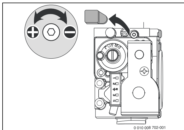
Bild 61 Plombe entfernen
