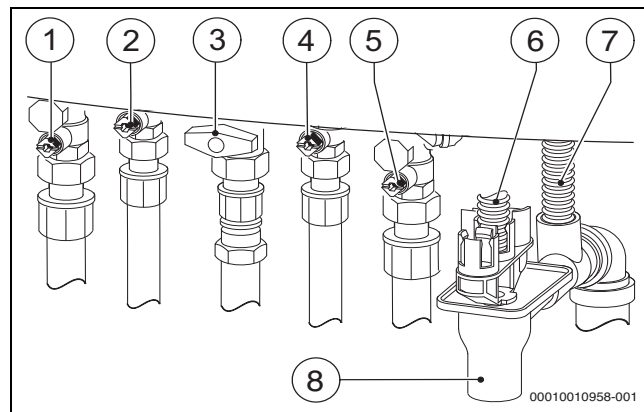
Bild 39 Gas- und wasserseitige Anschlüsse (Zubehör)
