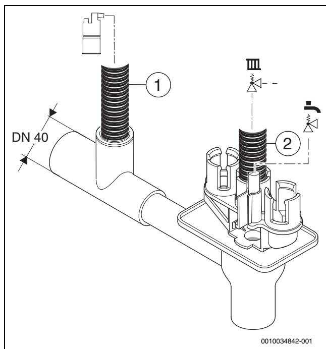
Bild 38 Kondensatschlauch und Schlauch vom Sicherheitsventil am Siphon montieren
