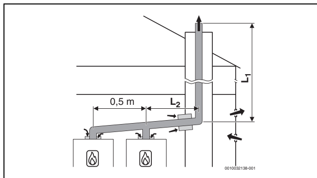
Bild 30 Kaskade mit 2 Geräten:
