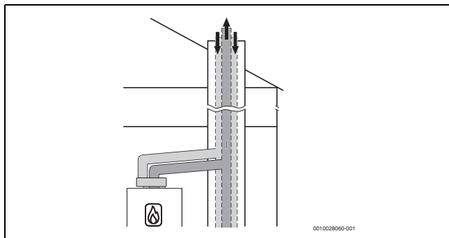
Bild 15 Luft-Abgas-Führung nach C 43 mit getrennten Rohren für Luftzufuhr und Abgasableitung im Aufstellraum
