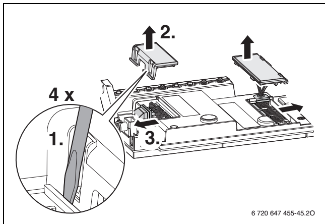
Bild 88 Abdeckung entfernen
