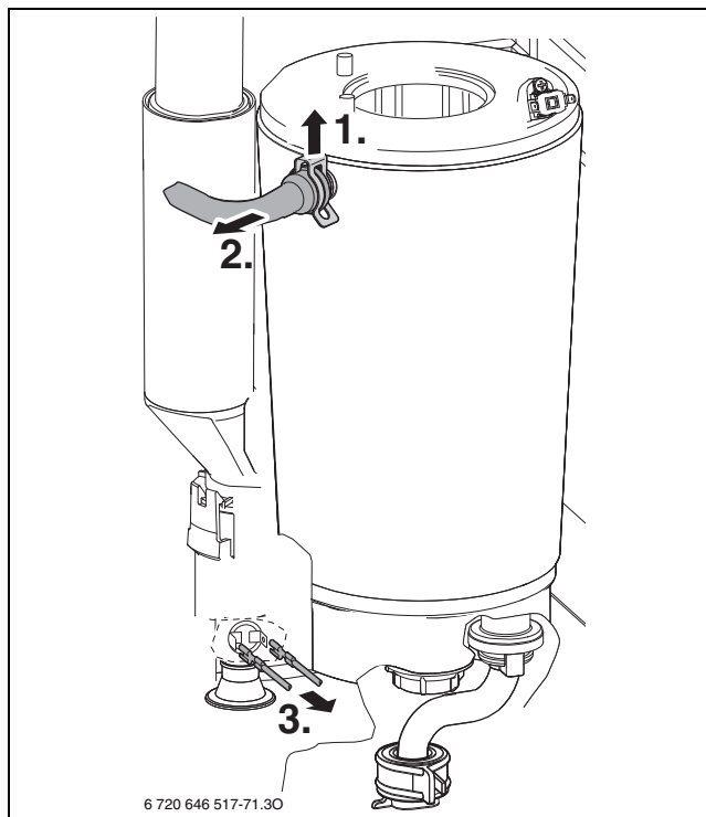
Bild 90 Vorlaufrohr lösen und Kabel abziehen
