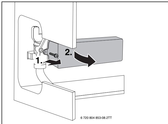
Bild 77 Plattenwärmetauscher ausbauen
