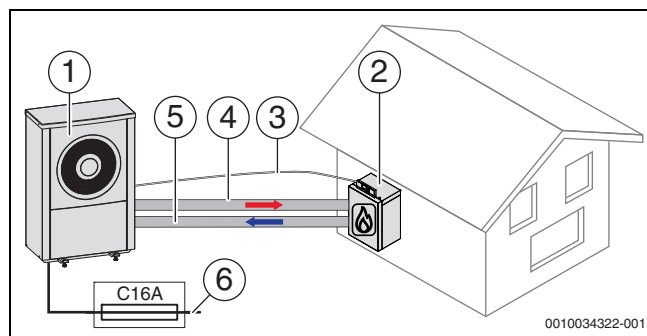
Bild 4 Verbindungsleitungen Außeneinheit zum Brennwert-Hybridsystem
