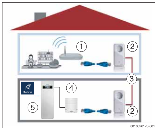
Bild 17 PowerLAN
