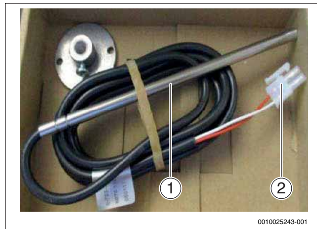
Bild 11 Referenzfühler TL2 mit Anschlusskabel
