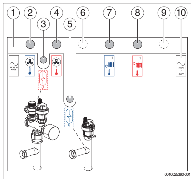
Bild 16 Anschlüsse der Komfort-Hydraulik-Inneneinheit mit 1 ungemischten Heizkreis
