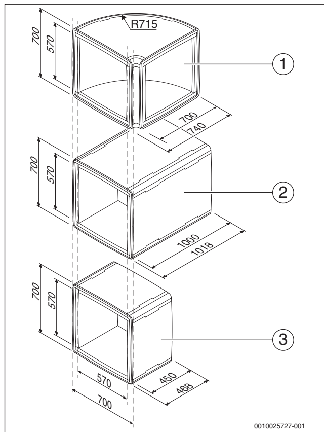
Bild 9 Beispiele für Luftkanäle Querschnitt 700 (alle Maße in mm)
