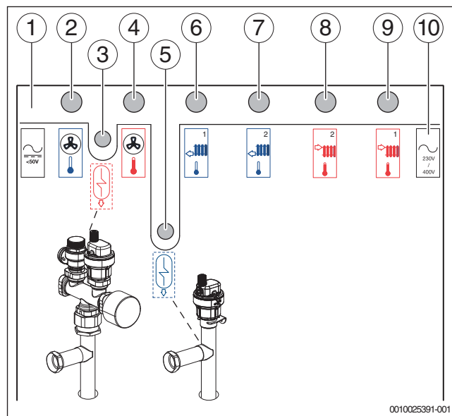
Bild 17 Anschlüsse der Komfort-Hydraulik-Inneneinheit mit 1 ungemischten und 1 gemischten Heizkreis
