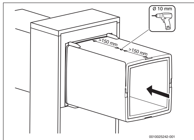
Bild 13 Montage des Referenzfühlers TL2 am Luftansaugkanal
