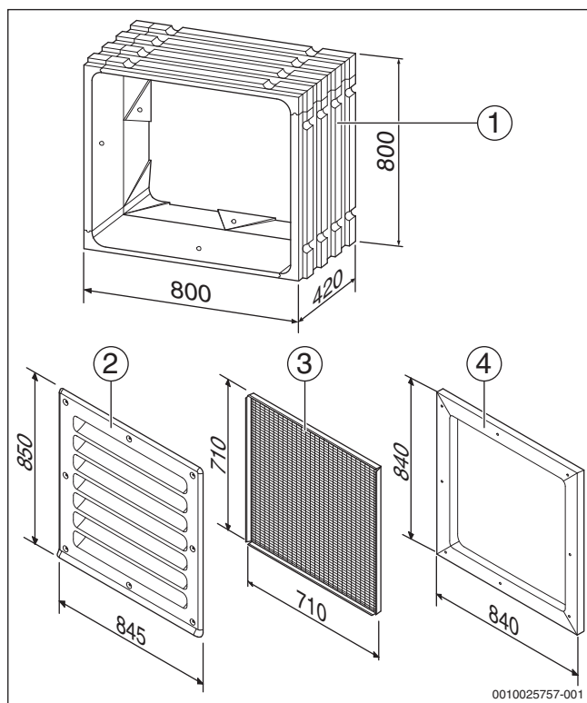
Bild 10 Wandschneidung und Zubehöre
