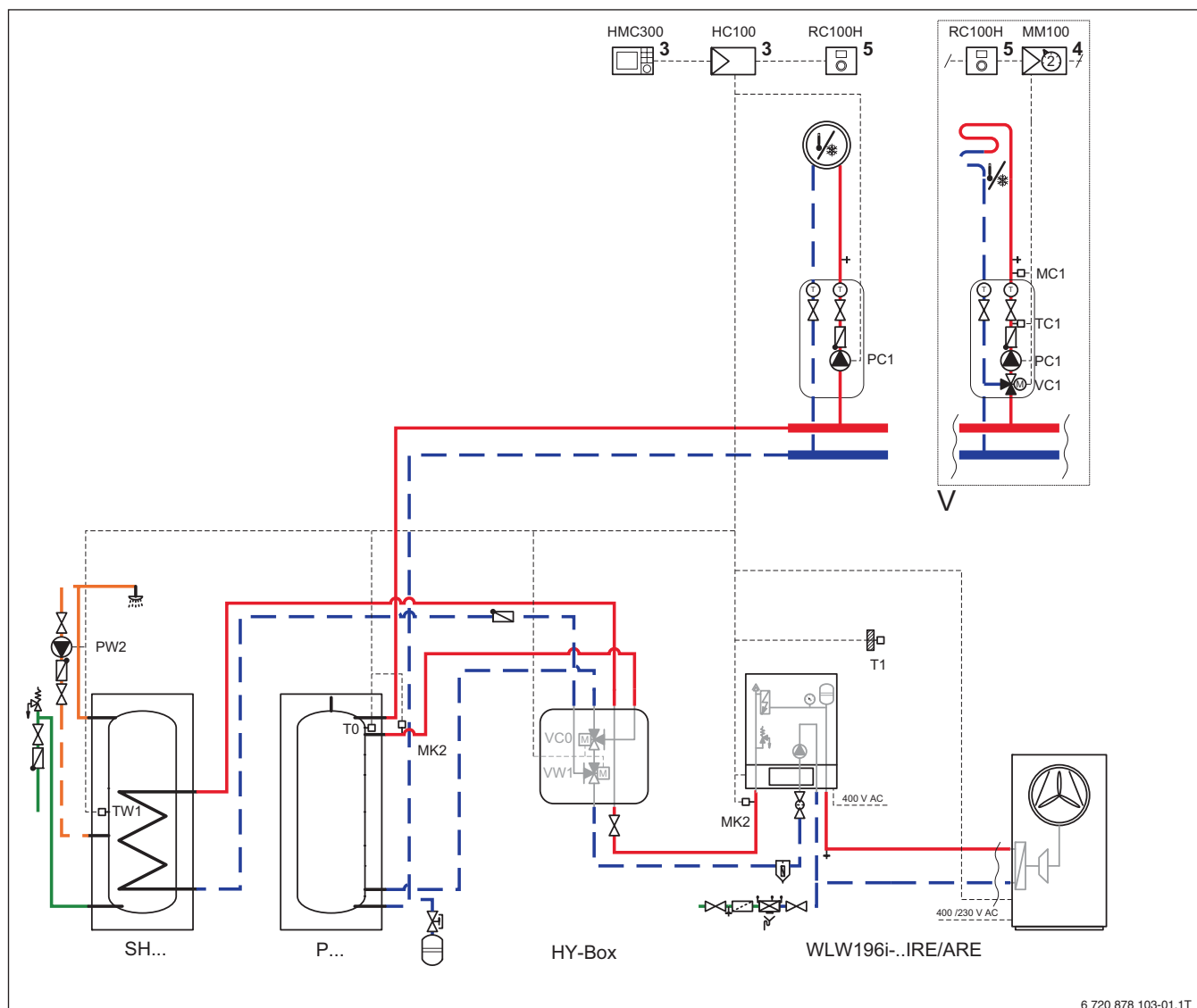
Bild 1 Hydraulik zum Anlagenbeispiel (unverbindliche Prinzipdarstellung)
