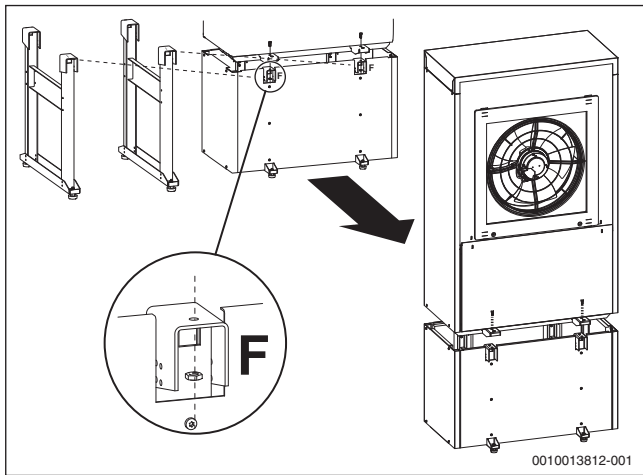
Bild 13 Wärmepumpe auf Sockel stellen
