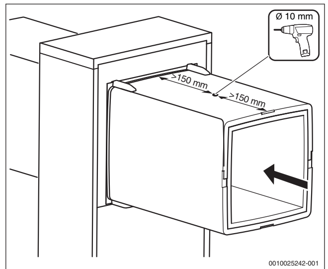
Bild 16 Montage des Referenzfühlers TL2 am Luftansaugkanal
