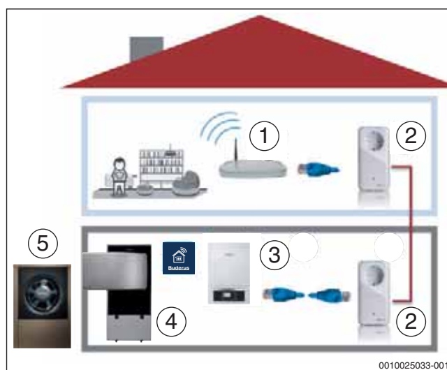
Bild 29 PowerLAN
