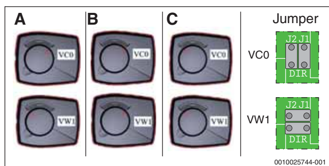
Bild 8 Schalterstellungen der einzelnen Betriebszustände
