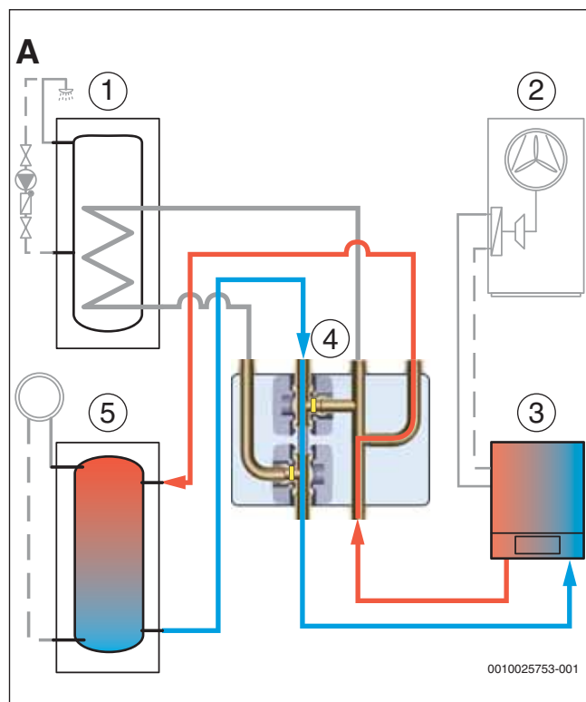
Bild 5 Betriebszustand A: Puffer-Kreis
