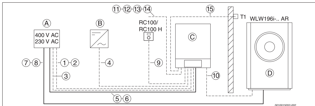
Bild 22 Kabelzugplan der elektrischen Leitungen bei Außenaufstellung (Prinzipdarstellung)
