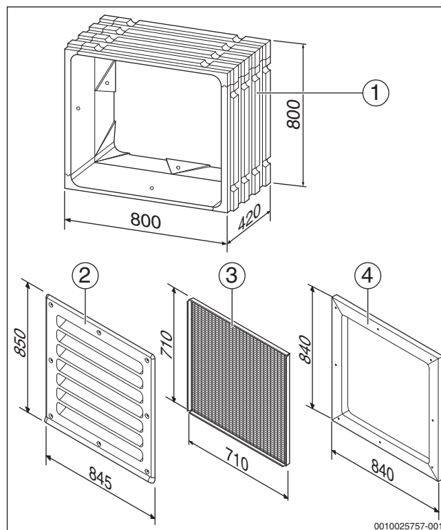
Bild 12 Wanddurchführung und Zubehör
