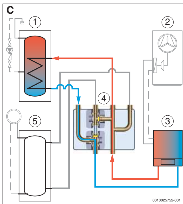
Bild 7 Betriebszustand C: Warmwasser-Kreis
