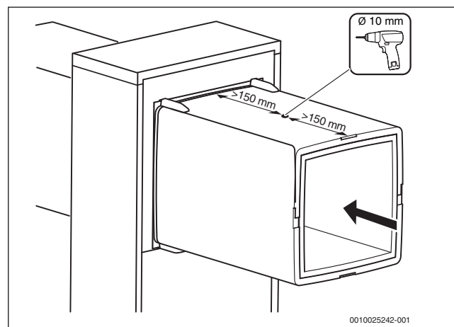
Bild 16 Montage des Referenzfühlers TL2 am Luftansaugkanal
