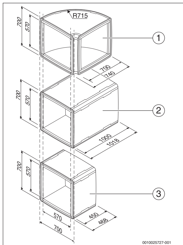
Bild 11 Beispiele für Luftkanäle Querschnitt 700 (alle Maße in mm)
