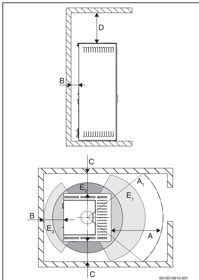
Bild 4 Mindestabstände
