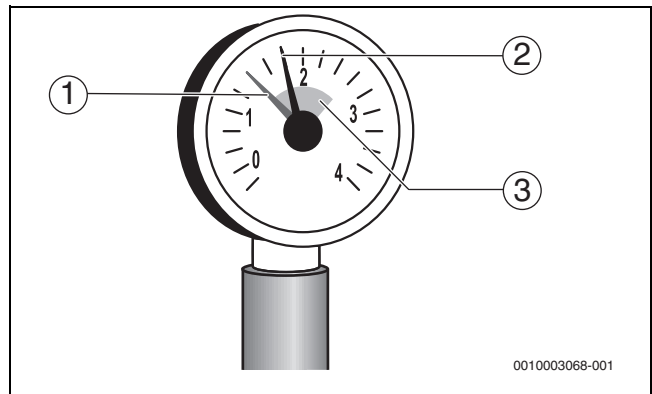
Bild 14 Manometer für geschlossene Anlagen
