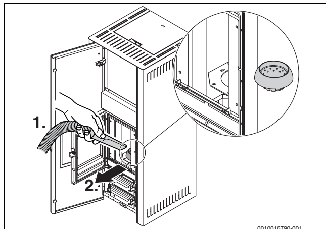
Bild 10 Asche entfernen
