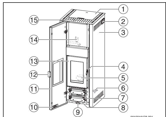
Bild 3 Produktübersicht
