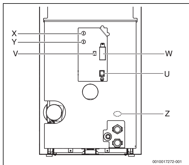
Bild 15 Anschlüsse Rückseite
