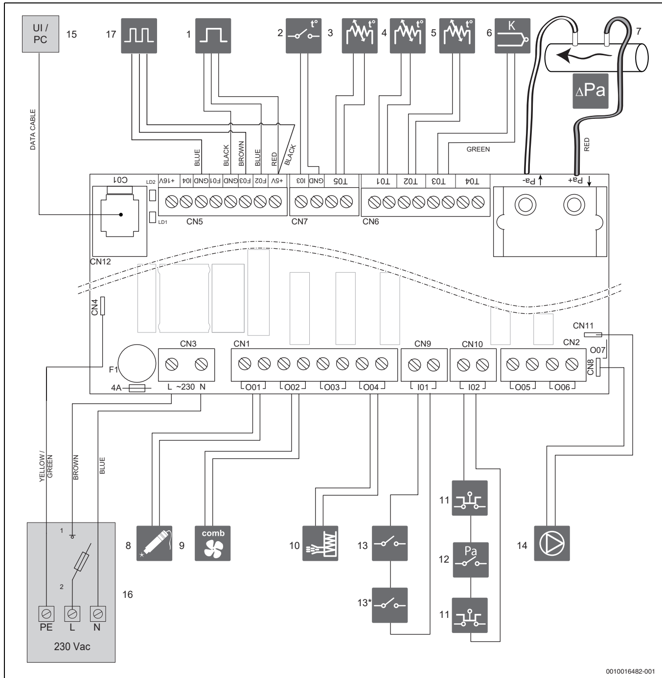
Bild 12 Anschlussplan
