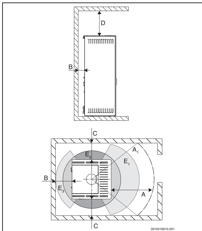
Bild 5 Mindestabstände
