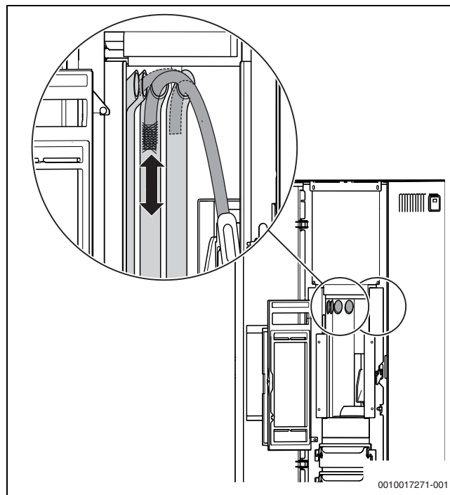
Bild 10 Rohre der Turbolatoren (2 x 4) mit der Bürste reinigen
