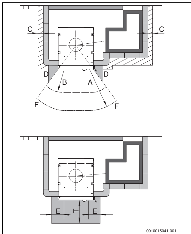
Bild 5 Äußere Mindestabstände
