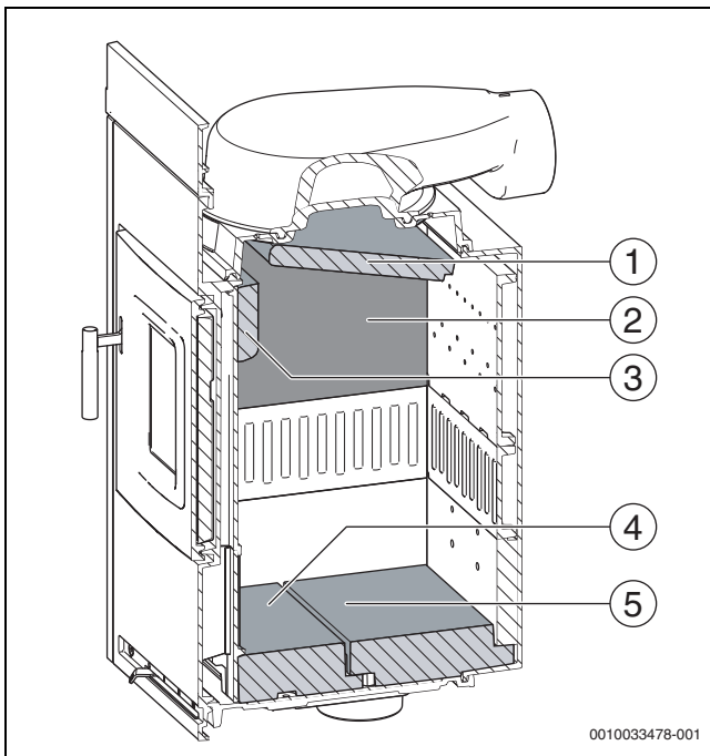
Bild 19 Seitlicher Schnitt
