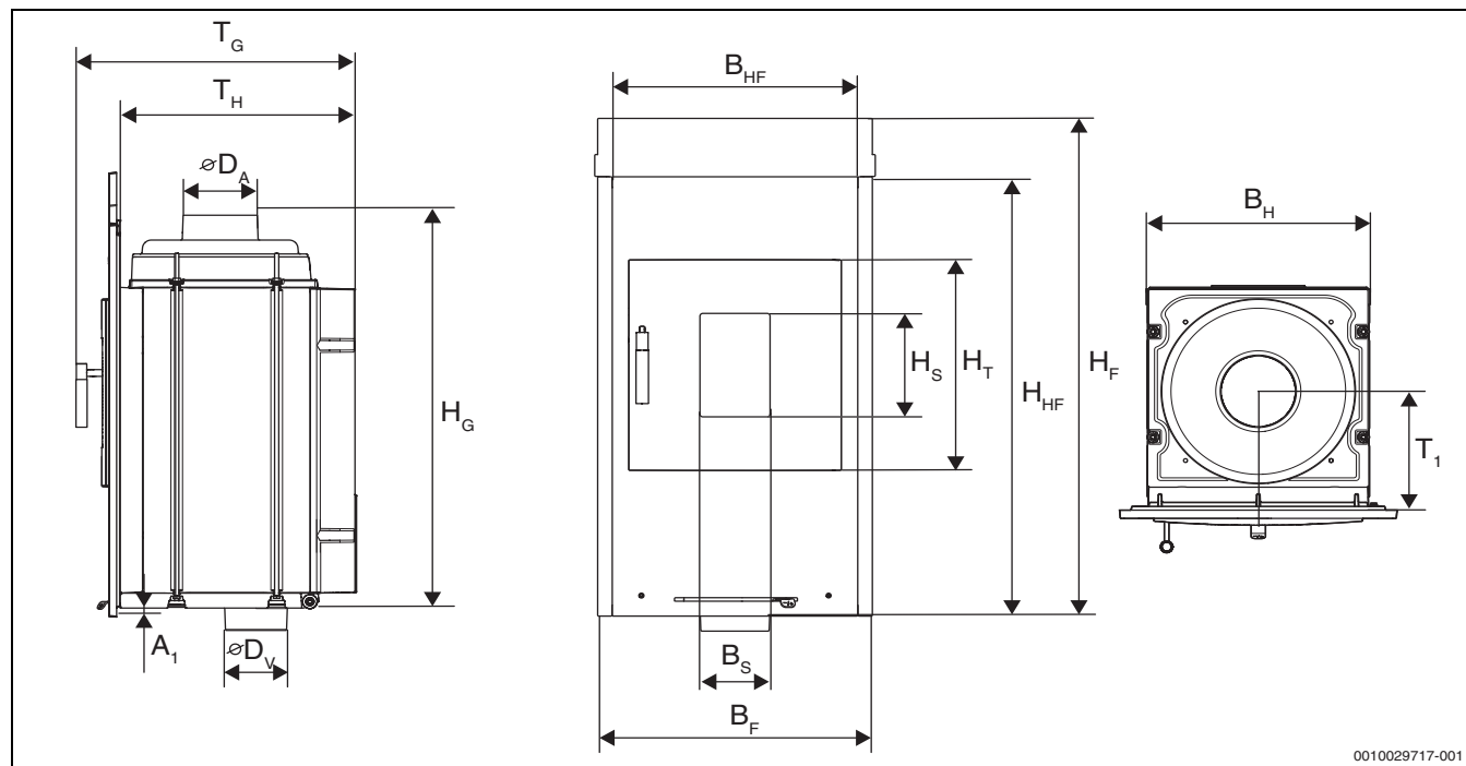
Bild 4 Abmessungen
