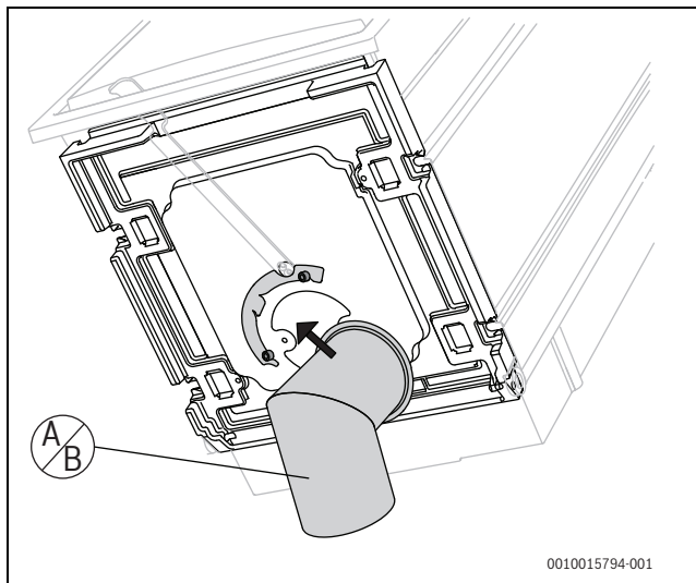
Bild 10 Verbrennungsluftstutzen installieren
