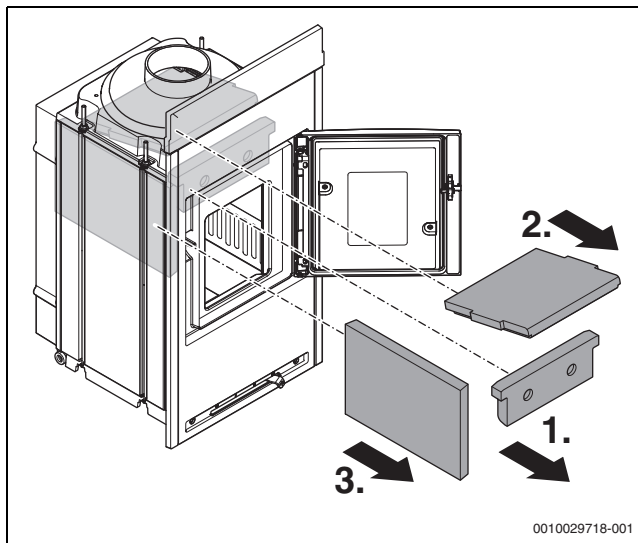
Bild 18 Feuerraumauskleidung ausbauen
