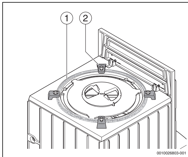
Bild 7 Kuppel montieren
