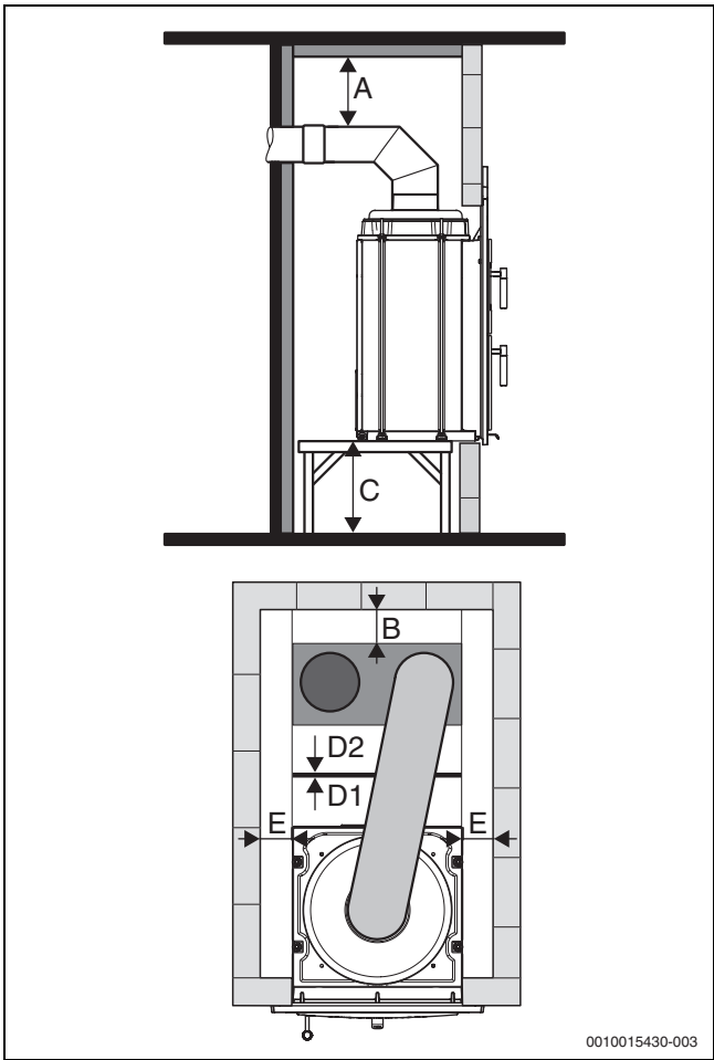
Bild 6 Heizkammer-Mindestabstände
