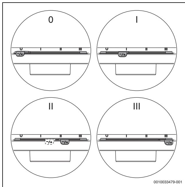
Bild 22 Verbrennungsluftschieber regulieren
