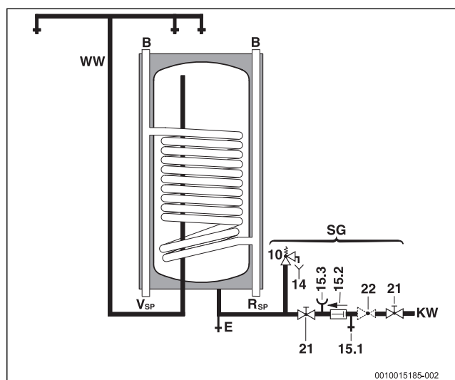
Afb. 6 Trinkwasserseitiges Anschluss-Schema, neben dem Heizgerät
