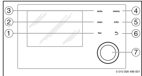
Bild 12 Bedienelemente
