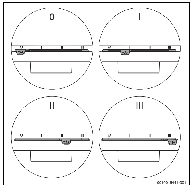
Bild 8 Verbrennungsluftschieber regulieren
