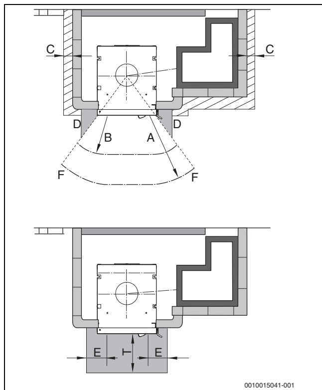
Bild 5 Äußere Mindestabstände
