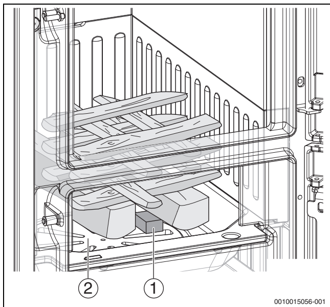
Bild 7 CO-armes Anheizen
