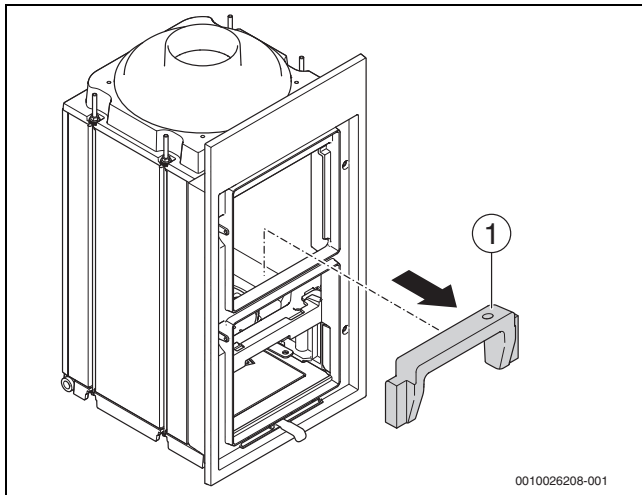
Bild 13 Frontstein (Hitzeschutzstein) ausbauen
