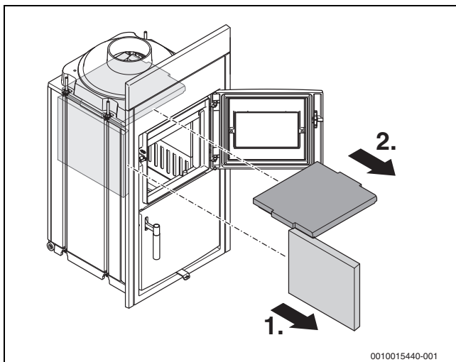
Bild 14 Feuerraumauskleidung ausbauen
