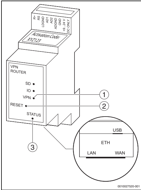
Bild 1 Geräteübersicht
