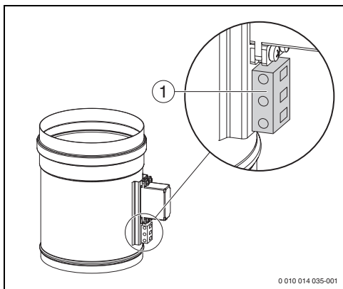
Bild 8 Drosselklappe
