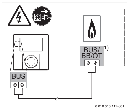
Bild 8 Anschluss der Bedieneinheit an einem Wärmerezeuger
