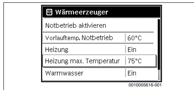
Bild 6 Maximale Vorlauftemperatur
