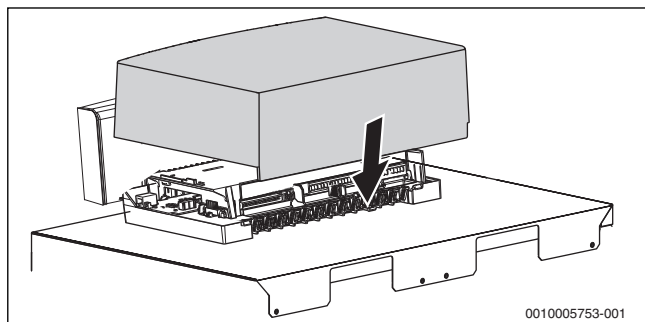
Bild 12 Abdeckhaube montieren
