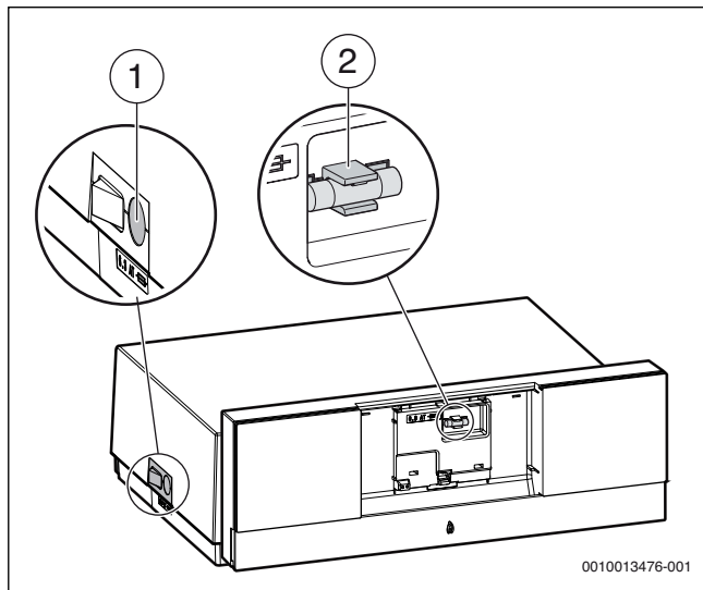
Bild 41 Sicherung ersetzen
