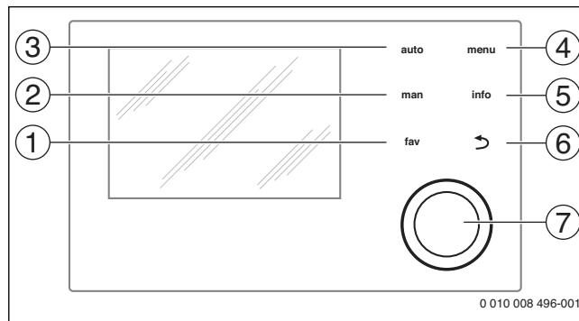
Bild 19 Bedienelemente
