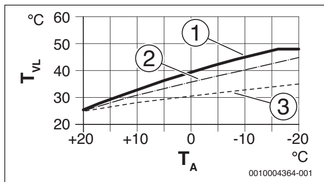
Bild 35 Einstellung der Heizkurve für Fußbodenheizung Steigung über Auslegungstemperatur T_{AL} und minimale Außentemperatur T_{A,min}
