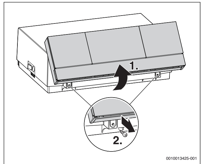
Bild 3 Schrauben entfernen
