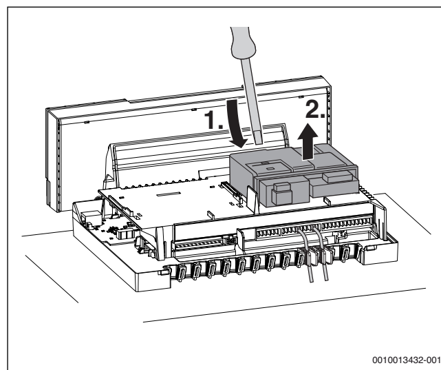
Bild 16 Funktionsmodul entnehmen
