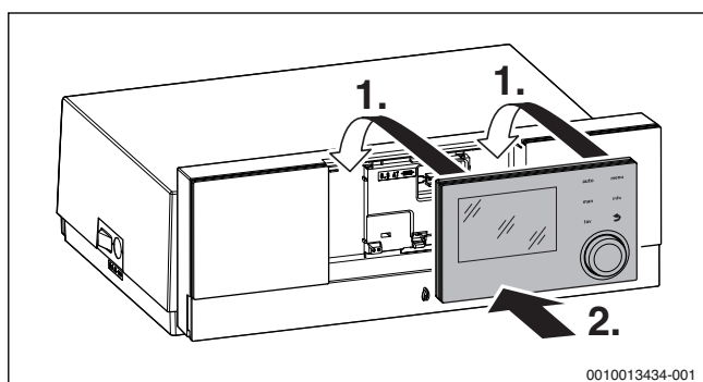
Bild 14 Bedieneinheit einhängen
