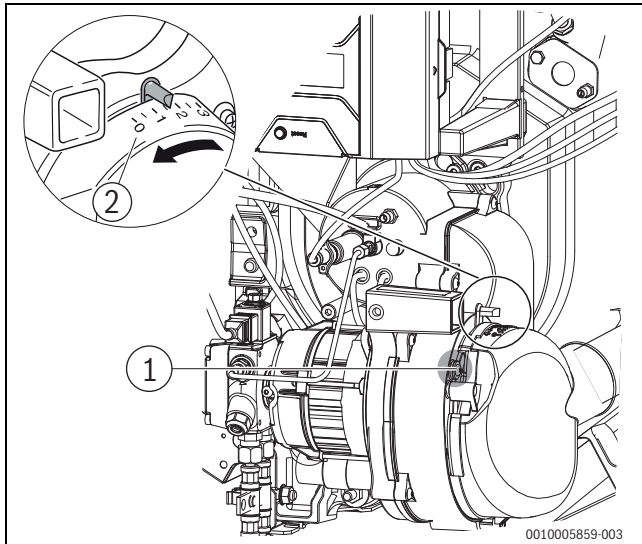
Bild 28 Ansaugluftführung einstellen
