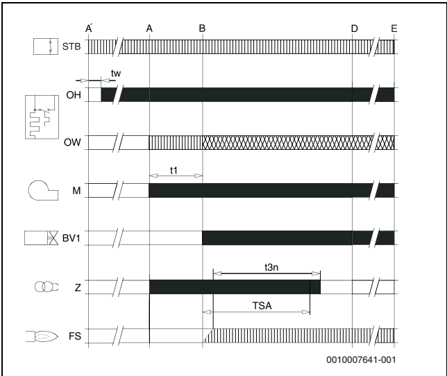
Bild 10 Programmablauf Feuerungsautomat
