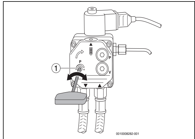
Bild 26 Druck einstellen – Ölpumpe Danfoss
