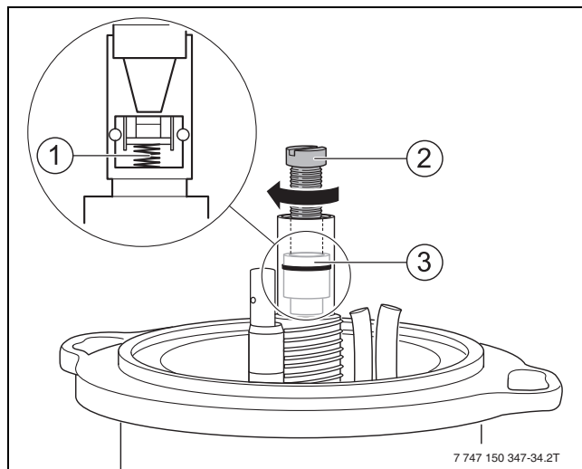
Bild 41 Abschlussventil austauschen
