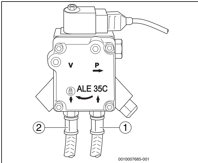
Bild 20 Ölpumpe – Suntec
