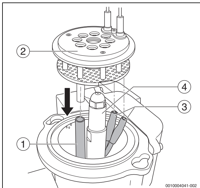
Bild 40 Mischsystem montieren
