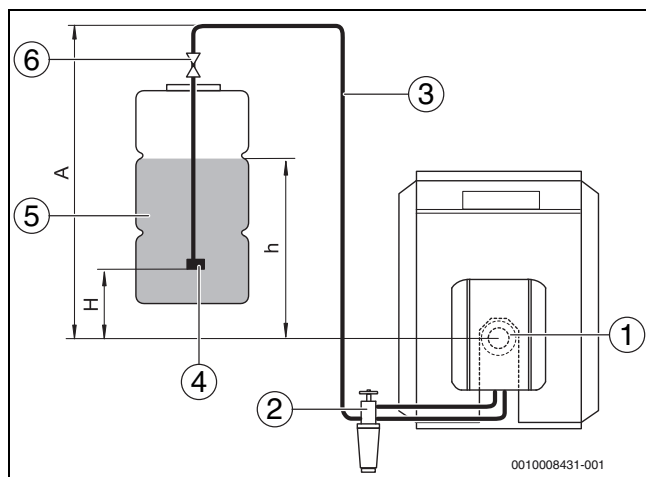
Bild 16 Öltank oberhalb der Pumpe
