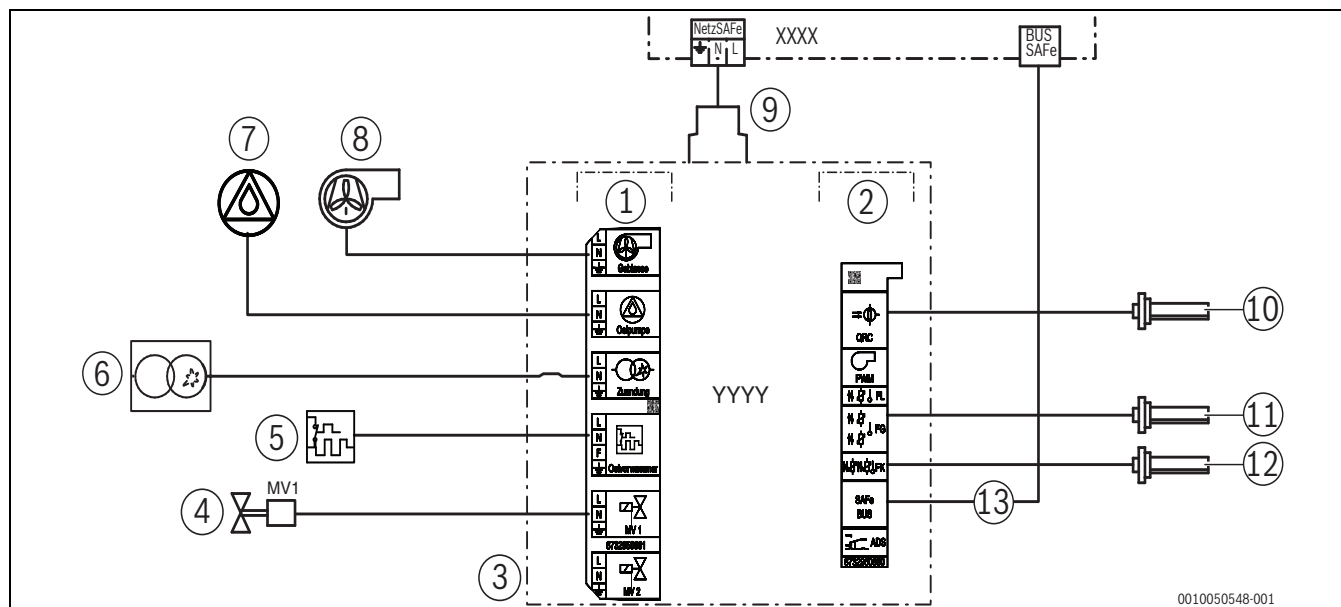
Bild 13 Anschlussplan digitaler Feuerungsautomat SAFe100
