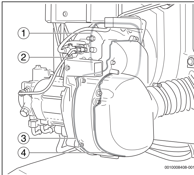
Bild 48 Zusätzliche Abdichtung
