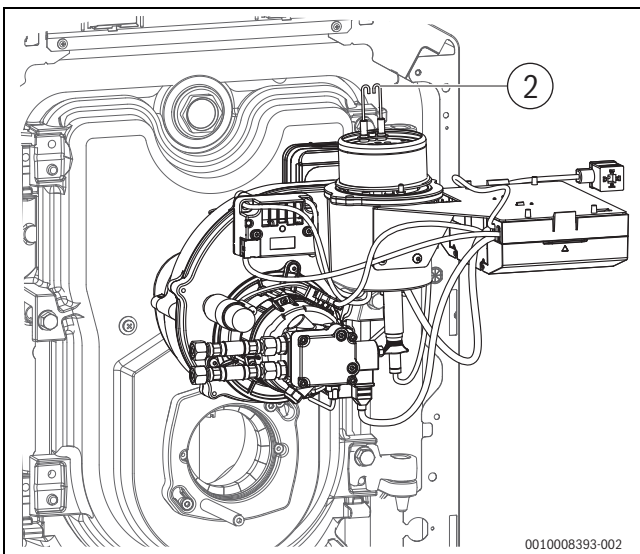
Bild 37 Brenner in Serviceposition aufstecken
