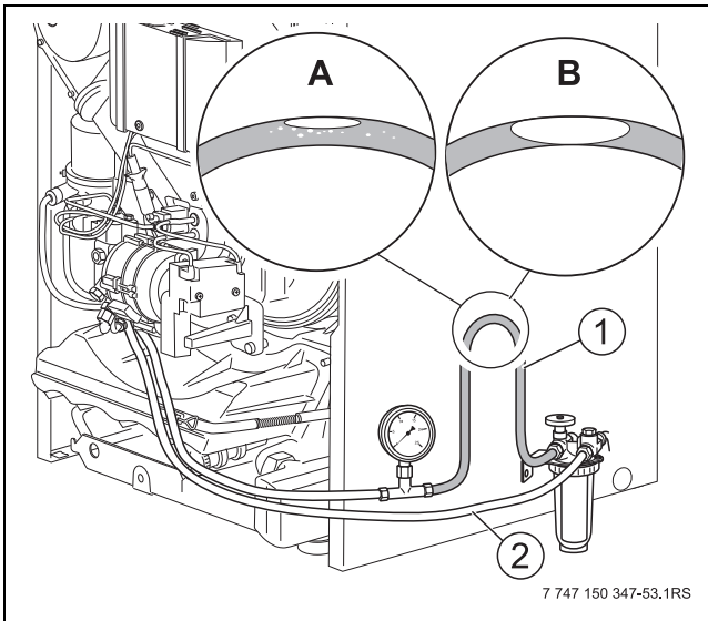
Bild 18 Transparenten Schlauch hochbinden
