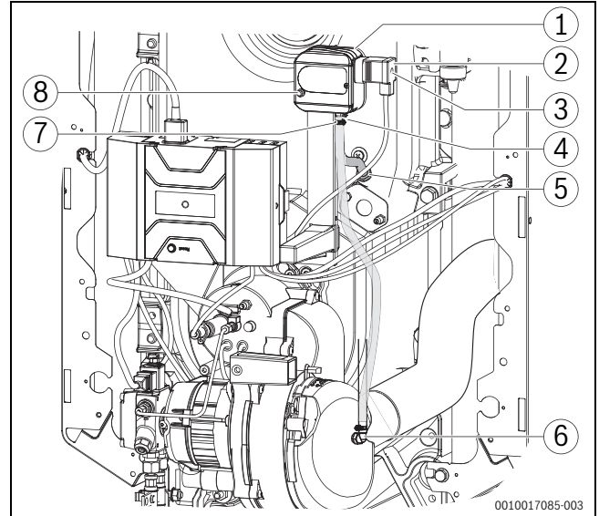
Bild 35 Brenner mit Druckwächter
