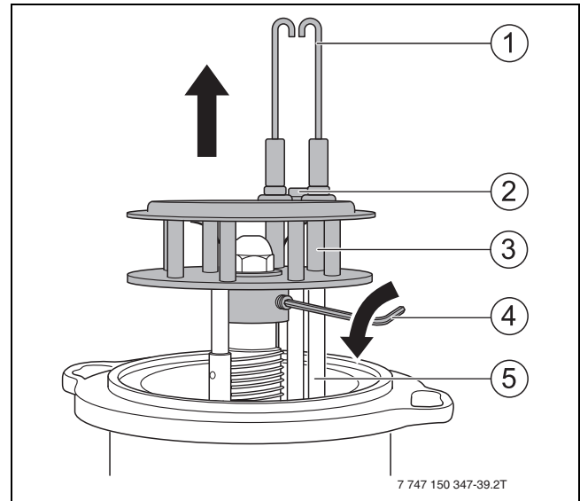
Bild 38 Mischsystem ausbauen
