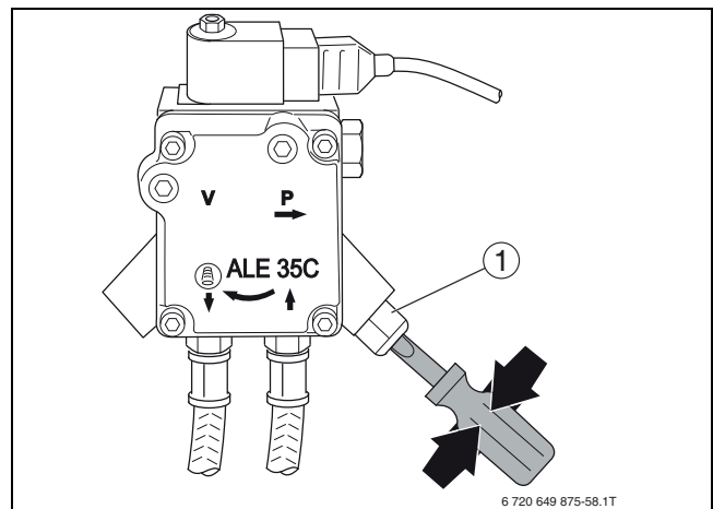
Bild 27 Druck einstellen – Ölpumpe Suntec
