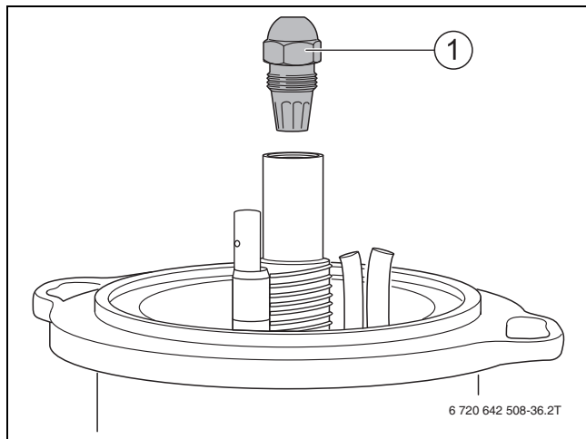
Bild 39 Düse abschrauben
