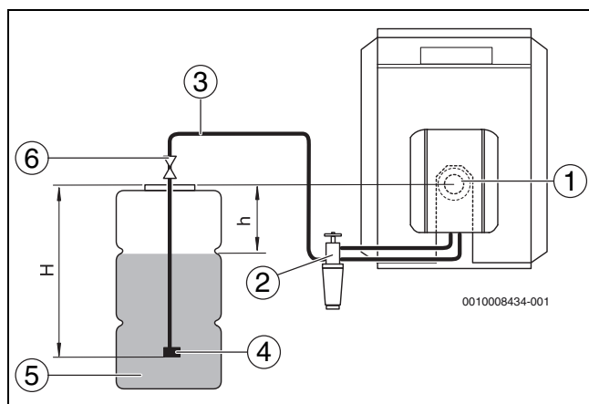
Bild 17 Öltank unterhalb der Pumpe
