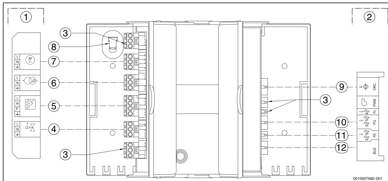
Bild 12 Anschlussplan digitaler Feuerungsautomat SAFe30
