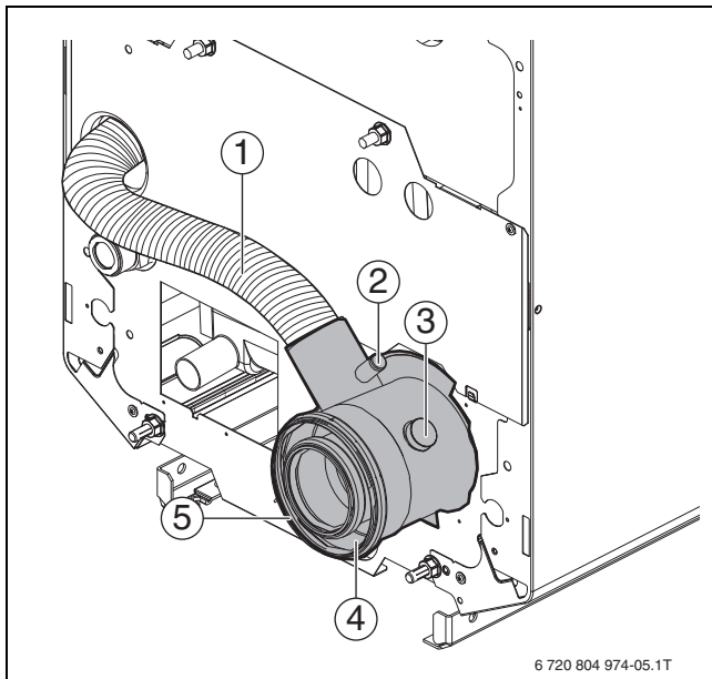
Bild 15 Luft-Abgas-Anschlussstutzen montieren
