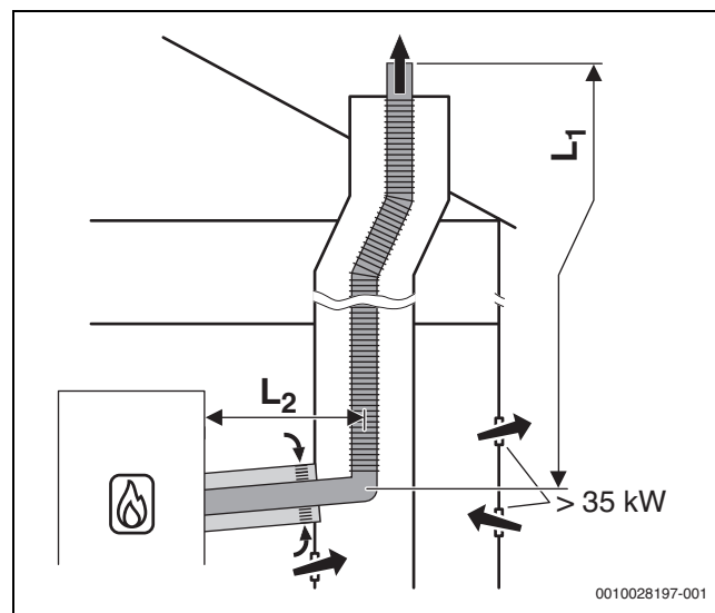
Bild 19 Flexible Abgasführung im Schacht nach B 33 mit raumluftabhängiger Luftzufuhr über die konzentrische Luft-Abgas-Führung im Aufstellraum
