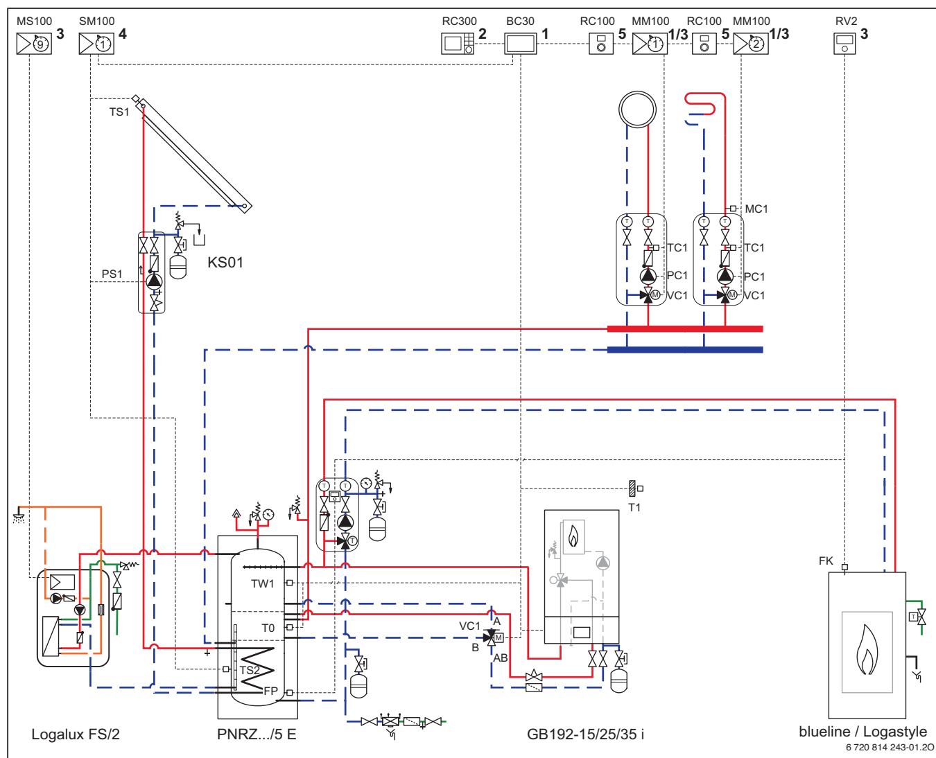
Bild 104 Anlagenschema mit Regelung (unverbindliche Prinzipdarstellung)
