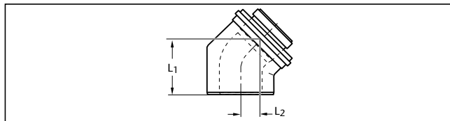
Bild 206 Konzentrischer Bogen Ø 110/160 (Maße → Tabelle 99)
