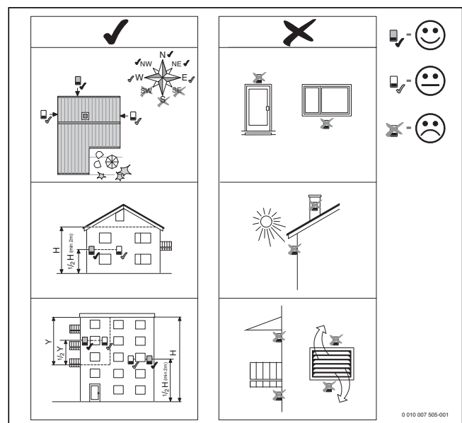
Bild 40 Anordnung des Außentemperaturfühlers (Maße in m)
