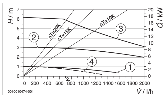
Bild 87 Leistungsfelder der Pumpen
