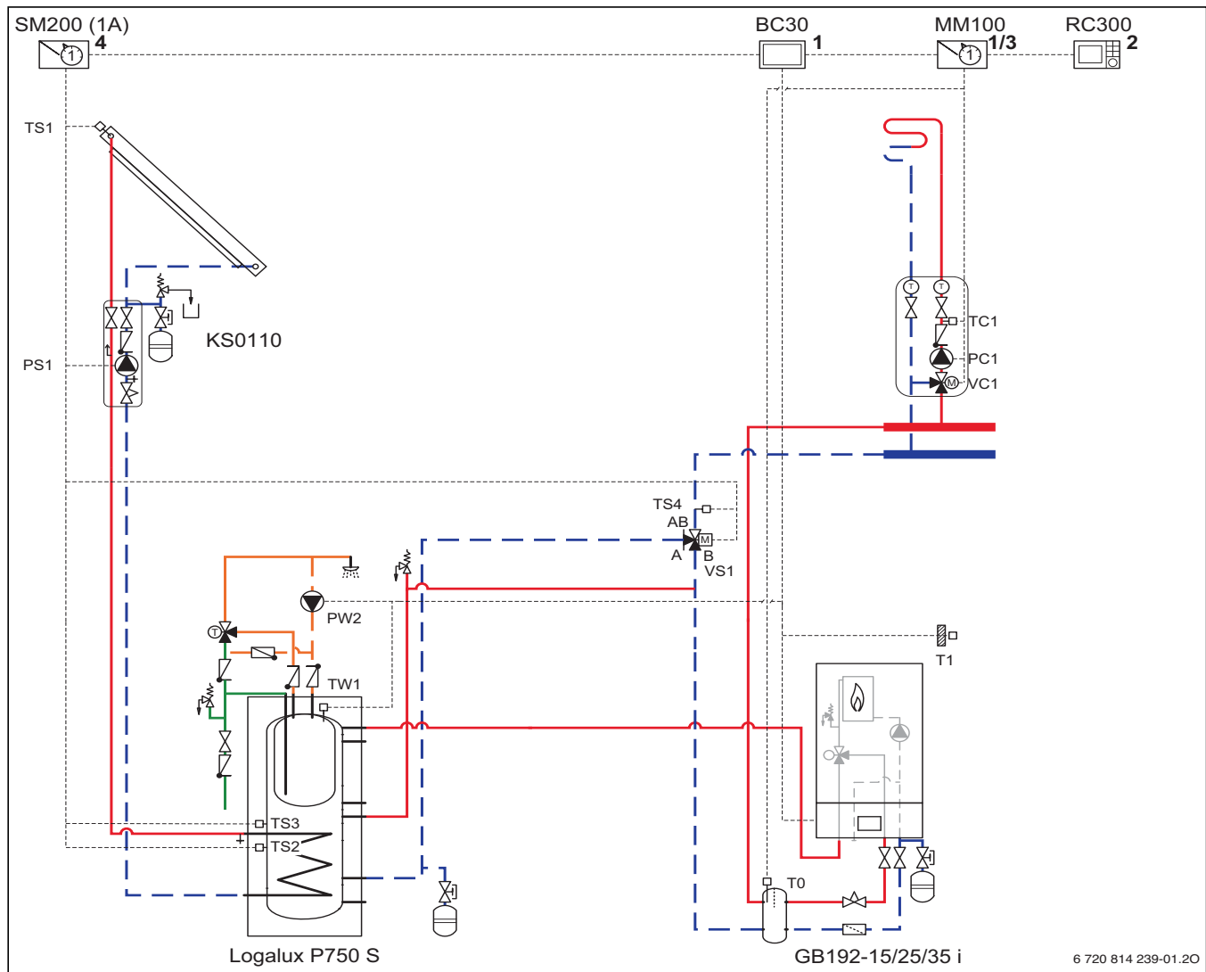
Bild 98 Anlagenschema mit Regelung (unverbindliche Prinzipdarstellung)
