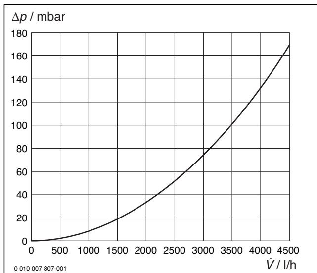
Bild 86 Druckverlust-Diagramm gemischter Heizkreis (HK2)
