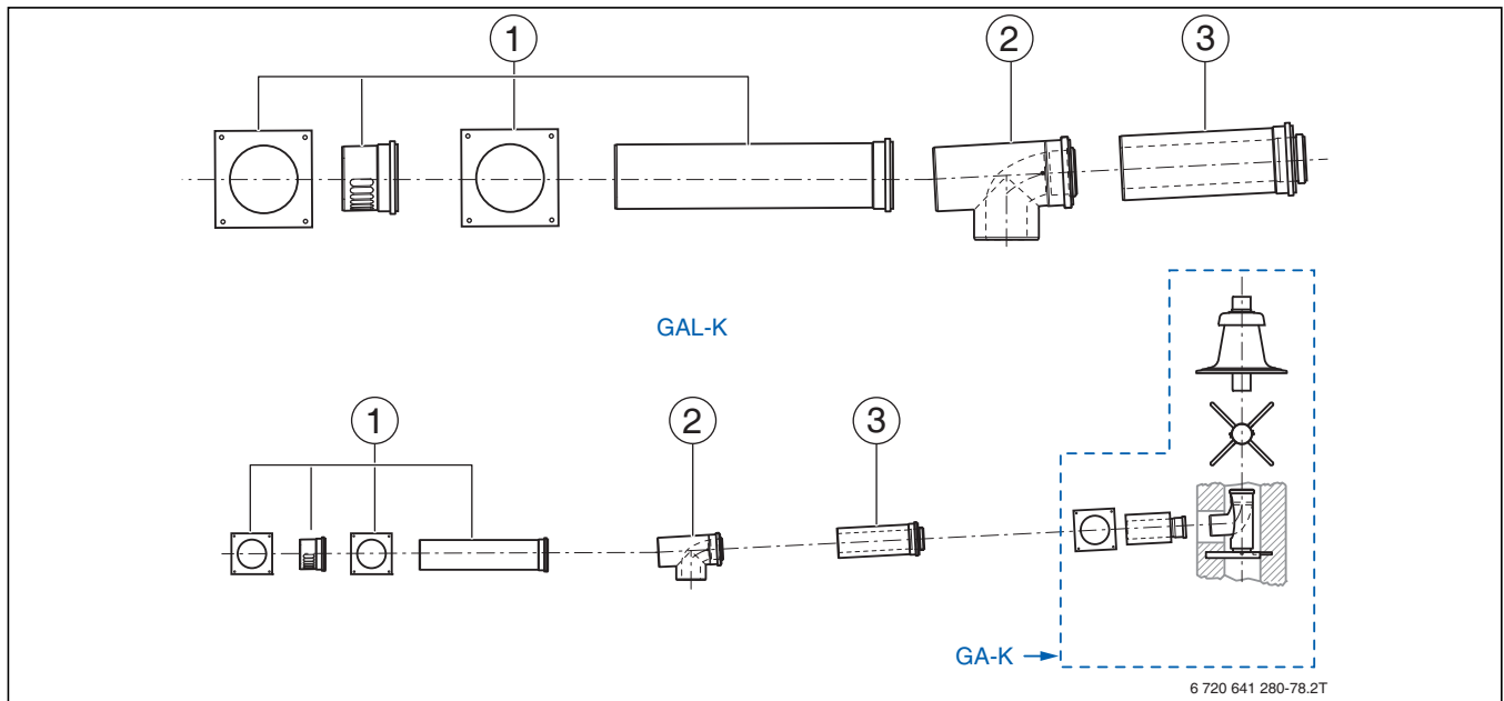
Bild 171 Bauteile des Grundbausatzes GAL-K aus Kunststoff
