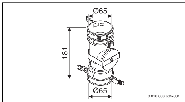
Bild 185 Verbindungsstück Flex mit Prüföffnung Ø 60 mm (Maße in mm)
