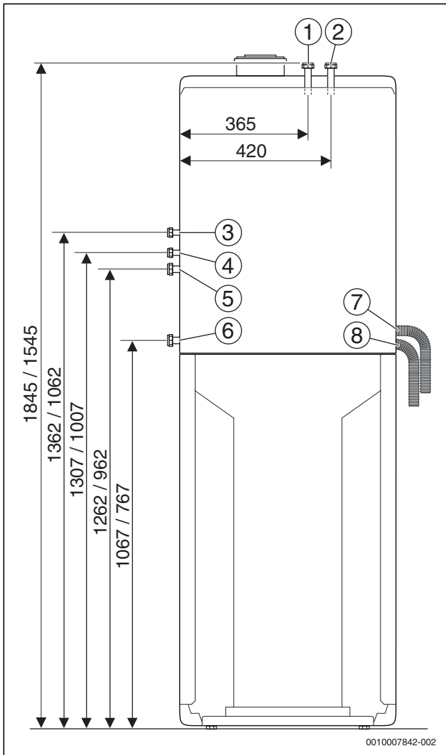
Bild 23 Anschlussmaße des Zubehörs Heizkreiserweiterung 1 (Maße in mm)
