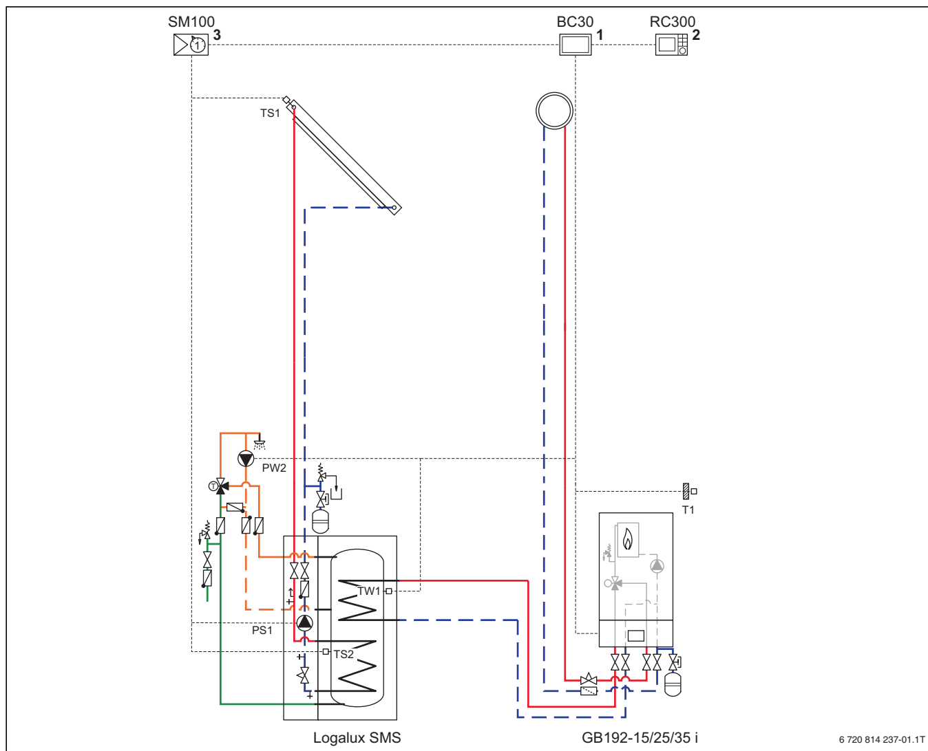
Bild 97 Anlagenschema mit Regelung (unverbindliche Prinzipdarstellung)
