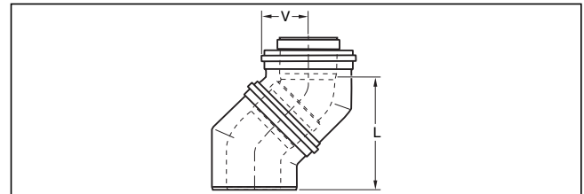
Bild 209 Versatzmaße konzentrischer Bogen Ø 110/160 (Maße → Tabelle 100)
