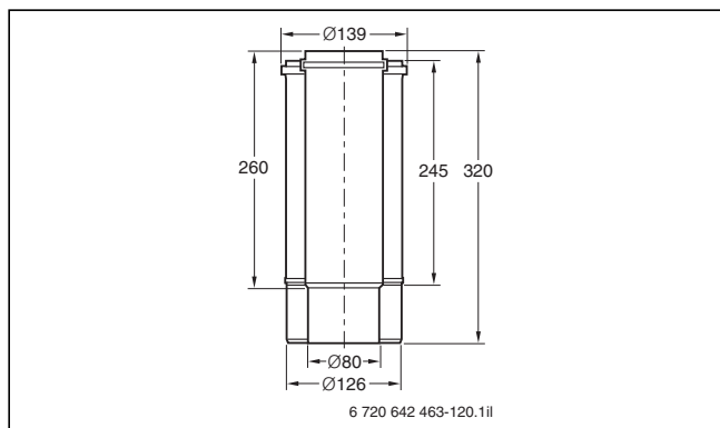
Bild 198 Konzentrisches Schiebestück (Maße in mm)
