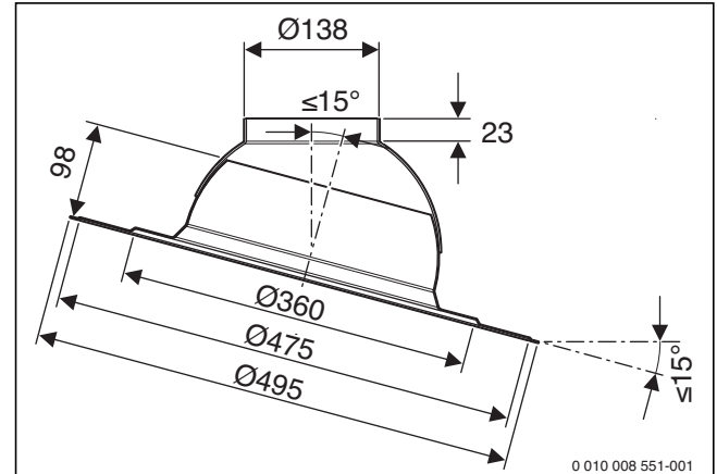
Bild 194 Flachdach-Klebeflansch für DN 80/125 (Maße in mm)
