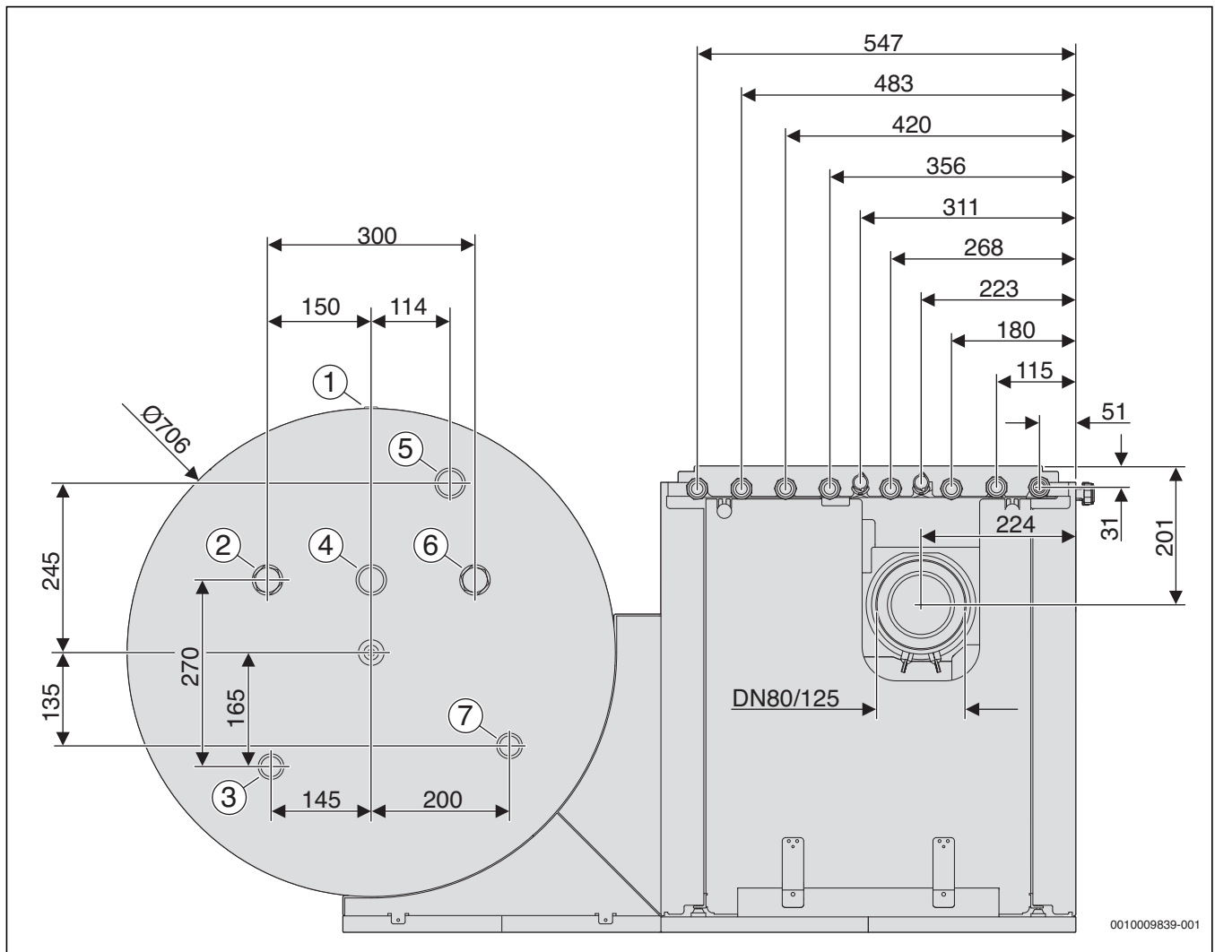
Bild 36 Aufsicht GBH192-... iT...
