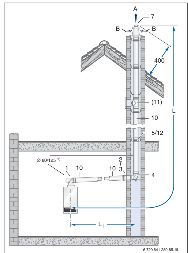
Bild 156 Montagevariante (Maße in mm)
