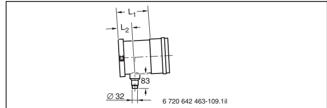
Bild 222 Endstück mit Kondensatablauf (Maße in mm)
