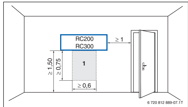
Bild 39 Position der Bedieneinheit RC200 oder RC300 im Referenzraum (Maße in m)
