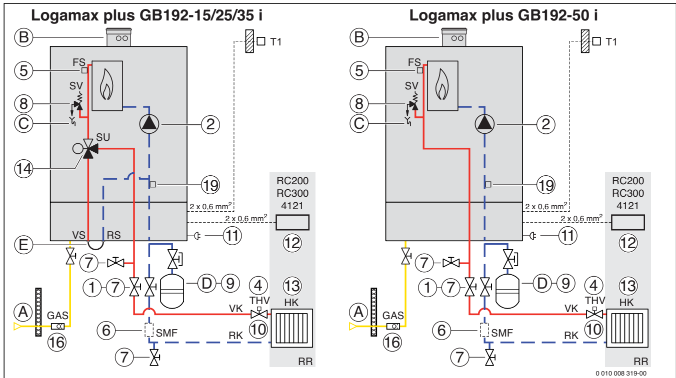
Bild 72 Hydraulik Logamax plus GB192i (Planungshinweise → Tabelle 29, Seite 76)
