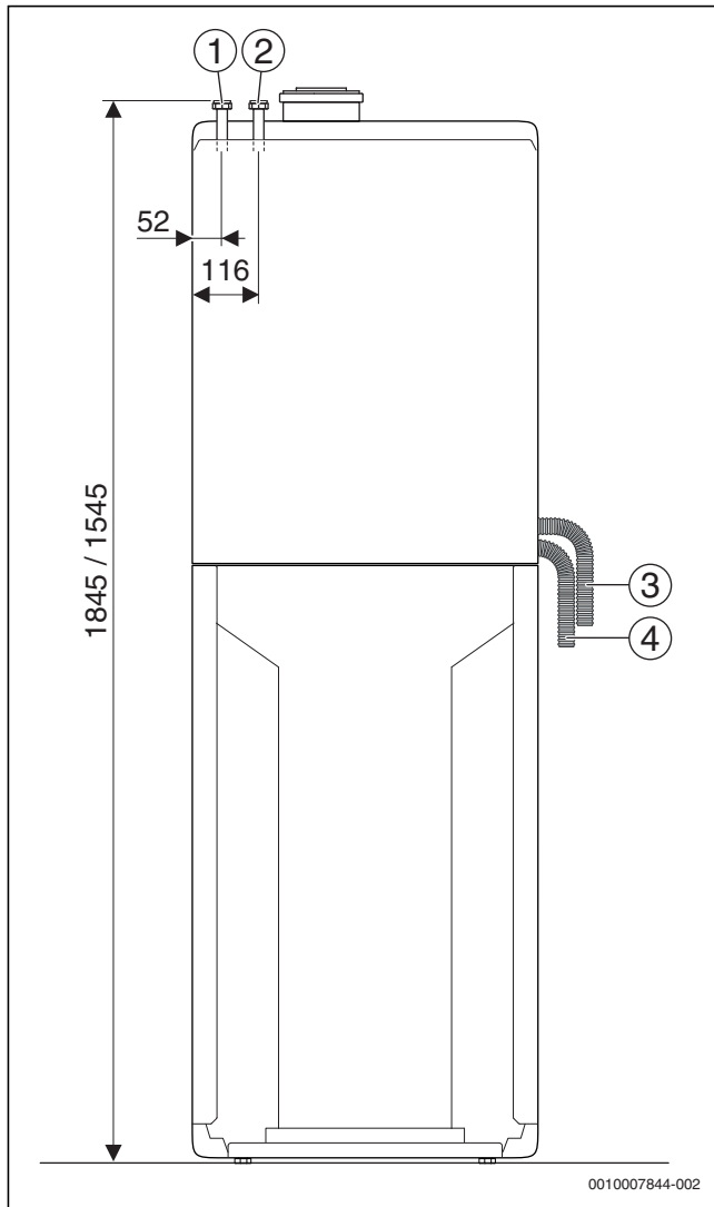
Bild 27 Anschlussmaße des Zubehörs Anschluss-Set Heizungsunterstützung HU (Maße in mm)
