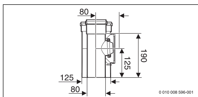
Bild 201 Konzentrisches Rohr mit Prüföffnung \varnothing 80/125 (Maße in mm)
