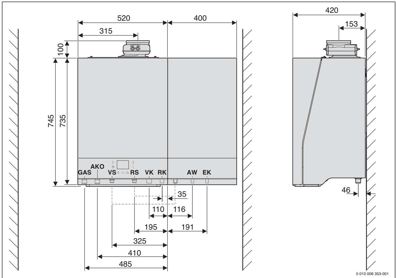
Bild 13 Abmessungen und Anschlüsse Logamax plus GB192-30 iT40S (Maße in mm)
