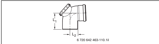
Bild 215 Bogen mit Prüföffnung
