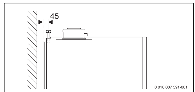
Bild 30 Anschlussmaße des Zubehörs Anschluss-Set solare Heizungsunterstützung SHU (Maße in mm)
