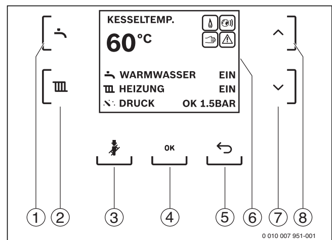
Bild 41 Anzeigen und Bedienelemente des Basiscontrollers Logamatic BC30
