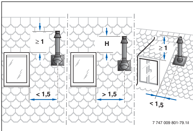
Bild 152 Mindestabstände zu Fenstern beim Bausatz DO; (Maße in m) (Beispiele nach der Muster-Feuerungsverordnung; Vorschriften → Seite 185)
