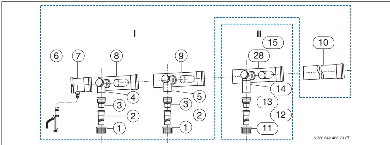
Bild 144 Anschlussstück und Bauteile des Grundbausatzes Abgaskaskade sowie des Erweiterungsbausatzes Abgaskaskade aus Kunststoff
