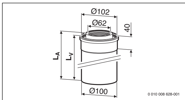
Bild 199 Konzentrisches Rohr \varnothing 60/100 (Maße in mm)
