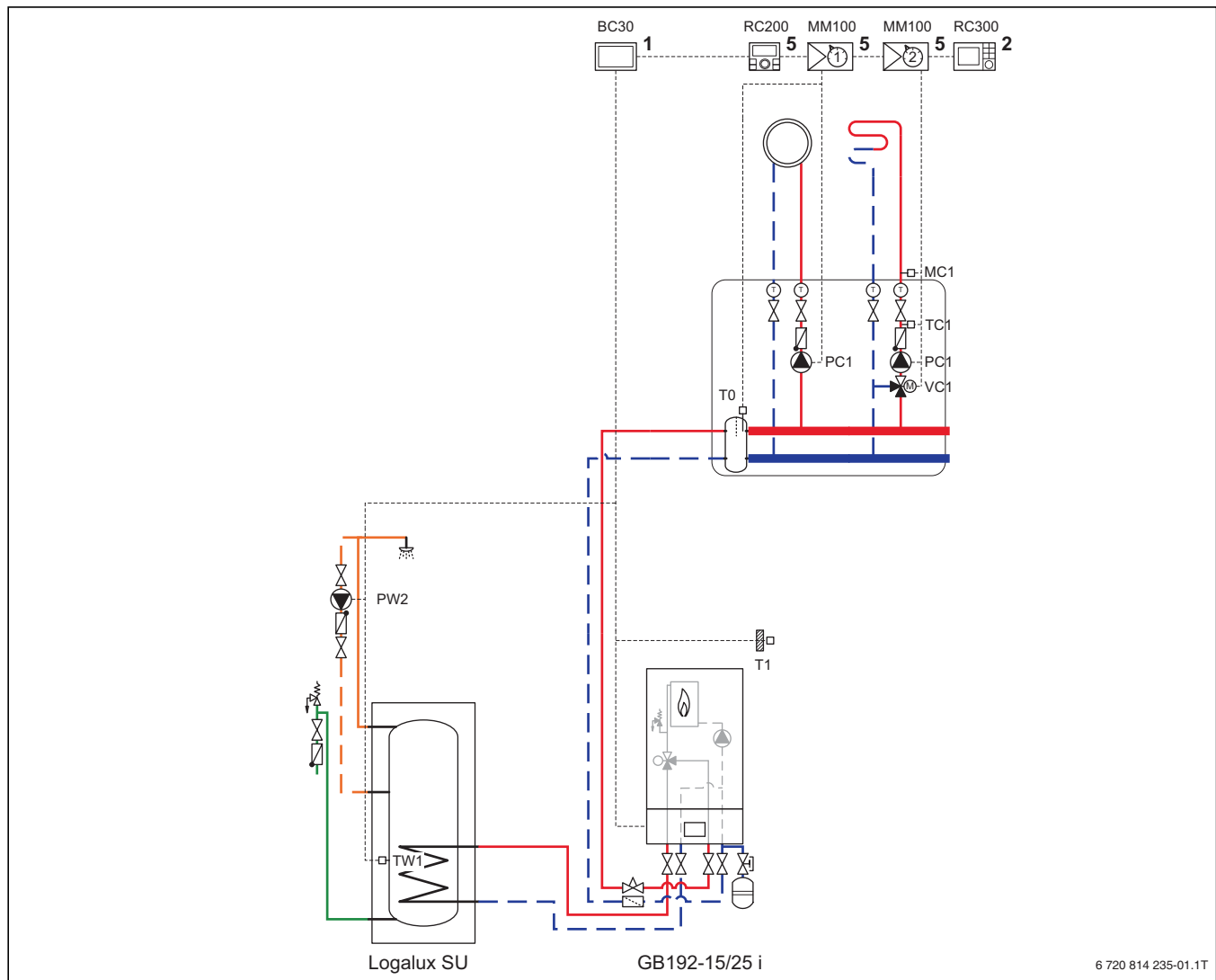
Bild 94 Anlagenschema mit Regelung (unverbindliche Prinzipdarstellung)
