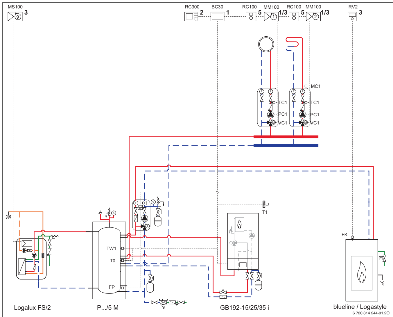
Bild 105 Anlagenschema mit Regelung (unverbindliche Prinzipdarstellung)
