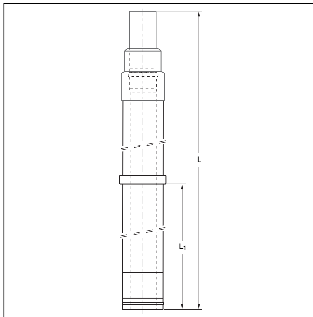
Bild 213 Dachdurchführung mit Mündungsabschluss
