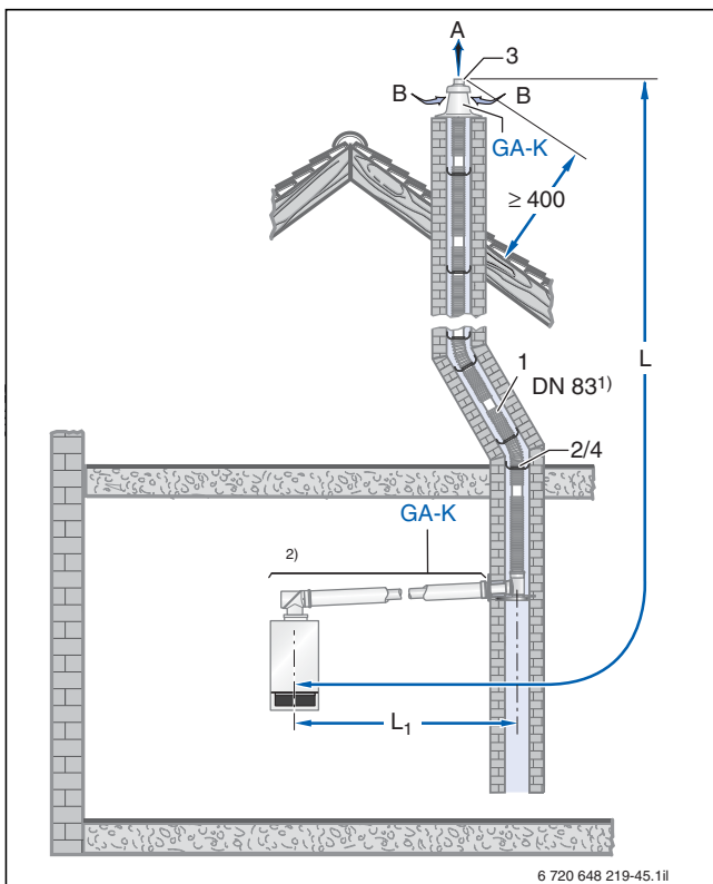
Bild 163 Montagevariante (Maße in mm)
