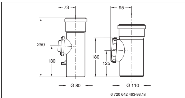
Bild 179 Rohr mit Prüföffnung (Maße in mm)
