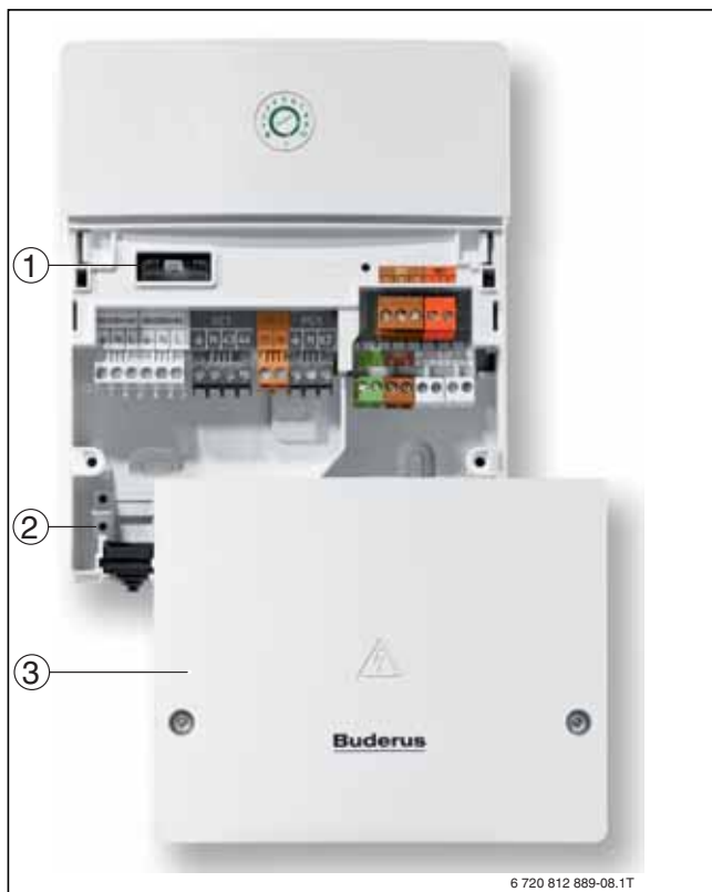
Bild 48 Funktionsmodul als Wandinstallation
