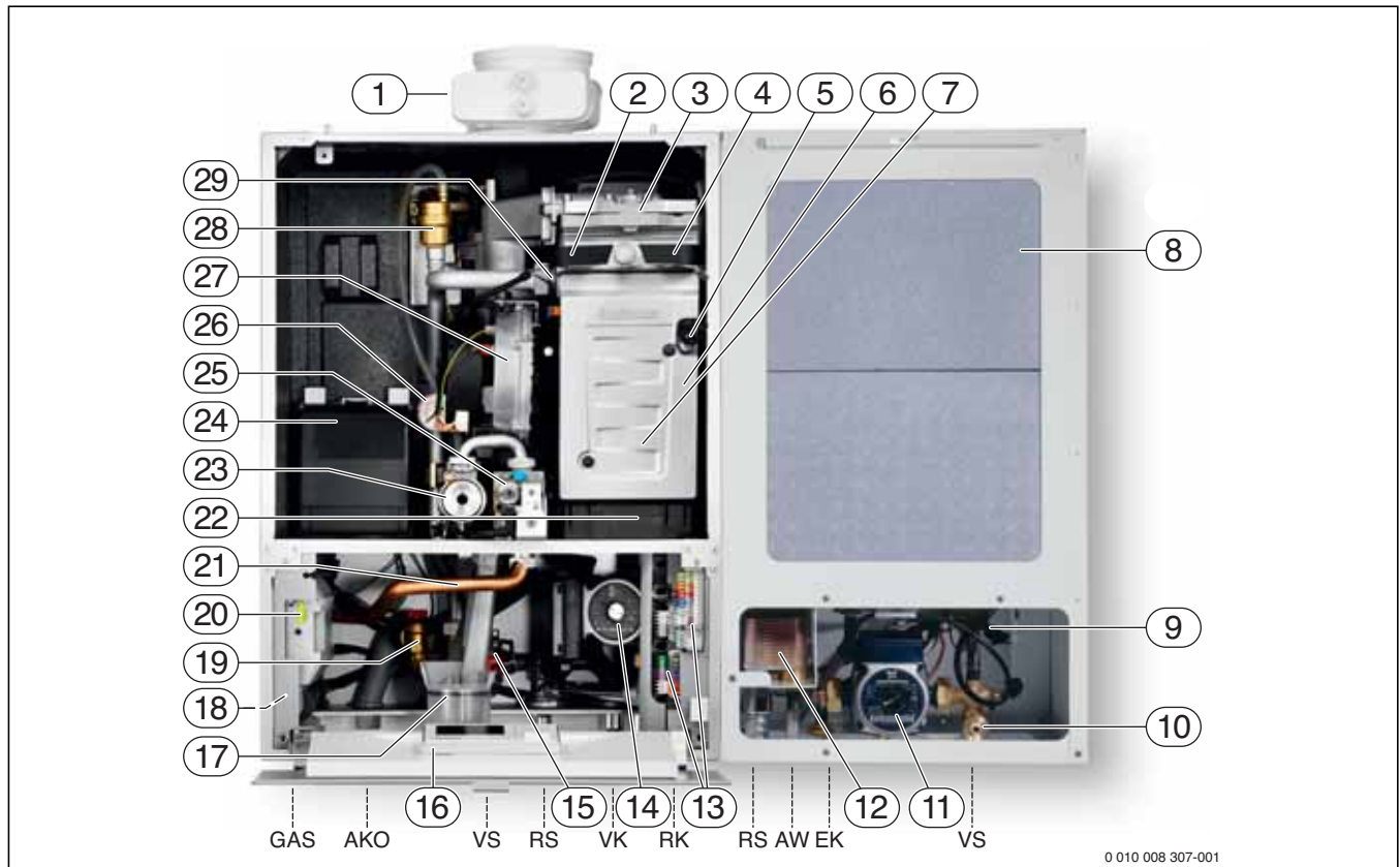
Bild 4 Ausgewählte Bauteile und Baugruppen Logamax plus GB192-30 iT40S (verdeckte Anschlüsse → Bild 8, Seite 15)
