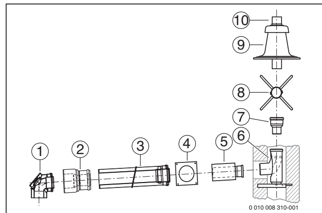
Bild 161 Bauteile des Grundbausatzes GA-K aus Kunststoff
