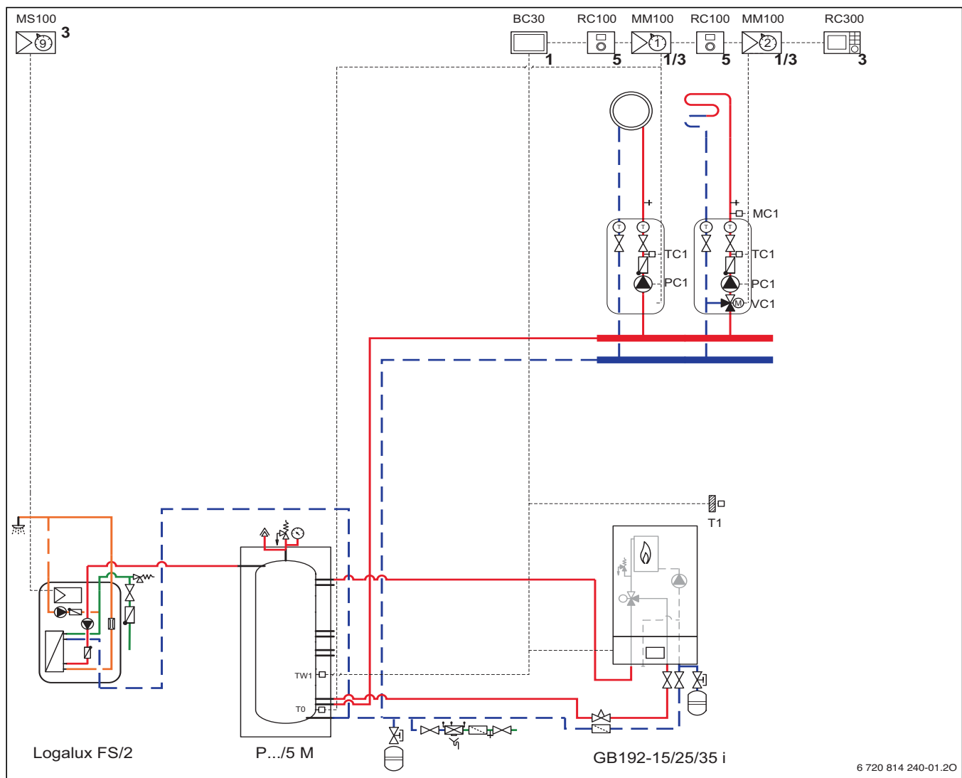
Bild 102 Anlagenschema mit Regelung (unverbindliche Prinzipdarstellung)
