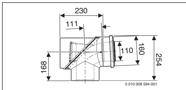
Bild 197 Konzentrisches T-Stück mit Prüföffnung \varnothing 110/160 (Maße in mm)
