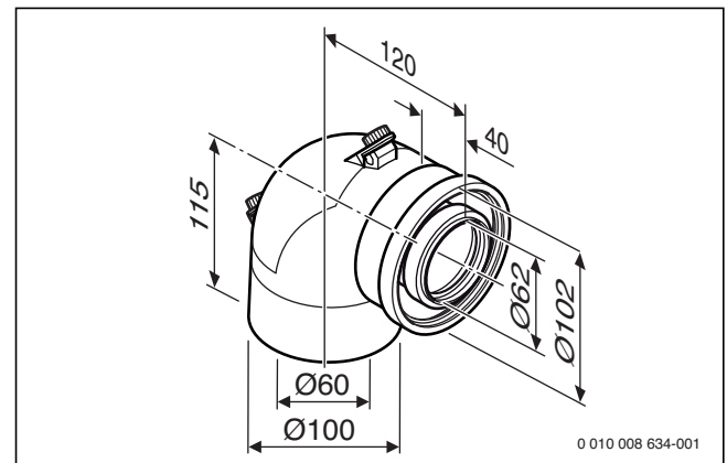
Bild 195 Konzentrischer Bogen mit Prüföffnung Ø 60/100 (Maße in mm)
