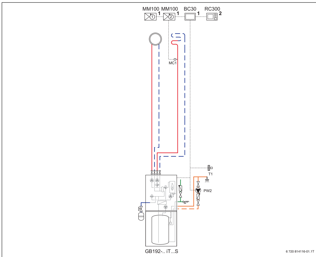
Bild 109 Anlagenschema mit Regelung (unverbindliche Prinzipdarstellung)
