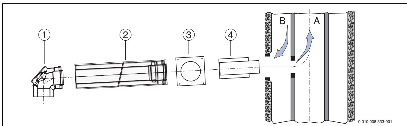
Bild 177 Bauteile des Grundbausatzes LAS-K aus Kunststoff DN 80/125
