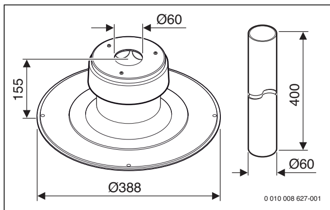
Bild 186 Schachtabdeckung für 60 mm, Aluminium (Maße in mm)
