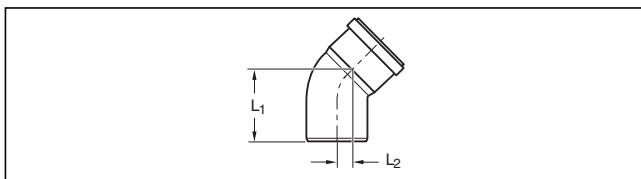
Bild 180 Bogen
