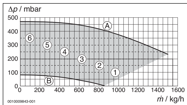
Bild 82 Pumpenkennfelder und Pumpenkennlinien
