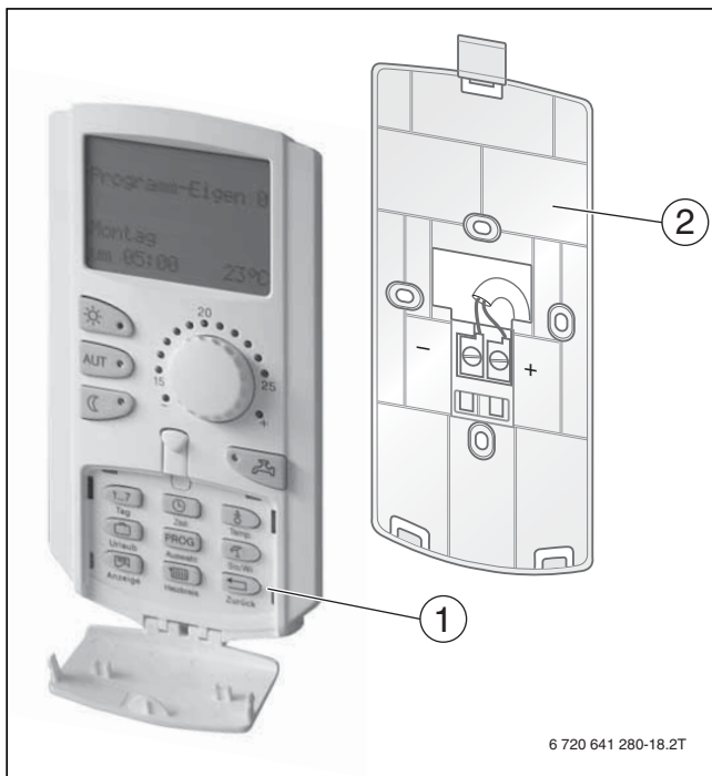
Bild 65 Bedieneinheit MEC2 mit integriertem Raumtemperaturfühler und Wandhalter
