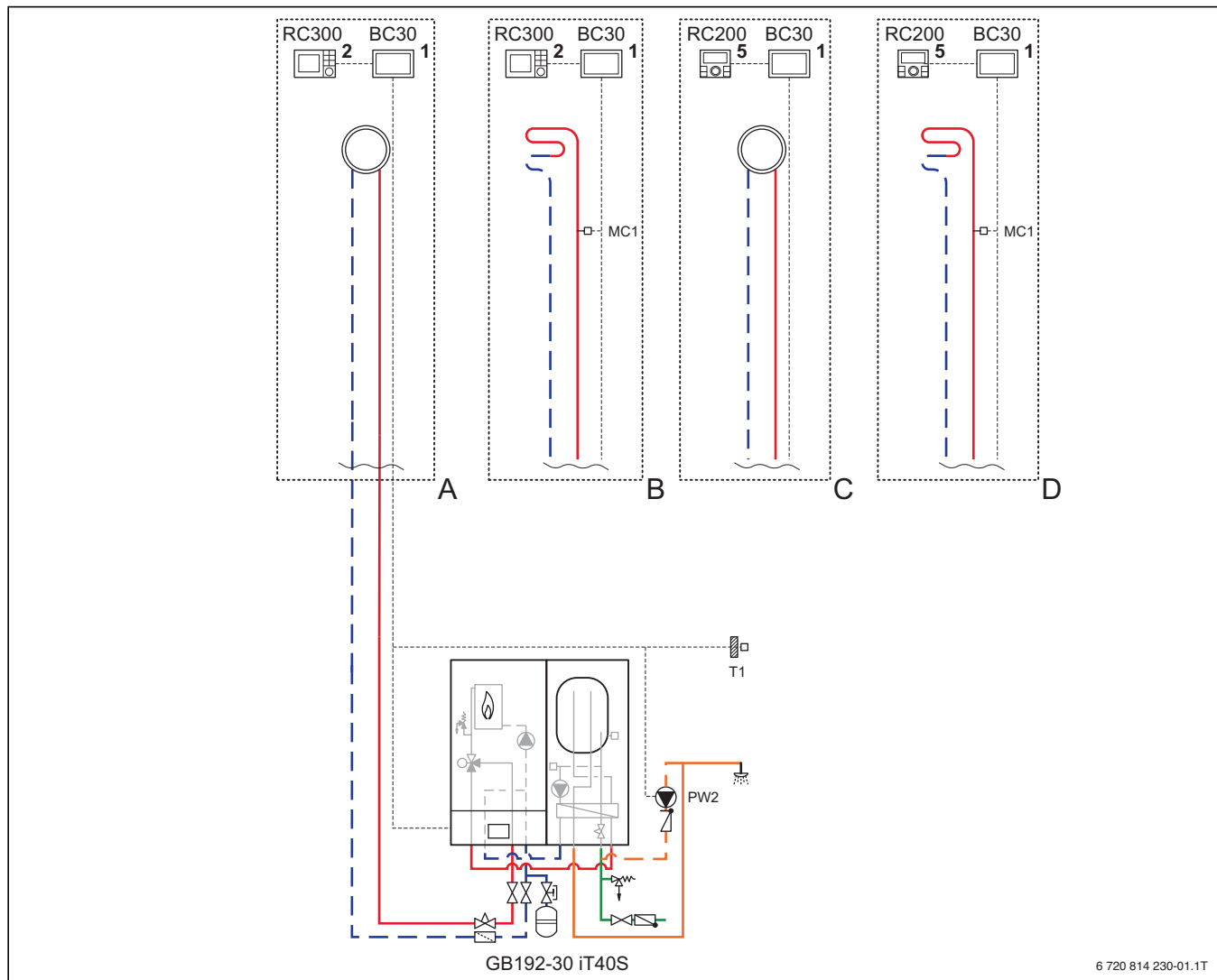
Bild 89 Anlagenschema mit Regelung (unverbindliche Prinzipdarstellung)
