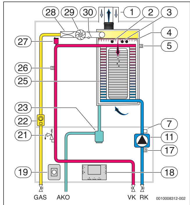
Bild 7 Funktionsschema Logamax plus GB192-50 i (Legende → Seite 15)
