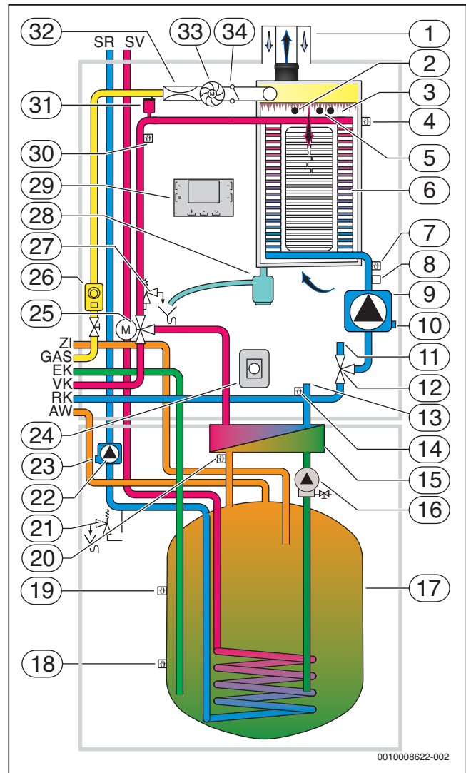
Bild 10 Funktionsschema Logamax plus GB192... iT210SR (Legende → Seite 15)
