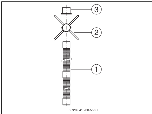
Bild 140 Bauteile des Grundbausatzes ÜB-Flex aus Kunststoff, DN 83
