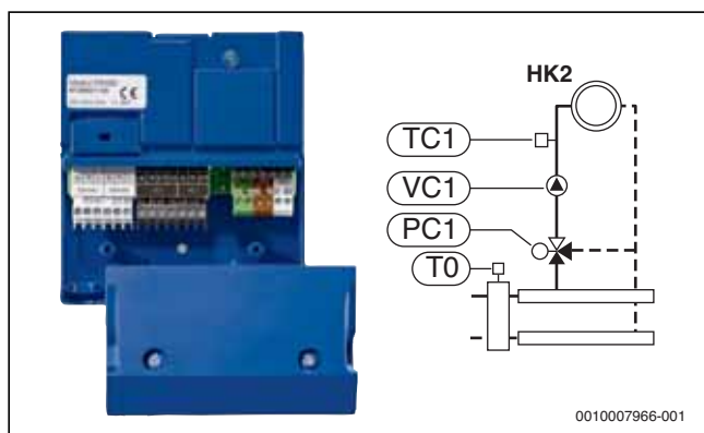
Bild 52 Heizkreismodul MM50
