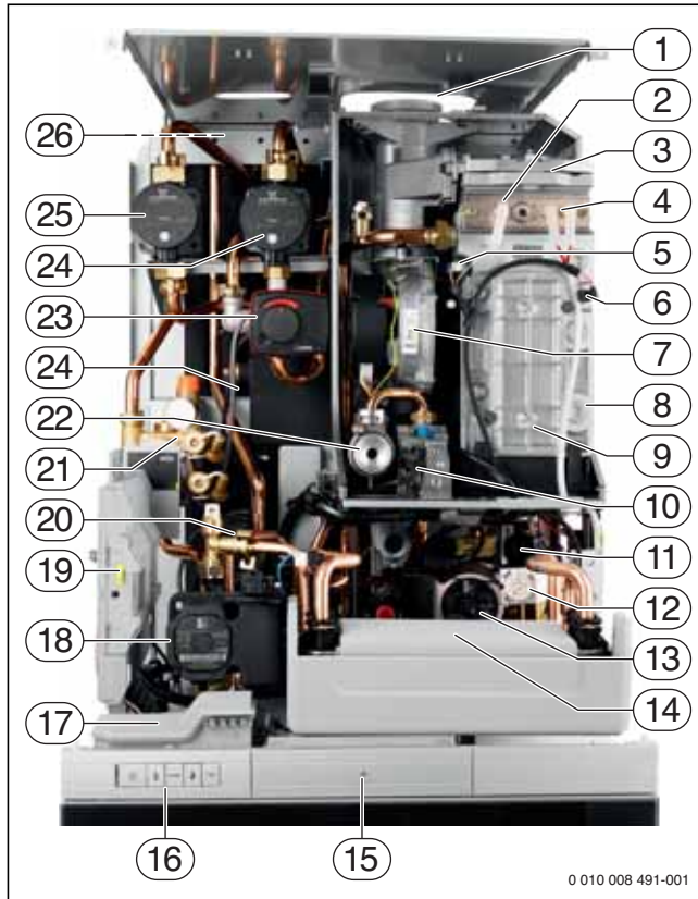
Bild 5 Ausgewählte Bauteile und Baugruppen Logamax plus GB192iT
