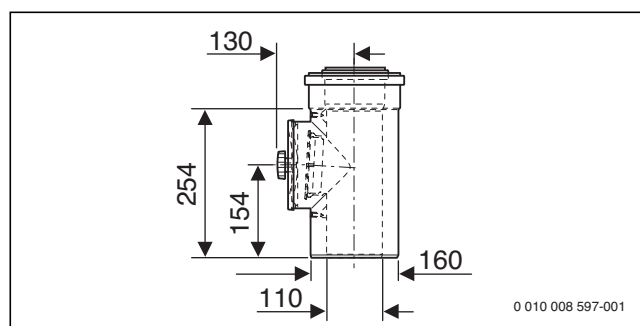
Bild 202 Konzentrisches Rohr mit Prüföffnung \varnothing 110/160 (Maße in mm)
