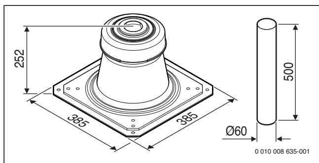
Bild 187 Schachtabdeckung für 60 mm, Kunststoff (Maße in mm)
