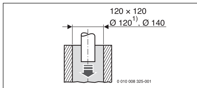
Bild 169 Mindestmaße des Schachtquerschnitts für die Montage der Abgasleitung (Maße in mm)
