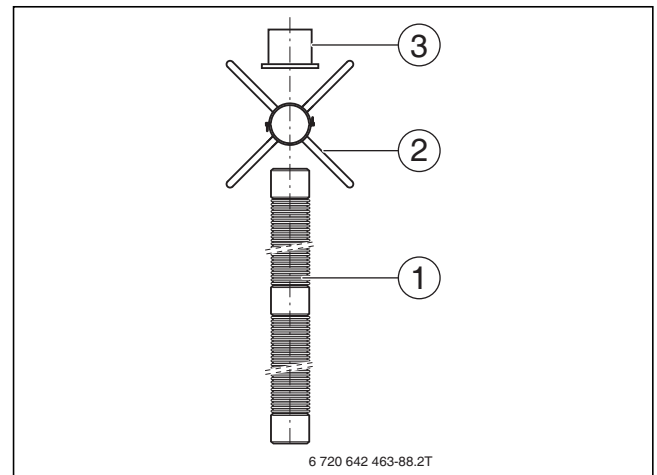
Bild 165 Bauteile des Grundbausatzes ÜB-Flex aus Kunststoff, DN 110, für Logamax plus GB192-50 i
