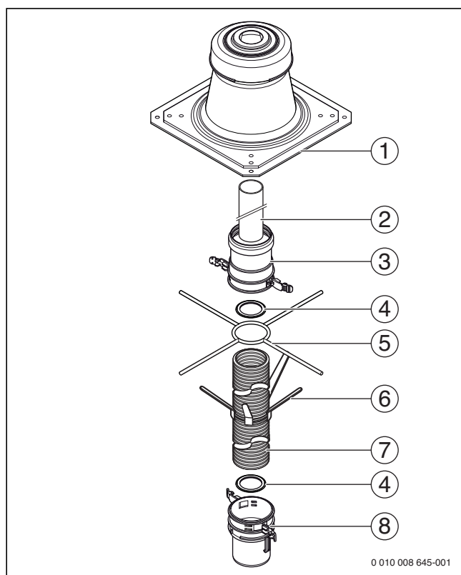
Bild 166 Bauteile des Grundbausatzes ÜB-Flex aus Kunststoff, DN 60, für Logamax plus GB192-15i(T) und GB192-25i(T)
