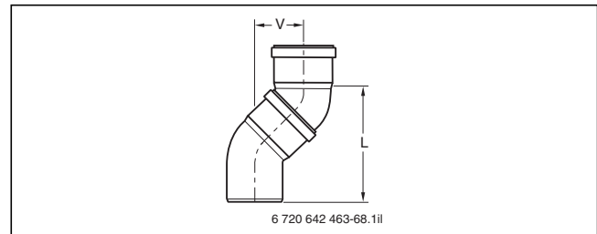
Bild 223 Versatzmaße
