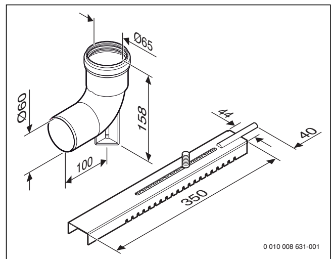
Bild 182 Stützbogen mit Auflageschiene Ø 60 mm (Maße in mm)
