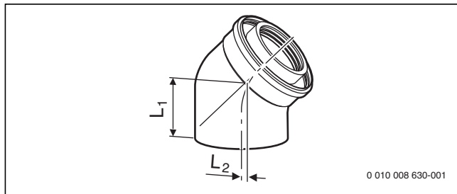
Bild 204 Konzentrischer Bogen Ø 60/100 (Maße → Tabelle 99)
