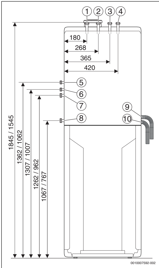
Bild 25 Anschlussmaße des Zubehörs Heizkreiserweiterung 2 (Maße in mm)
