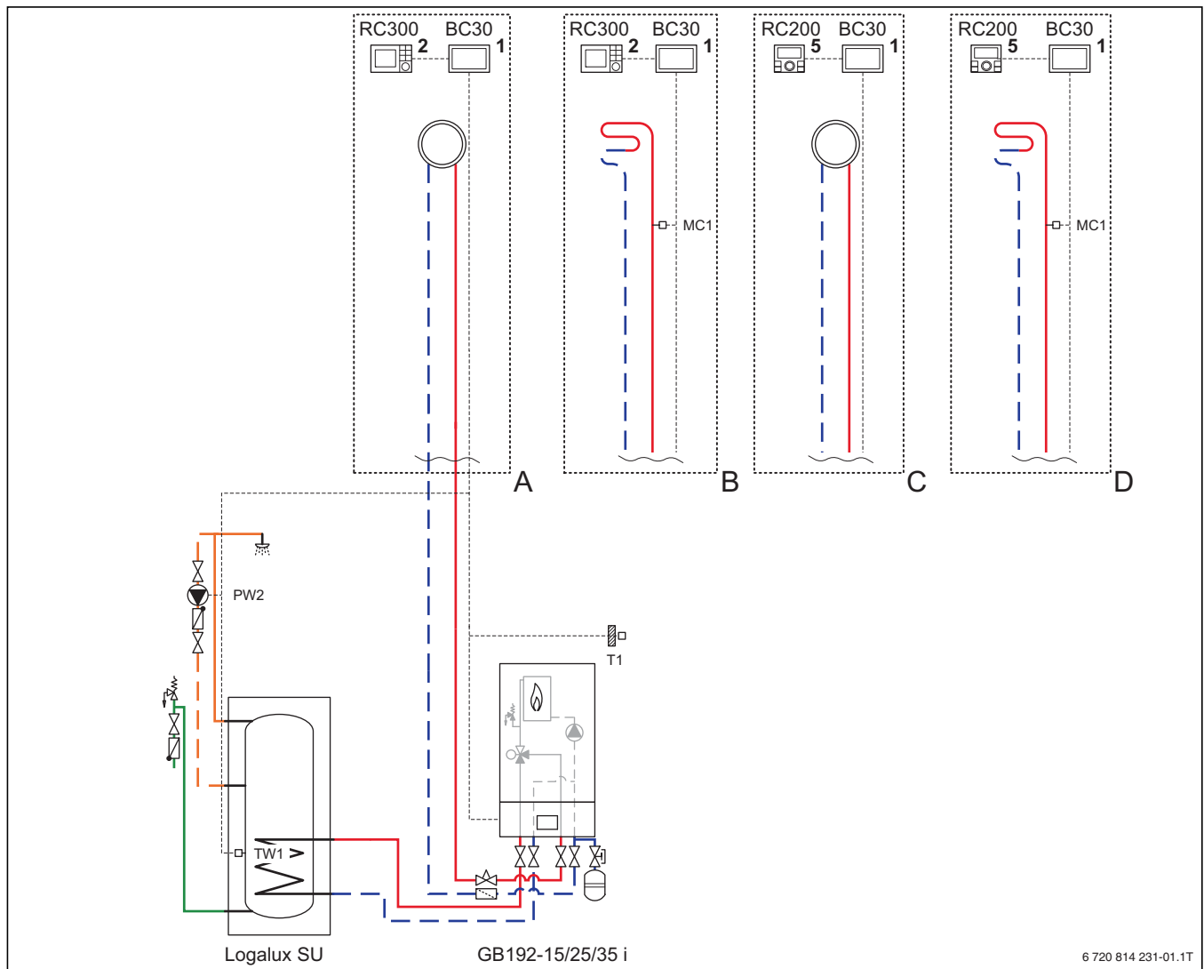
Bild 90 Anlagenschema mit Regelung (unverbindliche Prinzipschuldarstellung)
