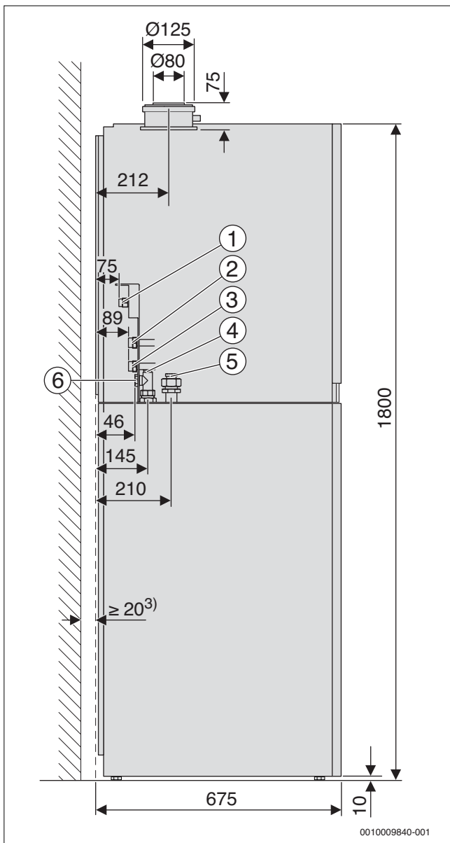
Bild 18 Abmessungen und Anschlüsse ohne Zubehör (Maße in mm)
