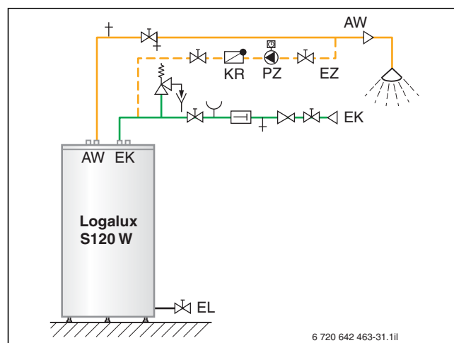
Bild 70 Variante einer Zirkulationsleitung für den Warmwasserspeicher Logalux S120/5W
