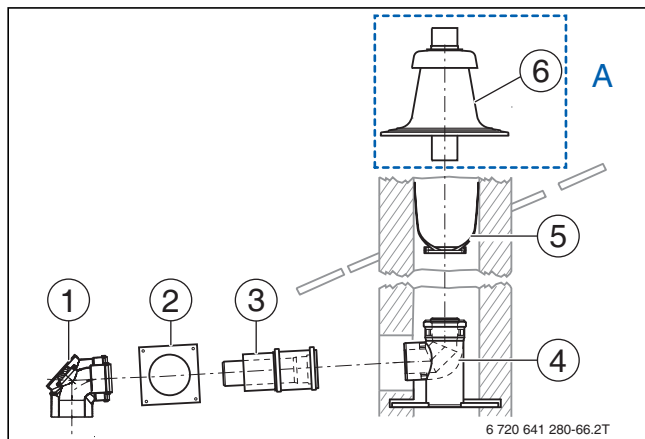
Bild 157 Bauteile Grundbausatz DO-S aus Kunststoff
