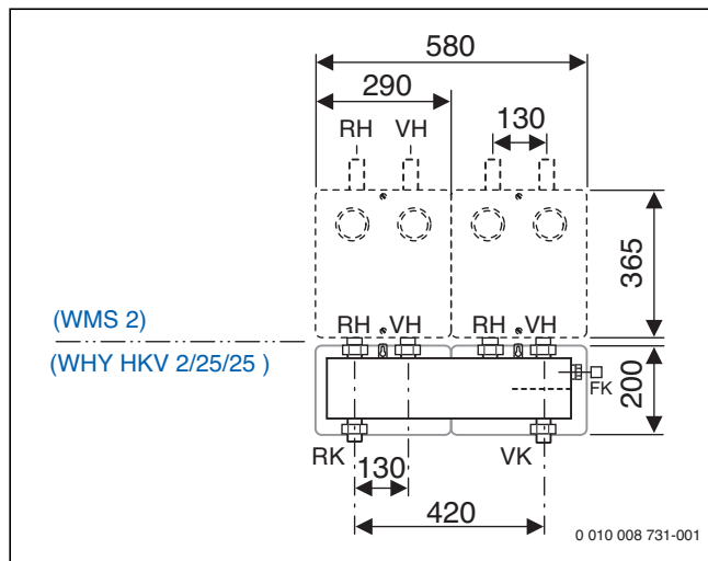
Bild 124 Abmessungen der Systemkombination Heizkreisverteiler mit integrierter hydraulischer Weiche für zwei Heizkreise (Maße in mm)
