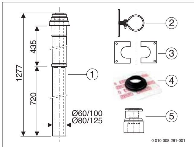
Bild 151 Bauteile des Grundbausatzes DO aus Kunststoff (Maße in mm)
