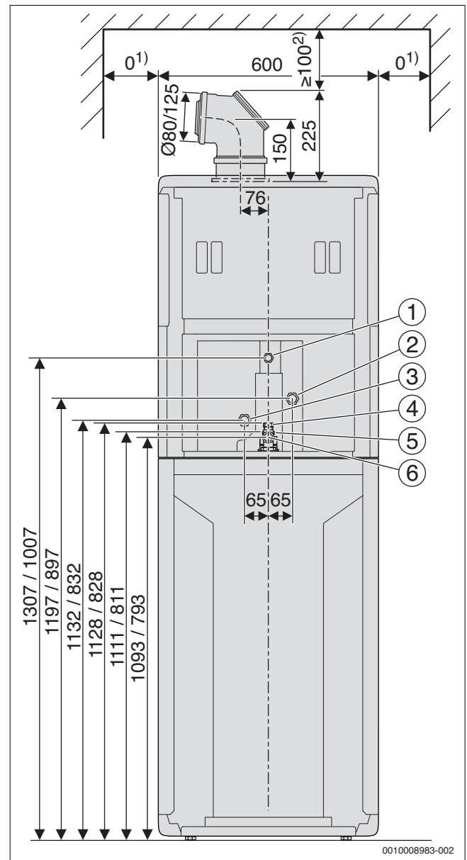
Bild 15 Abmessungen und Anschlüsse ohne Zubehöre, Rückansicht, (Maße in mm)
