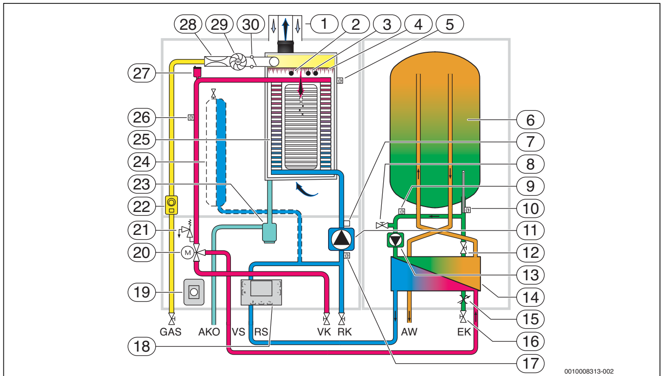
Bild 8 Funktionsschema Logamax plus GB192-30 iT40S
