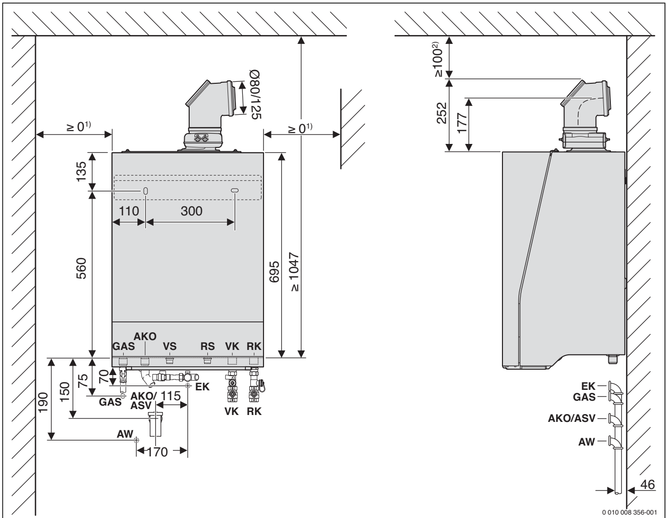
Bild 32 Montagemaße der Zuleitungen Logamax plus GB192-15/25/35 i bei Verwendung der Zubehör-Sets für die Aufputzinstallation (Maße in mm)
