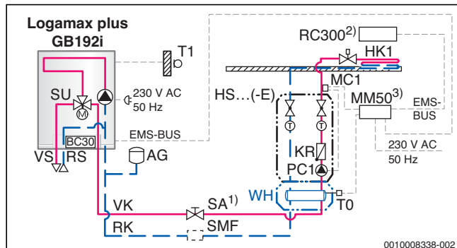
Bild 79 Beispiel für eine nicht direkt nachgeschaltete Fußbodenheizung (Abkürzungsverzeichnis → Seite 70)
