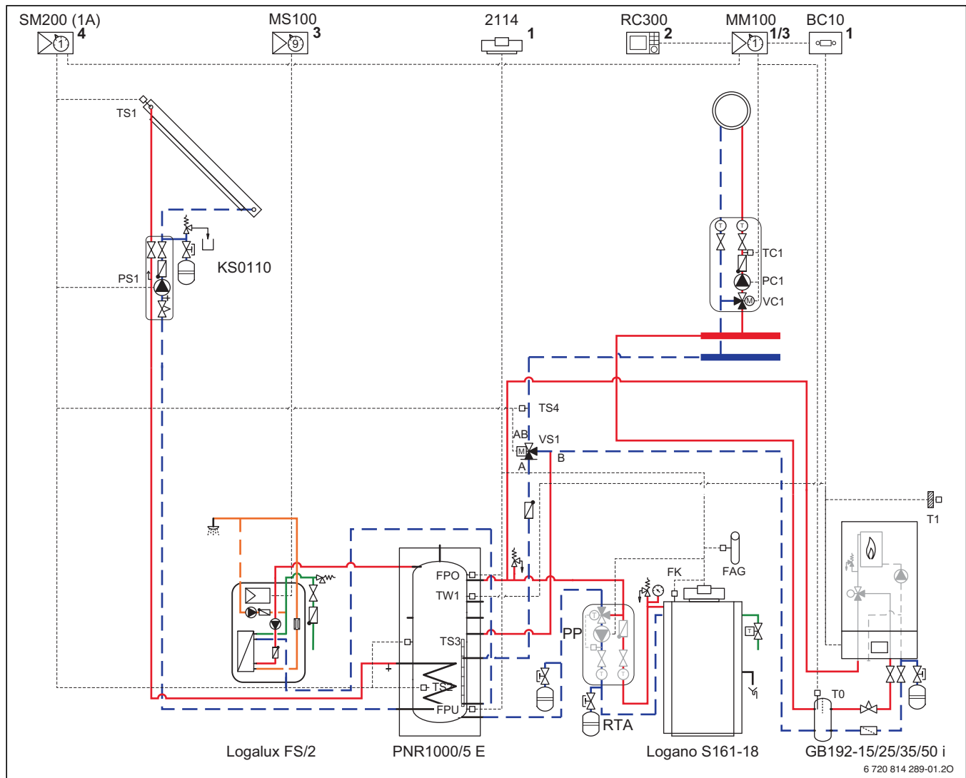
Bild 106 Anlagenschema mit Regelung (unverbindliche Prinzipdarstellung)
