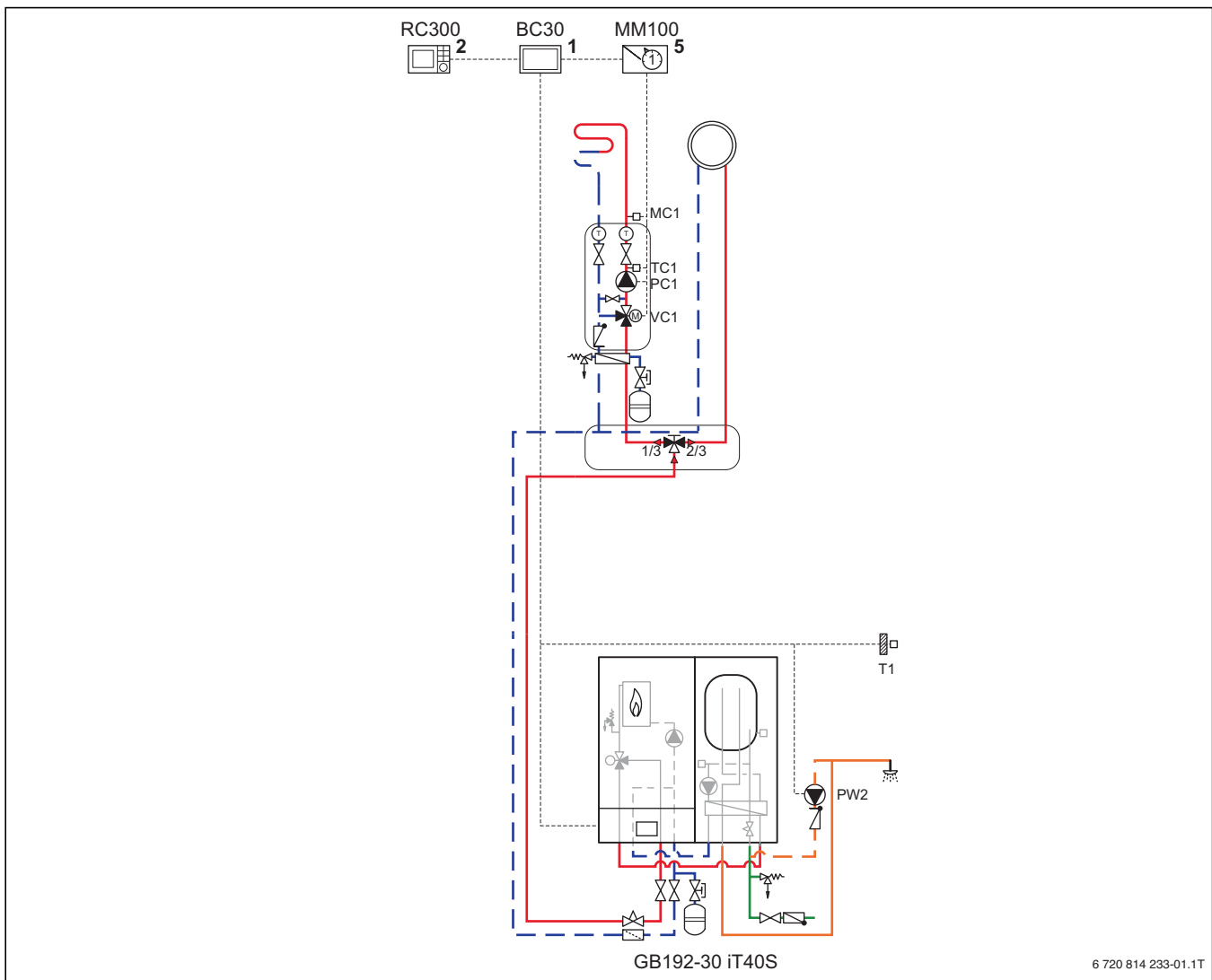
Bild 91 Anlagenschema mit Regelung (unverbindliche Prinzipdarstellung)
