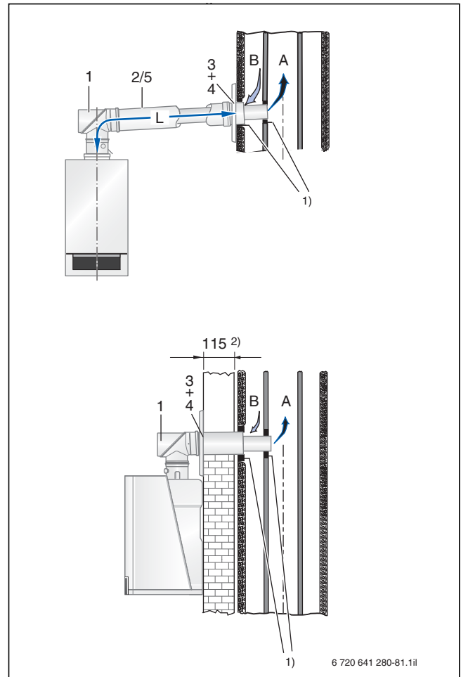
Bild 176 Montagevarianten (Maße in mm)
