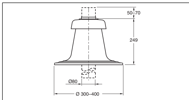
Bild 189 Schachtabdeckung für 110 mm (Maße in mm)
