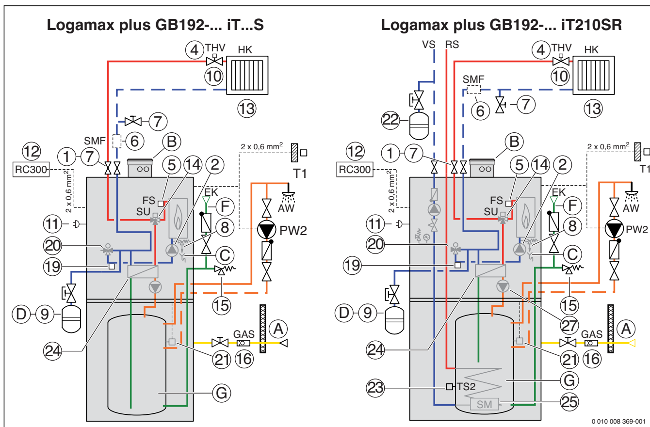
Bild 74 Hydraulik Logamax plus GB192... iT...S und GB192... iT210SR (Planungshinweise → Tabelle 29, Seite 76)
