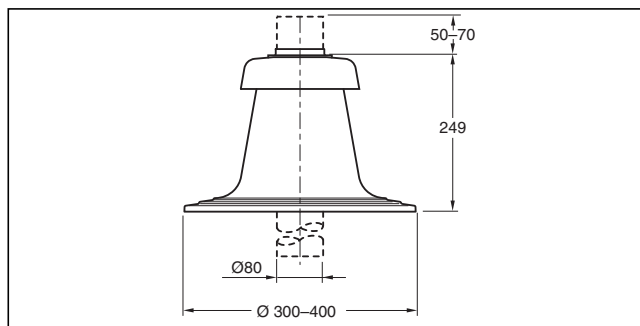
Bild 188 Schachtabdeckung für 80 mm (Maße in mm)
