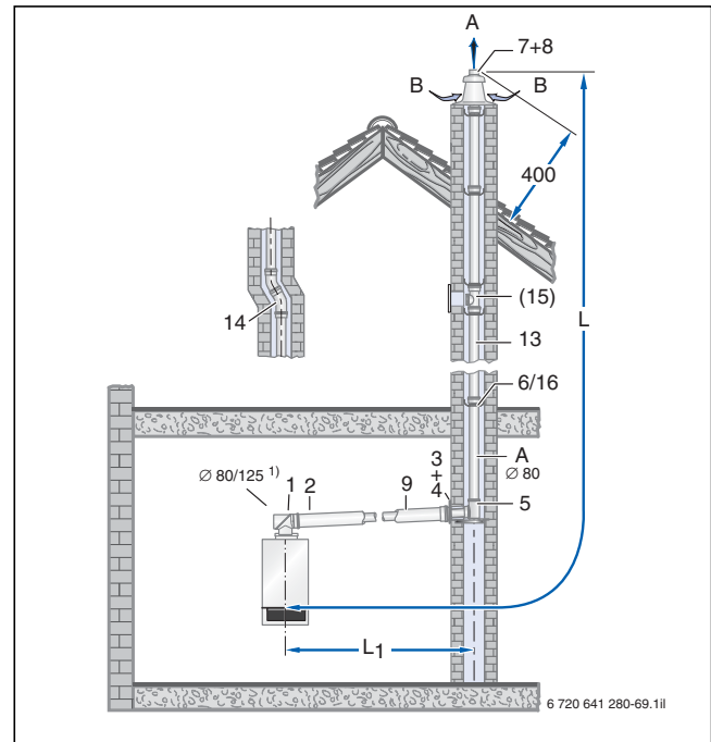
Bild 160 Montagevariante (Maße in mm)
