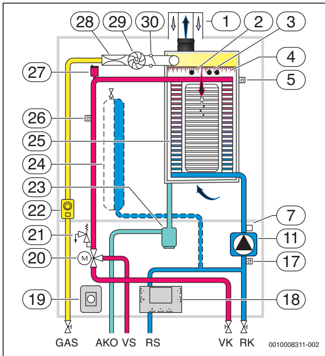
Bild 6 Funktionsschema Logamax plus GB192-15/25/35 i (Legende → Seite 15)
