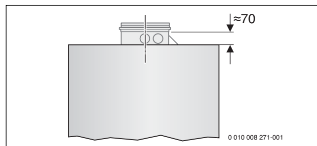
Bild 150 Montage der konzentrischen Anschlussstücke
