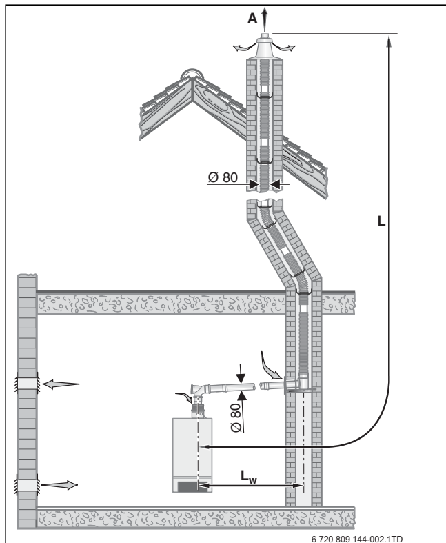
A Abgas B Hinterlüftung C Zuluft 1) Lüftungsöffnung ins Freie 1 \times 150 \text{ cm}^2 oder 2 \times 75 \text{ cm}^2
