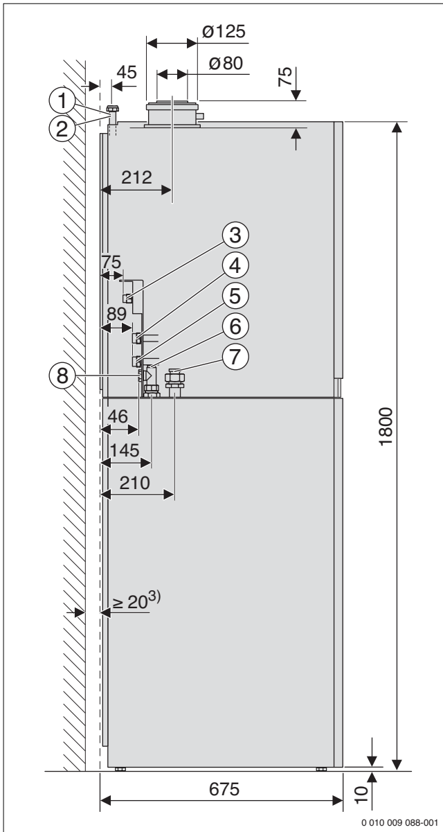
Bild 16 Abmessungen und Anschlüsse ohne Zubehöre (Maße in mm)
