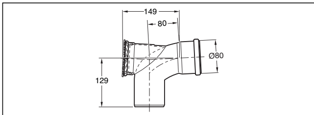
Bild 178 Bogen mit Prüföffnung lang (Maße in mm)
