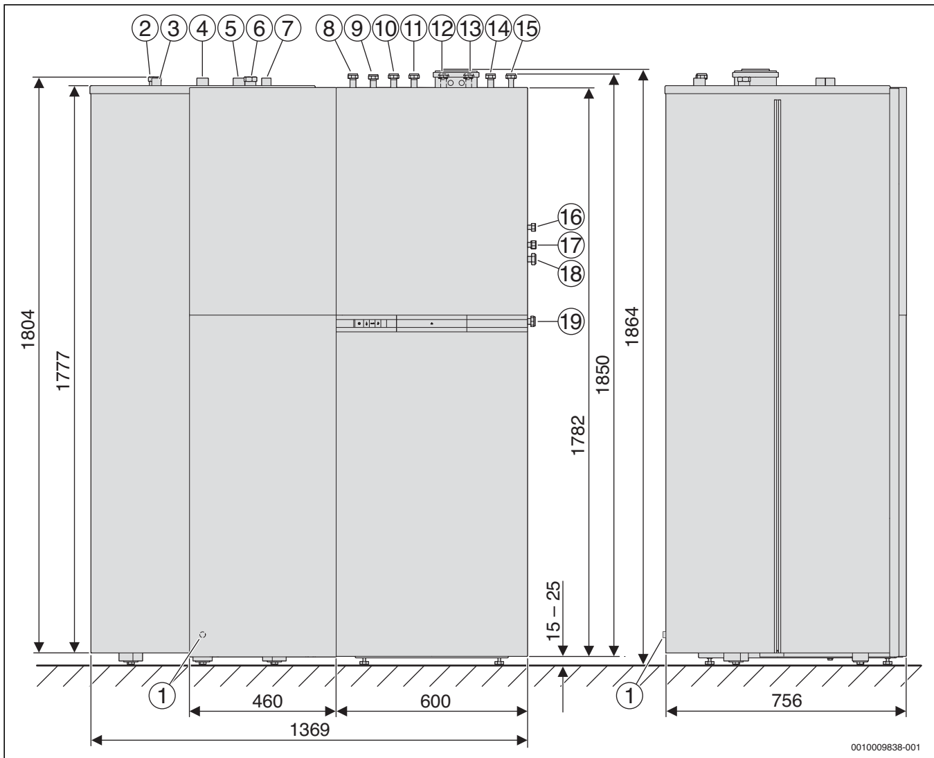
Bild 35 Ansicht GBH192-... iT150...
