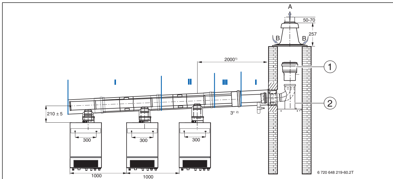
Bild 175 Bauteile des Bausatzes Kaskade RLU, DN 110/160
