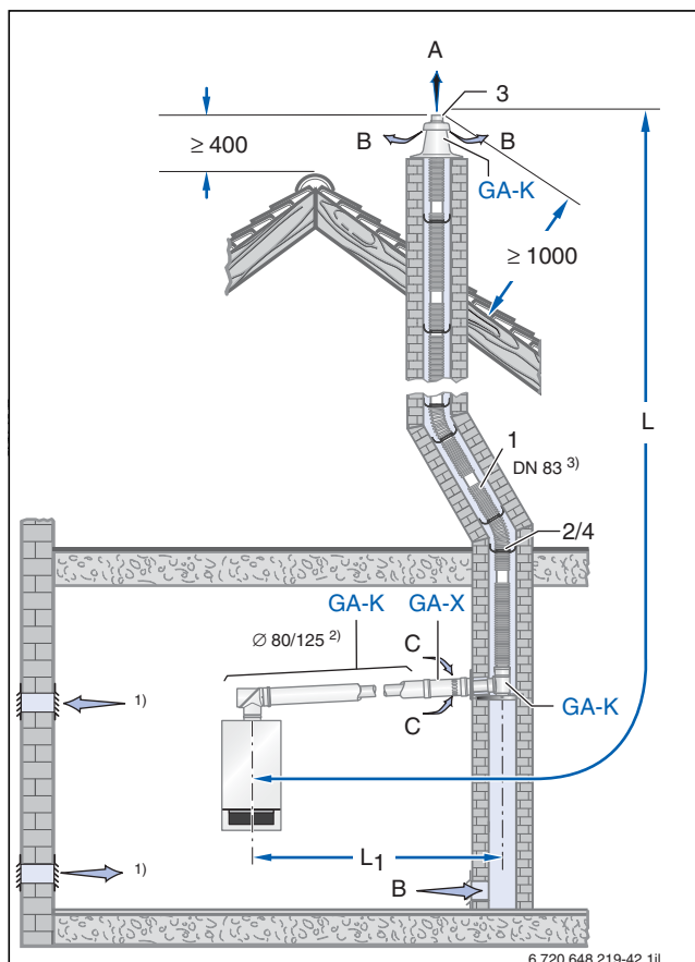
Bild 139 Montagevariante (Maße in mm)
