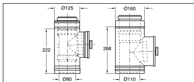
Bild 203 Konzentrisches Rohr mit Prüföffnung (Maße in mm)
