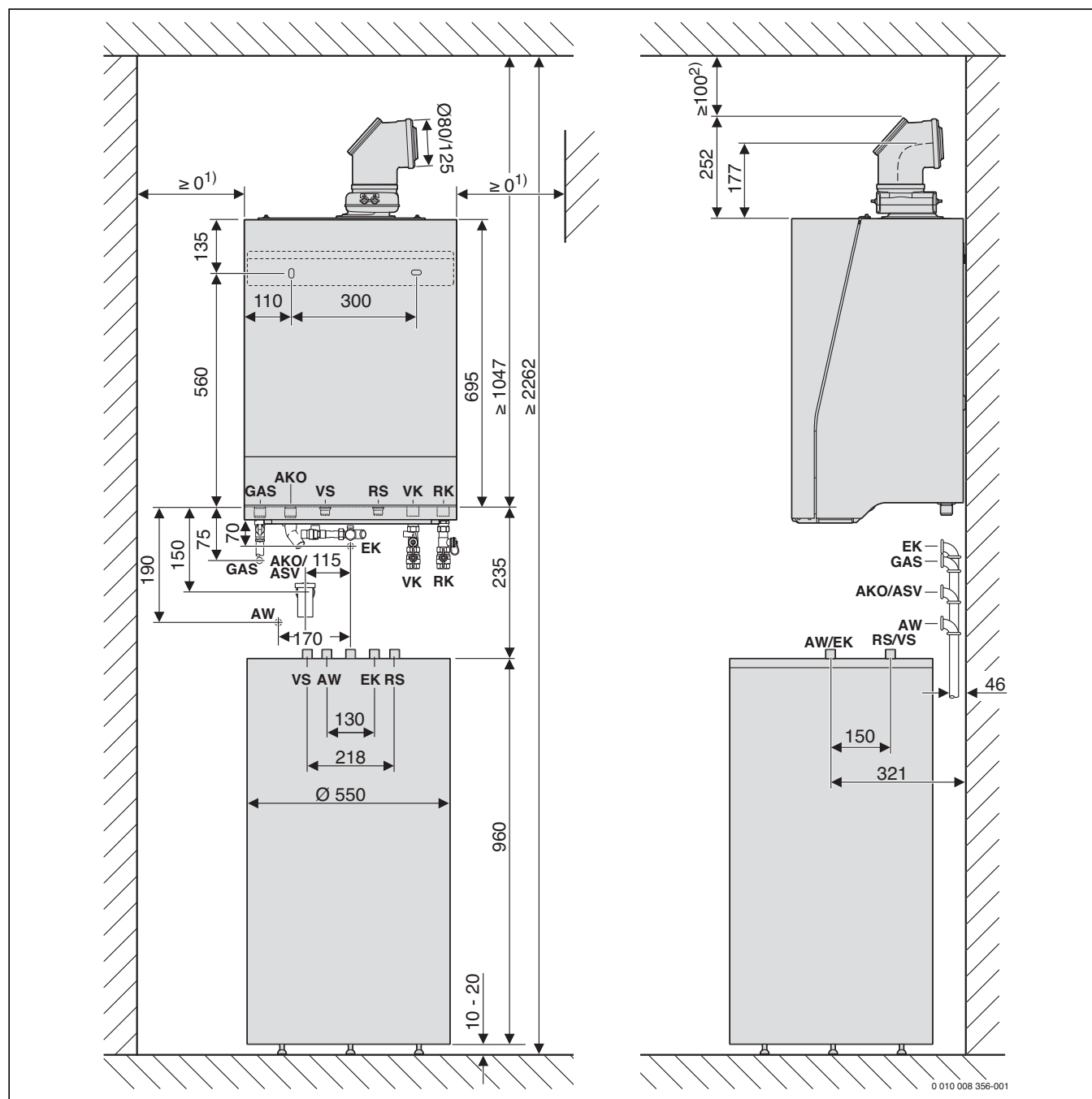
Bild 33 Montagemaße der Zuleitungen bei Verwendung der Zubehör-Sets für die Aufputzinstallation und Anordnung Logalux S120/5W unter Logamax plus GB192-15/25/35 i (Maße in mm)
