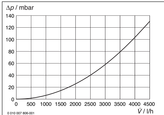
Bild 85 Druckverlust-Diagramm ungemischter Heizkreis (HK1)
