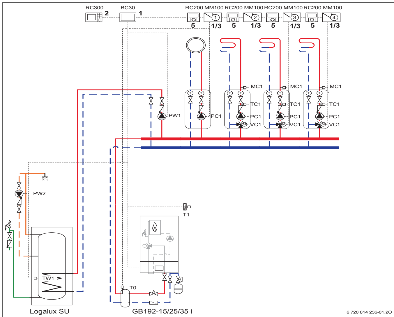
Bild 95 Anlagenschema mit Regelung (unverbindliche Prinzipschuldarstellung)
