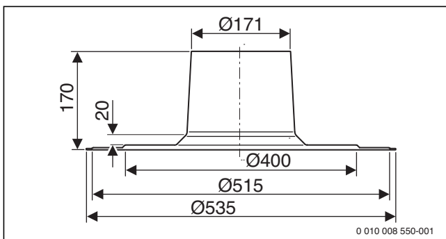
Bild 193 Flachdach-Klebeflansch für DN 110/160 (Maße in mm)
