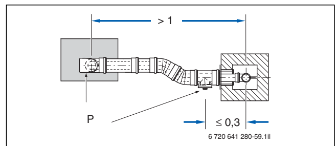
Bild 148 Beispiel zur Anordnung der Prüföffnungen (P) bei einer waagerechten Abgasleitung mit Umlenkung im Aufstellraum – Draufsicht (Maße in m)
