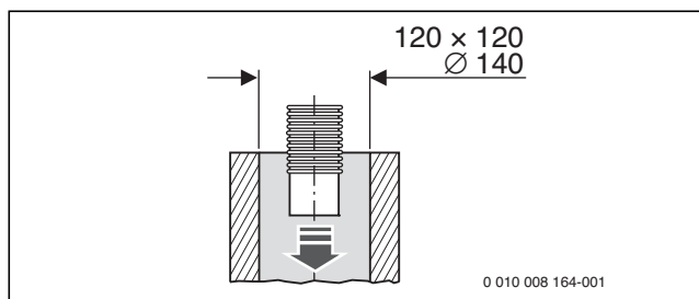
Bild 138 Mindestmaße des Schachtquerschnitts für die Montage der flexiblen Abgasleitung bis Kesselgröße 50 kW (Maße in mm)
