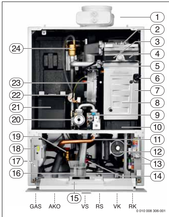
Bild 3 Ausgewählte Bauteile und Baugruppen Logamax plus GB192i (verdeckte Anschlüsse → Bild 6 und Bild 7, Seite 14)
