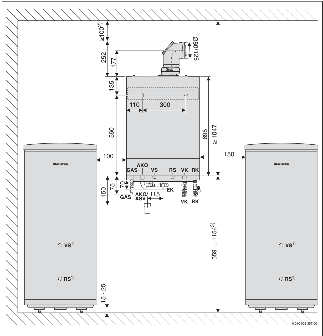
Bild 34 Montagemaße der Zuleitungen bei Verwendung der Zubehör-Sets für die Aufputzinstallation und Anordnung Logalux SU... /5W rechts oder links neben Logamax plus GB192-15/25/35 i (Maße in mm)
