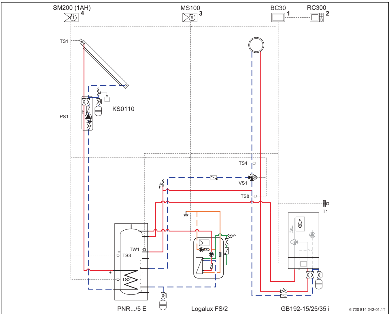
Bild 99 Anlagenschema mit Regelung (unverbindliche Prinzipdarstellung)
