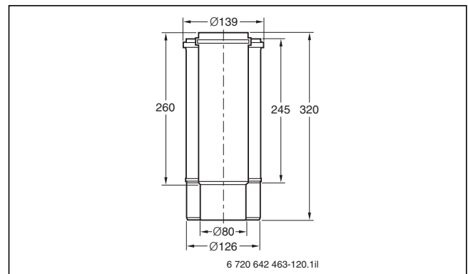
Bild 154 Konzentrisches Schiebestück DN 80/125 (Maße in mm)
