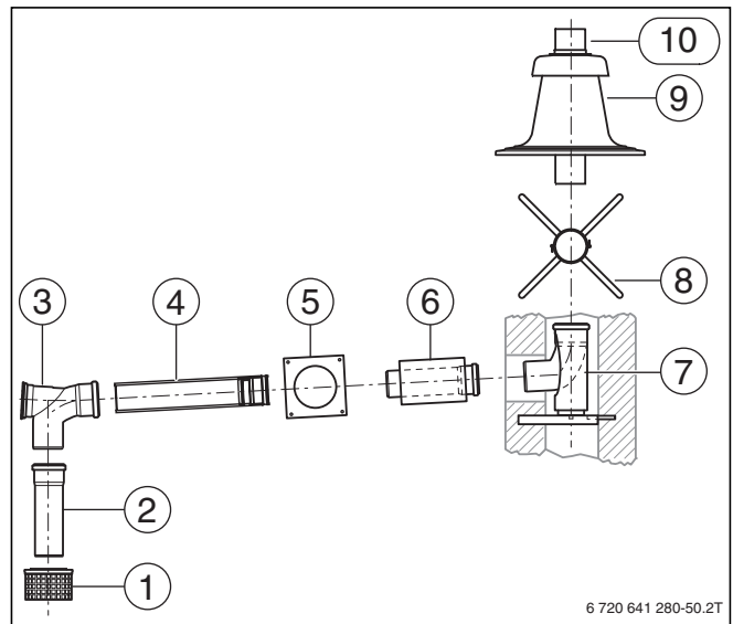
[1] Zuluftgitter [2] Abgasrohr, 250 mm lang [3] Bogen mit Prüfföffnung [4] Abgasrohr, 500 mm lang [5] Blende [6] Konzentrische Mauerdurchführung, Ø 80 mm, 500 mm lang Ø 125 mm, 300 mm lang [7] Bogen 87° inklusive Abstützung und Auflage- schiene [8] Abstandshalter (6 Stück) [9] Schachtabdeckung [10] Mündungsrohr ohne Muffe, Ø 80 mm, 500 mm lang Im Lieferumfang zusätzlich enthalten: - eine Tube Centrocerein - Systemzertifizierungsaufkleber
