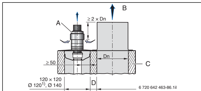
Bild 159 Mindestmaße des Schachtquerschnitts und der Schachtmündung für die Abgasleitung (Maße in mm)
