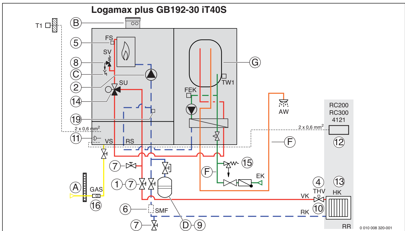
Bild 73 Hydraulik Logamax plus GB192-30 iT40S (Planungshinweise → Tabelle 29, Seite 76)
