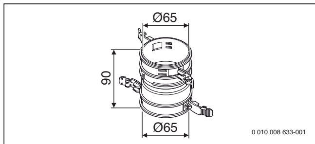
Bild 184 Verbindungsstück Flex Ø 60 mm (Maße in mm)
