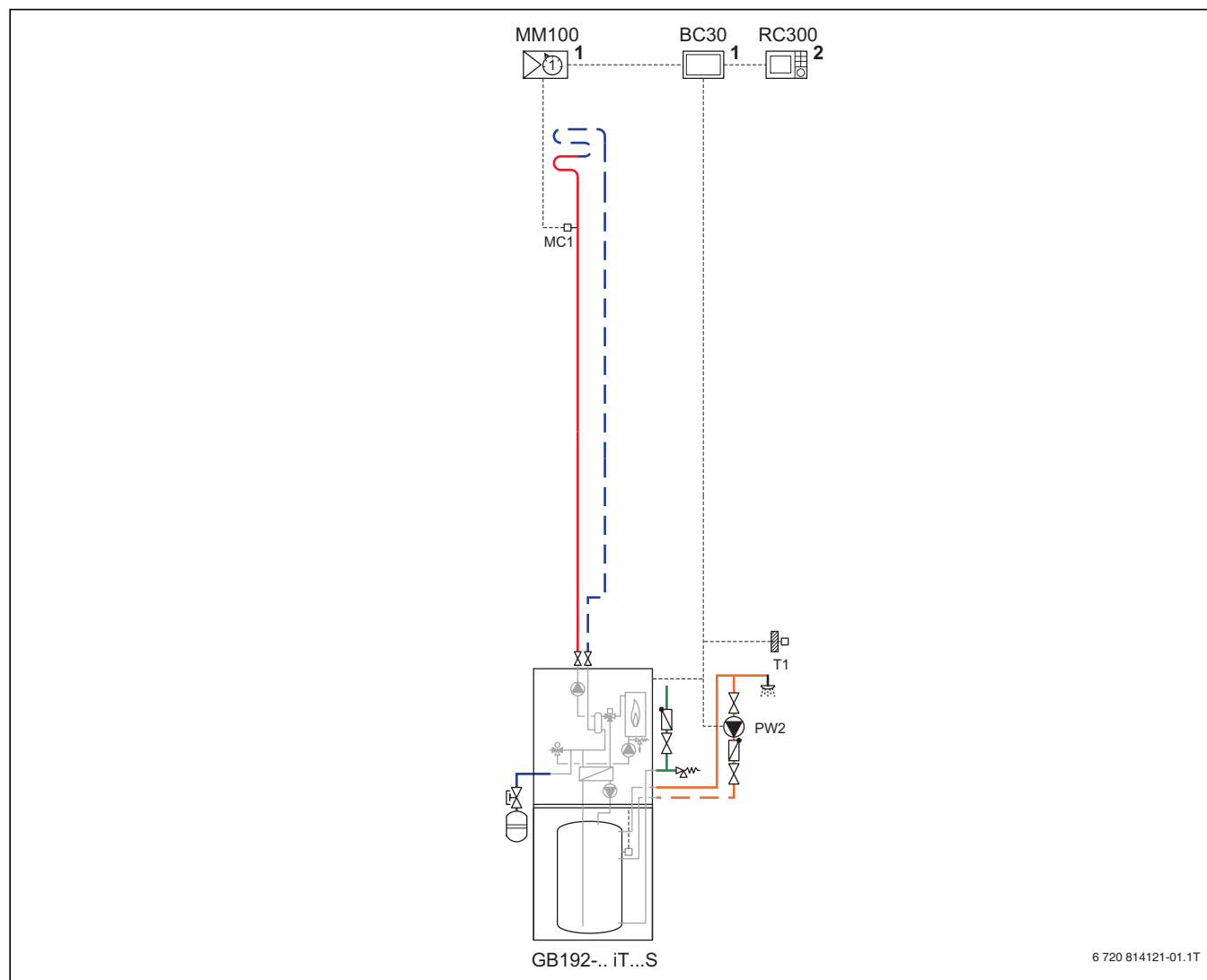
Bild 108 Anlagenschema mit Regelung (unverbindliche Prinzipdarstellung)
