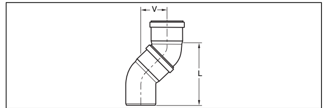
Bild 181 Versatzmaße Bogen
