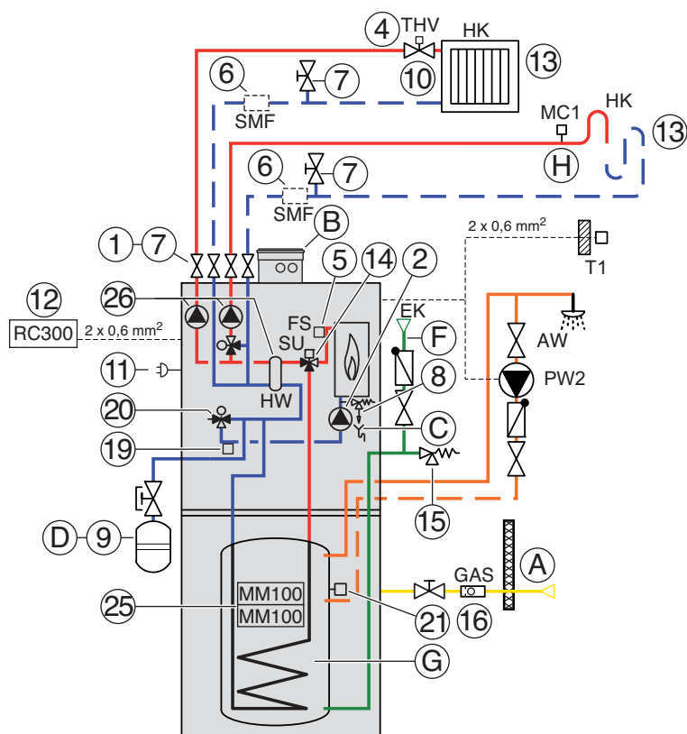
Bild 75 Hydraulik Logamax plus GB192-15/25 iT150 (Planungshinweise → Tabelle 29, Seite 76)
