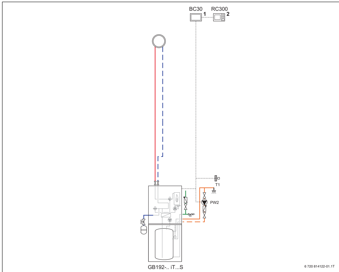
Bild 107 Anlagenschema mit Regelung (unverbindliche Prinzipdarstellung)
