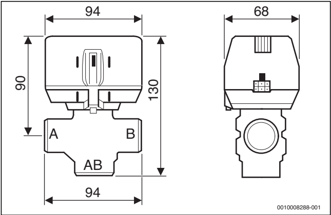
Bild 68 Maße des externen 3-Wege-Ventils für Logamax plus GB192-50 i
