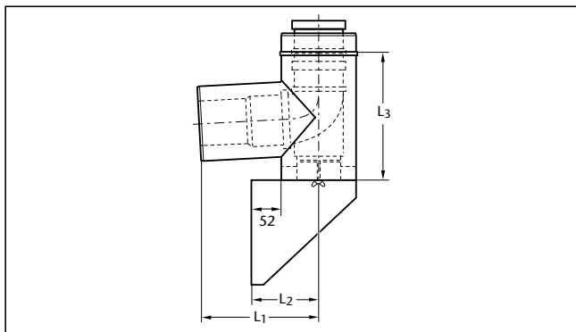
Bild 211 Konzentrisches Zuluft-T-Stück (Maße → Tabelle 102)
