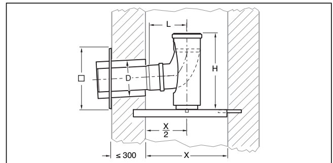
Bild 210 Konzentrischer Schornsteinanschluss (Maße in mm)
