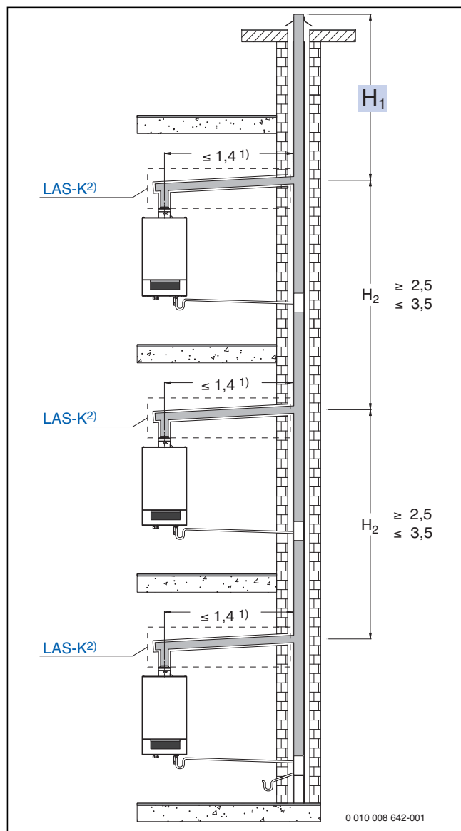
Bild 172 Montagevarianten (Maße in m)
