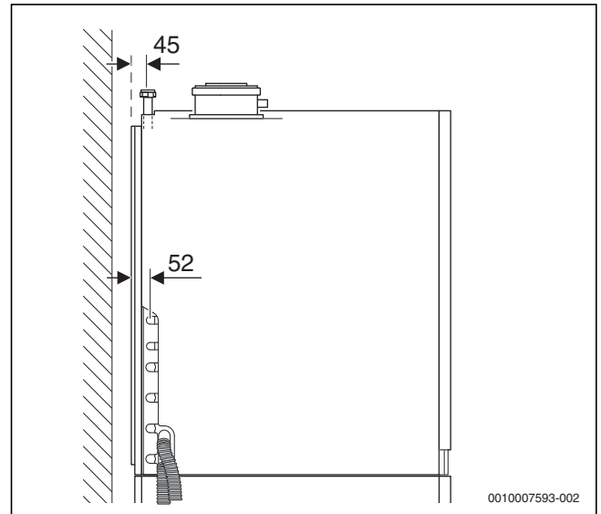
Bild 24 Anschlussmaße des Zubehörs Heizkreiserweiterung 1 (Maße in mm)
