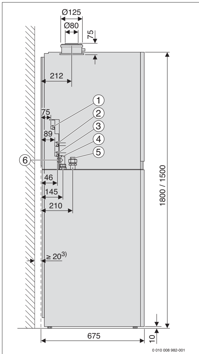
Bild 14 Abmessungen und Anschlüsse ohne Zubehöre (Maße in mm)
