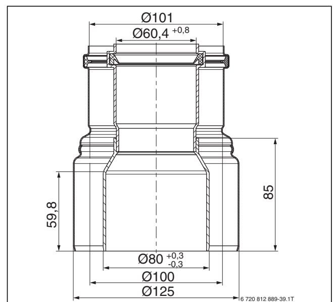
Bild 228 Konzentrische Reduktion DN 80/125 auf DN 60/100
