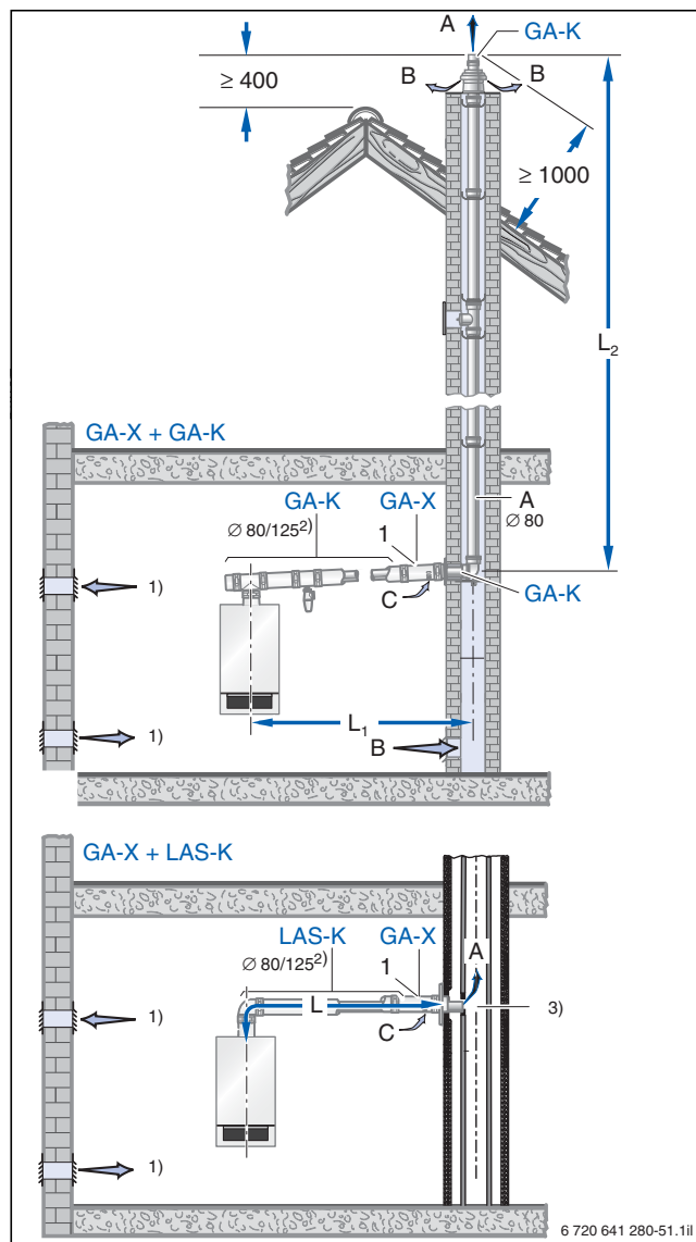
Bild 136 Montagevariante (Maße in mm)
