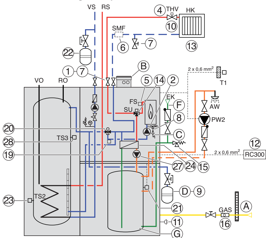
Bild 76 Hydraulik Logamax plus GBH192-... iT...S (Planungshinweise → Tabelle 29, Seite 76)
