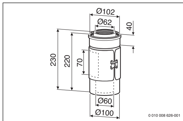
Bild 200 Konzentrisches Rohr mit Prüföffnung \varnothing 60/100 (Maße in mm)
