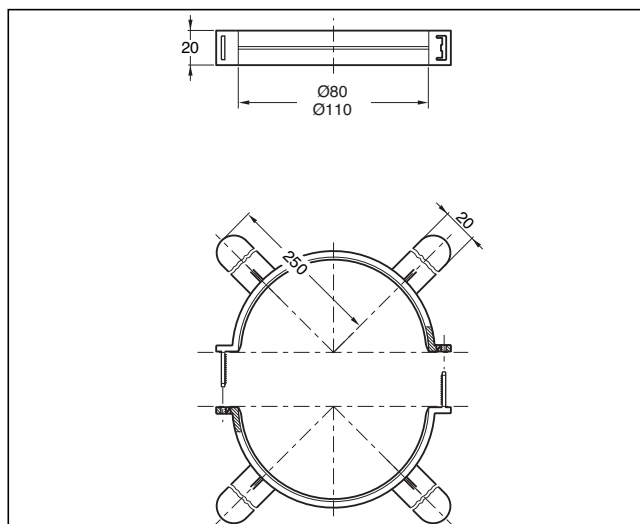
Bild 190 Abstandshalter für Abgasleitung im Schacht (Maße in mm)
