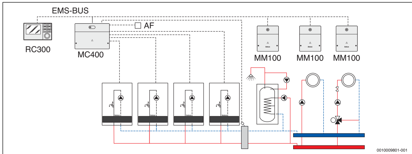
Bild 56 Kaskadenmodul MC400
