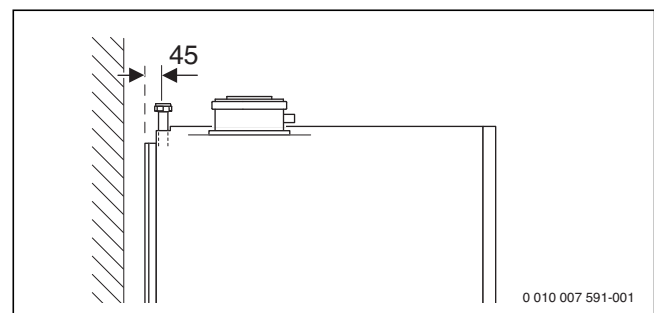
Bild 22 Anschlussmaße des Zubehörs AS-V1/Vertikales Anschluss-Set (Maße in mm)
