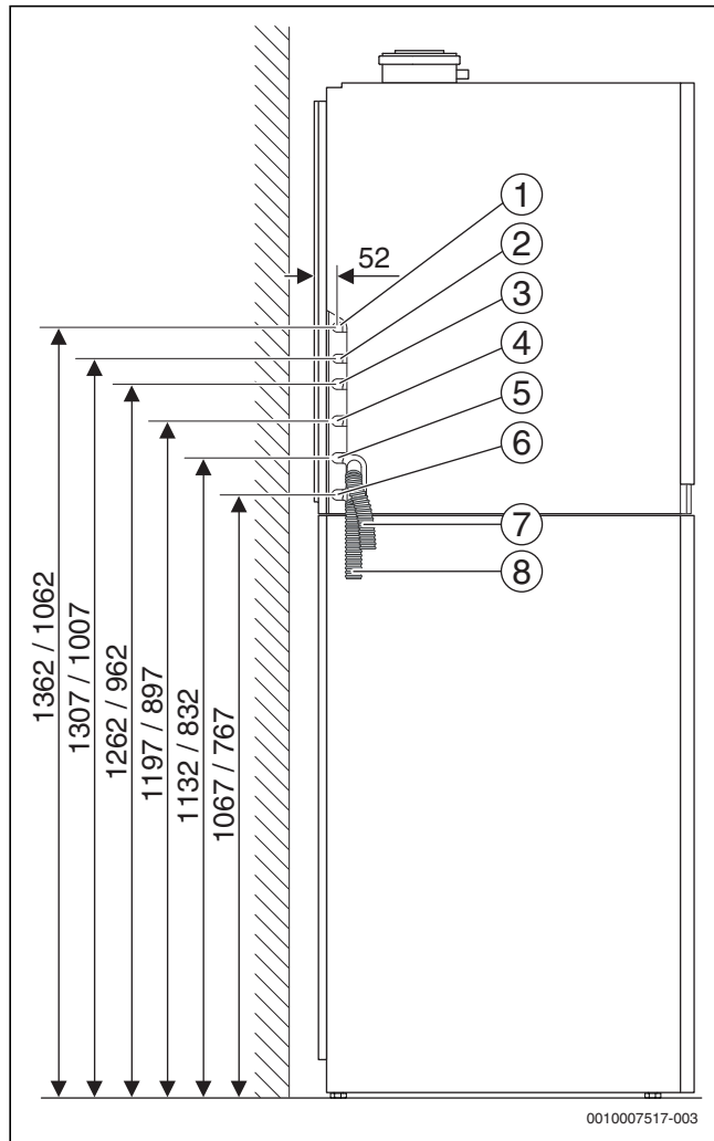
Bild 20 Anschlussmaße des Zubehörs AS-H1/Horizontales Anschluss-Set (Maße in mm)
