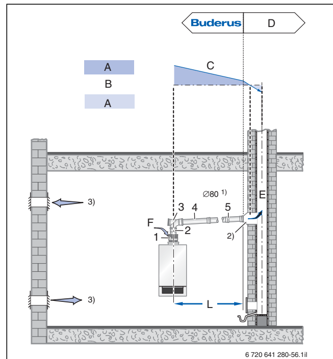
Bild 141 Montagevariante (Maße in mm)
