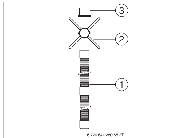
Bild 164 Bauteile des Grundbausatzes ÜB-Flex aus Kunststoff, DN 83, für Logamax plus GB192i(T)
