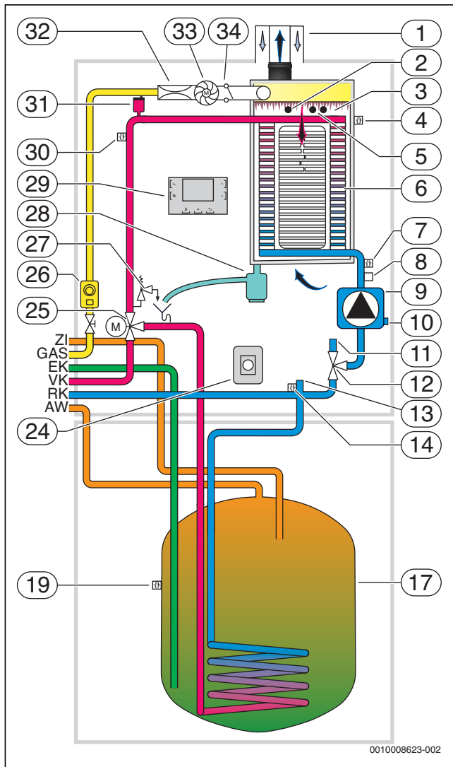
Bild 11 Funktionsschema Logamax plus GB192... iT... (Legende → Seite 15)
