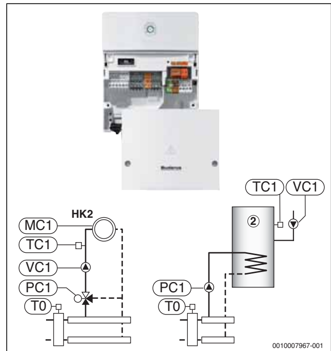
Bild 53 Heizkreismodul MM100
