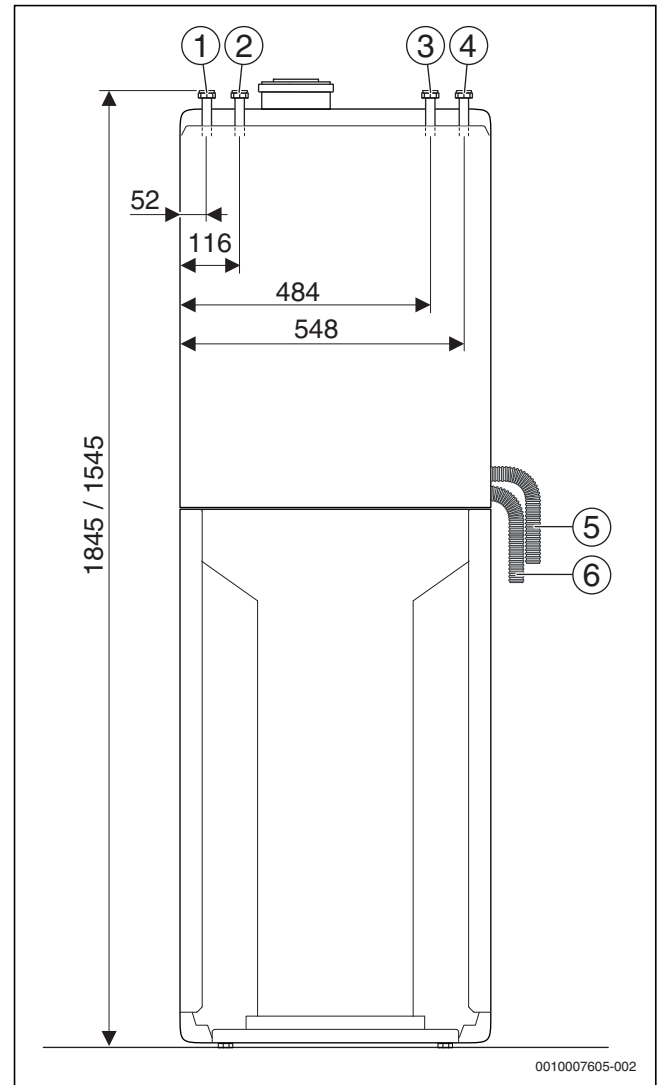
Bild 29 Anschlussmaße des Zubehörs Anschluss-Set solare Heizungsunterstützung SHU (Maße in mm)
