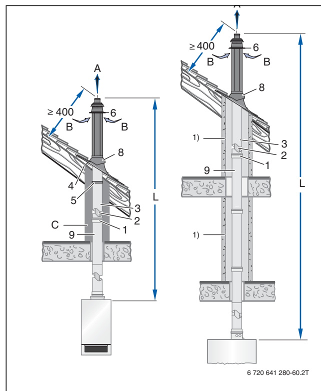
Bild 149 Montagevarianten (Maße in mm)
