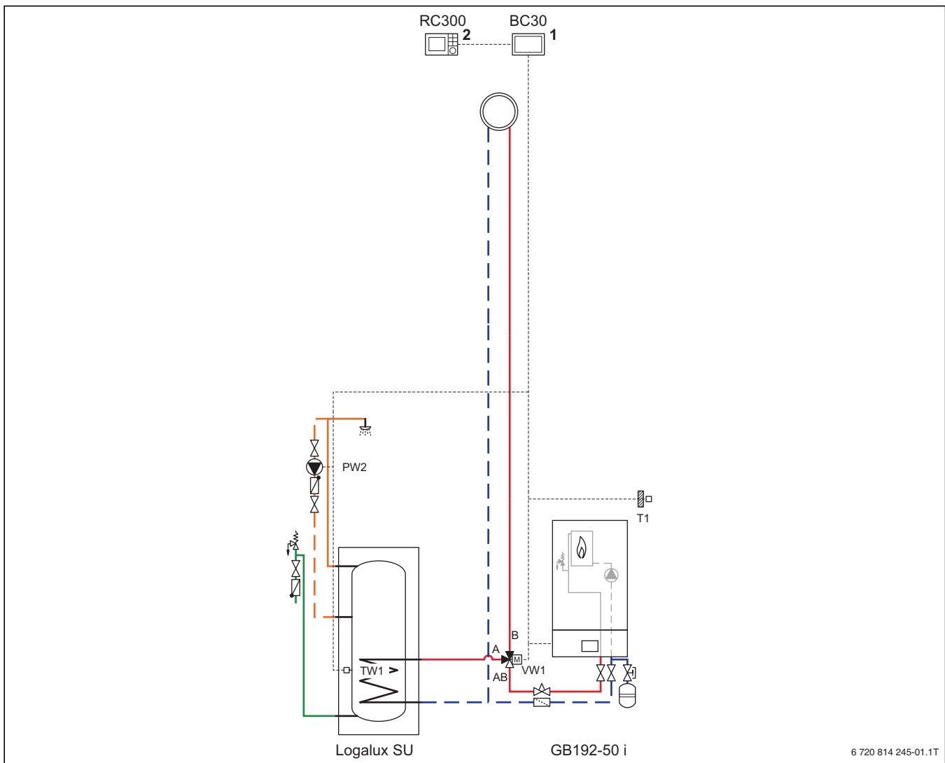
Bild 96 Anlagenschema mit Regelung (unverbindliche Prinzipdarstellung)
