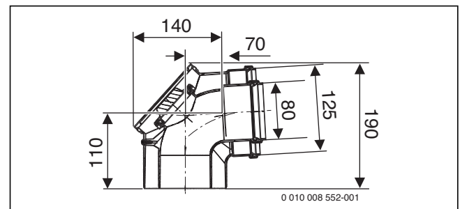
Bild 196 Konzentrischer Bogen mit Prüföffnung Ø 80/125 (Maße in mm)
