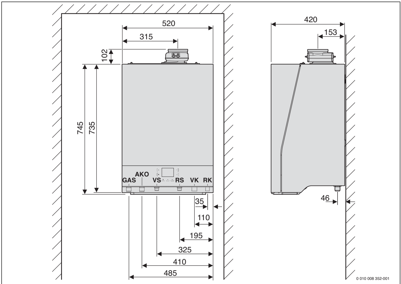
Bild 12 Abmessungen und Anschlüsse Logamax plus GB192i (Maße in mm)
