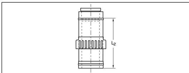
Bild 212 Konzentrischer Zuluftstutzen
