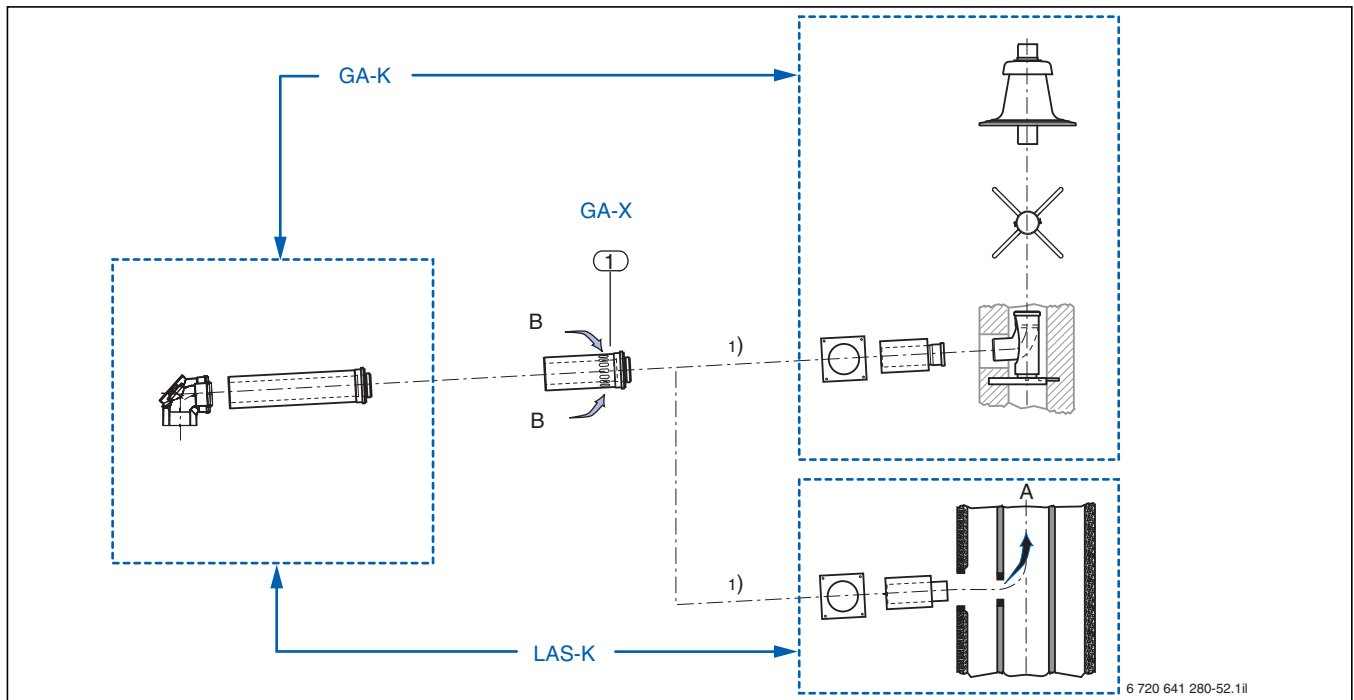
Bild 137 Bauteile des Grundbausatzes GA-X aus Kunststoff in Verbindung mit dem Grundbausatz GA-K (→ Tabelle 74, Seite 195) oder LAS-K (→ Tabelle 92, Seite 211)
