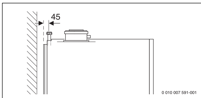
Bild 28 Anschlussmaße des Zubehörs Anschluss-Set Heizungsunterstützung HU (Maße in mm)
