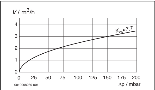
Bild 69 Durchflusskennlinie der externen 3-Wege-Ventile
