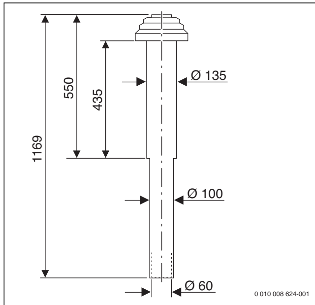
Bild 214 Dachdurchführung Ø 60/100 (Maße in mm)
