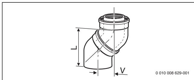
Bild 207 Versatzmaße konzentrischer Bogen Ø 60/100 (Maße → Tabelle 100)
