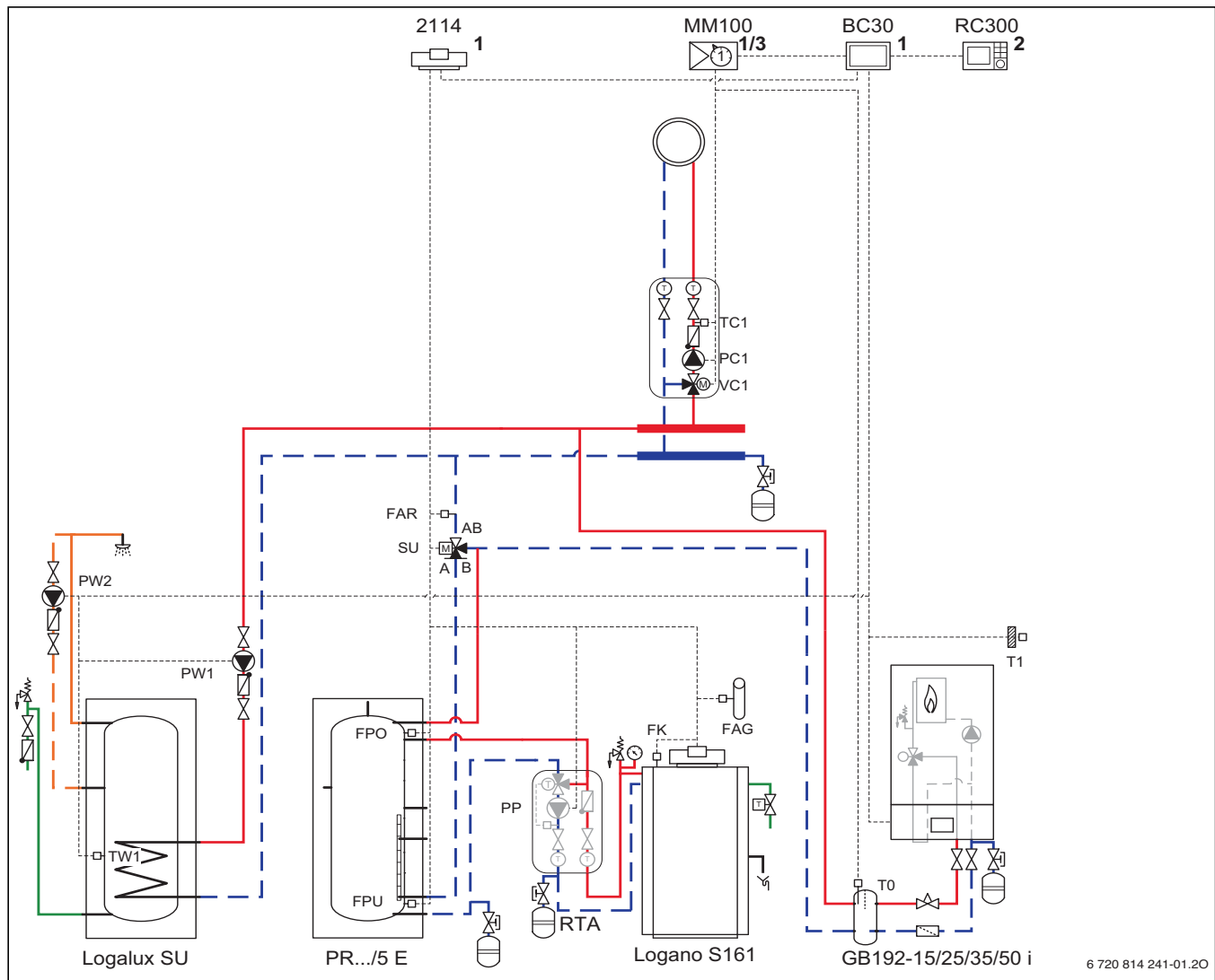
Bild 103 Anlagenschema mit Regelung (unverbindliche Prinzipdarstellung)
