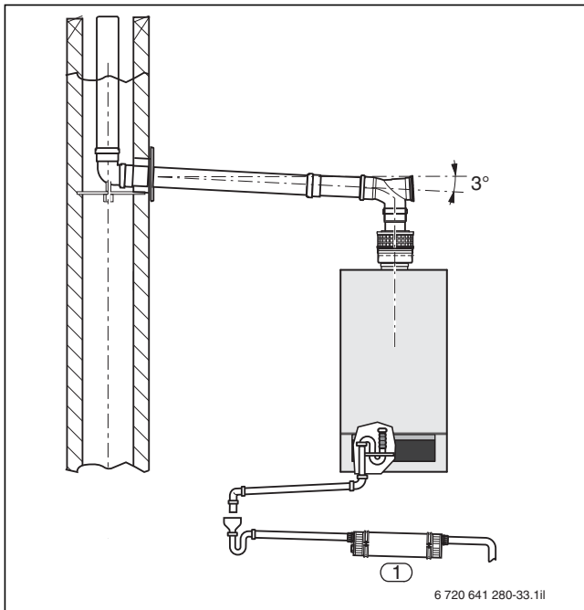
Bild 121 Kondensatschlauch aus dem Gas-Brennwertgerät und eine Kondensatableitung über die Neutralisationseinrichtung
