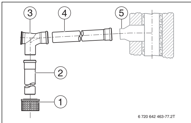
Bild 142 Bauteile des Grundbausatzes GN aus Kunststoff
