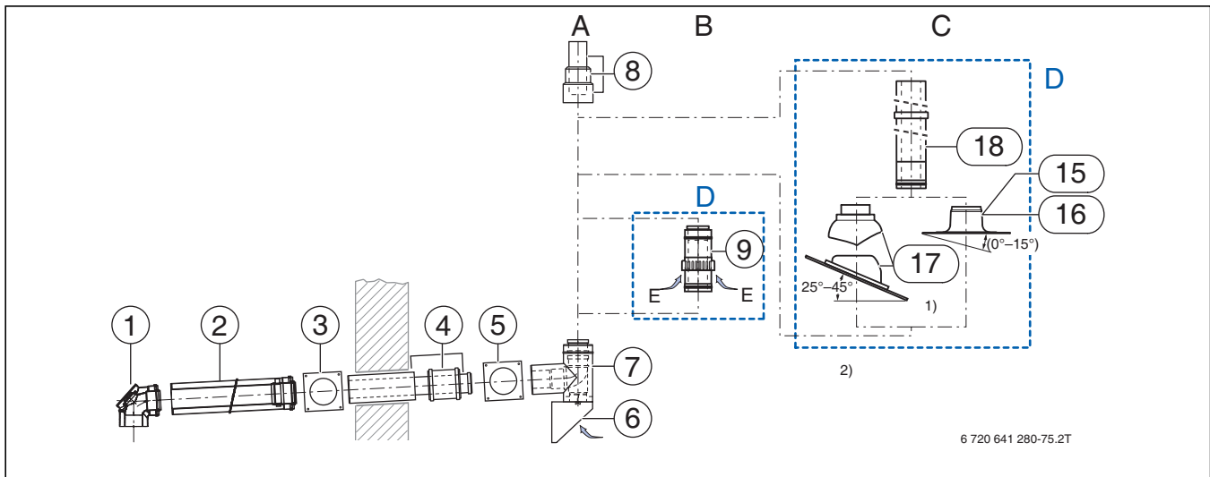
Bild 168 Bauteile des Grundbausatzes GAF-K aus Kunststoff
