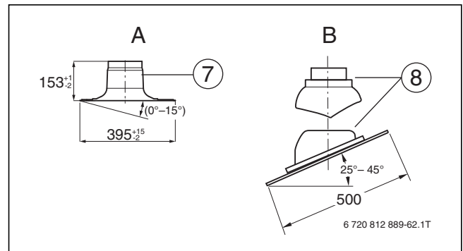
Bild 153 Universaldachpfannen und Flachdach-Klebeflansch als Zusatzausstattung für den Grundbausatz DO (unbedingt mitbestellen), (Maße in mm)
