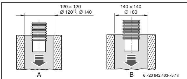
Bild 162 Mindestmaße des Schachtquerschnitts für die Montage der flexiblen Abgasleitung (Maße in mm)
