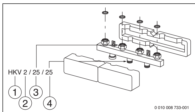
Bild 126 Nennweite Heizkreis-Schnellmontage-Systeme (Beispiel)
