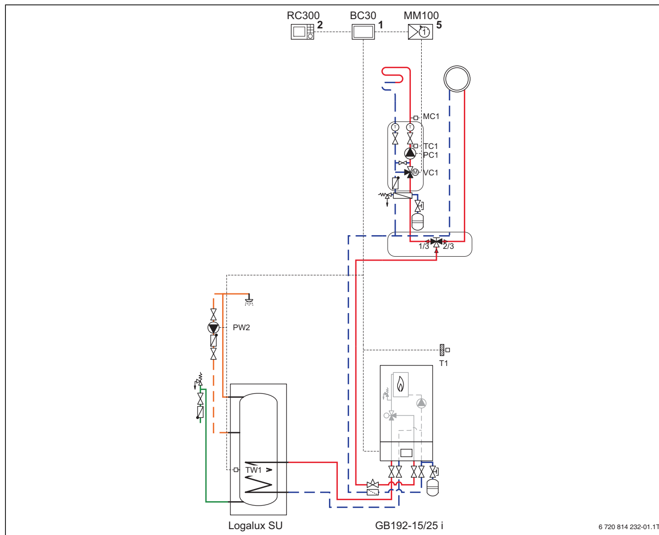
Bild 92 Anlagenschema mit Regelung (unverbindliche Prinzipdarstellung)
