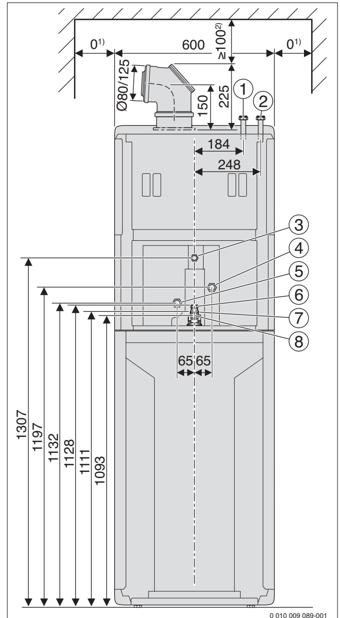
Bild 17 Abmessungen und Anschlüsse ohne Zubehöre, Rückansicht, (Maße in mm)
