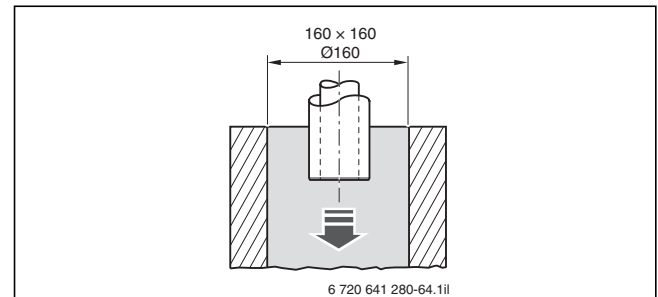
Bild 155 Mindestmaße des Schachtquerschnitts für die Montage der Luft-Abgas-Leitung (Maße in mm)
