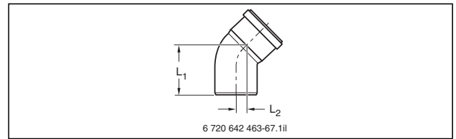
Bild 217 Bogen
