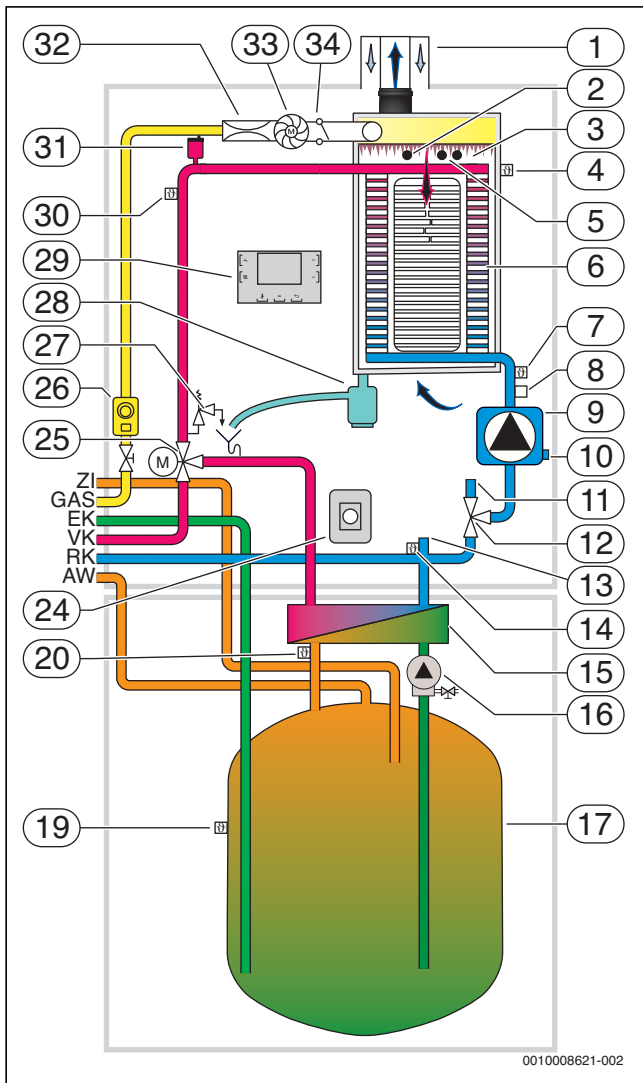
Bild 9 Funktionsschema Logamax plus GB192... iT...S (Legende → Seite 15)
