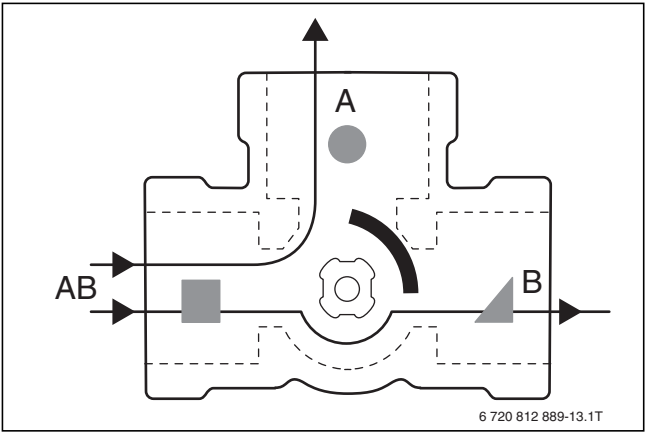
Bild 100 Mischventil als Verteilventil
