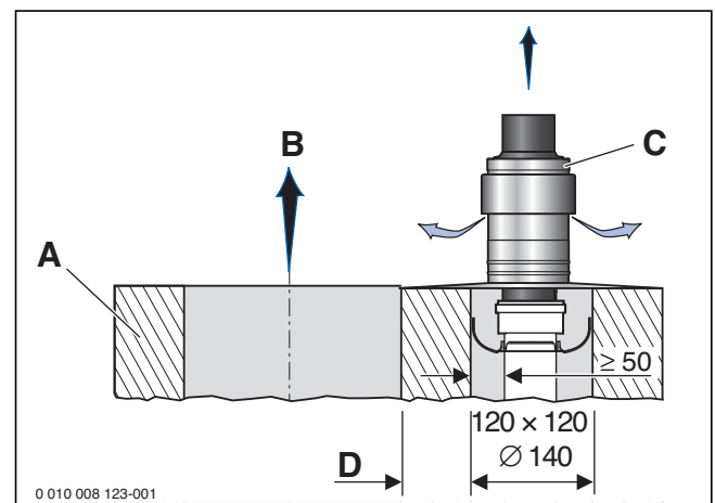
Bild 132 Mindestmaße des Schachtquerschnitts und der Schachtmündung für die Abgasleitung (Maße in mm)
