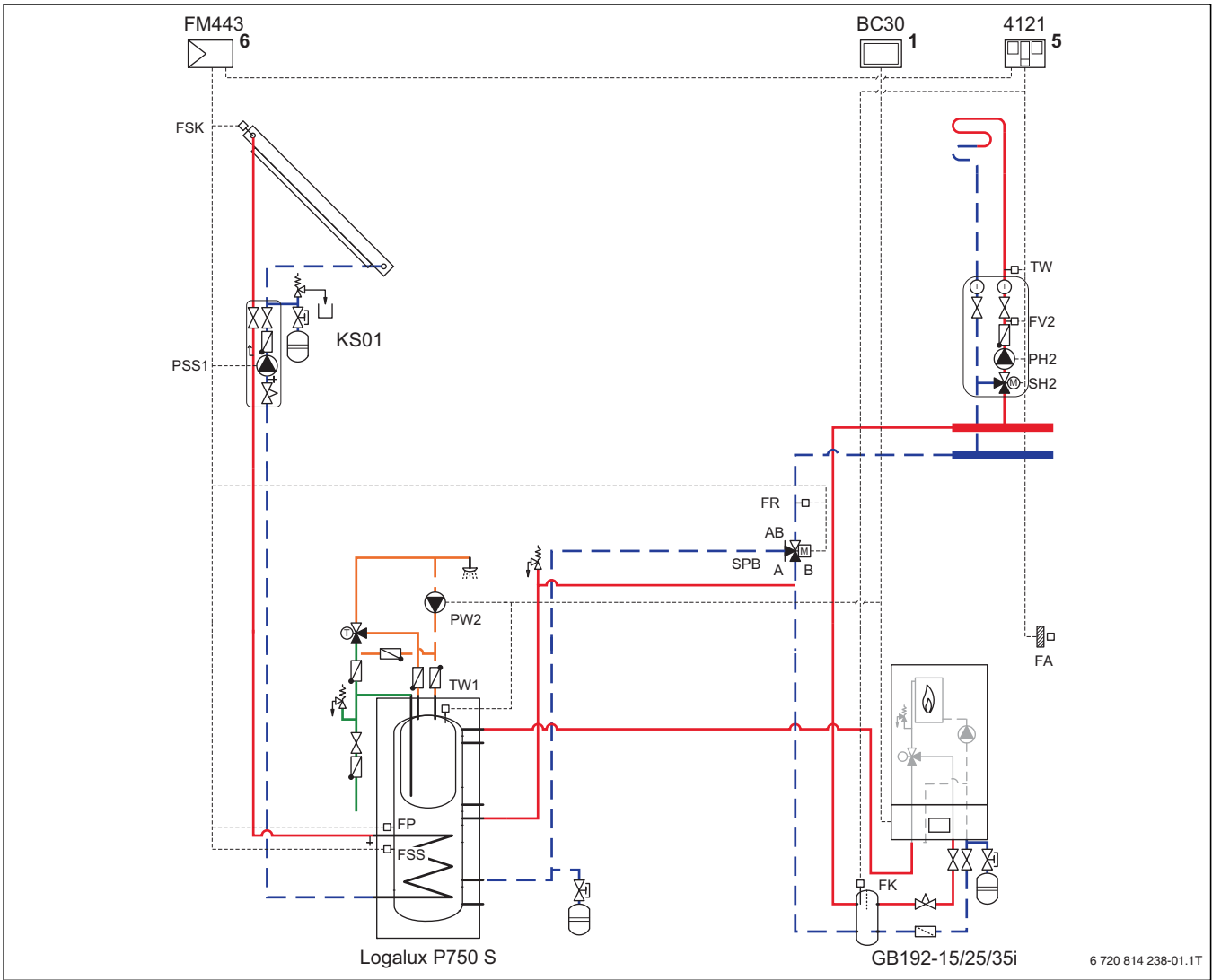
Bild 101 Anlagenschema mit Regelung (unverbindliche Prinzipdarstellung)
