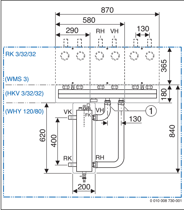
Bild 123 Abmessungen der Schnellmontage-Systemkombinationen RK 3/32/32 für 3 Heizkreise (Maße in mm)
