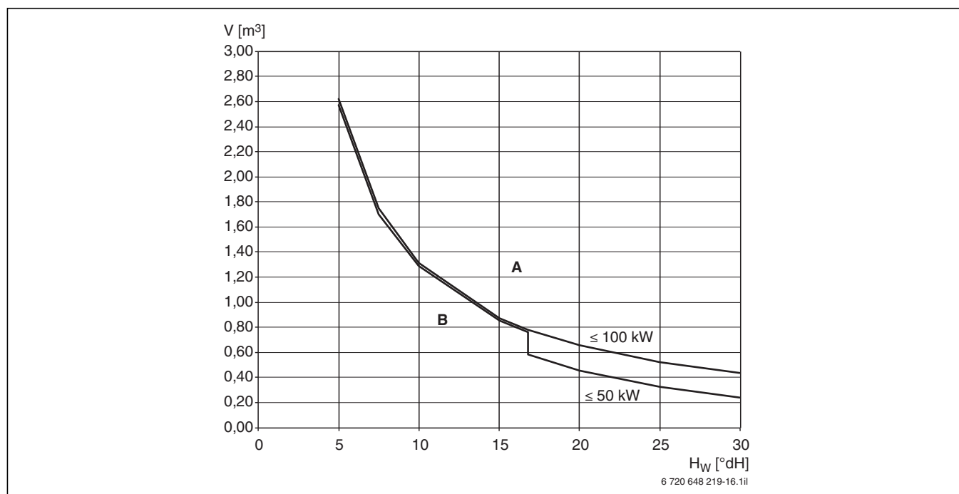
Bild 77 Grenzen zur Wasserbehandlung bei 1-Kessel-Anlagen \leq 50 \text{ kW} und \leq 100 \text{ kW}
