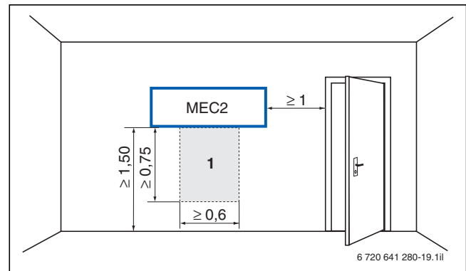
Bild 66 Position des Wandhalters für die Bedieneinheit MEC2 im Referenzraum (Maße in m)
