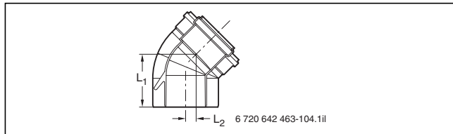
Bild 205 Konzentrischer Bogen Ø 80/125 (Maße → Tabelle 99)
