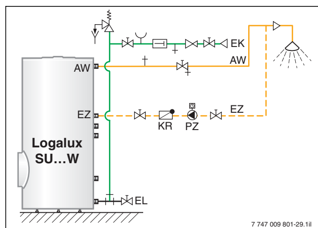
Bild 71 Variante einer Zirkulationsleitung für die Warmwasserspeicher Logalux SU... W
