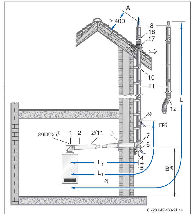
Bild 167 Montagevariante mit dem Bausatz GAF-K (Maße in mm)
