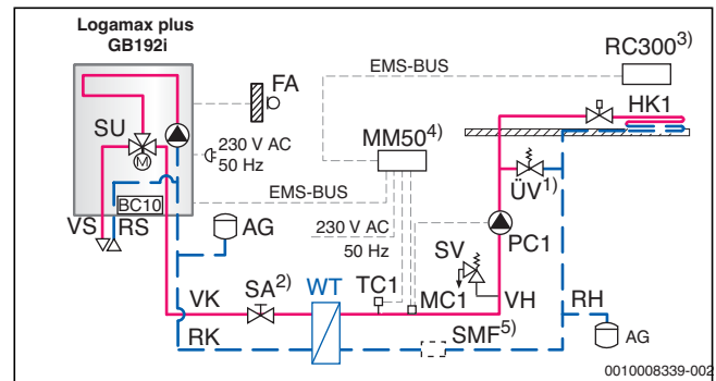
Bild 80 Beispiel für eine Fußbodenheizung mit Systemtrennung über einen Wärmetauscher bei nicht sauerstoffdichten Rohren (Abkürzungsverzeichnis → Seite 70)
