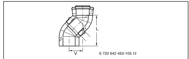
Bild 208 Versatzmaße konzentrischer Bogen Ø 80/125 (Maße → Tabelle 100)
