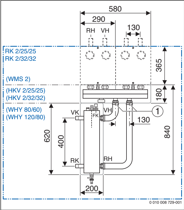
Bild 122 Abmessungen der Schnellmontage-Systemkombinationen RK 2/25/25 und RK 2/32/32 für zwei Heizkreise (Maße in mm)
