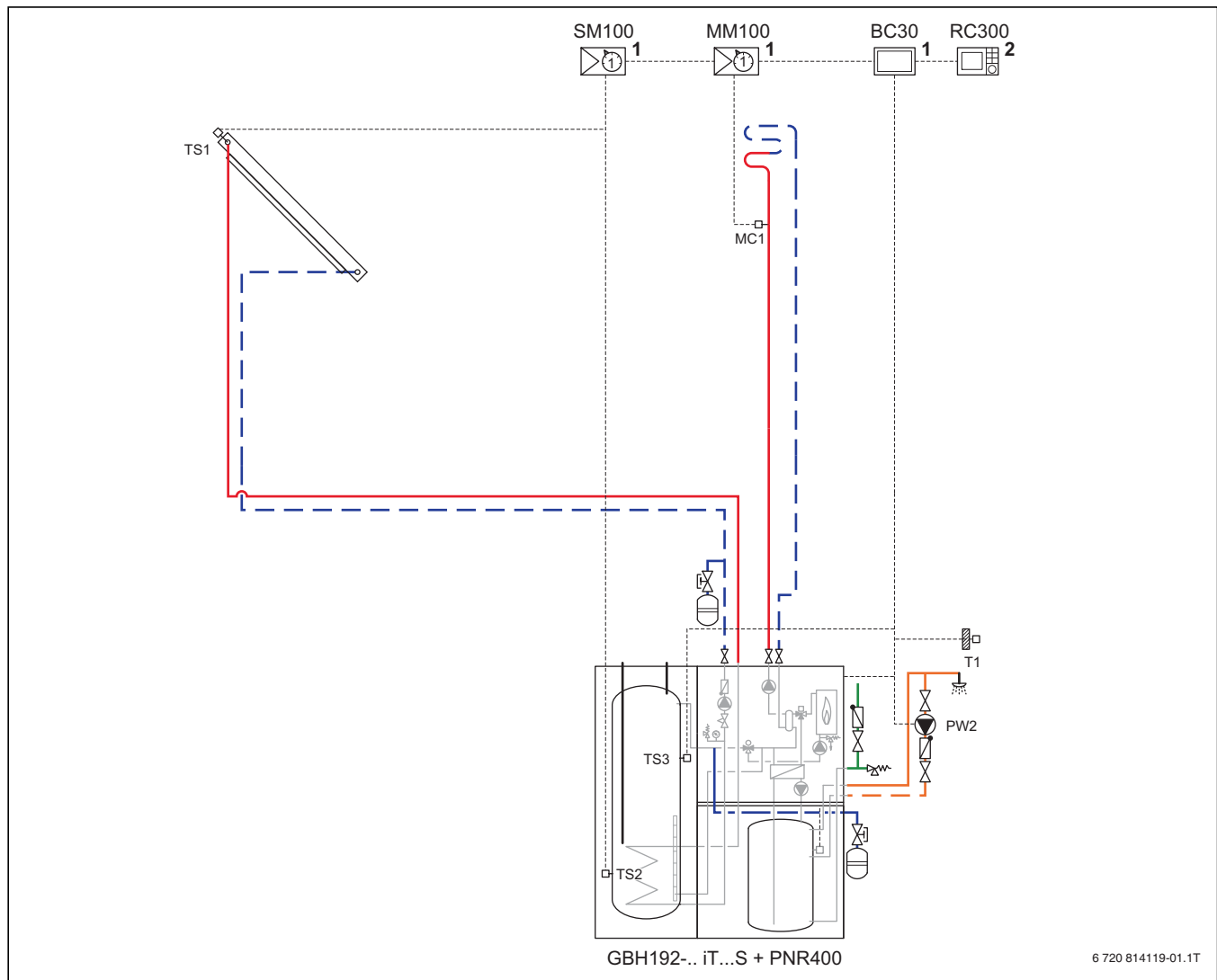
Bild 118 Anlagenschema mit Regelung (unverbindliche Prinzipdarstellung)
