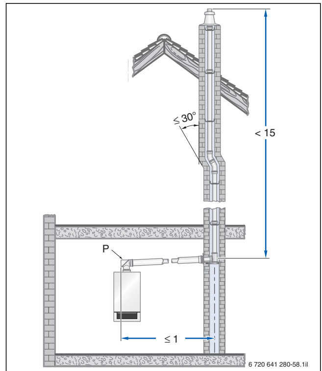
Bild 147 Beispiel zur Anordnung der Prüföffnung (P) bei einer waagerechten Abgasleitung ohne Umlenkung im Aufstellraum (Maße in m)
