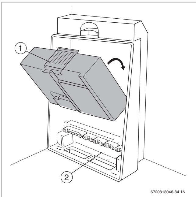
Bild 46 Einbau in wandhängendes Gas-Brennwertgerät
