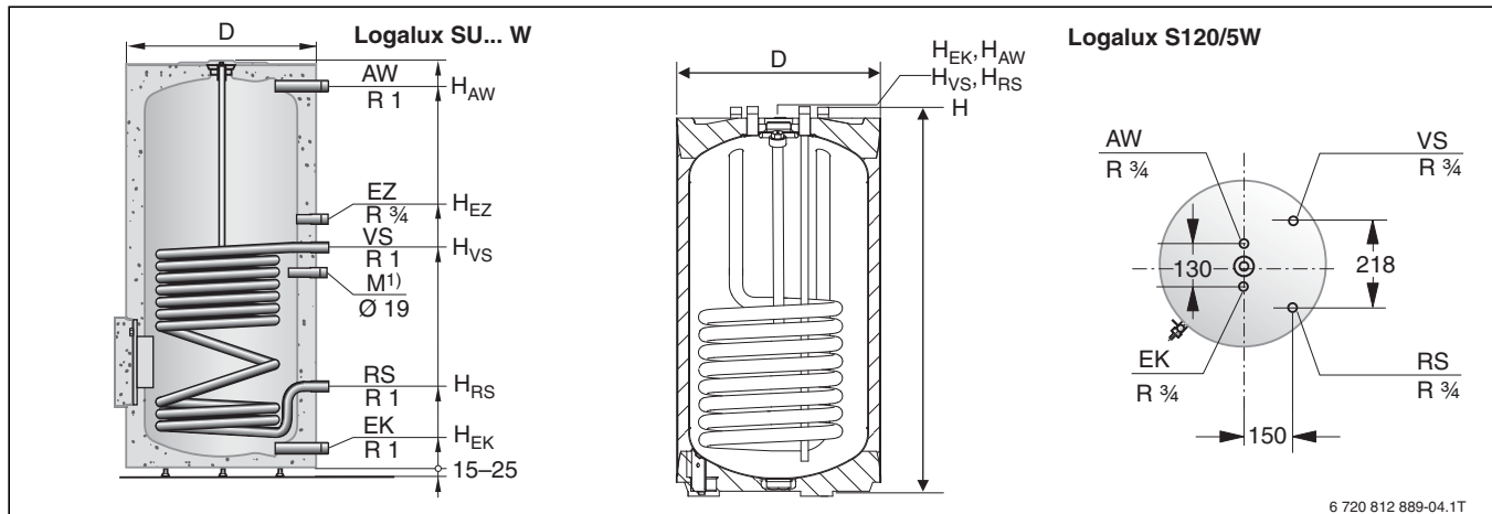
Bild 31 Abmessungen und Anschlüsse Logalux S120/5W und SU.../5W (Maße in mm)
