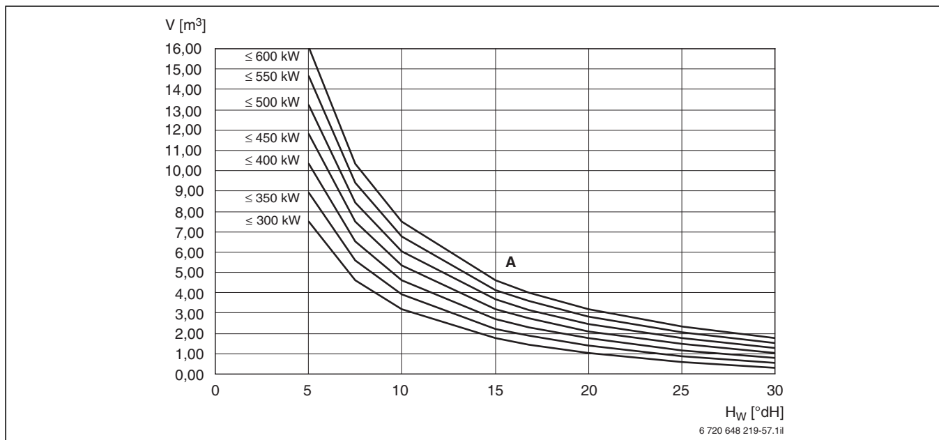
Bild 78 Grenzen zur Wasserbehandlung bei Mehr-Kessel-Kaskaden
