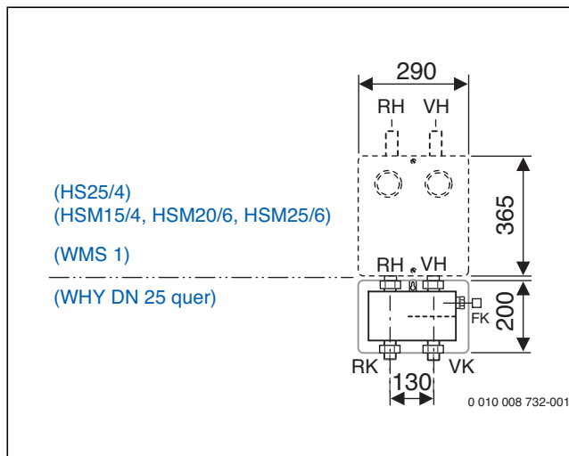
Bild 125 Abmessungen der Systemkombination mit hydraulischer Weiche quer zur direkten Verbindung mit einem Heizkreis-Anschluss-Set für einen Heizkreis (Maße in mm)
