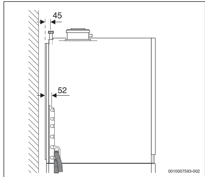
Bild 26 Anschlussmaße des Zubehörs Heizkreiserweiterung 2 (Maße in mm)
