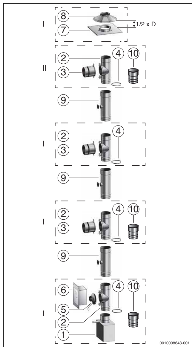
Bild 173 Bauteile des Bausatzes Mehrfachbelegung
