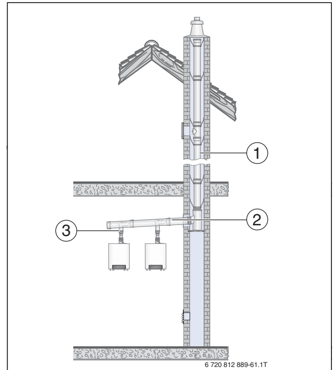
Bild 174 Baussatz Kaskade RLU
