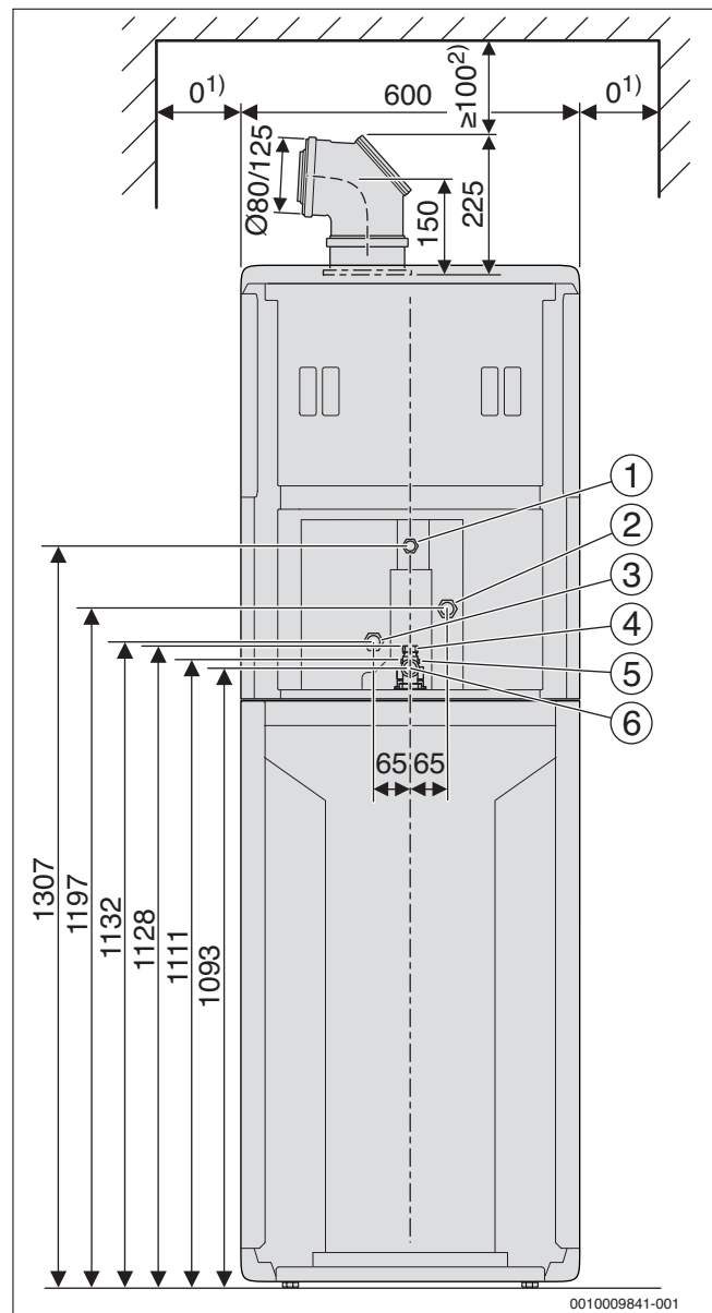
Bild 19 Abmessungen und Anschlüsse ohne Zubehör, Rückansicht, (Maße in mm)
