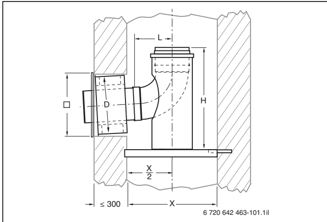
Bild 191 Schornsteinanschluss (Maße in mm)
