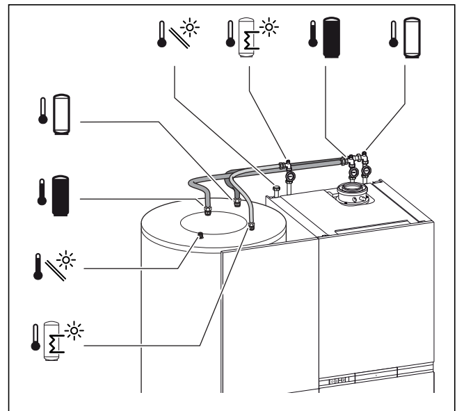
Bild 37 Anschluss mit Verbindungsleitung Puffer (CS18)
