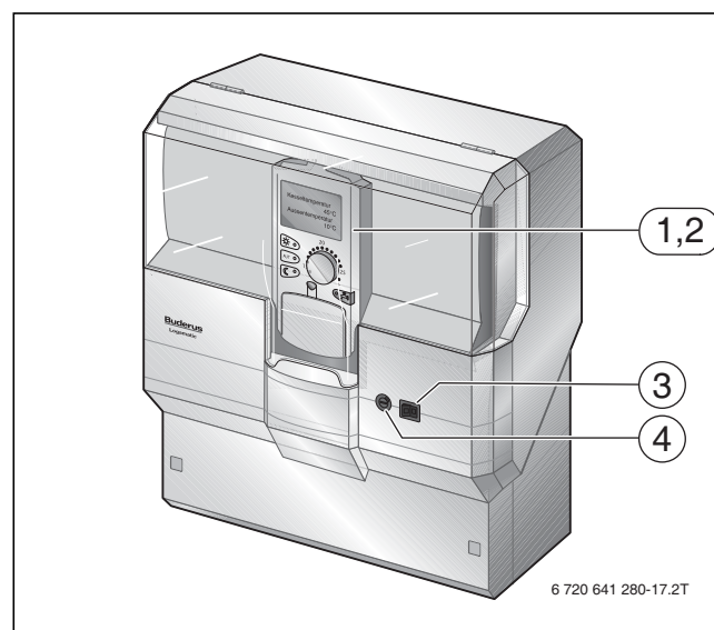
Bild 64 Regelgerät Logamatic 4122 in Grundausstattung als Variante mit Bedieneinheit MEC2; wahlweise mit Display erhältlich
