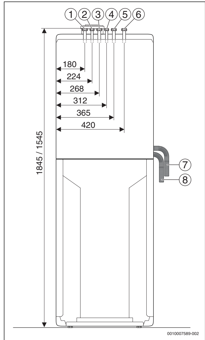
Bild 21 Anschlussmaße des Zubehörs AS-V1/Vertikales Anschluss-Set (Maße in mm)
