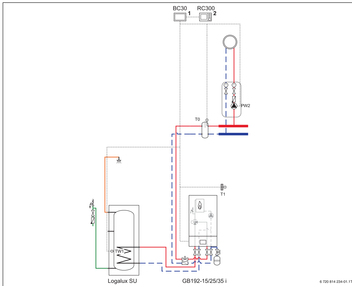
Bild 93 Anlagenschema mit Regelung (unverbindliche Prinzipdarstellung)
