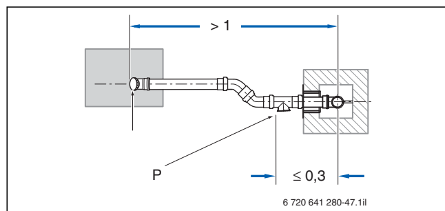
Bild 131 Beispiel zur Anordnung der Prüföffnungen (P) bei einer waagerechten Abgasleitung mit Umlenkung im Aufstellraum – Draufsicht (Maße in m)
