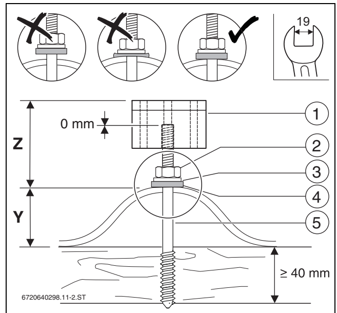
Bild 30 Montierte Stockschrabe mit Haltebock
