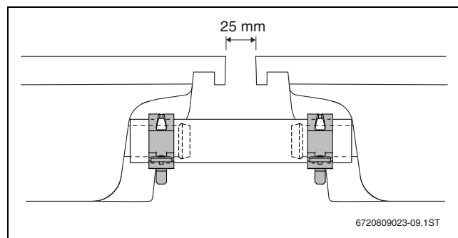
Bild 49 Kollektoren zusammengeschoben
