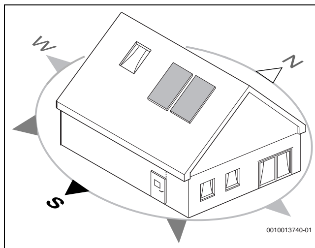
Bild 8 Kollektorfeld ausrichten
