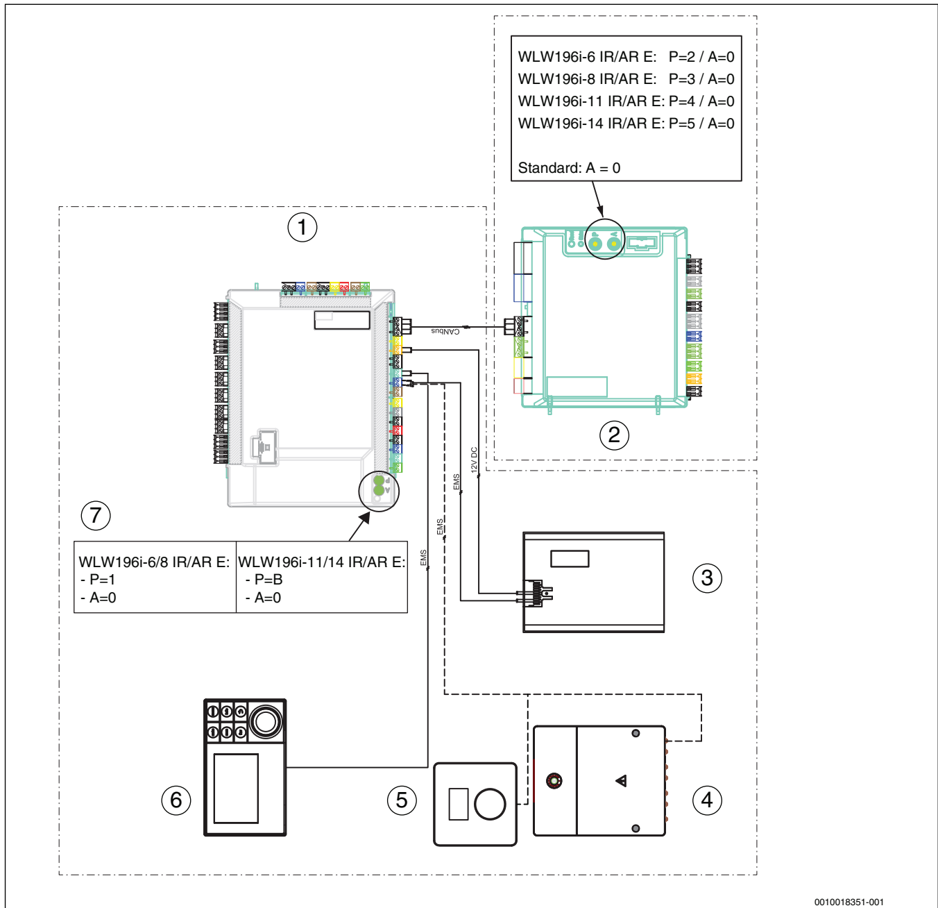
Bild 17 Kreisschema Wärmepumpenmodule
