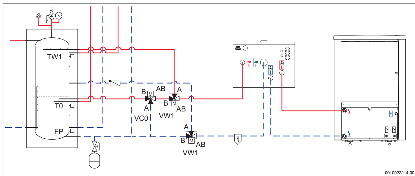
Bild 9 Hydraulische Verbindung zwischen Pufferspeicher, Inneneinheit und Wärmepumpeneinheit
