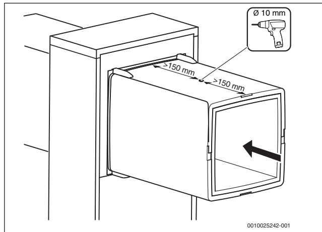
Bild 15 Montage des Referenzfühlers TL2 am Luftansaugkanal
