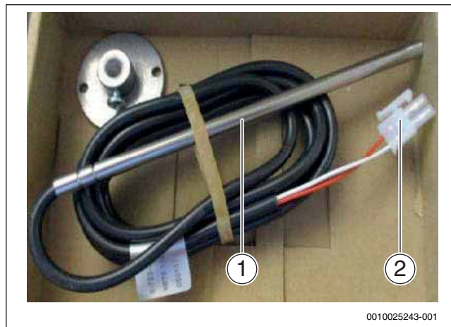
Bild 13 Referenzfühler TL2 mit Anschlusskabel
