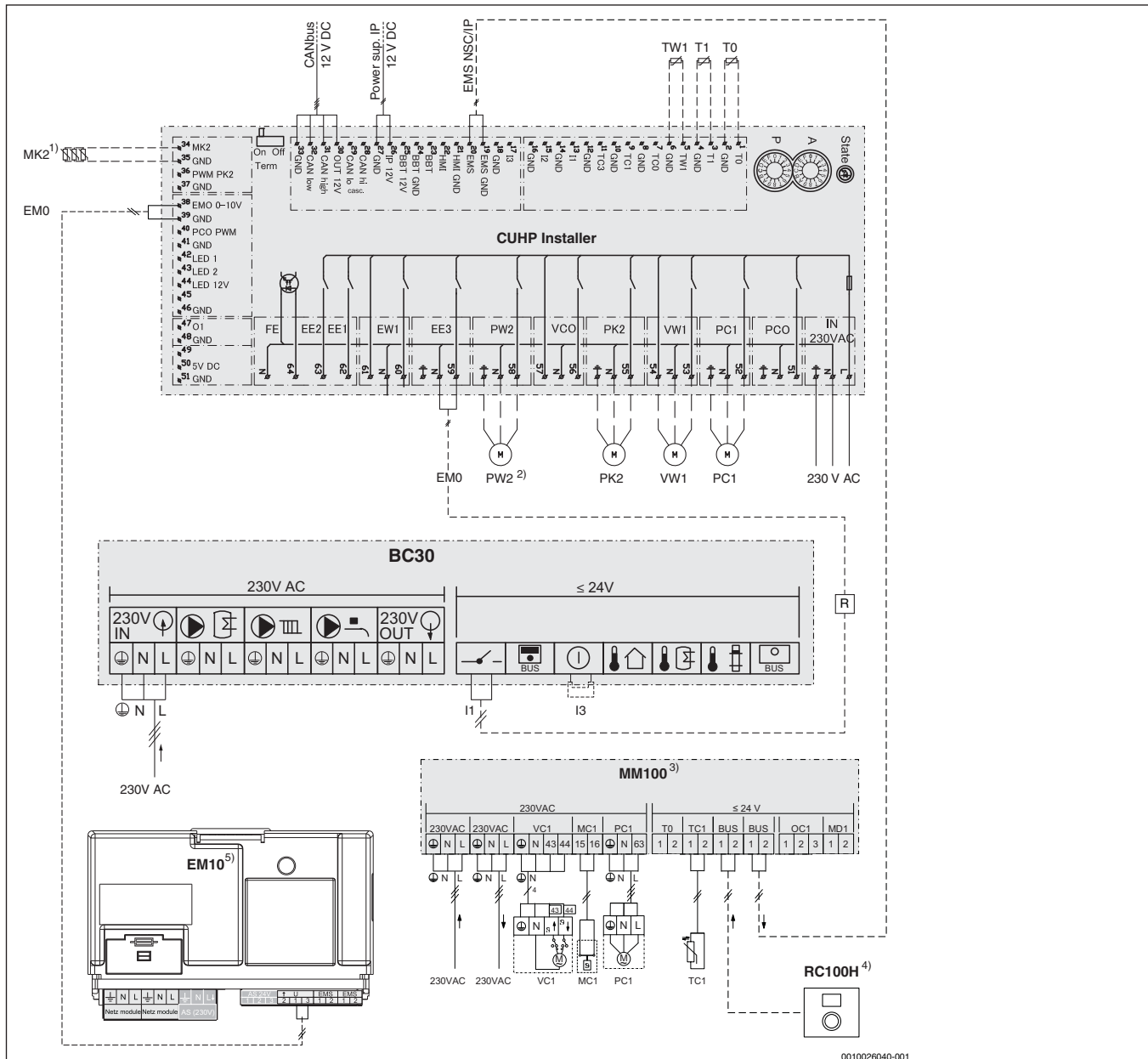
Bild 23 Schaltplan zum Anlagenbeispiel
