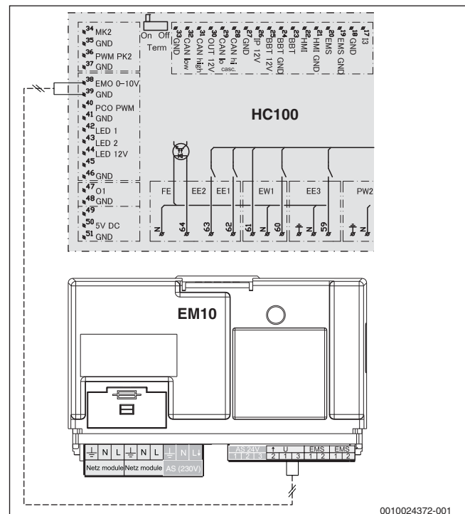
Bild 4 Schaltplan zur Anforderung über das Modul EM10
