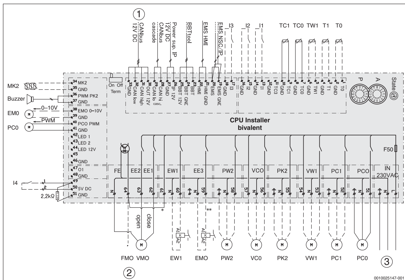
Bild 27 Schaltplan Installationsmodul WLW196i RB mit Mischer für den Anschluss einer externen Wärmequelle
