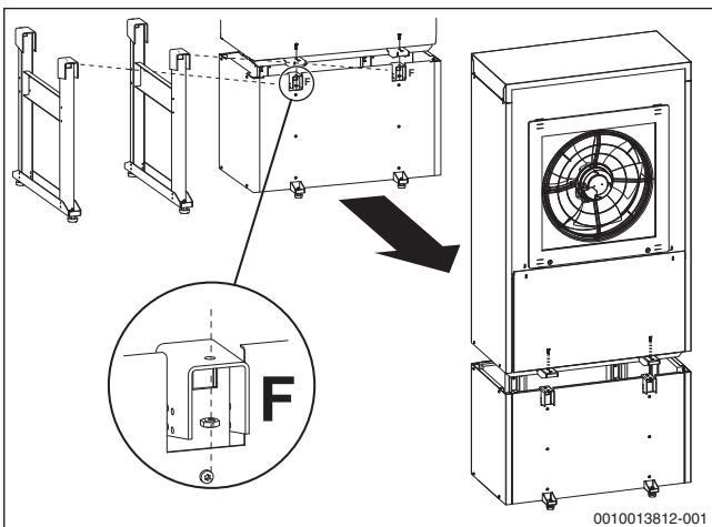
Bild 11 Wärmepumpe auf Sockel stellen
