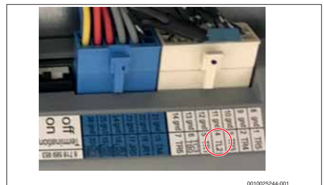
Bild 13 Referenzfühler TL2 an der I/O-Modul-Platine
