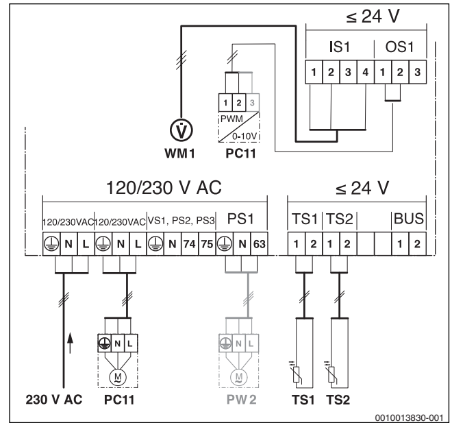
Bild 19 Anschlussklemmen FS20/2
