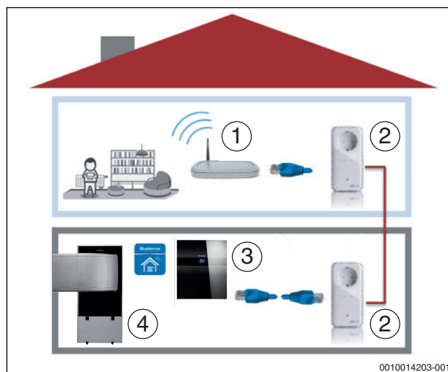
Bild 20 PowerLAN
