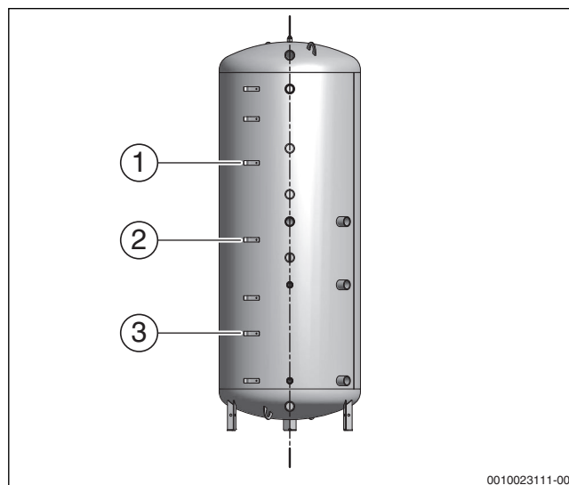
Bild 10 Empfohlene Fühlerpositionen des Pufferspeichers PNRZ,,
