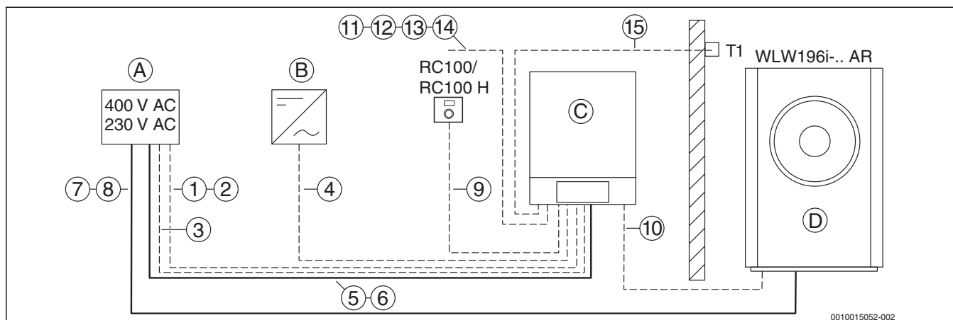
Bild 16 Kabelzugplan der elektrischen Leitungen bei Außenaufstellung (Prinzipdarstellung)
