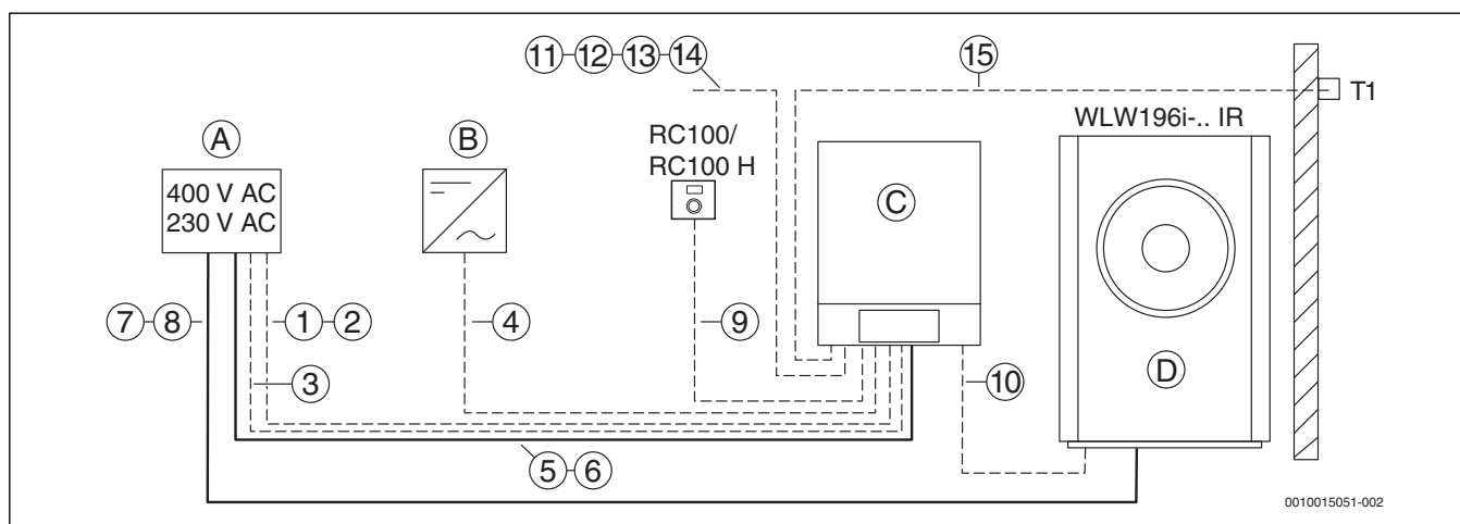
Bild 17 Kabelzugplan der elektrischen Leitungen bei Innenaufstellung (Prinzipdarstellung)
