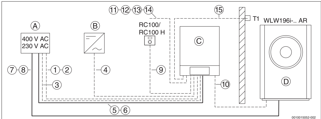
Bild 20 Kabelzugplan der elektrischen Leitungen bei Außenaufstellung (Prinzipdarstellung)
