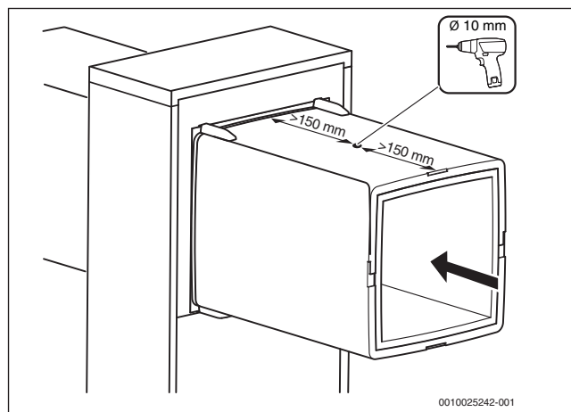
Bild 11 Montage des Referenzfühlers TL2 am Luftansaugkanal
