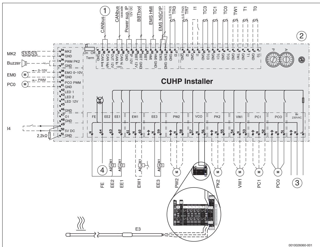
Bild 22 Schaltplan Installationsmodul HC100 mit Elektrozuheizer (IDUS E)
