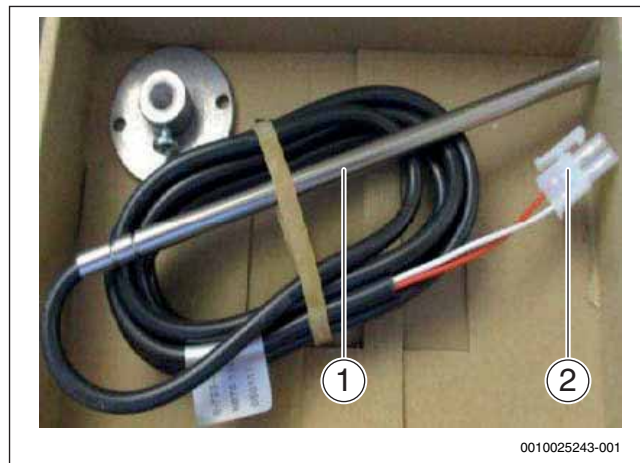
Bild 9 Referenzfühler TL2 mit Anschlusskabel
