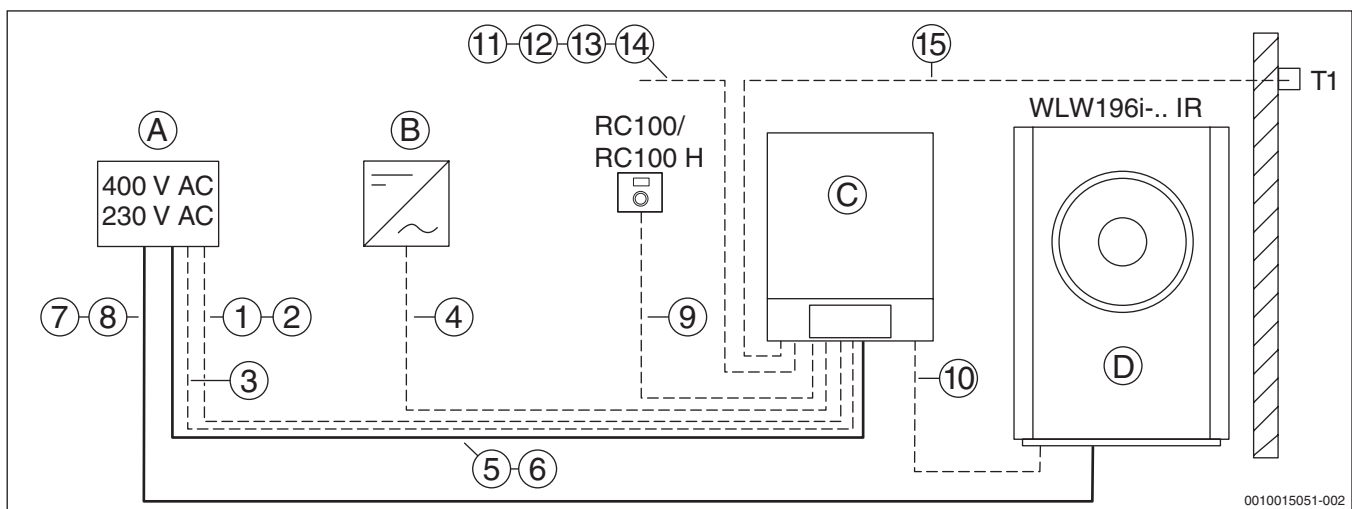
Bild 21 Kabelzugplan der elektrischen Leitungen bei Innenaufstellung (Prinzipdarstellung)
