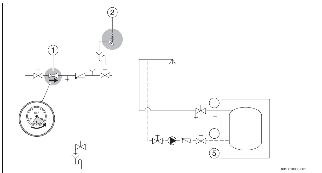
Bild 9 Hydraulischer Anschluss des Warmwasserspeichers
