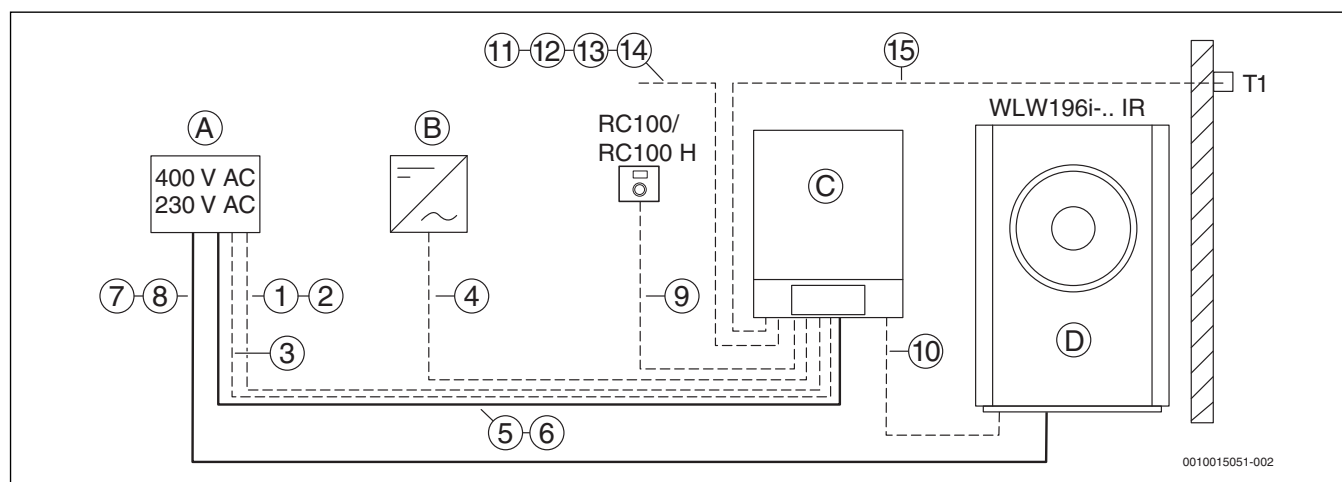
Bild 14 Kabelzugplan der elektrischen Leitungen bei Innenaufstellung (Prinzipdarstellung)
