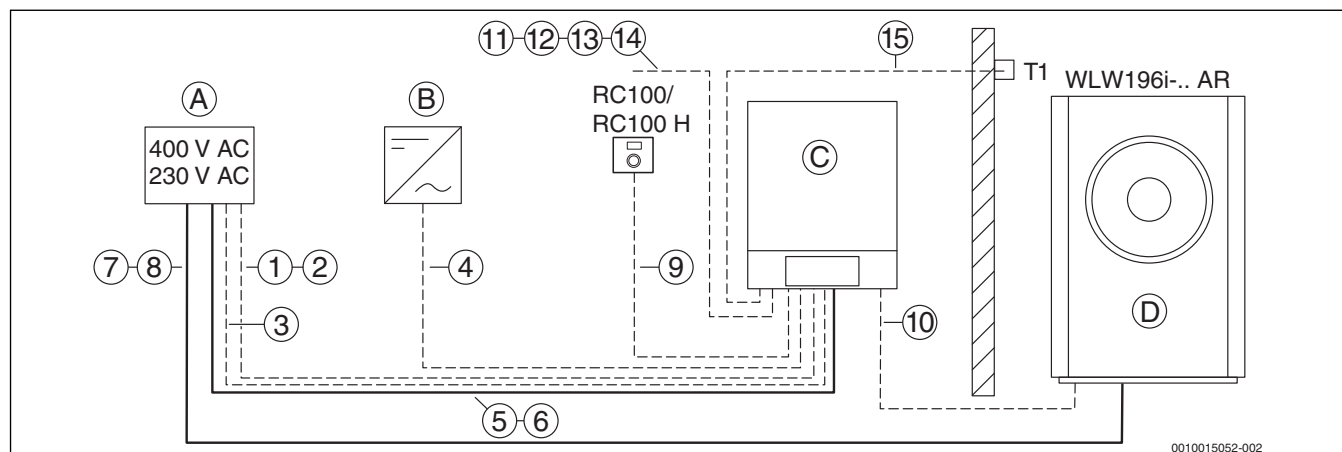
Bild 13 Kabelzugplan der elektrischen Leitungen bei Außenaufstellung (Prinzipdarstellung)
