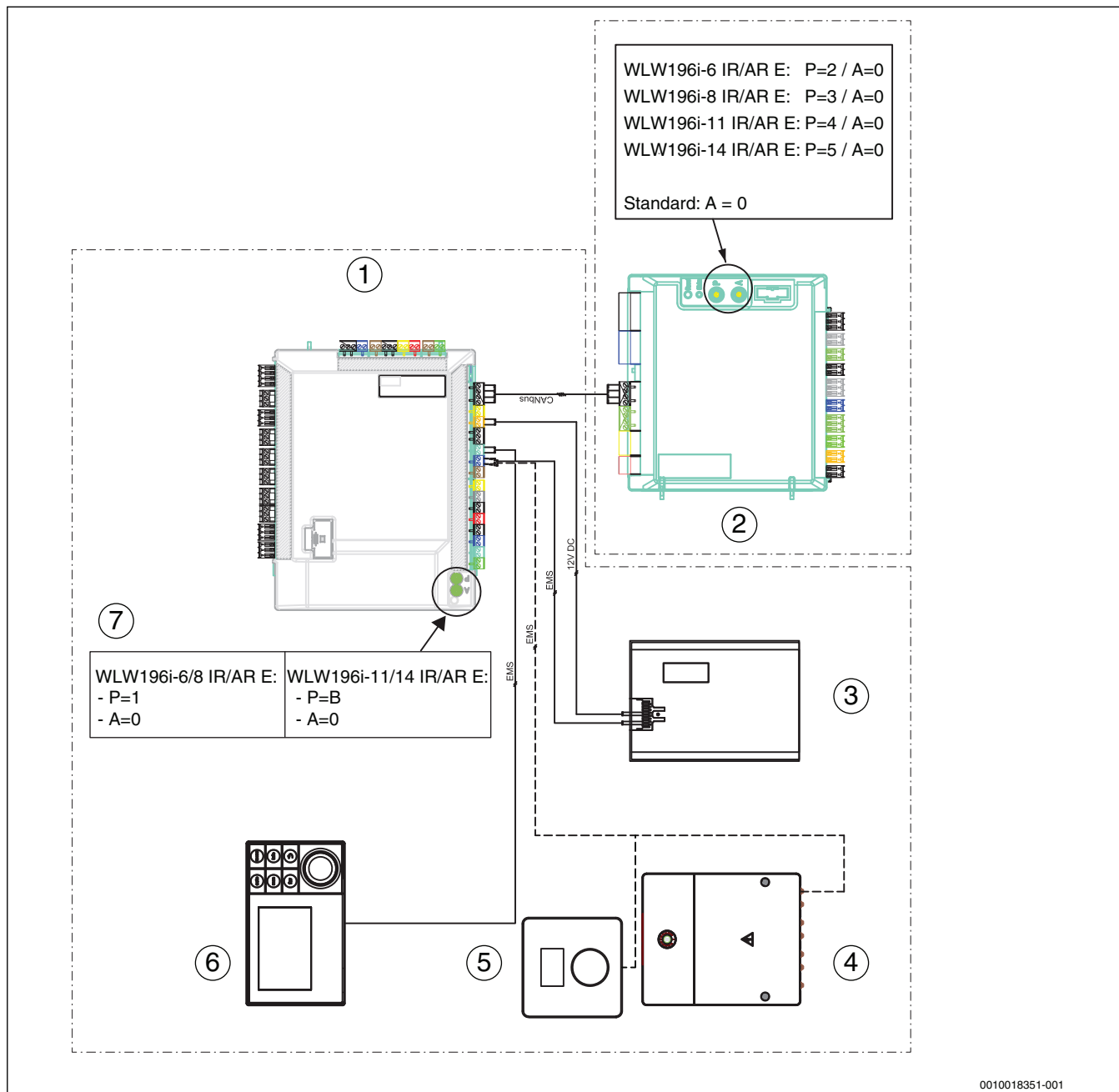
Bild 12 Kreisschema Wärmepumpenmodule
