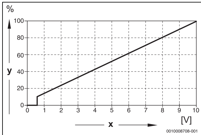
Bild 27 0...10-V-Eingang Leistung
