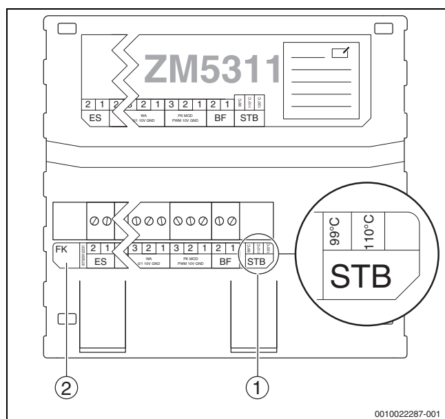
Bild 22 Elektronischer Sicherheitstemperaturbegrenzer beim ZM5311
