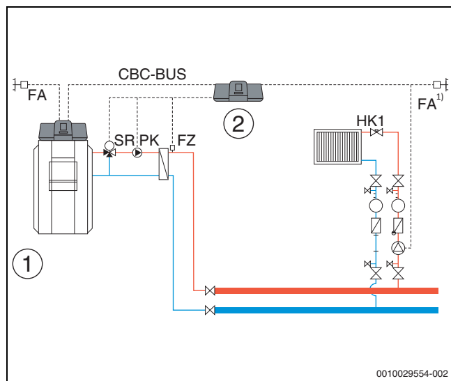
Bild 31 Variante 1: Unterstation mit Vormischfunktion, Kompensation Wärmeverluste über FZ, Lastbegrenzung
