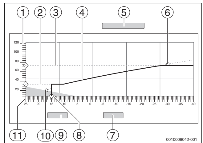
Bild 41 Heizkurve
