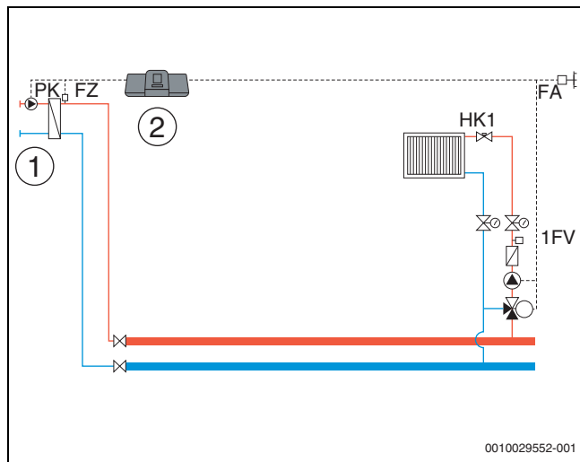
Bild 29 Variante 2: Fremde Wärmequelle ohne Zubringerpumpe, Lastbegrenzung und Kompensation Wärmeverluste über FZ
