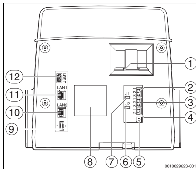
Bild 21 Rückseite Bedieneinheit
