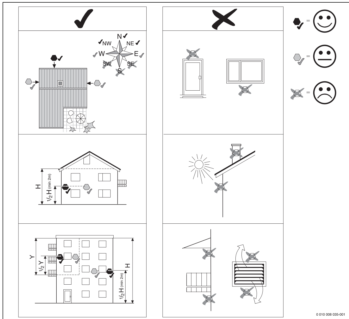
Bild 8 Außentemperaturfühler montieren
