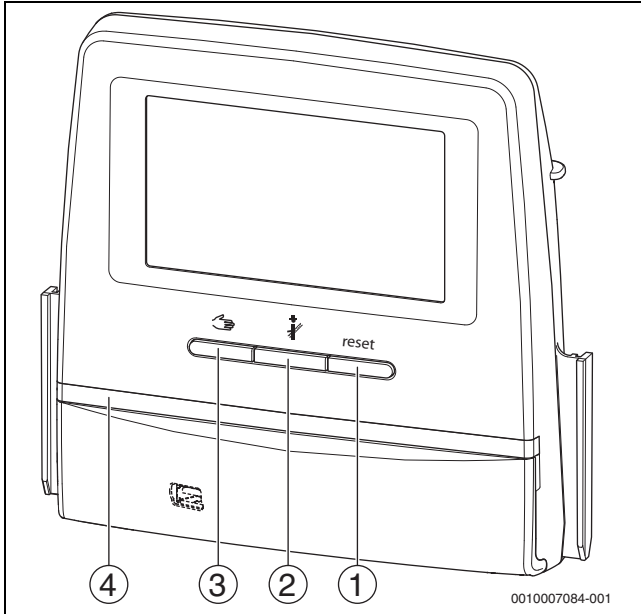
Bild 18 Funktionstasten
