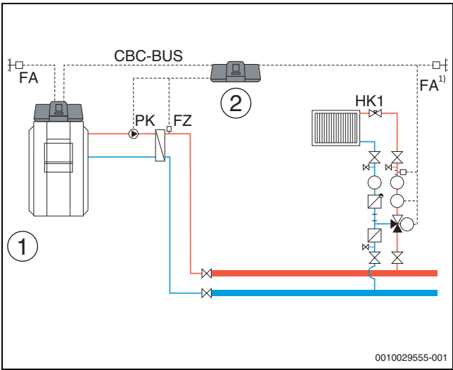
Bild 32 Variante 2: Unterstation mit Kompensation Wärmeverluste über FZ, Lastbegrenzung
