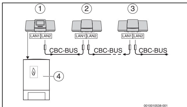
Bild 43 Regelgeräteanbindung
