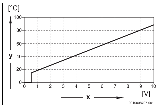
Bild 26 0...10-V-Eingang Temp.
