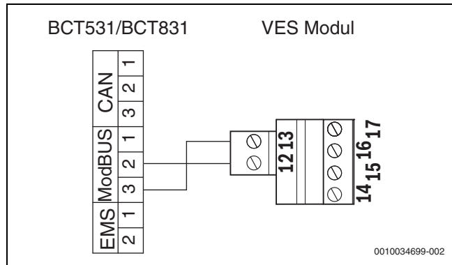
Bild 35 Anschluss des Regelgeräts an das VES Modul
