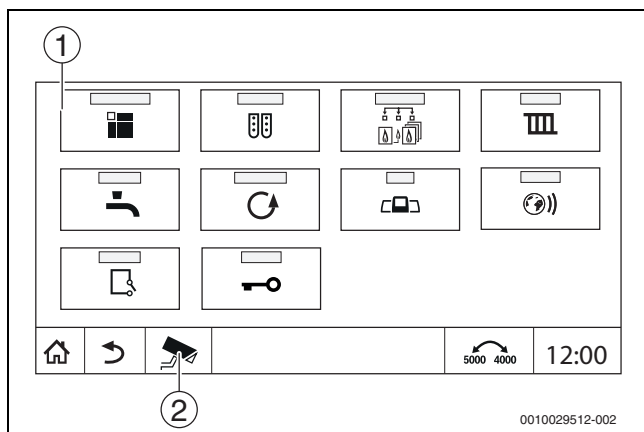
Bild 17 Servicemenü (Beispiel)
