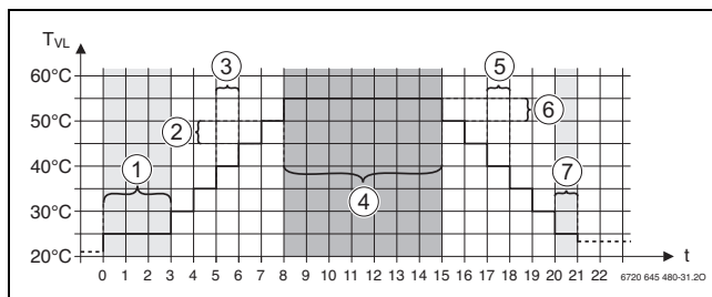
Bild 42 Estrichtrocknung
