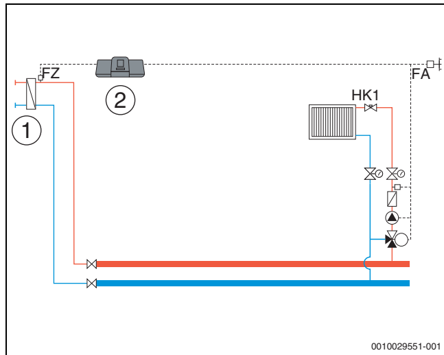
Bild 28 Variante 1: Fremde Wärmequelle mit Zubringerpumpe, Lastbegrenzung und Kompensation Wärmeverluste über FZ
