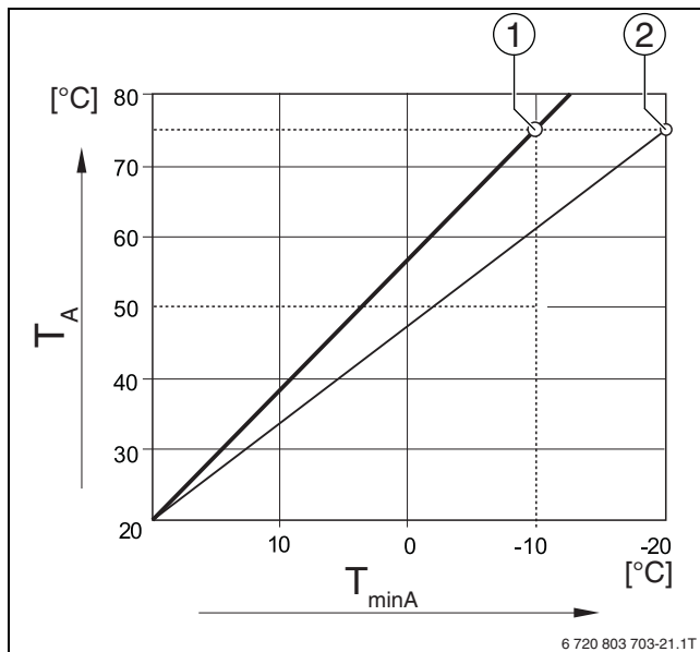
Bild 25 Einstellung der Heizkurve: Einstellung der Steigung über Auslegungstemperatur und minimale Außentemperatur
