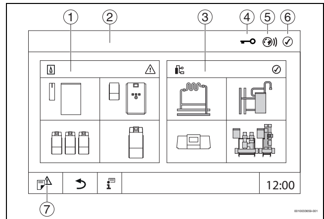
Bild 9 Systemübersicht (Beispiel)
