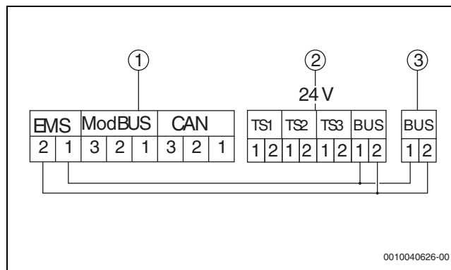
Bild 5 Elektrischer Anschluss
