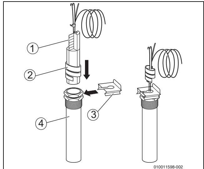
Bild 7 Kunststoffspirale in Tauchhülse einsetzen@@
