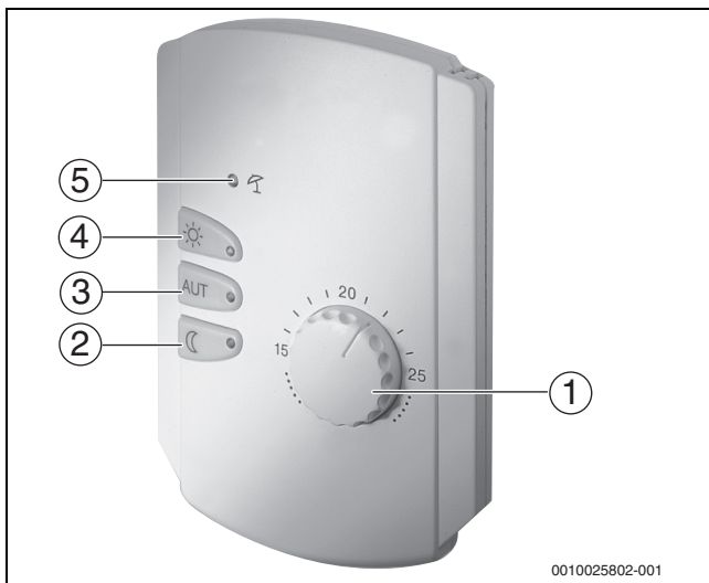
Bild 37 Fernbedienung
