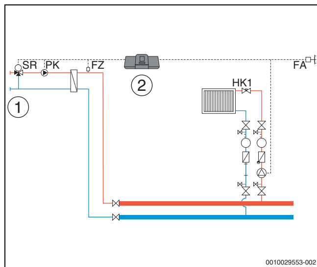
Bild 30 Variante 3: Fremde Wärmequelle ohne Zubringerpumpe, Lastbegrenzung, Vormischfunktion, Kompensation Wärmeverluste über FZ
