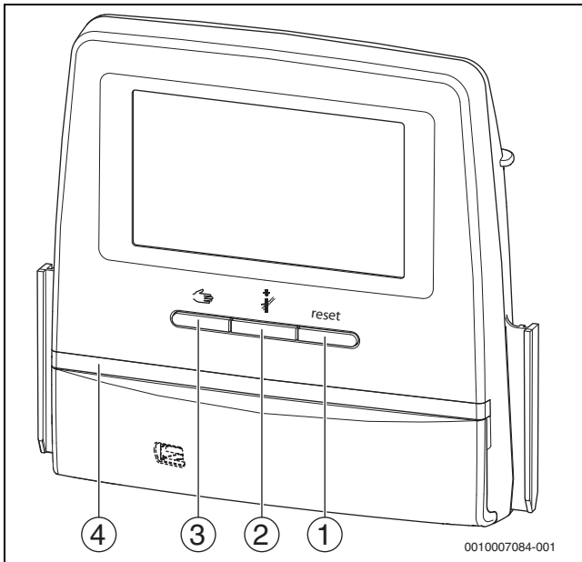
Bild 15 Funktionstasten
