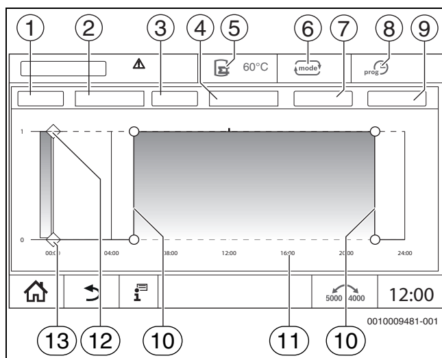
Bild 29 Zirkulationsprogramm
