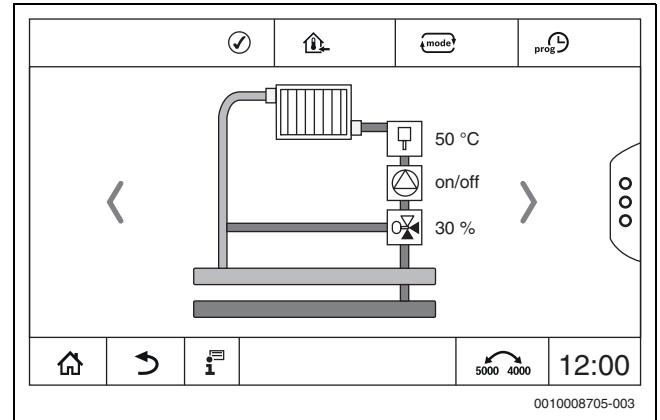
Bild 12 Heizkreisansicht Serie 5000
